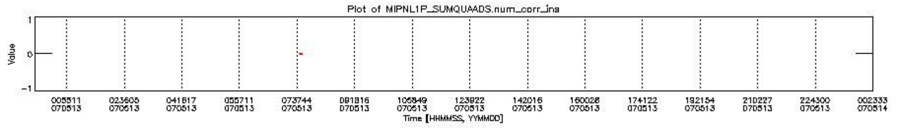
mipas_daily_report_level1_OFL_MIPAS_4_67_P_20070513_4.PNG
