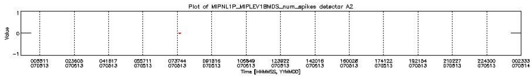
mipas_daily_report_level1_OFI_MIPAS_4_67_P_20070513_18.PNG
