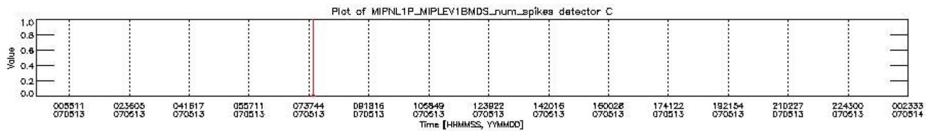
mipas_daily_report_level1_OFL_MIPAS_4_67_P_20070513_24.PNG
