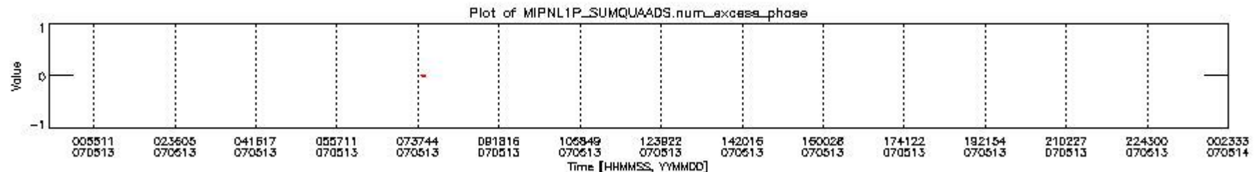
mipas_daily_report_level1_OFI_MIPAS_4_67_P_20070513_8.PNG
