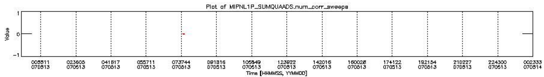
mipas_daily_report_level1_OFL_MIPAS_4_67_P_20070513_2.PNG
