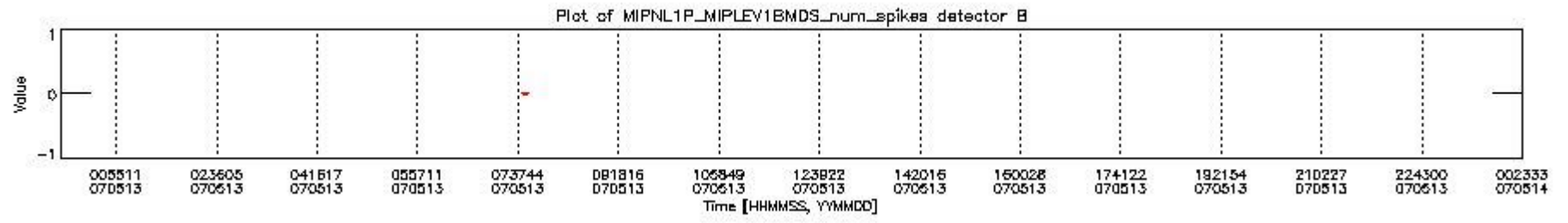
mipas_daily_report_level1_OFL_MIPAS_4_67_P_20070513_22.PNG
