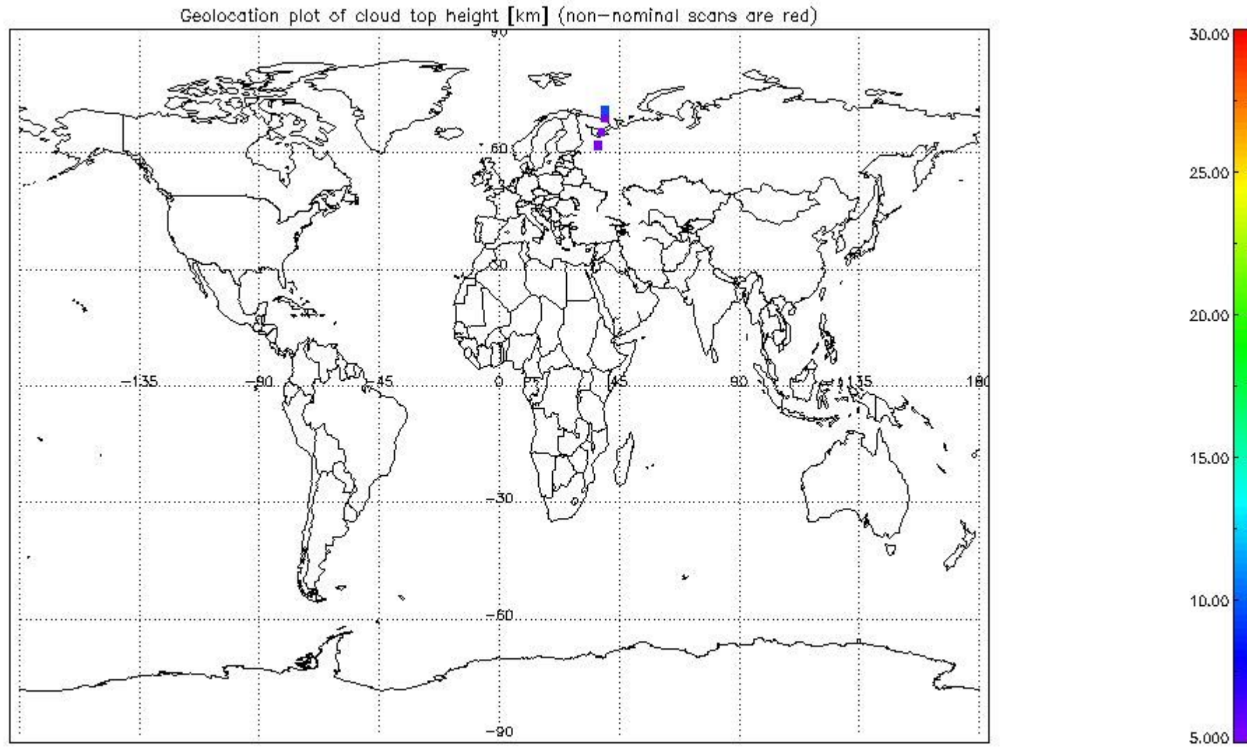
mipas_daily_report_level1_OFL_MIPAS_4_67_P_20070513_51.PNG
