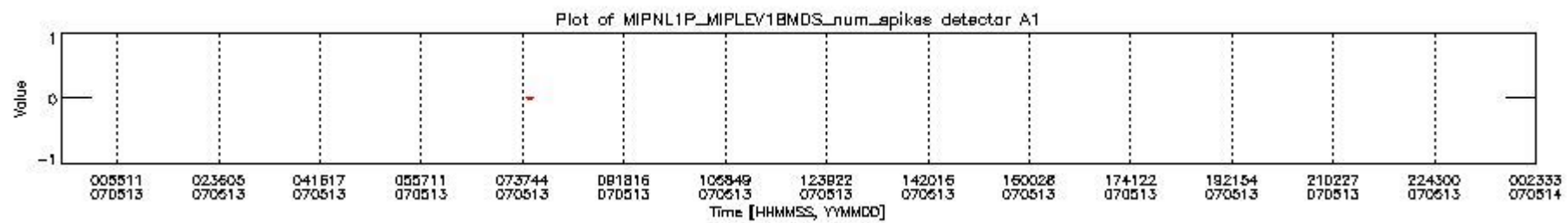
mipas_daily_report_level1_OFL_MIPAS_4_67_P_20070513_16.PNG
