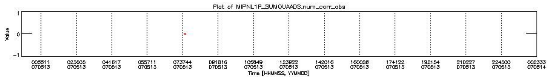
mipas_daily_report_level1_OFL_MIPAS_4_67_P_20070513_6.PNG
