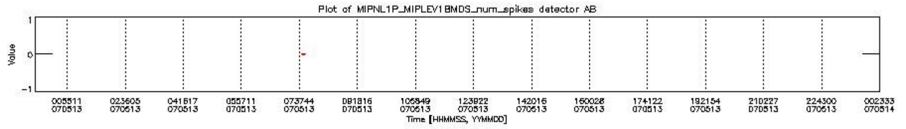
mipas_daily_report_level1_OFL_MIPAS_4_67_P_20070513_20.PNG
