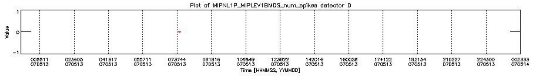
mipas_daily_report_level1_OFL_MIPAS_4_67_P_20070513_26.PNG
