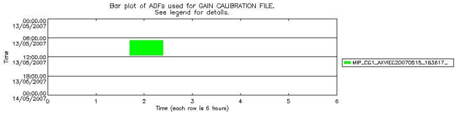
mipas_daily_report_level1_OFI_MIPAS_4_67_P_20070513_54.PNG
