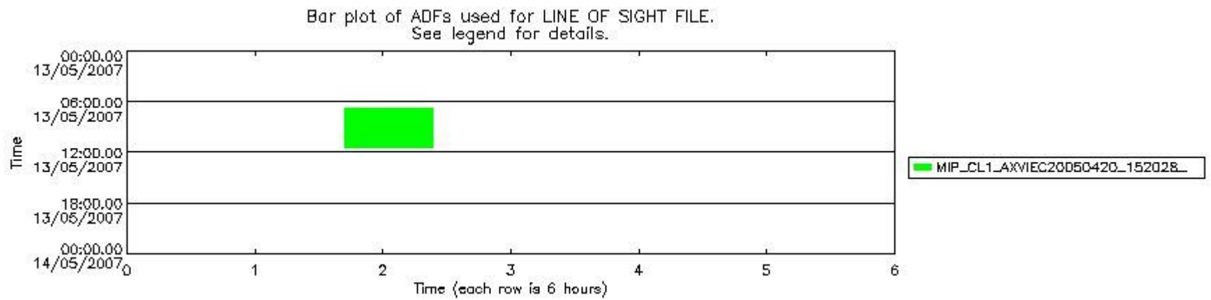
mipas_daily_report_level1_OFI_MIPAS_4_67_P_20070513_55.PNG
