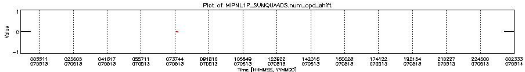
mipas_daily_report_level1_OFL_MIPAS_4_67_P_20070513_10.PNG
