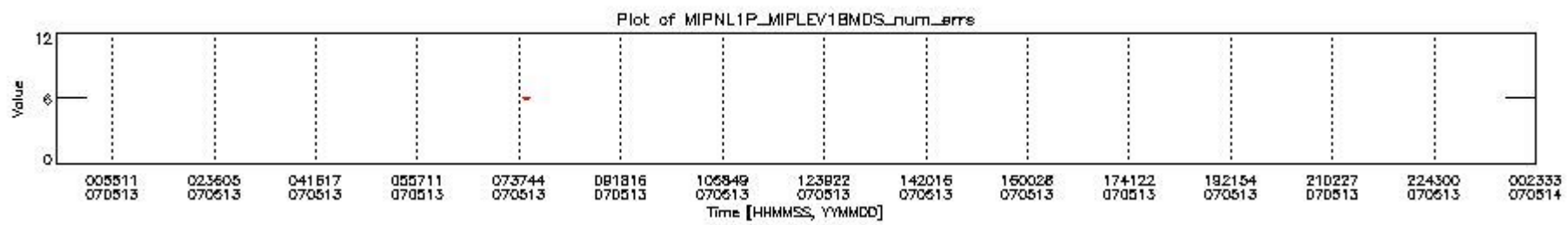
mipas_daily_report_level1_OFL_MIPAS_4_67_P_20070513_28.PNG
