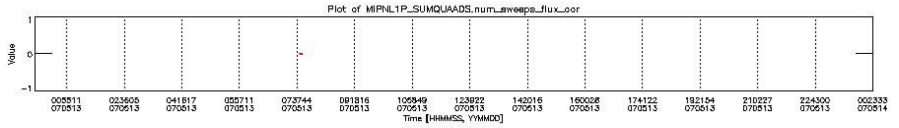
mipas_daily_report_level1_OFL_MIPAS_4_67_P_20070513_12.PNG
