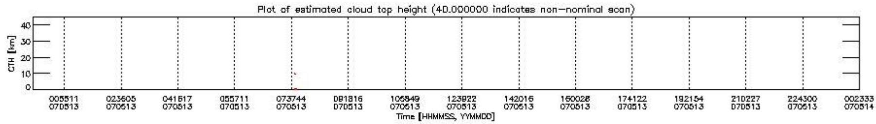
mipas_daily_report_level1_OFL_MIPAS_4_67_P_20070513_51.PNG
