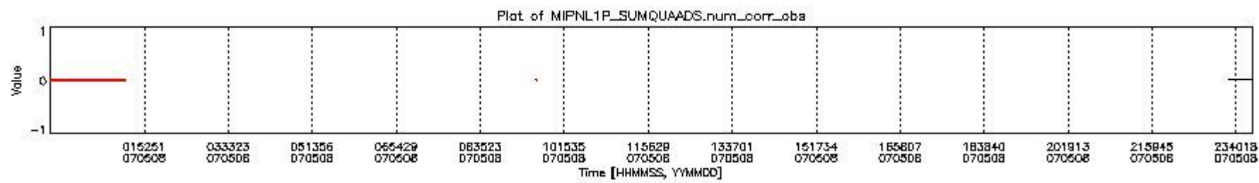
mipas_daily_report_level1_OFI_MIPAS_4_67_P_20070508_6.PNG
