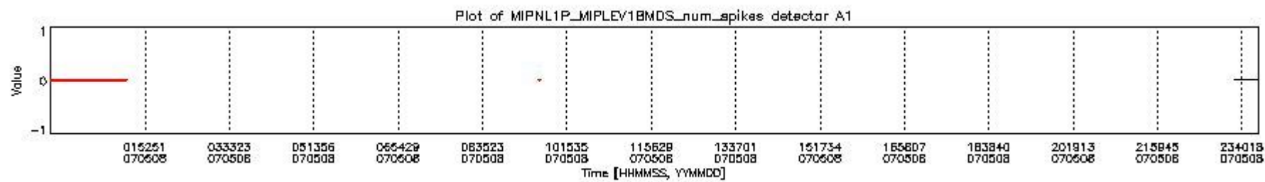
mipas_daily_report_level1_OFL_MIPAS_4_67_P_20070508_16.PNG
