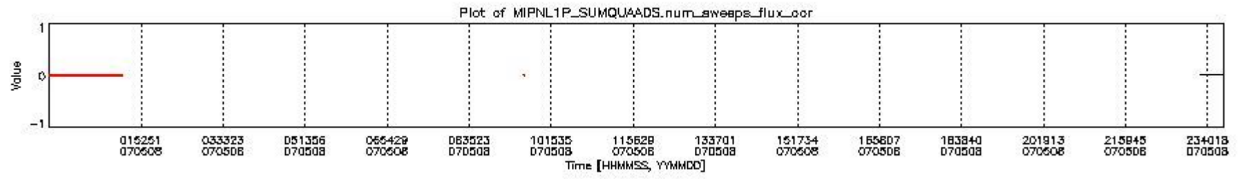
mipas_daily_report_level1_OFL_MIPAS_4_67_P_20070508_12.PNG
