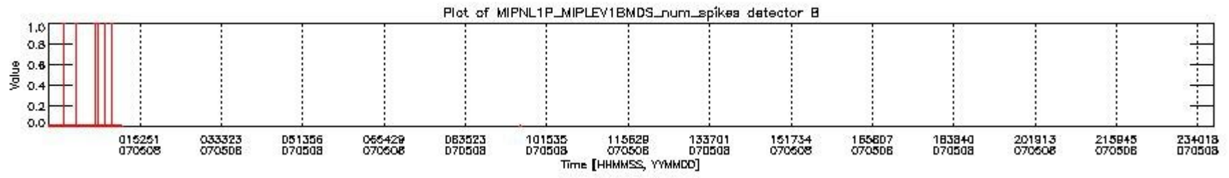
mipas_daily_report_level1_OFI_MIPAS_4_67_P_20070508_22.PNG
