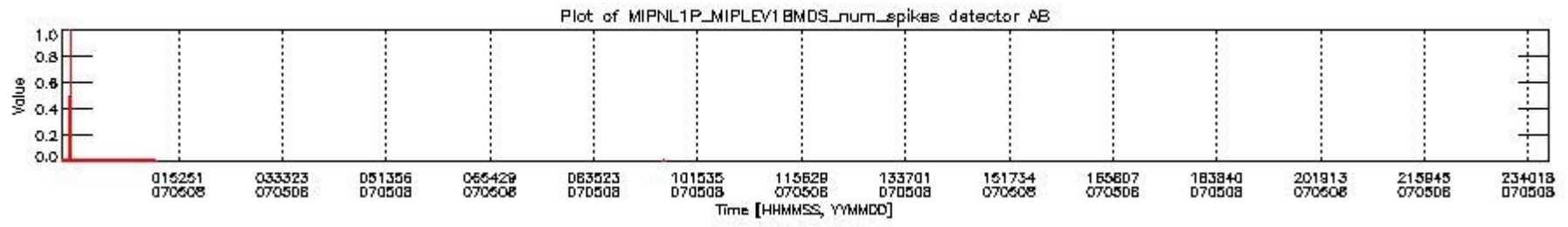
mipas_daily_report_level1_OFI_MIPAS_4_67_P_20070508_20.PNG
