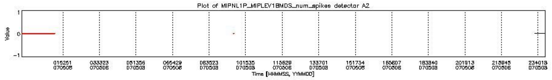
mipas_daily_report_level1_OFI_MIPAS_4_67_P_20070508_18.PNG
