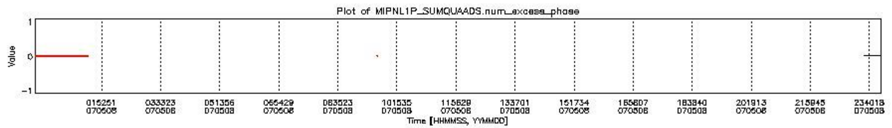
mipas_daily_report_level1_OFI_MIPAS_4_67_P_20070508_8.PNG
