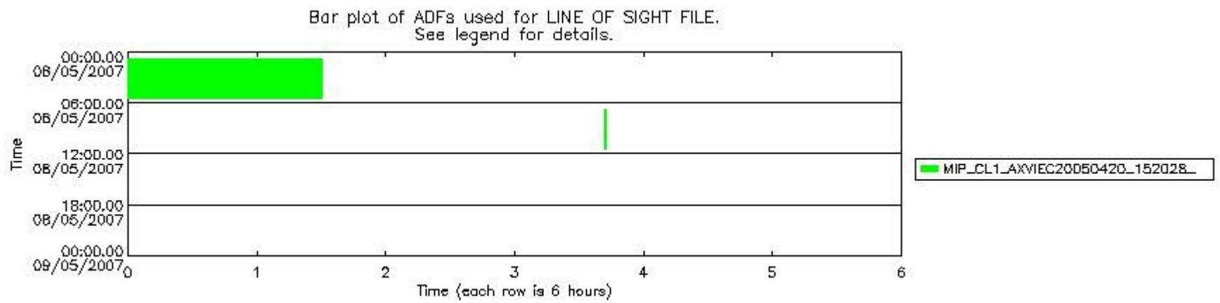
mipas_daily_report_level1_OFL_MIPAS_4_67_P_20070508_55.PNG
