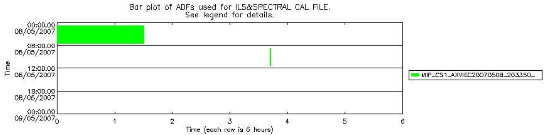
mipas_daily_report_level1_OFL_MIPAS_4_67_P_20070508_53.PNG
