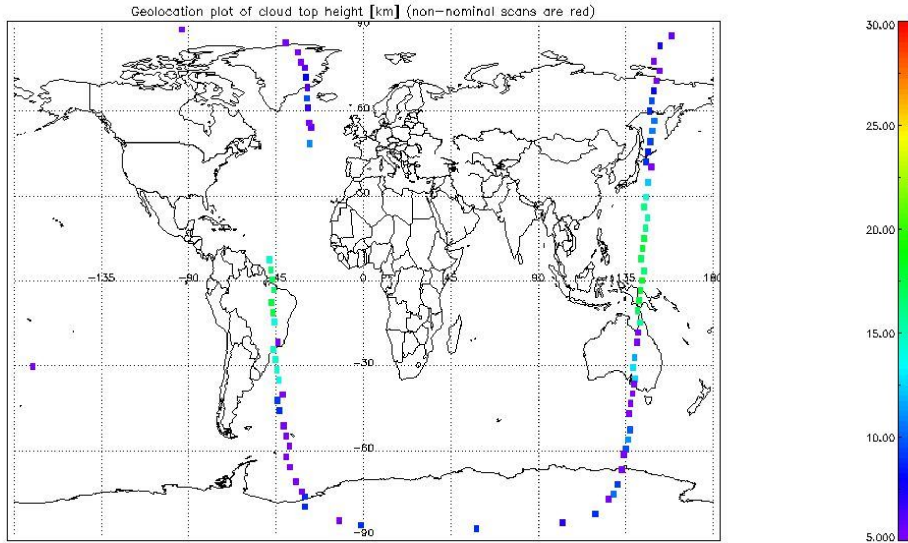
mipas_daily_report_level1_OFL_MIPAS_4_67_P_20070508_51.PNG
