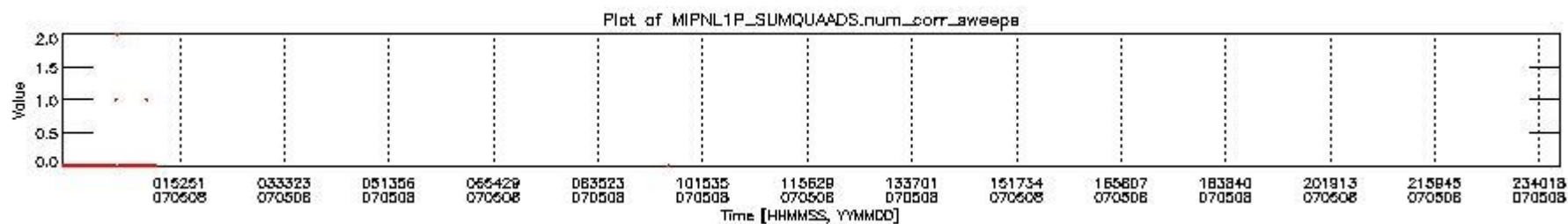
mipas_daily_report_level1_OFL_MIPAS_4_67_P_20070508_2.PNG
