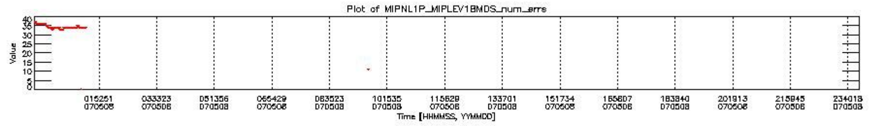
mipas_daily_report_level1_OFI_MIPAS_4_67_P_20070508_28.PNG
