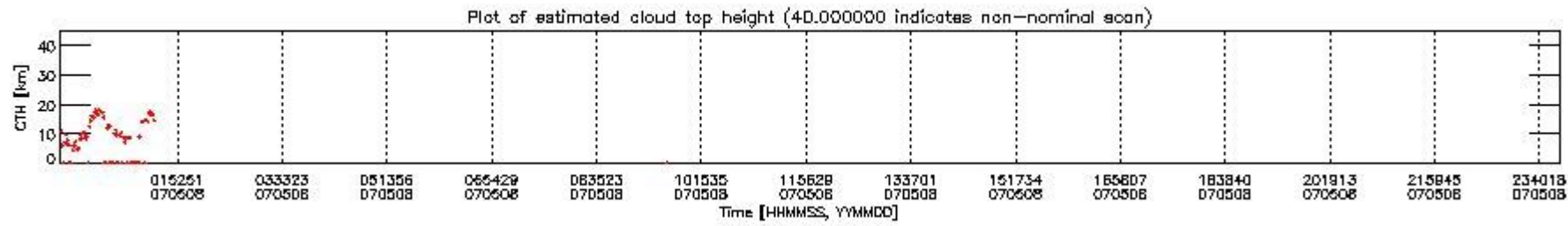
mipas_daily_report_level1_OFL_MIPAS_4_67_P_20070508_51.PNG
