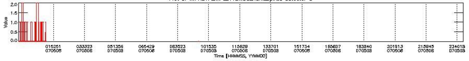
mipas_daily_report_level1_OFI_MIPAS_4_67_P_20070508_24.PNG
