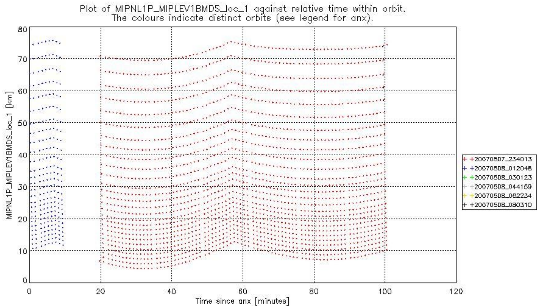
mipas_daily_report_level1_OFL_MIPAS_4_67_P_20070508_50.PNG
