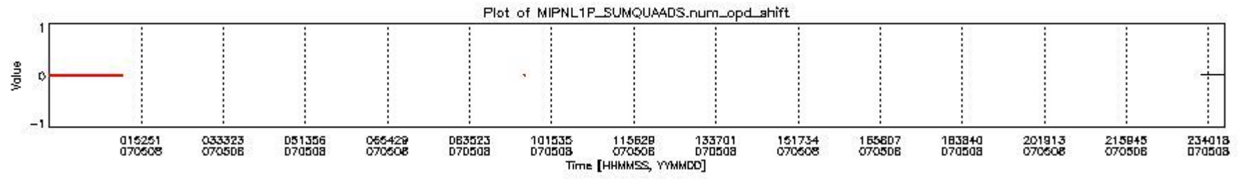
mipas_daily_report_level1_OFL_MIPAS_4_67_P_20070508_10.PNG
