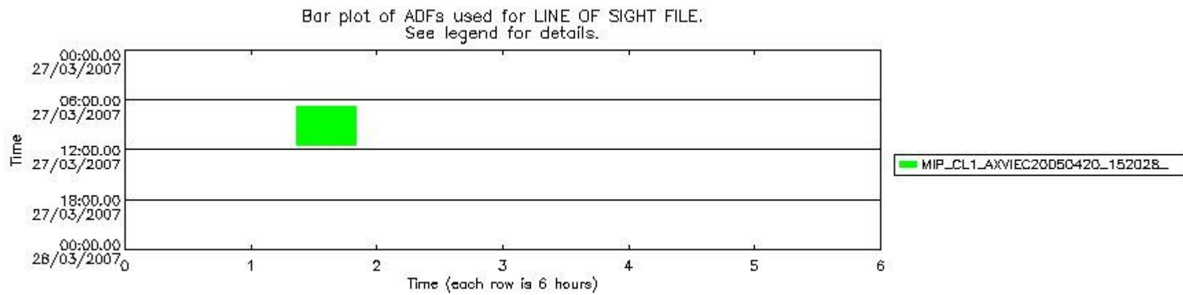
mipas_daily_report_level1_OFI_MIPAS_4_67_P_20070327_55.PNG
