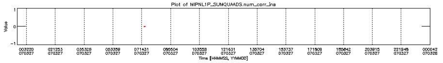
mipas_daily_report_level1_OFI_MIPAS_4_67_P_20070327_4.PNG
