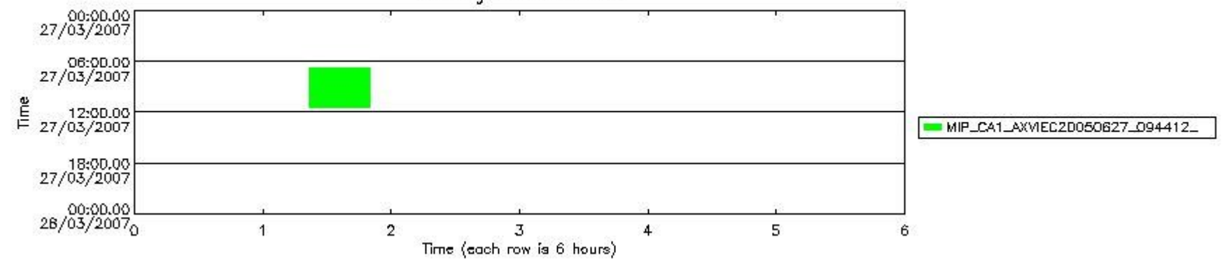
mipas_daily_report_level1_OFL_MIPAS_4_67_P_20070327_56.PNG
