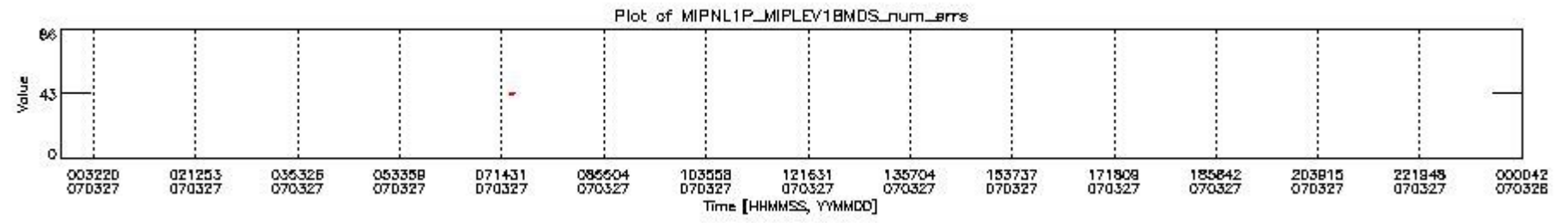
mipas_daily_report_level1_OFL_MIPAS_4_67_P_20070327_28.PNG
