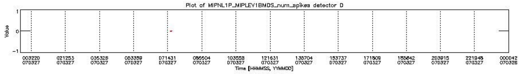
mipas_daily_report_level1_OFL_MIPAS_4_67_P_20070327_26.PNG
