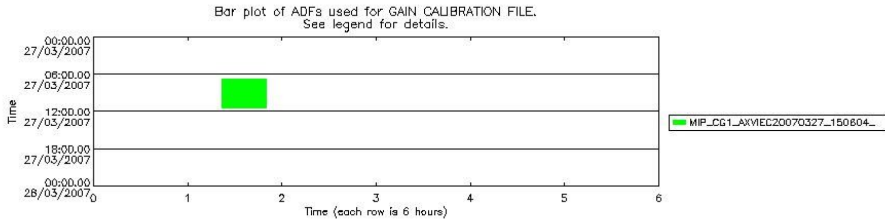
mipas_daily_report_level1_OFI_MIPAS_4_67_P_20070327_54.PNG
