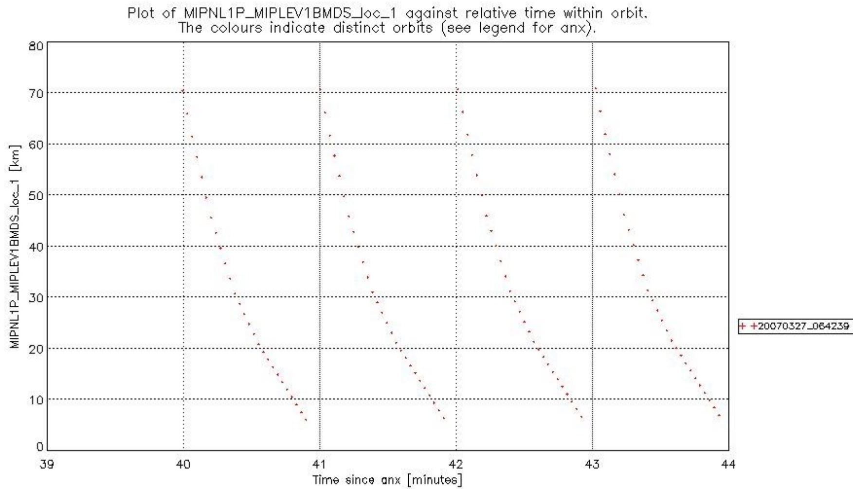
mipas_daily_report_level1_OFL_MIPAS_4_67_P_20070327_50.PNG
