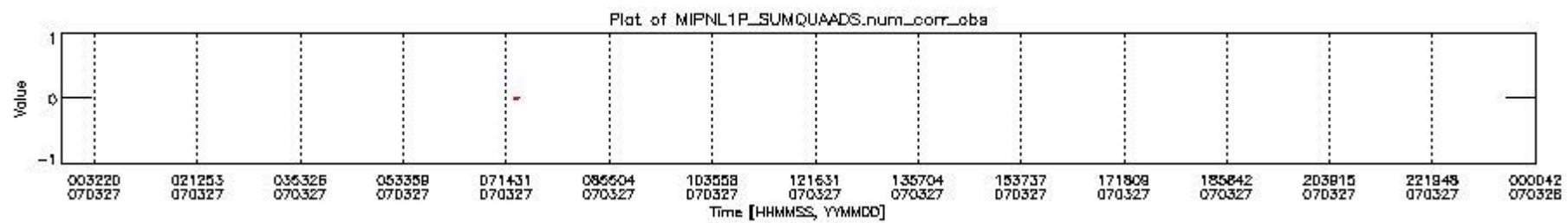
mipas_daily_report_level1_OFI_MIPAS_4_67_P_20070327_6.PNG
