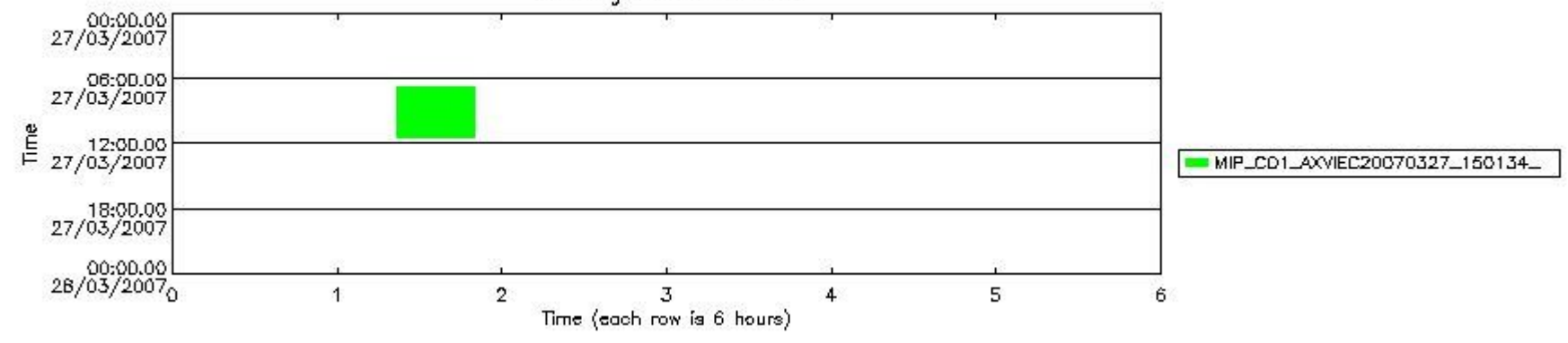
mipas_daily_report_level1_OFL_MIPAS_4_67_P_20070327_57.PNG
