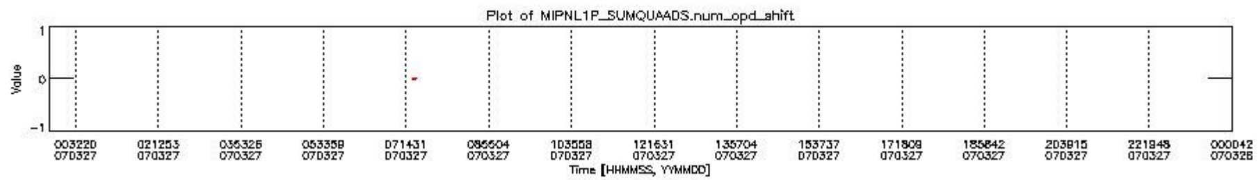
mipas_daily_report_level1_OFL_MIPAS_4_67_P_20070327_10.PNG
