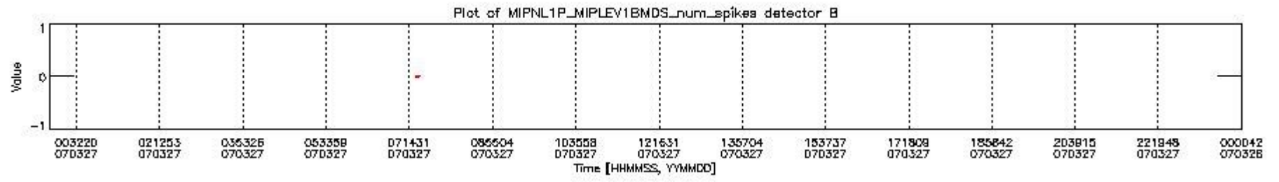
mipas_daily_report_level1_OFL_MIPAS_4_67_P_20070327_22.PNG
