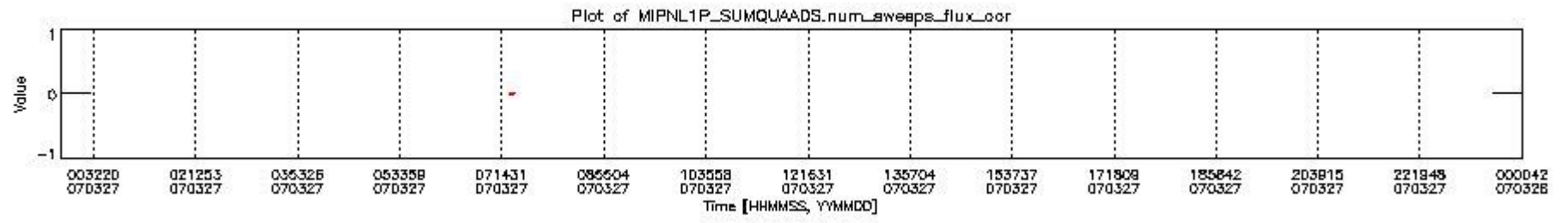
mipas_daily_report_level1_OFL_MIPAS_4_67_P_20070327_12.PNG
