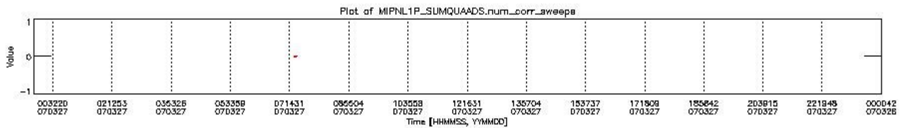
mipas_daily_report_level1_OFI_MIPAS_4_67_P_20070327_2.PNG
