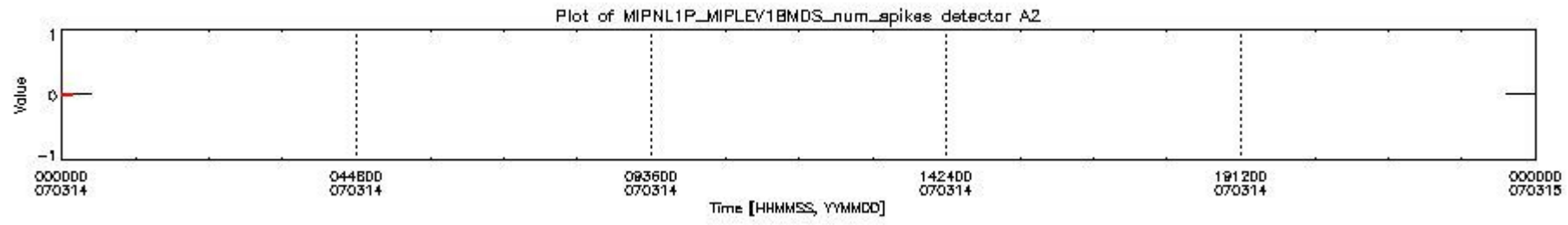
mipas_daily_report_level1_OFL_MIPAS_4_67_P_20070314_18.PNG
