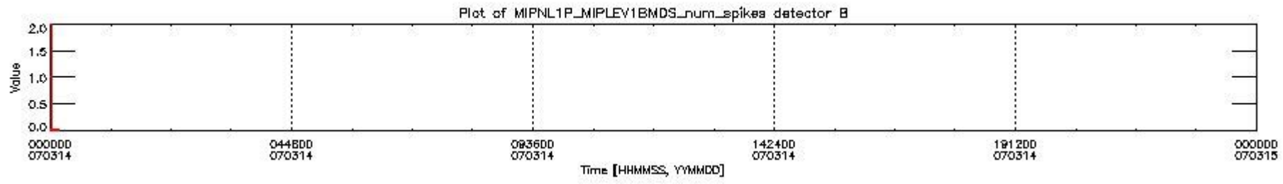
mipas_daily_report_level1_OFL_MIPAS_4_67_P_20070314_22.PNG
