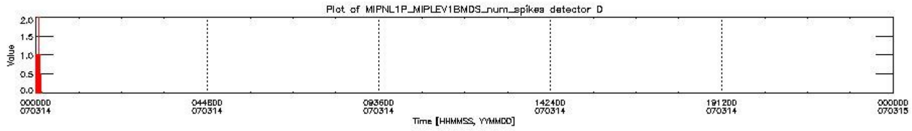
mipas_daily_report_level1_OFL_MIPAS_4_67_P_20070314_26.PNG
