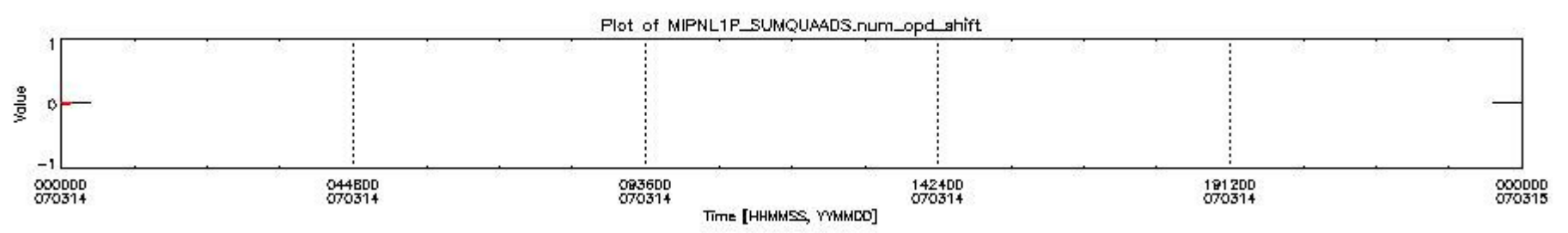
mipas_daily_report_level1_OFI_MIPAS_4_67_P_20070314_10.PNG
