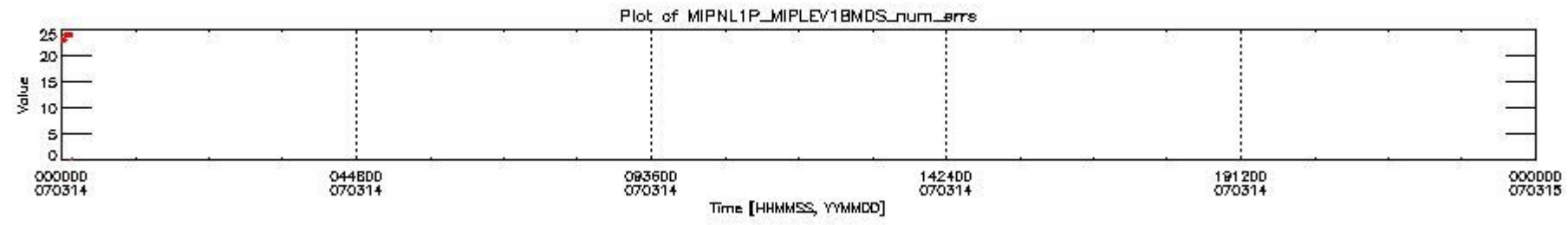
mipas_daily_report_level1_OFL_MIPAS_4_67_P_20070314_28.PNG
