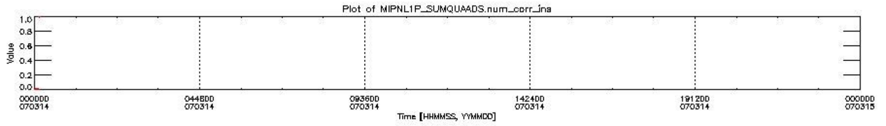
mipas_daily_report_level1_OFI_MIPAS_4_67_P_20070314_4.PNG
