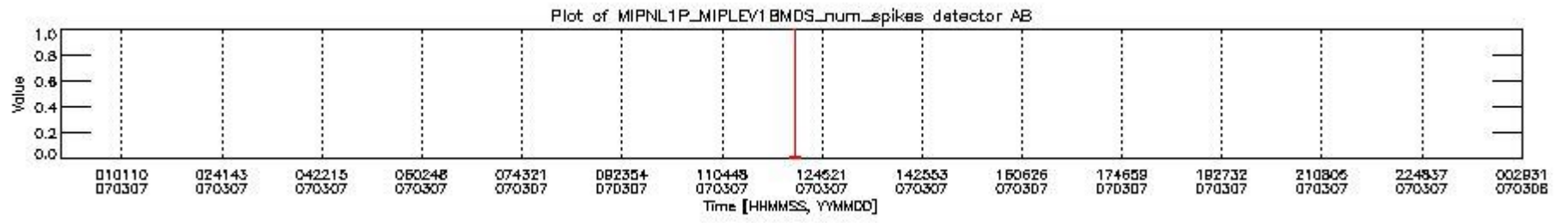
mipas_daily_report_level1_OFL_MIPAS_4_67_P_20070307_20.PNG
