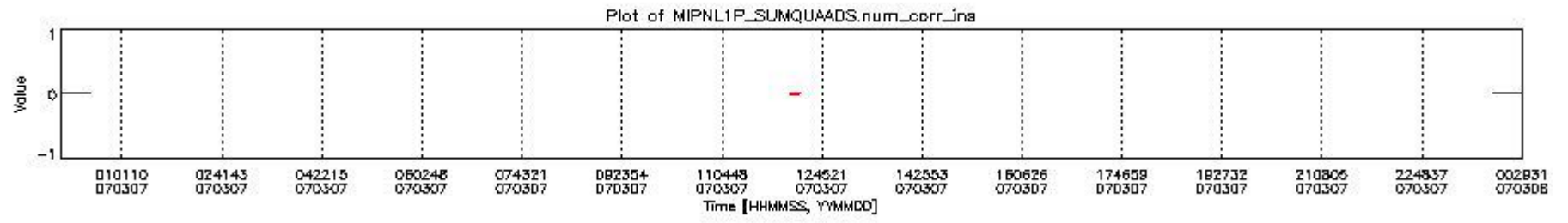
mipas_daily_report_level1_OFL_MIPAS_4_67_P_20070307_4.PNG
