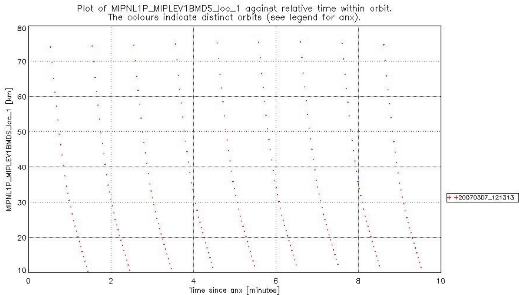
mipas_daily_report_level1_OFL_MIPAS_4_67_P_20070307_50.PNG
