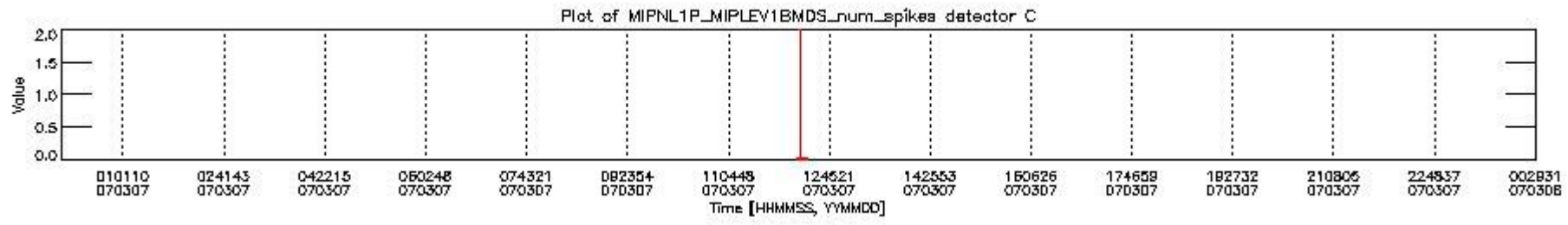
mipas_daily_report_level1_OFL_MIPAS_4_67_P_20070307_24.PNG
