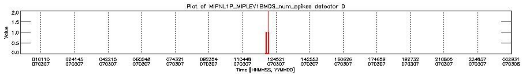
mipas_daily_report_level1_OFL_MIPAS_4_67_P_20070307_26.PNG
