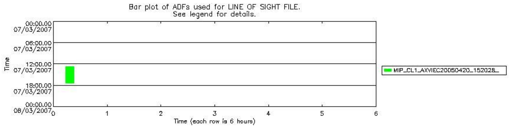
mipas_daily_report_level1_OFL_MIPAS_4_67_P_20070307_55.PNG
