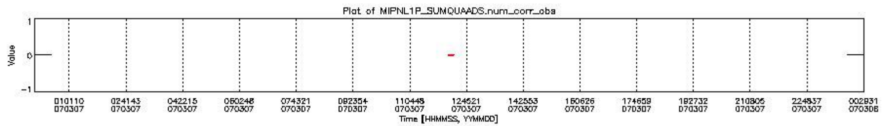
mipas_daily_report_level1_OFI_MIPAS_4_67_P_20070307_6.PNG
