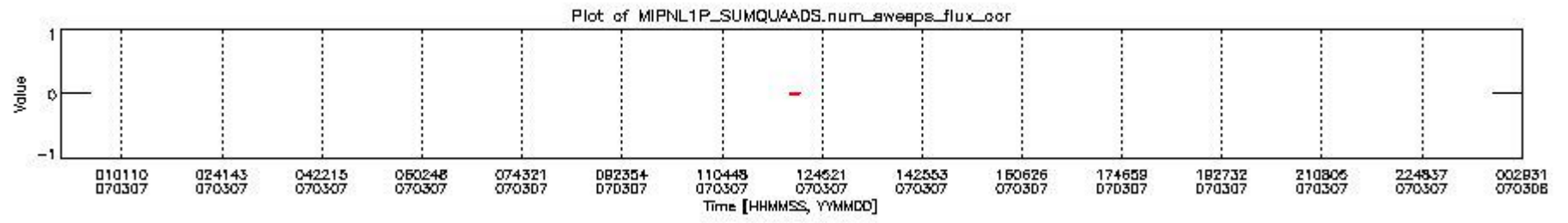
mipas_daily_report_level1_OFL_MIPAS_4_67_P_20070307_12.PNG
