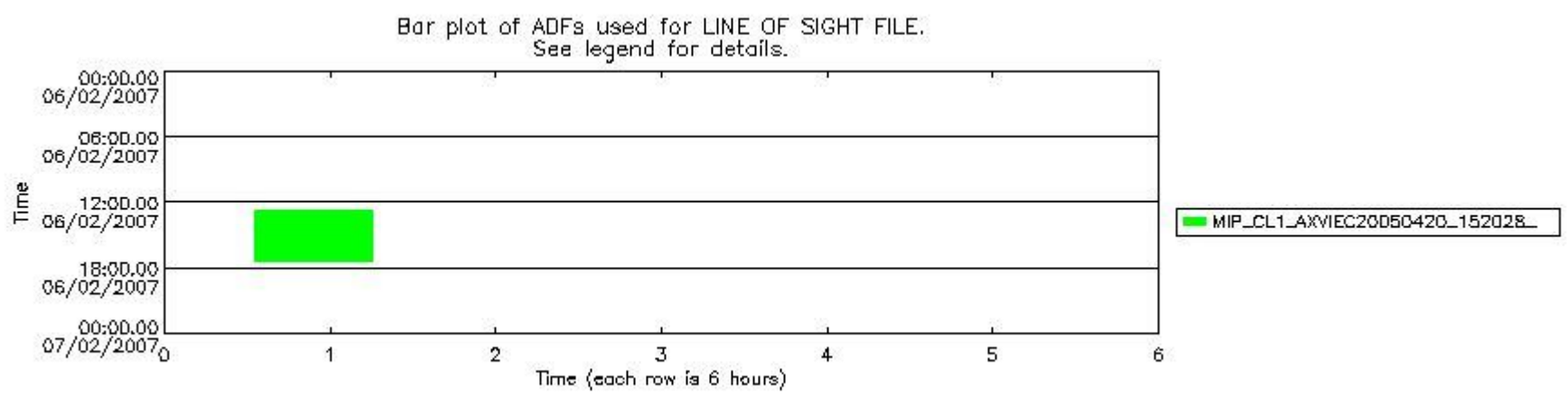
mipas_daily_report_level1_OFI_MIPAS_4_67_P_20070206_55.PNG
