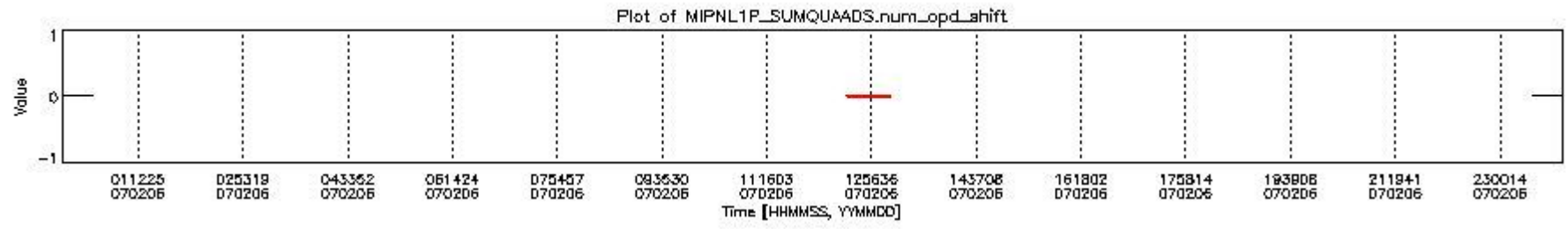
mipas_daily_report_level1_OFL_MIPAS_4_67_P_20070206_10.PNG
