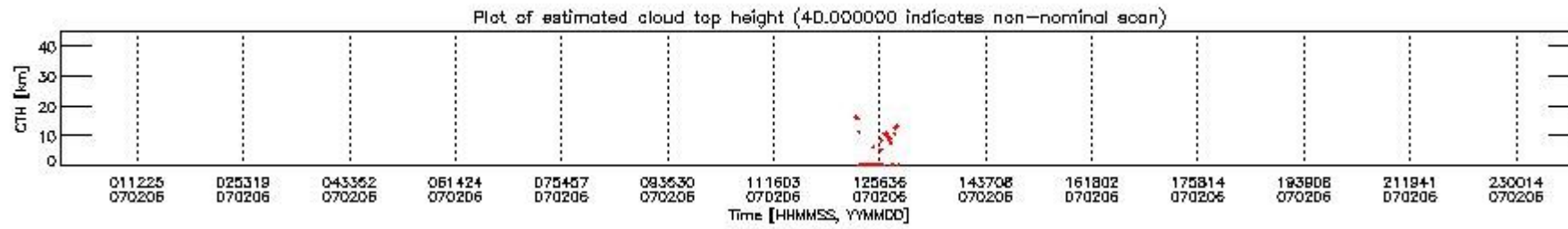
mipas_daily_report_level1_OFL_MIPAS_4_67_P_20070206_51.PNG
