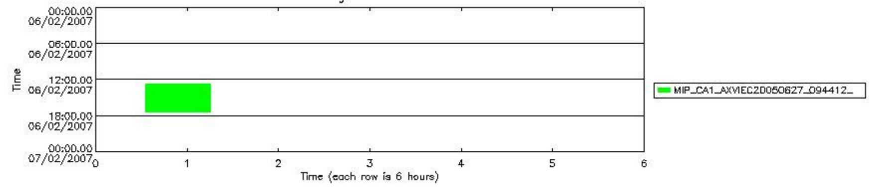
mipas_daily_report_level1_OFL_MIPAS_4_67_P_20070206_56.PNG
