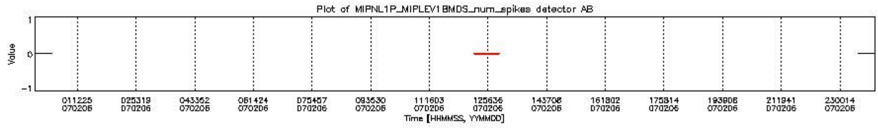
mipas_daily_report_level1_OFL_MIPAS_4_67_P_20070206_20.PNG
