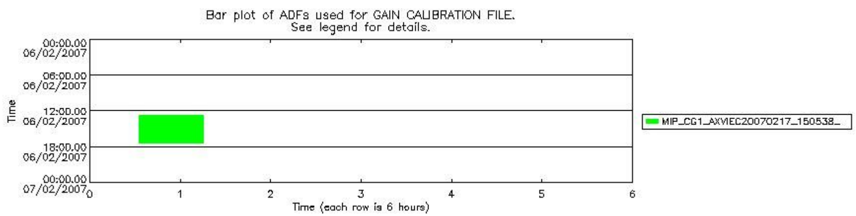
mipas_daily_report_level1_OFI_MIPAS_4_67_P_20070206_54.PNG
