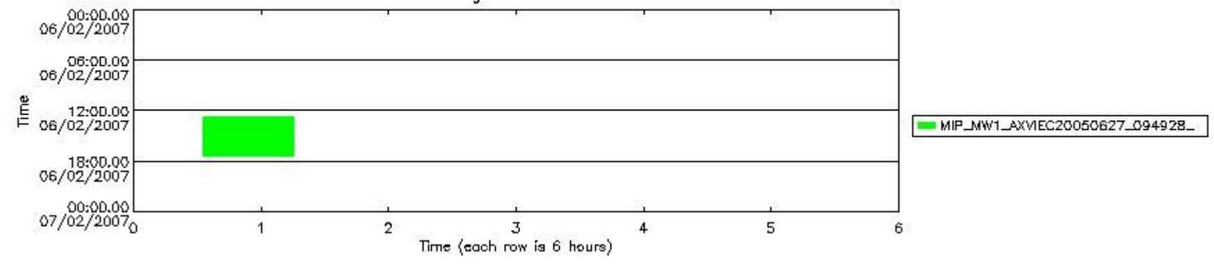
mipas_daily_report_level1_OFL_MIPAS_4_67_P_20070206_58.PNG
