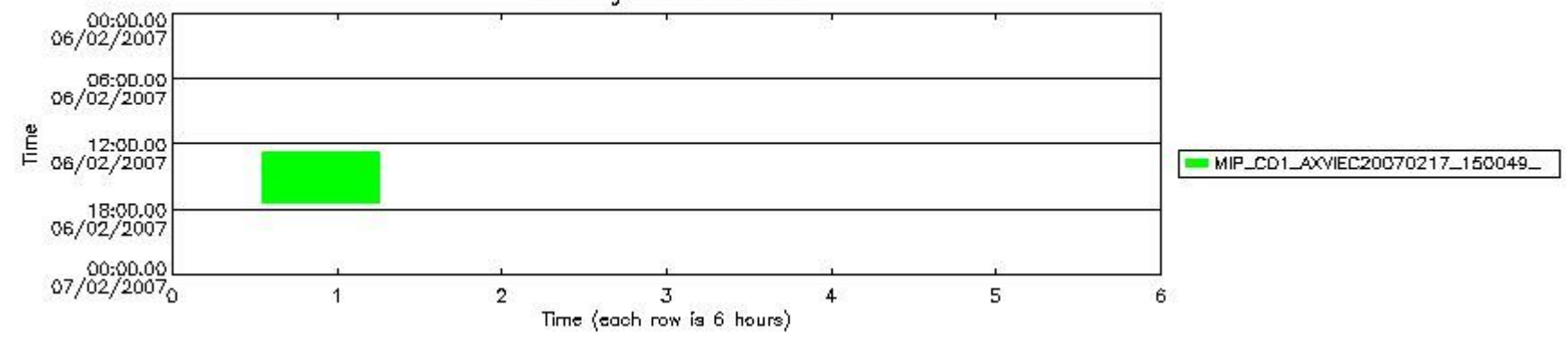
mipas_daily_report_level1_OFL_MIPAS_4_67_P_20070206_57.PNG
