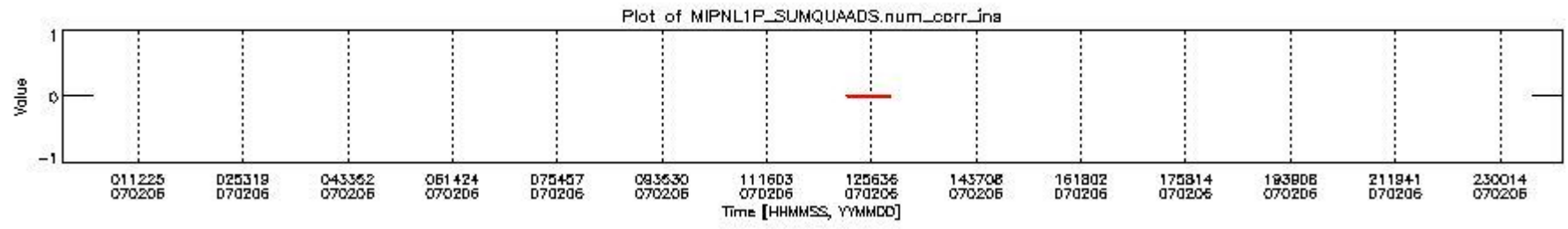
mipas_daily_report_level1_OFI_MIPAS_4_67_P_20070206_4.PNG
