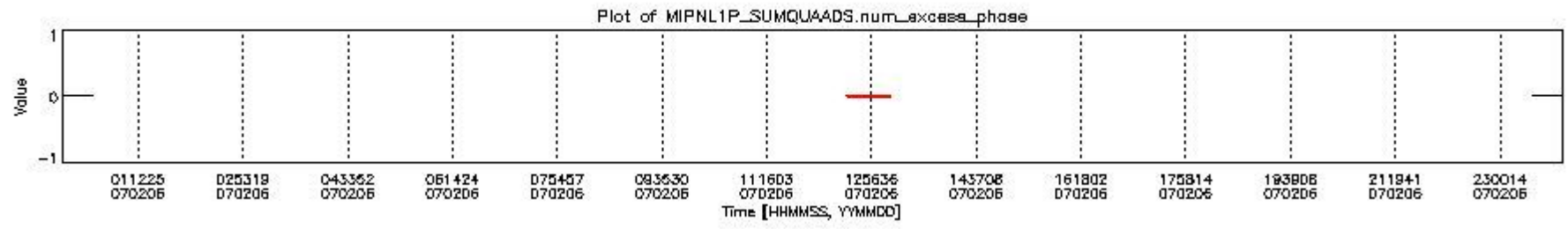
mipas_daily_report_level1_OFI_MIPAS_4_67_P_20070206_8.PNG
