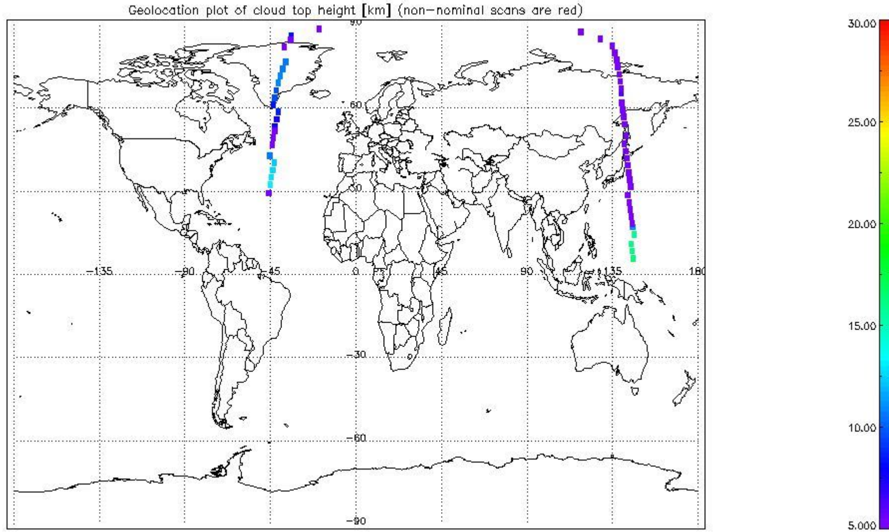
mipas_daily_report_level1_OFL_MIPAS_4_67_P_20070206_51.PNG
