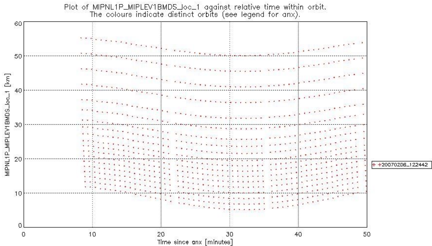
mipas_daily_report_level1_OFL_MIPAS_4_67_P_20070206_50.PNG
