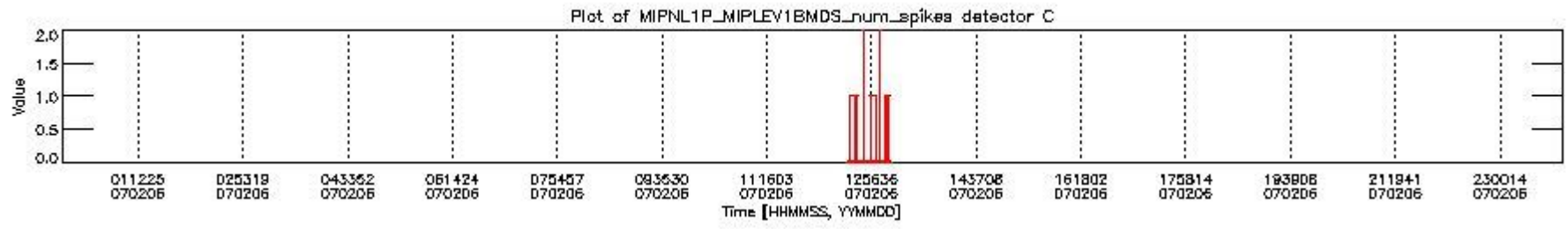
mipas_daily_report_level1_OFI_MIPAS_4_67_P_20070206_24.PNG
