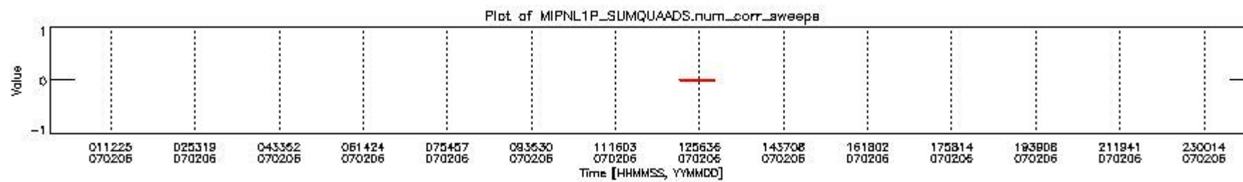
mipas_daily_report_level1_OFL_MIPAS_4_67_P_20070206_2.PNG
