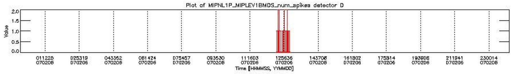
mipas_daily_report_level1_OFL_MIPAS_4_67_P_20070206_26.PNG
