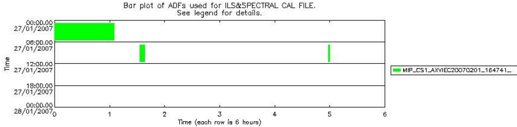
mipas_daily_report_level1_OFL_MIPAS_4_67_P_20070127_53.PNG
