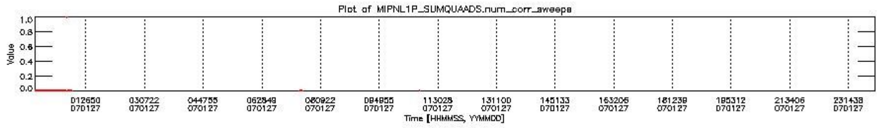
mipas_daily_report_level1_OFL_MIPAS_4_67_P_20070127_2.PNG
