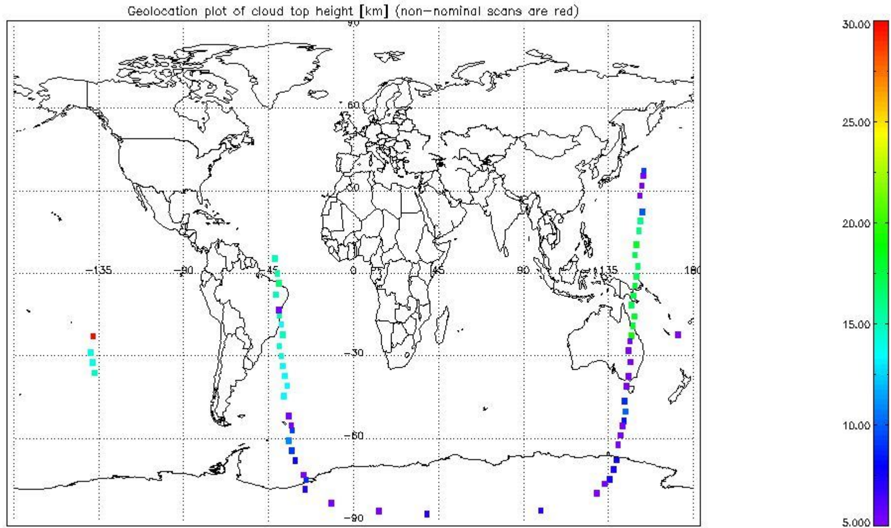
mipas_daily_report_level1_OFL_MIPAS_4_67_P_20070127_51.PNG
