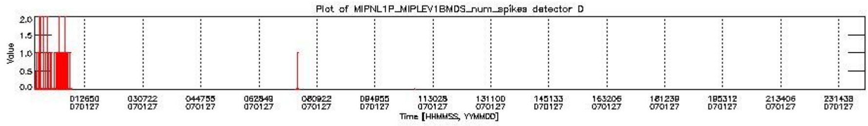
mipas_daily_report_level1_OFL_MIPAS_4_67_P_20070127_26.PNG
