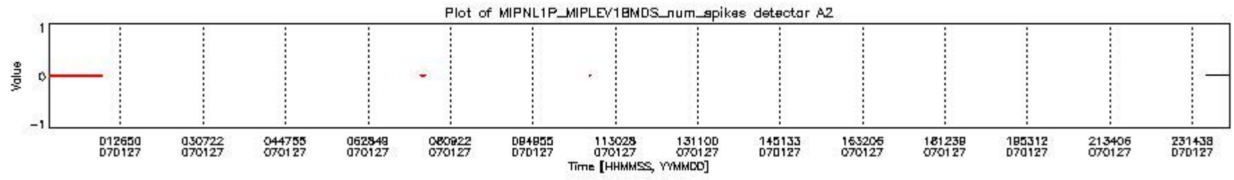
mipas_daily_report_level1_OFL_MIPAS_4_67_P_20070127_18.PNG
