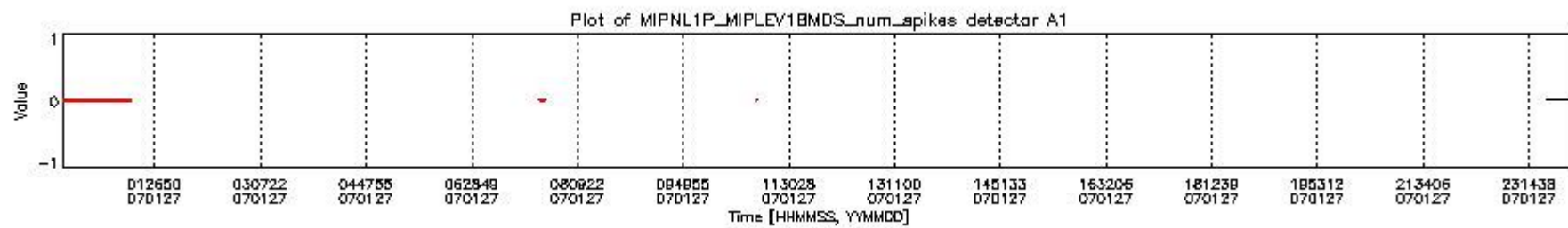
mipas_daily_report_level1_OFL_MIPAS_4_67_P_20070127_16.PNG
