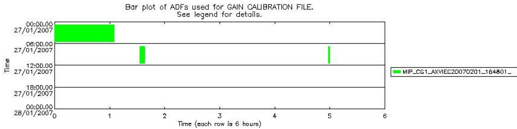
mipas_daily_report_level1_OFL_MIPAS_4_67_P_20070127_54.PNG
