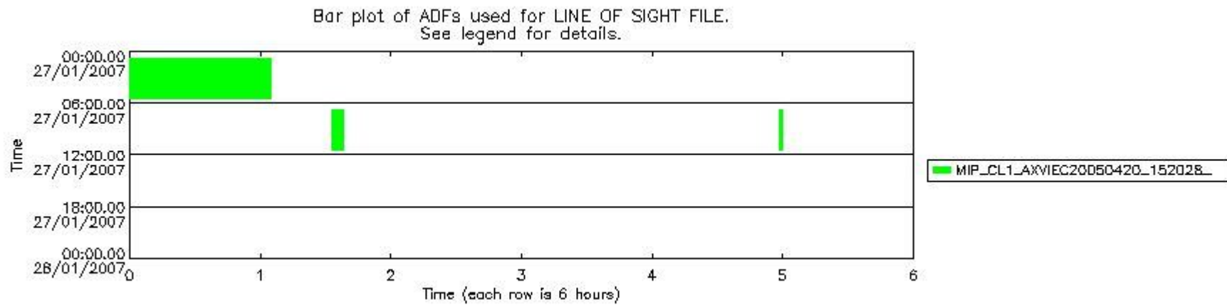
mipas_daily_report_level1_OFL_MIPAS_4_67_P_20070127_55.PNG
