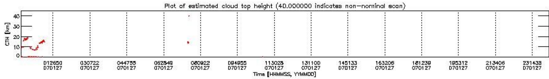
mipas_daily_report_level1_OFL_MIPAS_4_67_P_20070127_51.PNG
