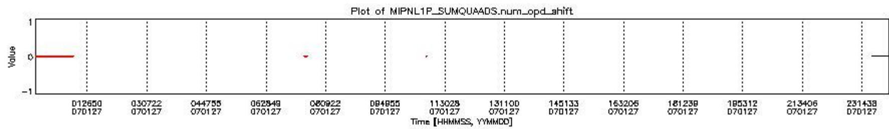
mipas_daily_report_level1_OFL_MIPAS_4_67_P_20070127_10.PNG
