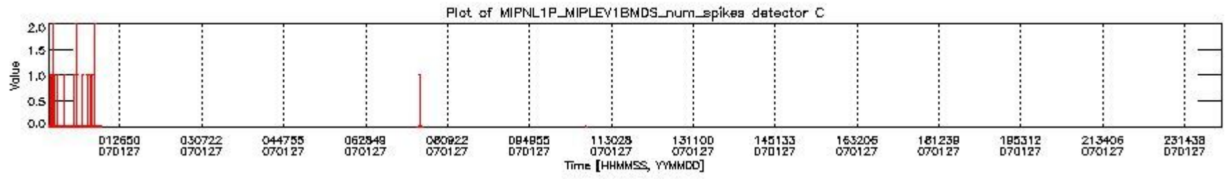
mipas_daily_report_level1_OFL_MIPAS_4_67_P_20070127_24.PNG
