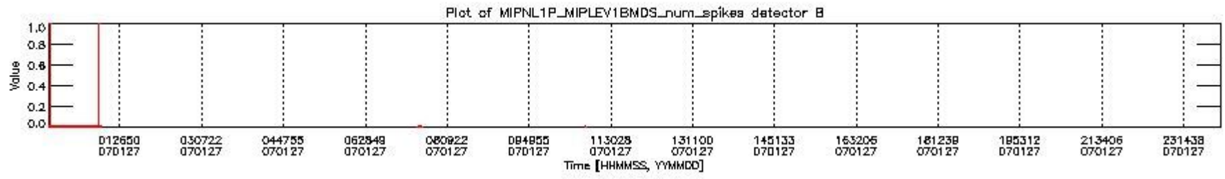
mipas_daily_report_level1_OFL_MIPAS_4_67_P_20070127_22.PNG
