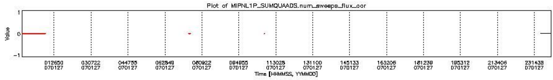
mipas_daily_report_level1_OFL_MIPAS_4_67_P_20070127_12.PNG
