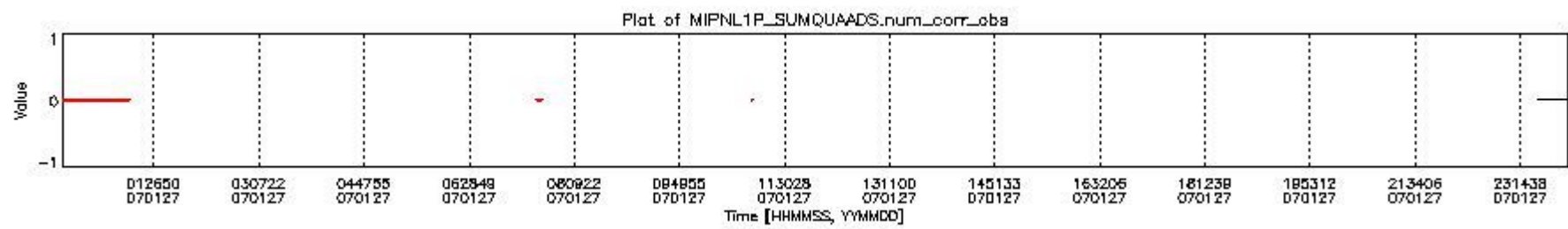
mipas_daily_report_level1_OFI_MIPAS_4_67_P_20070127_6.PNG
