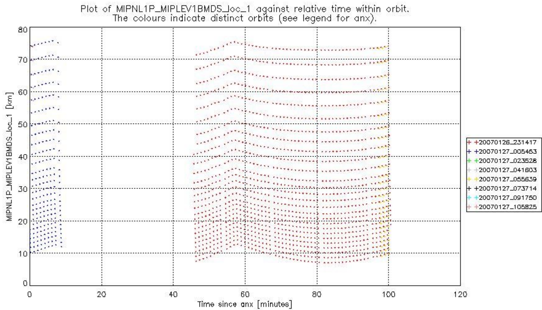
mipas_daily_report_level1_OFL_MIPAS_4_67_P_20070127_50.PNG
