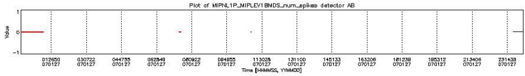
mipas_daily_report_level1_OFL_MIPAS_4_67_P_20070127_20.PNG
