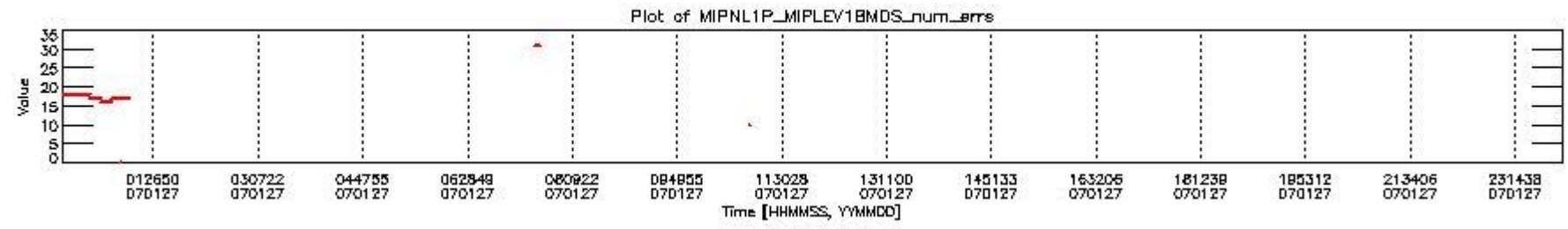
mipas_daily_report_level1_OFL_MIPAS_4_67_P_20070127_28.PNG
