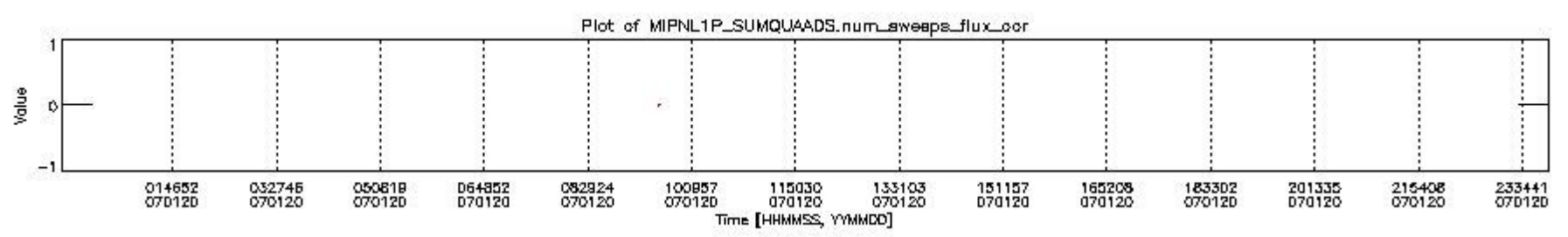
mipas_daily_report_level1_OFL_MIPAS_4_67_P_20070120_12.PNG
