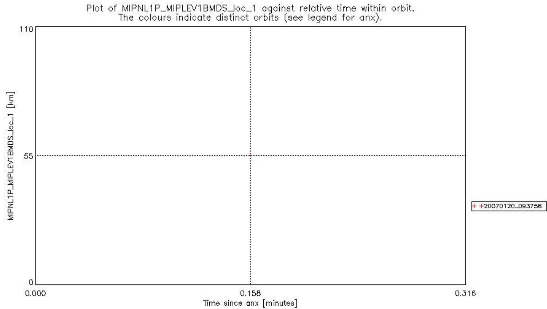
mipas_daily_report_level1_OFL_MIPAS_4_67_P_20070120_50.PNG
