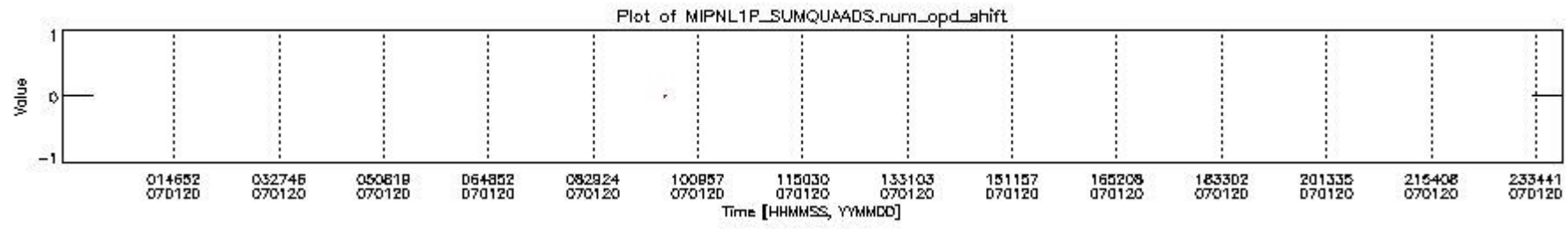
mipas_daily_report_level1_OFL_MIPAS_4_67_P_20070120_10.PNG
