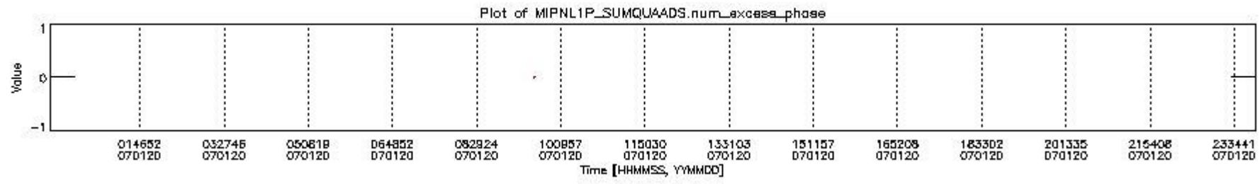
mipas_daily_report_level1_OFI_MIPAS_4_67_P_20070120_8.PNG
