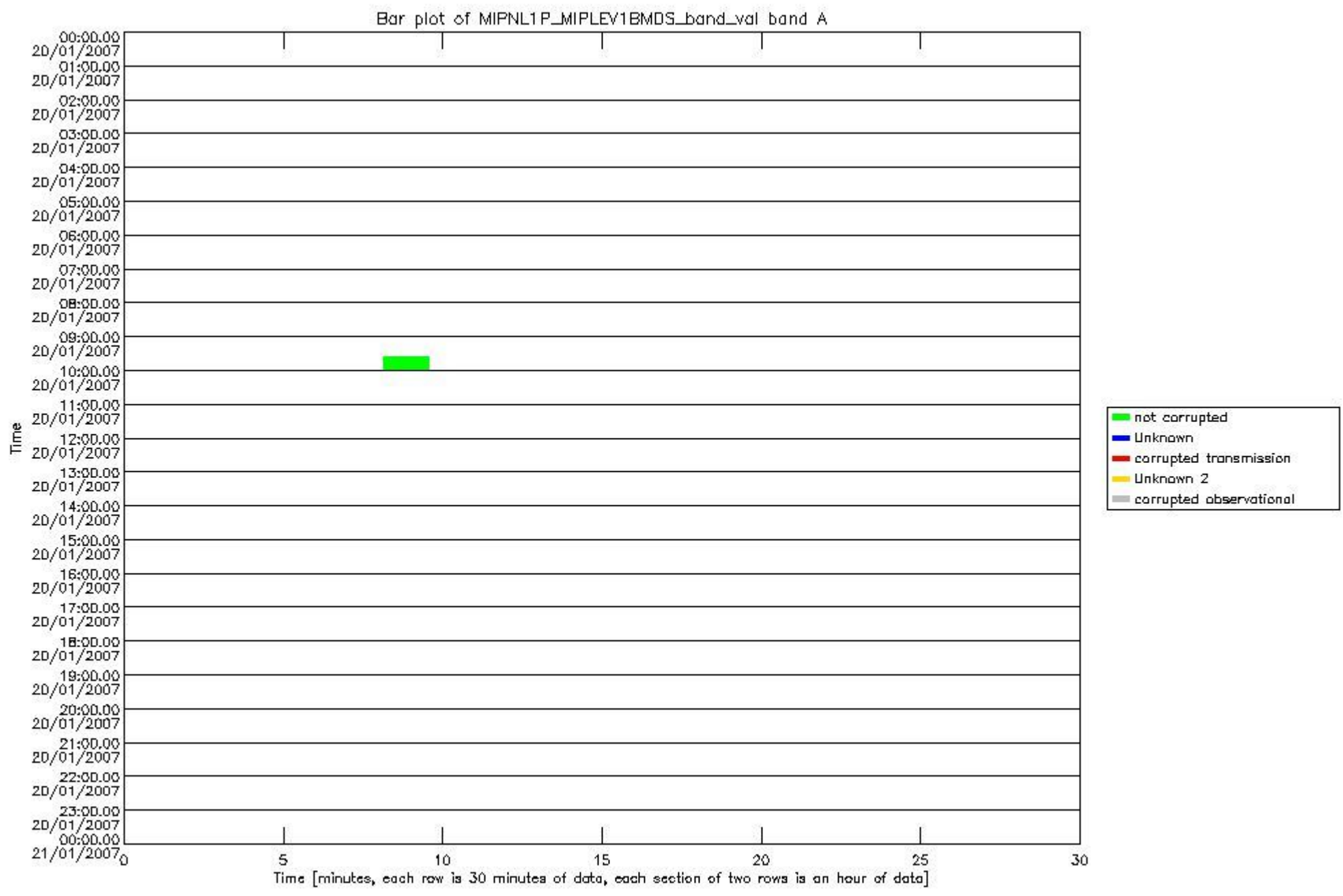
mipas_daily_report_level1_OFI_MIPAS_4_67_P_20070120_30.PNG
