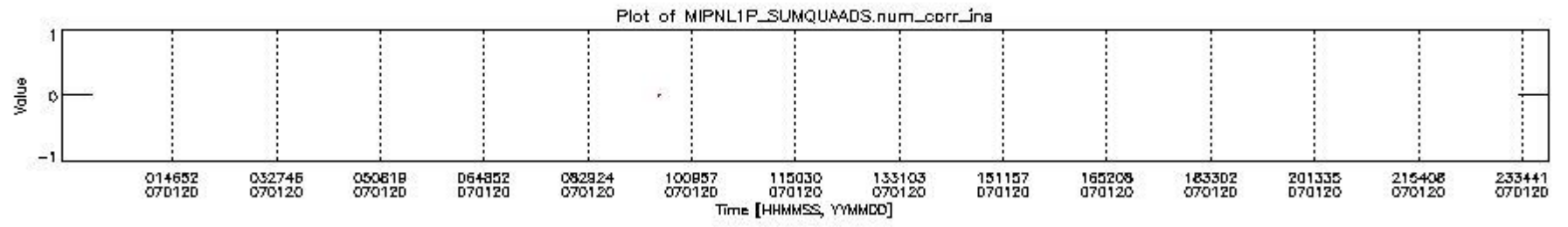
mipas_daily_report_level1_OFI_MIPAS_4_67_P_20070120_4.PNG
