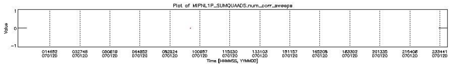
mipas_daily_report_level1_OFI_MIPAS_4_67_P_20070120_2.PNG
