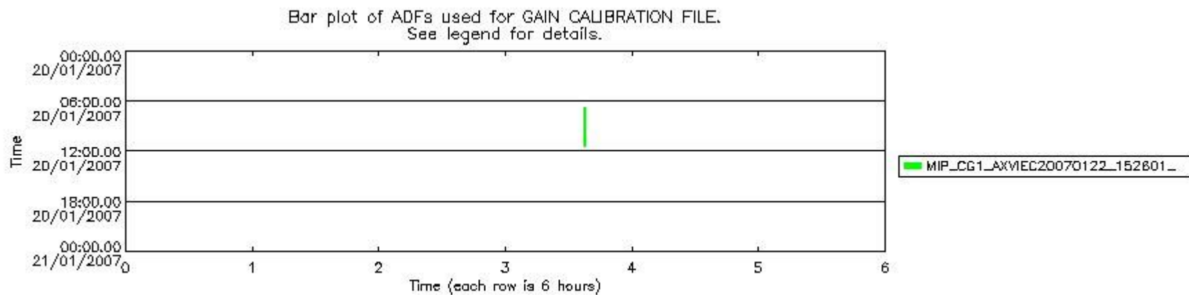
mipas_daily_report_level1_OFL_MIPAS_4_67_P_20070120_52.PNG
