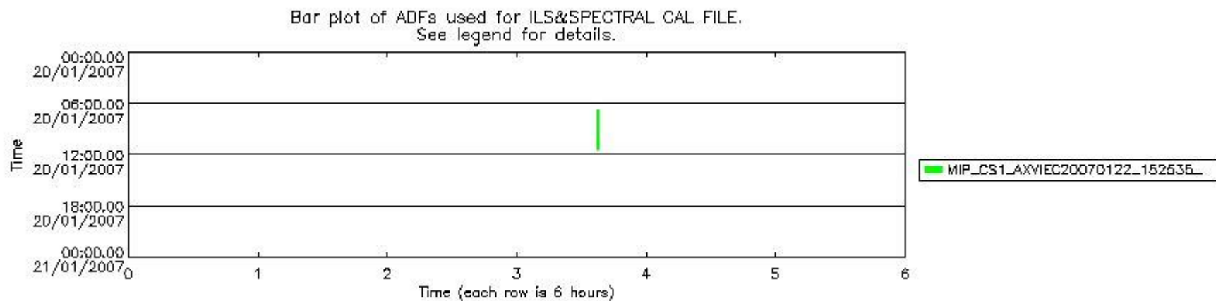
mipas_daily_report_level1_OFL_MIPAS_4_67_P_20070120_51.PNG
