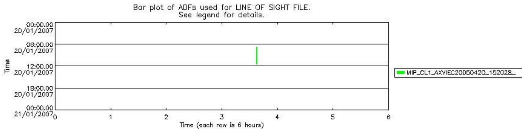
mipas_daily_report_level1_OFL_MIPAS_4_67_P_20070120_53.PNG
