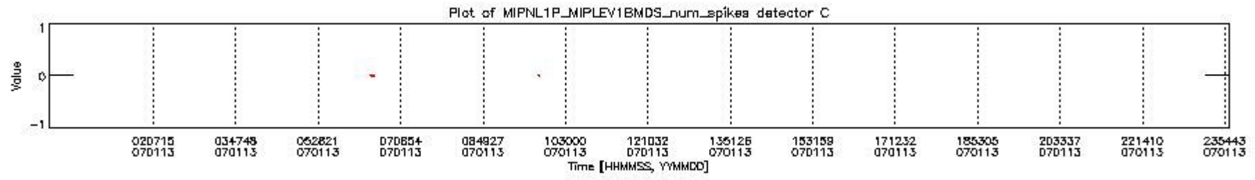
mipas_daily_report_level1_OFI_MIPAS_4_67_P_20070113_24.PNG
