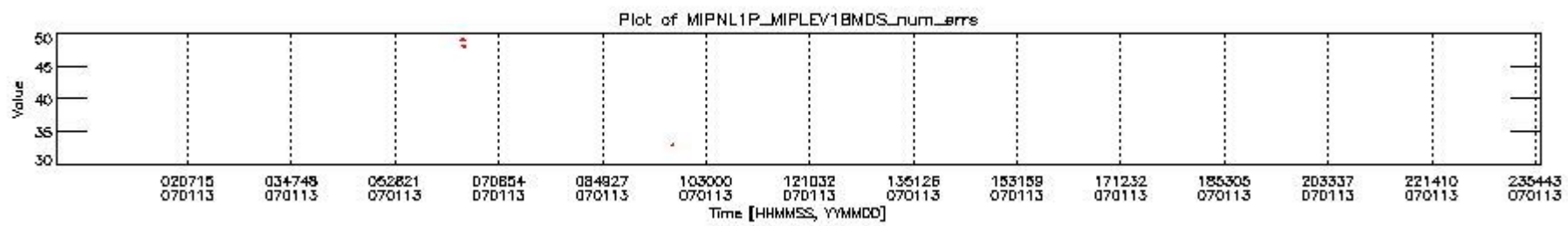
mipas_daily_report_level1_OFI_MIPAS_4_67_P_20070113_28.PNG
