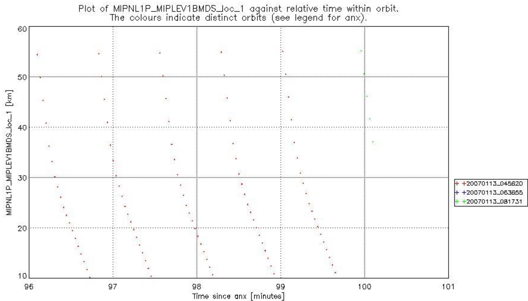
mipas_daily_report_level1_OFL_MIPAS_4_67_P_20070113_50.PNG
