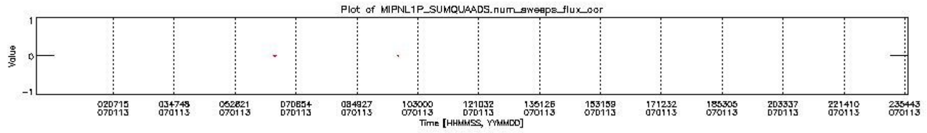
mipas_daily_report_level1_OFI_MIPAS_4_67_P_20070113_12.PNG
