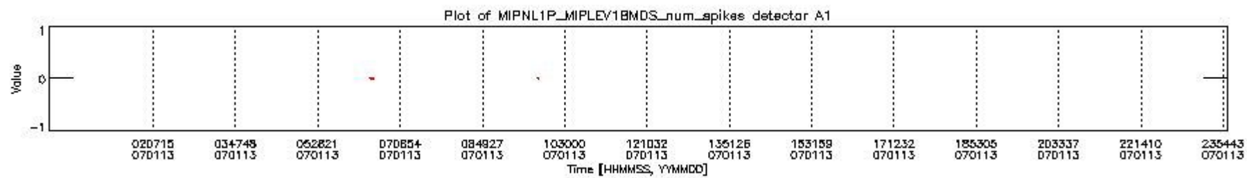
mipas_daily_report_level1_OFL_MIPAS_4_67_P_20070113_16.PNG
