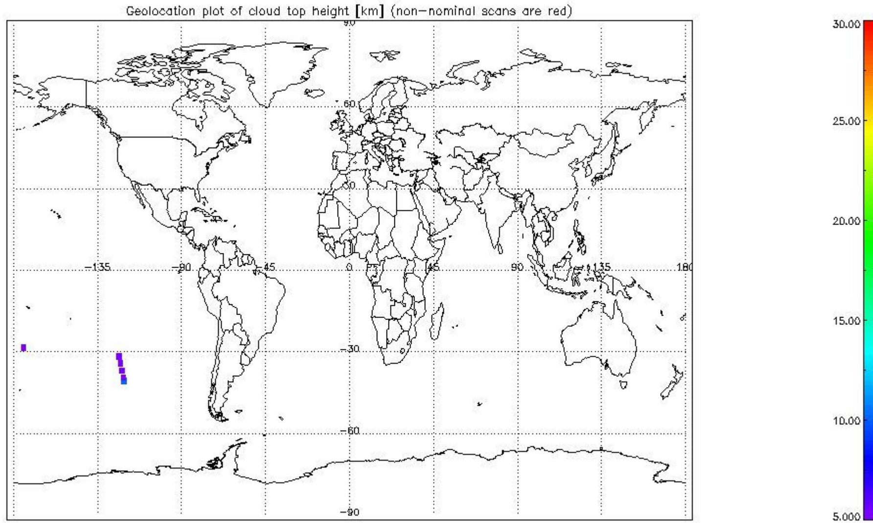
mipas_daily_report_level1_OFL_MIPAS_4_67_P_20070113_51.PNG
