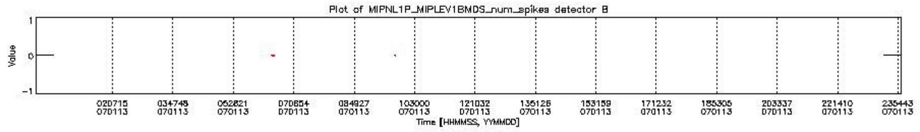
mipas_daily_report_level1_OFI_MIPAS_4_67_P_20070113_22.PNG
