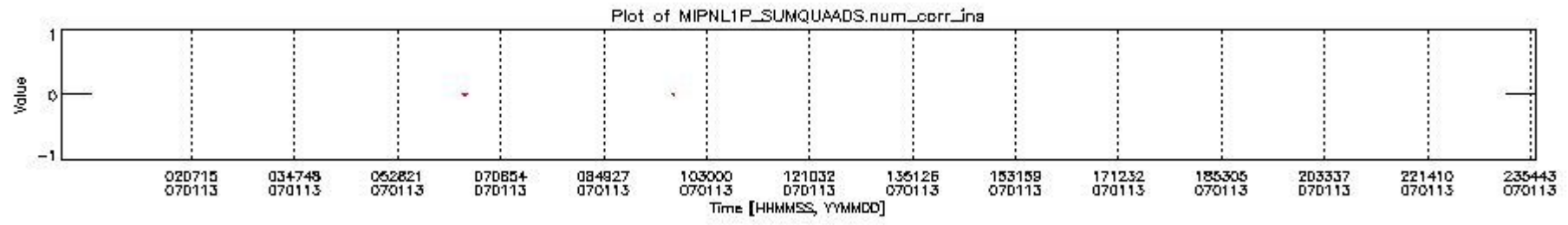
mipas_daily_report_level1_OFL_MIPAS_4_67_P_20070113_4.PNG
