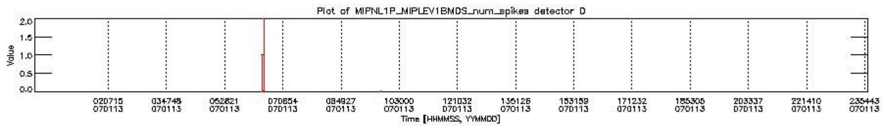
mipas_daily_report_level1_OFI_MIPAS_4_67_P_20070113_26.PNG
