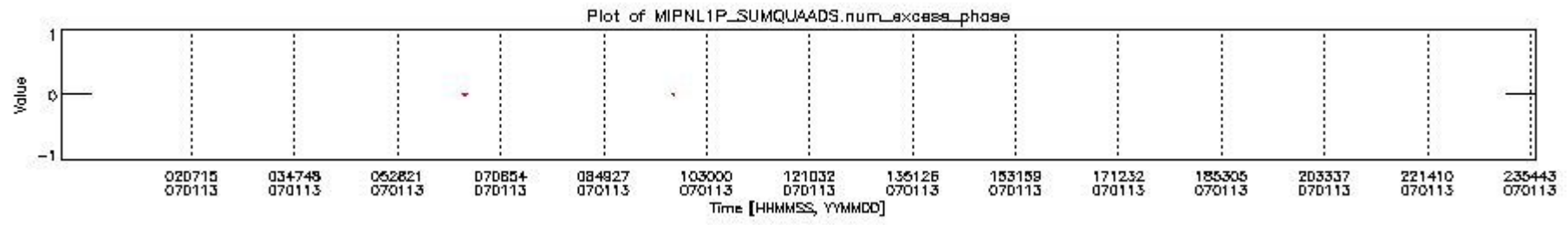
mipas_daily_report_level1_OFI_MIPAS_4_67_P_20070113_8.PNG
