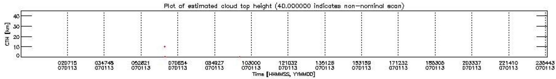
mipas_daily_report_level1_OFL_MIPAS_4_67_P_20070113_51.PNG
