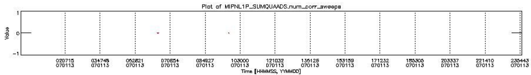
mipas_daily_report_level1_OFL_MIPAS_4_67_P_20070113_2.PNG
