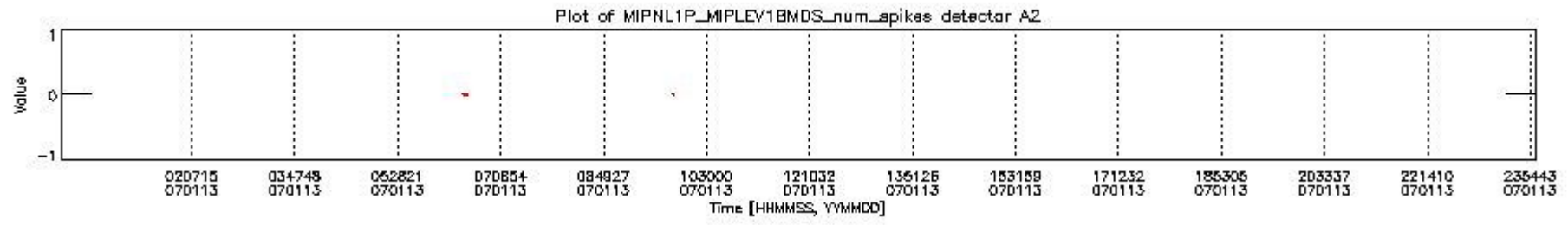
mipas_daily_report_level1_OFI_MIPAS_4_67_P_20070113_18.PNG
