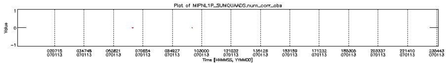
mipas_daily_report_level1_OFI_MIPAS_4_67_P_20070113_6.PNG
