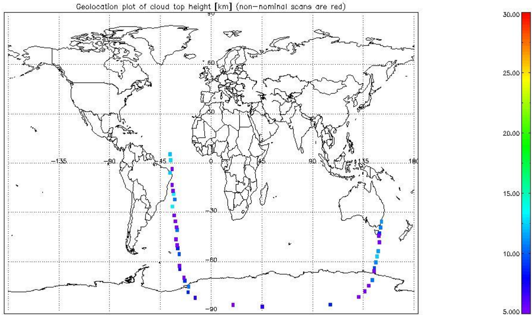
mipas_daily_report_level1_OFL_MIPAS_4_67_P_20061230_51.PNG
