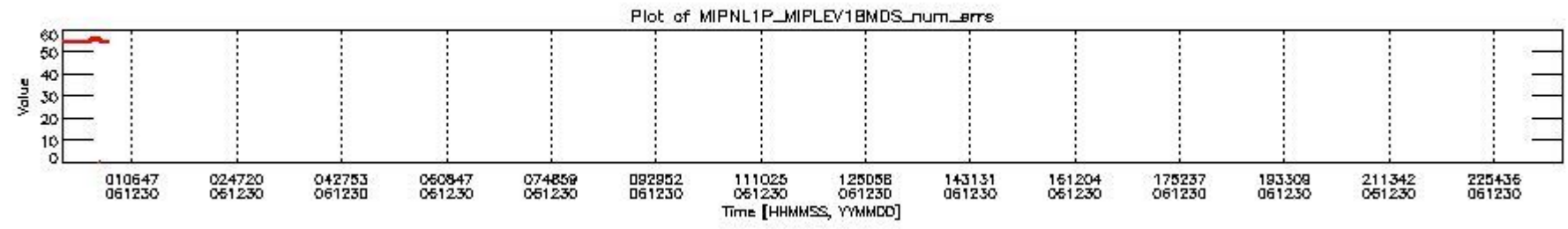
mipas_daily_report_level1_OFI_MIPAS_4_67_P_20061230_28.PNG
