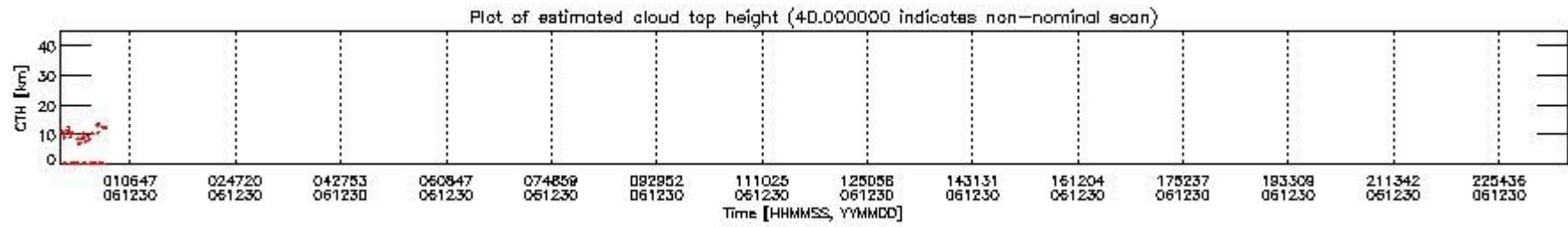
mipas_daily_report_level1_OFL_MIPAS_4_67_P_20061230_51.PNG
