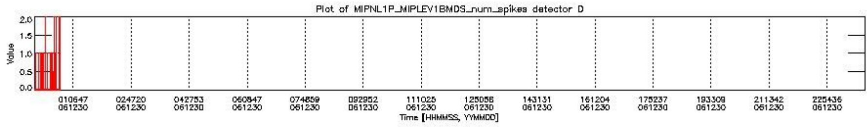
mipas_daily_report_level1_OFI_MIPAS_4_67_P_20061230_26.PNG
