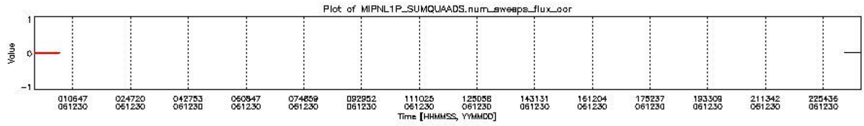
mipas_daily_report_level1_OFL_MIPAS_4_67_P_20061230_12.PNG
