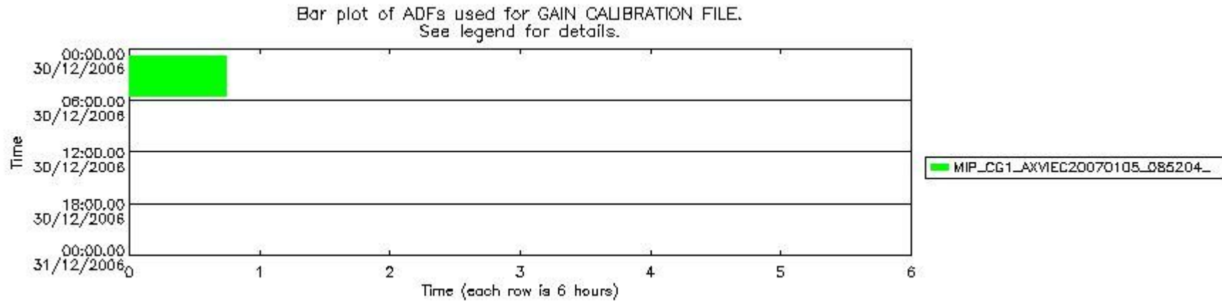
mipas_daily_report_level1_OFL_MIPAS_4_67_P_20061230_54.PNG
