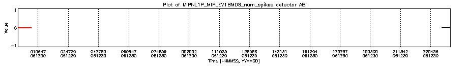
mipas_daily_report_level1_OFI_MIPAS_4_67_P_20061230_20.PNG
