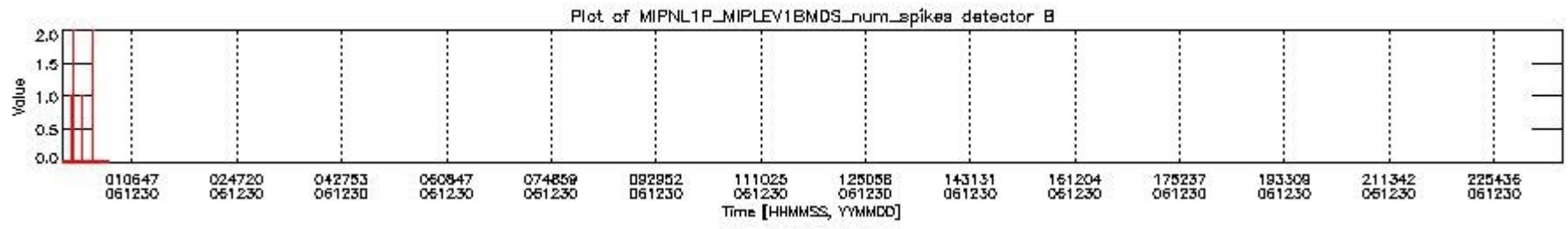
mipas_daily_report_level1_OFI_MIPAS_4_67_P_20061230_22.PNG
