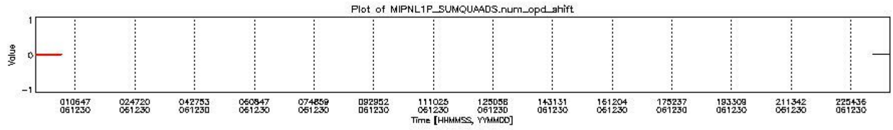
mipas_daily_report_level1_OFI_MIPAS_4_67_P_20061230_10.PNG
