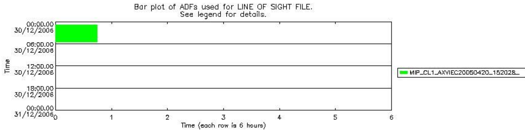
mipas_daily_report_level1_OFL_MIPAS_4_67_P_20061230_55.PNG
