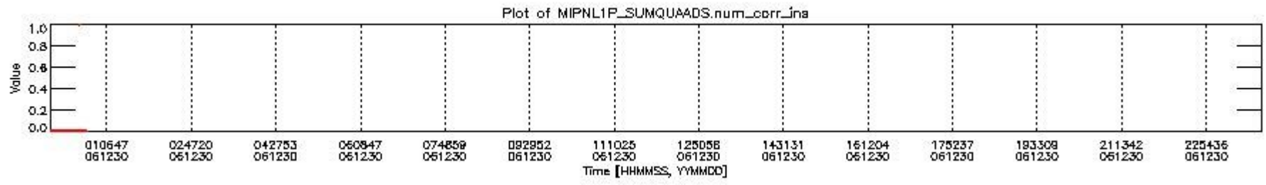
mipas_daily_report_level1_OFI_MIPAS_4_67_P_20061230_4.PNG
