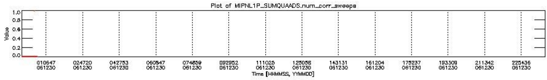
mipas_daily_report_level1_OFI_MIPAS_4_67_P_20061230_2.PNG
