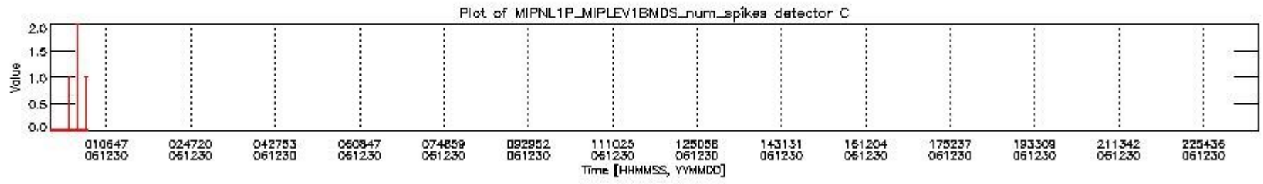
mipas_daily_report_level1_OFI_MIPAS_4_67_P_20061230_24.PNG
