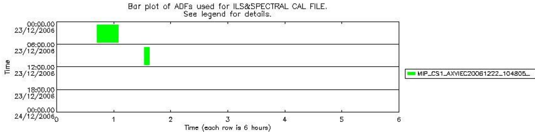
mipas_daily_report_level1_OFI_MIPAS_4_67_P_20061223_53.PNG
