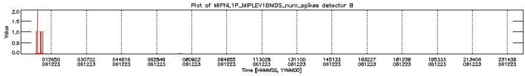
mipas_daily_report_level1_OFL_MIPAS_4_67_P_20061223_22.PNG
