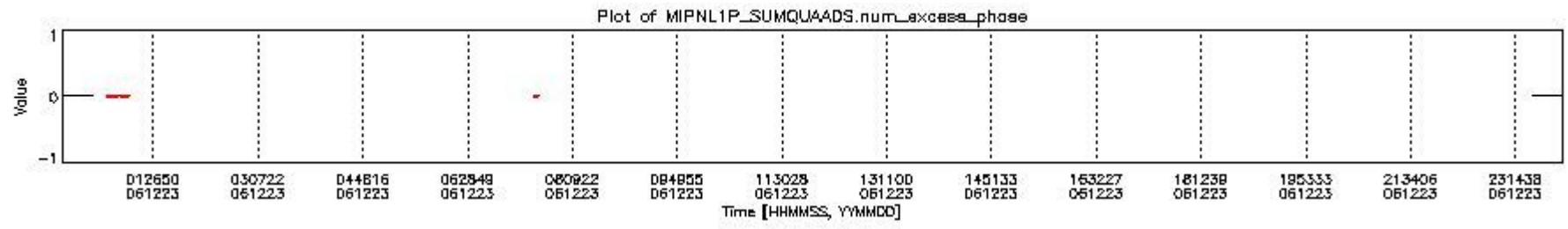
mipas_daily_report_level1_OFI_MIPAS_4_67_P_20061223_8.PNG
