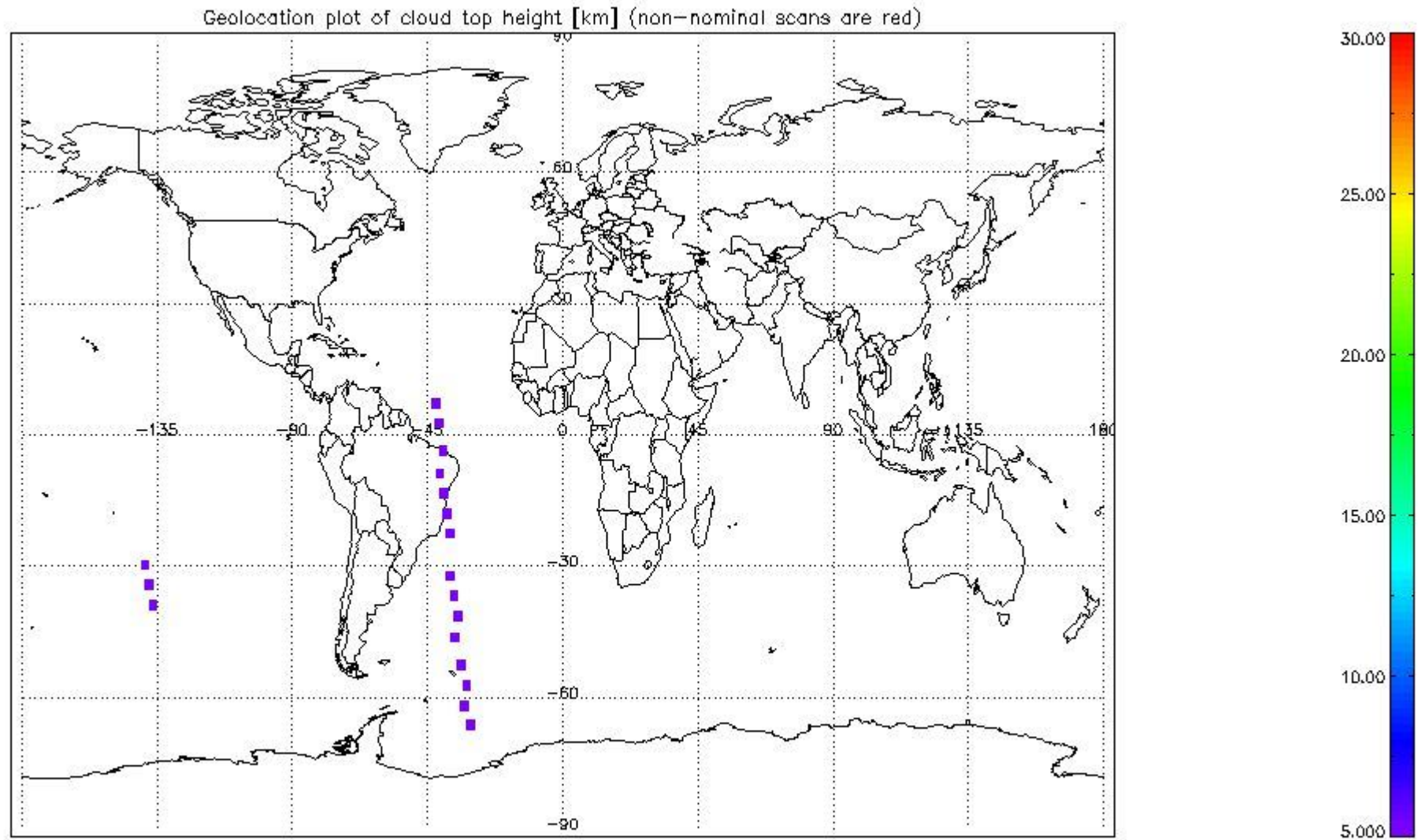
mipas_daily_report_level1_OFL_MIPAS_4_67_P_20061223_51.PNG
