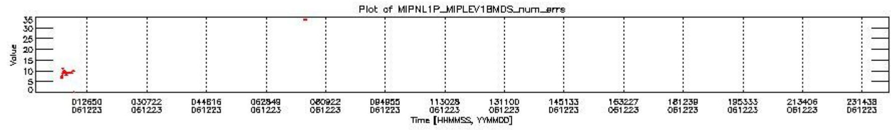
mipas_daily_report_level1_OFL_MIPAS_4_67_P_20061223_28.PNG
