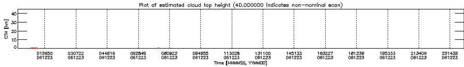
mipas_daily_report_level1_OFL_MIPAS_4_67_P_20061223_51.PNG
