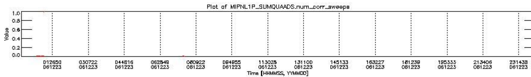
mipas_daily_report_level1_OFL_MIPAS_4_67_P_20061223_2.PNG
