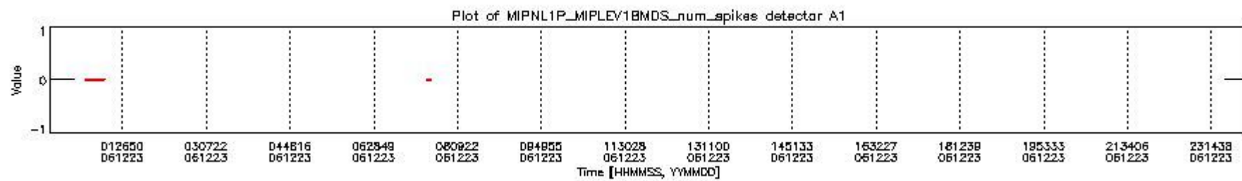
mipas_daily_report_level1_OFL_MIPAS_4_67_P_20061223_16.PNG
