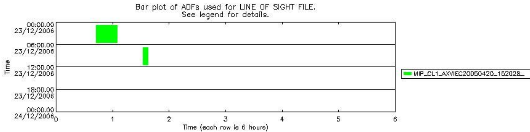
mipas_daily_report_level1_OFI_MIPAS_4_67_P_20061223_55.PNG
