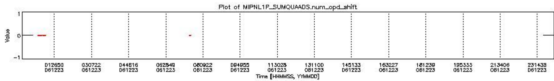
mipas_daily_report_level1_OFL_MIPAS_4_67_P_20061223_10.PNG
