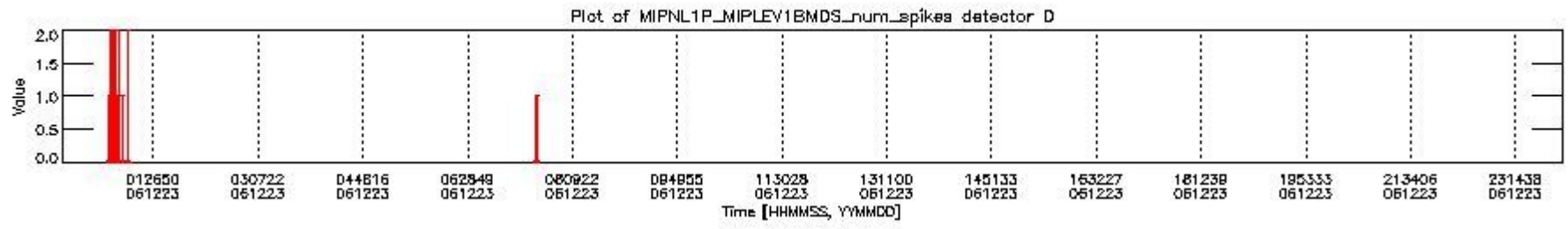
mipas_daily_report_level1_OFL_MIPAS_4_67_P_20061223_26.PNG
