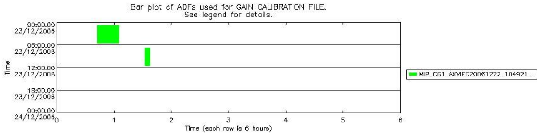
mipas_daily_report_level1_OFI_MIPAS_4_67_P_20061223_54.PNG
