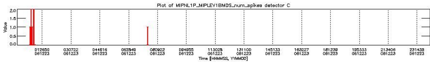
mipas_daily_report_level1_OFL_MIPAS_4_67_P_20061223_24.PNG
