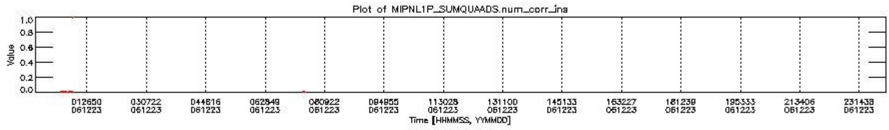
mipas_daily_report_level1_OFI_MIPAS_4_67_P_20061223_4.PNG
