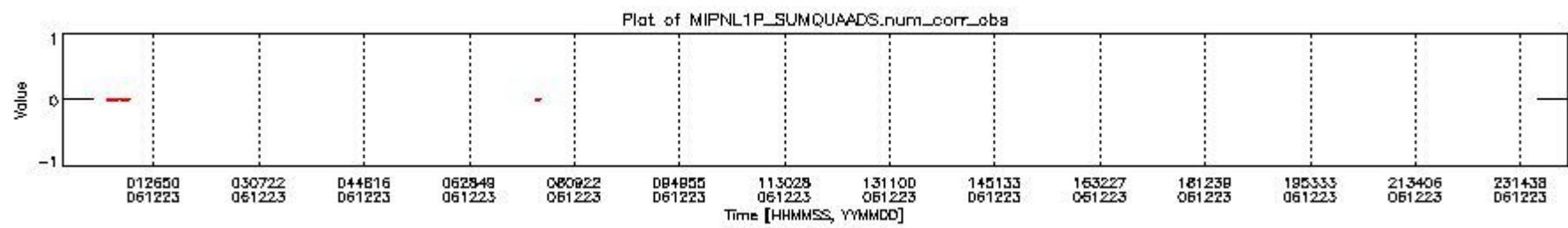
mipas_daily_report_level1_OFI_MIPAS_4_67_P_20061223_6.PNG
