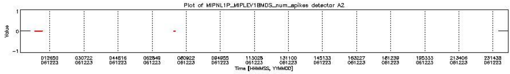
mipas_daily_report_level1_OFL_MIPAS_4_67_P_20061223_18.PNG
