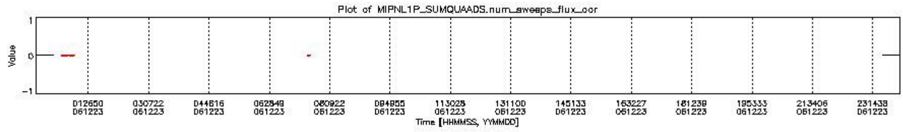
mipas_daily_report_level1_OFL_MIPAS_4_67_P_20061223_12.PNG
