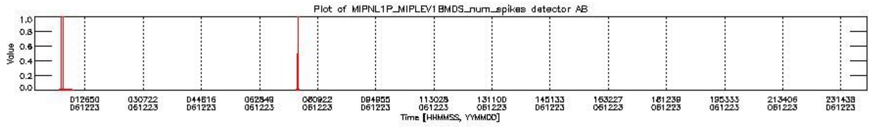
mipas_daily_report_level1_OFL_MIPAS_4_67_P_20061223_20.PNG
