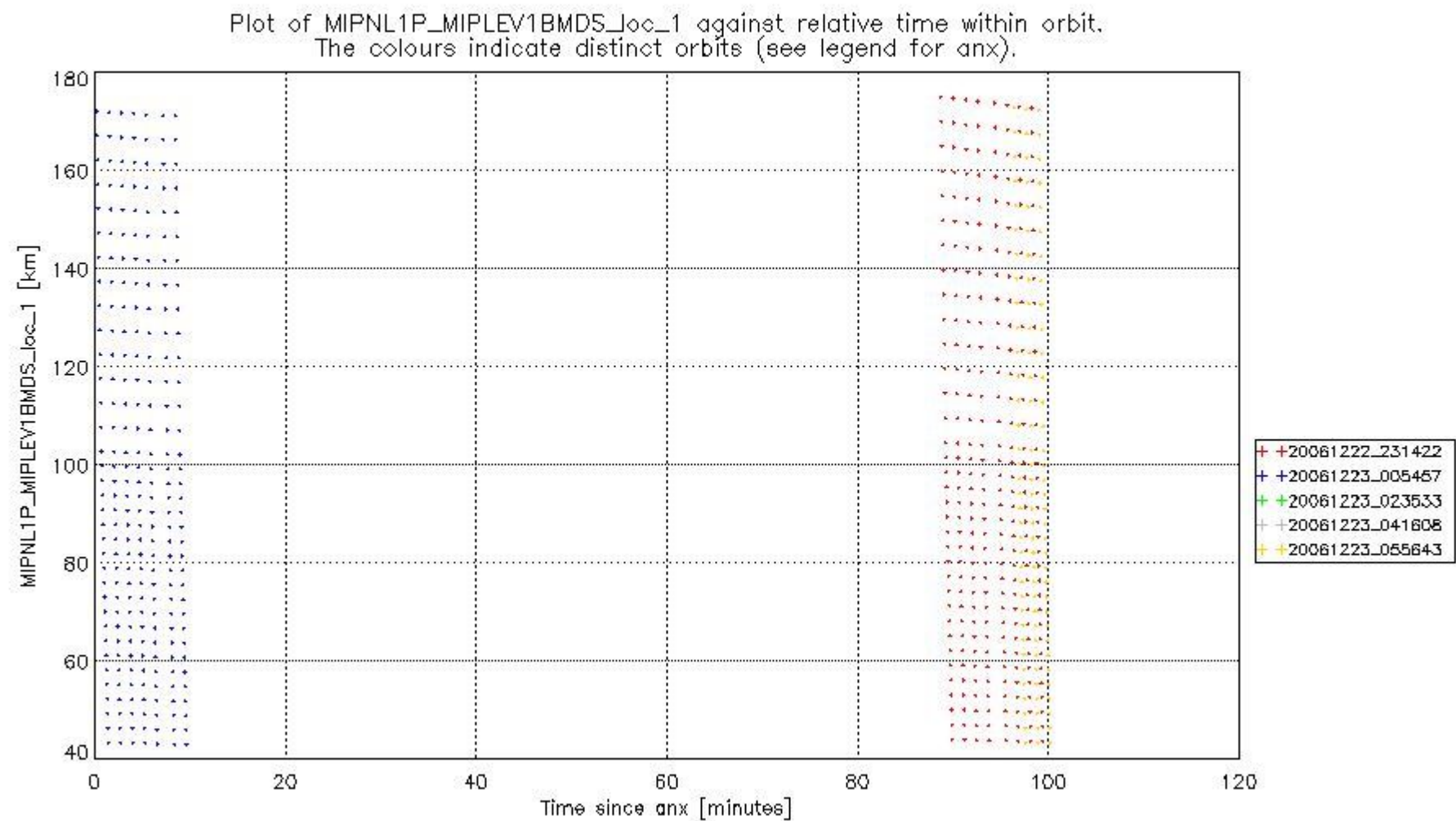
mipas_daily_report_level1_OFL_MIPAS_4_67_P_20061223_50.PNG
