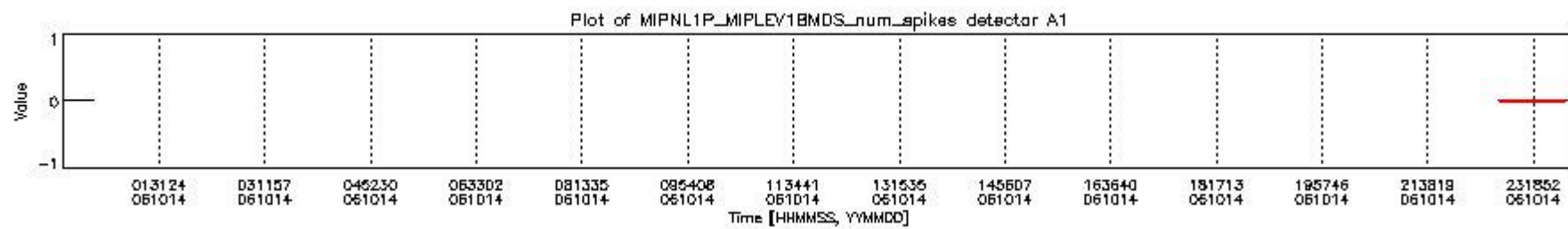
mipas_daily_report_level1_OFL_MIPAS_4_67_P_20061014_16.PNG
