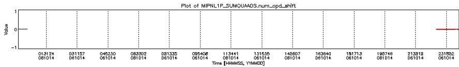
mipas_daily_report_level1_OFL_MIPAS_4_67_P_20061014_10.PNG
