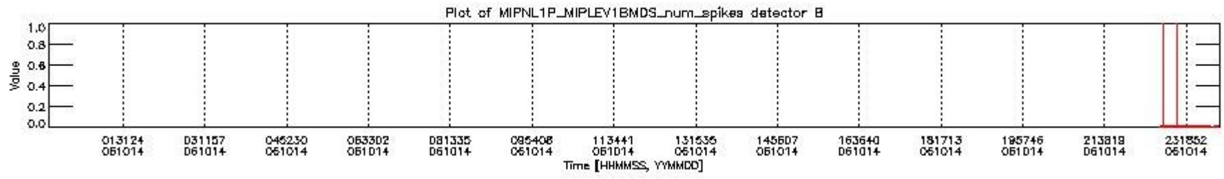
mipas_daily_report_level1_OFL_MIPAS_4_67_P_20061014_22.PNG
