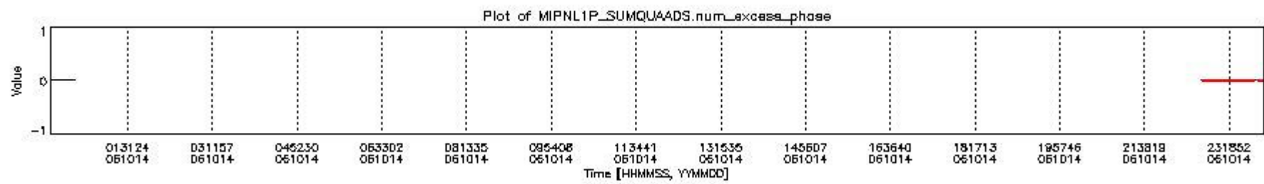
mipas_daily_report_level1_OFI_MIPAS_4_67_P_20061014_8.PNG
