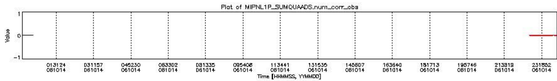
mipas_daily_report_level1_OFI_MIPAS_4_67_P_20061014_6.PNG
