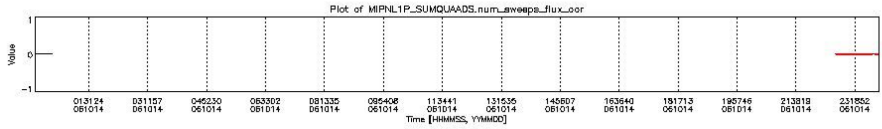
mipas_daily_report_level1_OFL_MIPAS_4_67_P_20061014_12.PNG
