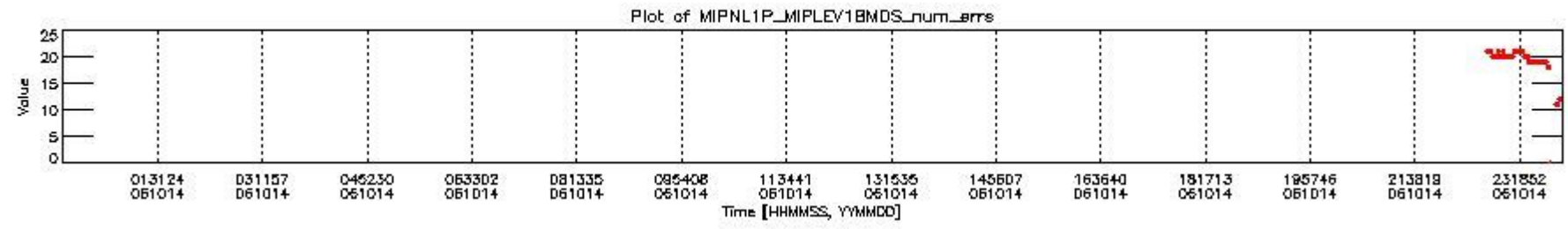
mipas_daily_report_level1_OFI_MIPAS_4_67_P_20061014_28.PNG
