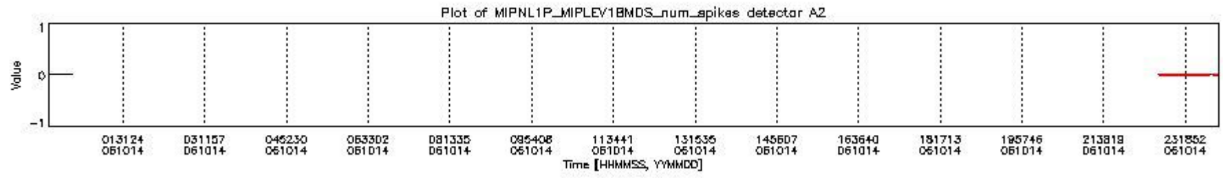
mipas_daily_report_level1_OFI_MIPAS_4_67_P_20061014_18.PNG
