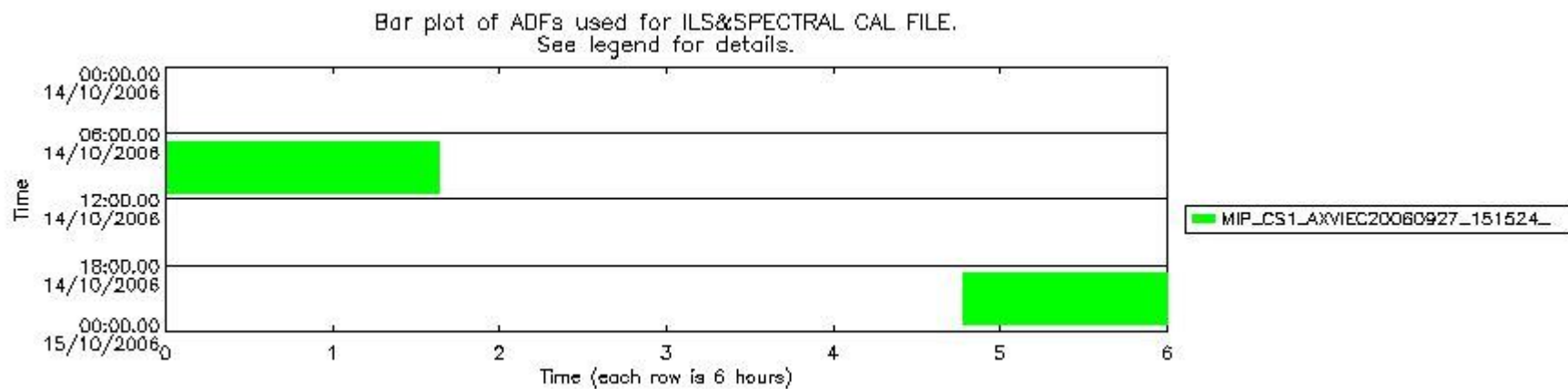
mipas_daily_report_level1_OFL_MIPAS_4_67_P_20061014_53.PNG
