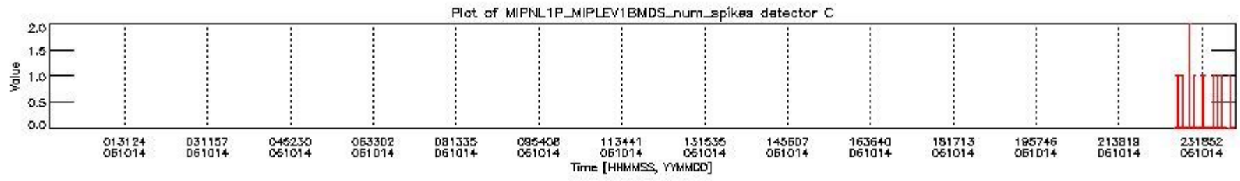
mipas_daily_report_level1_OFL_MIPAS_4_67_P_20061014_24.PNG
