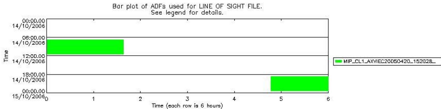
mipas_daily_report_level1_OFL_MIPAS_4_67_P_20061014_55.PNG
