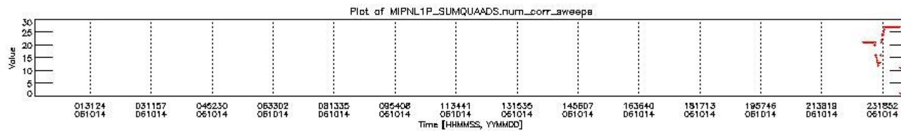
mipas_daily_report_level1_OFL_MIPAS_4_67_P_20061014_2.PNG
