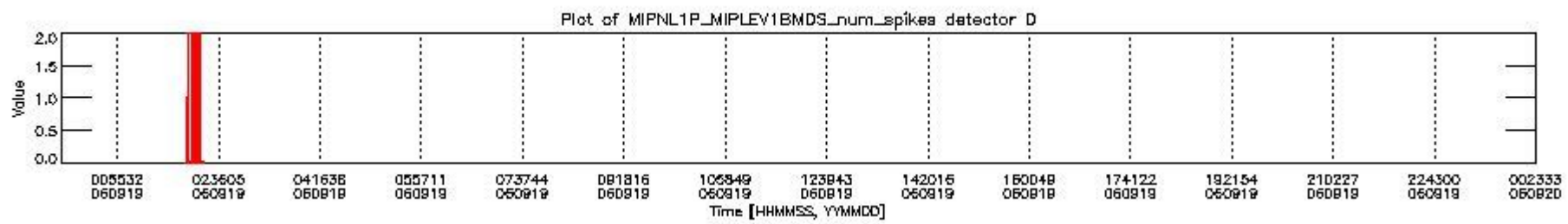
mipas_daily_report_level1_OFL_MIPAS_4_67_P_20060919_26.PNG
