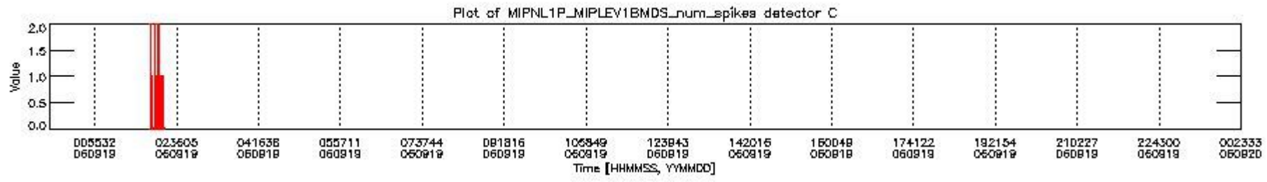
mipas_daily_report_level1_OFL_MIPAS_4_67_P_20060919_24.PNG
