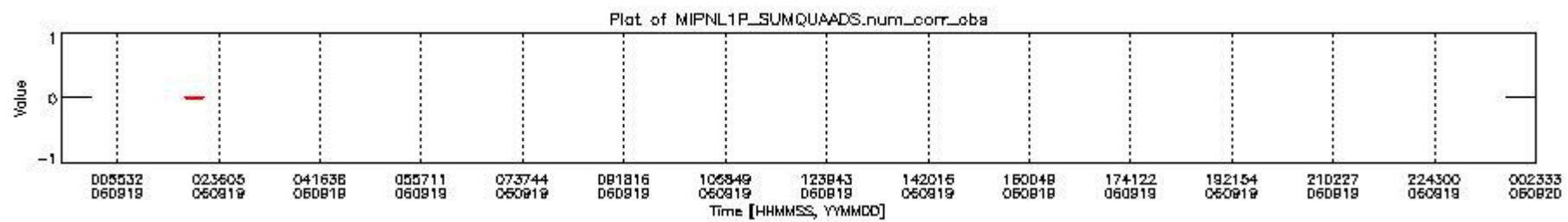
mipas_daily_report_level1_OFL_MIPAS_4_67_P_20060919_6.PNG
