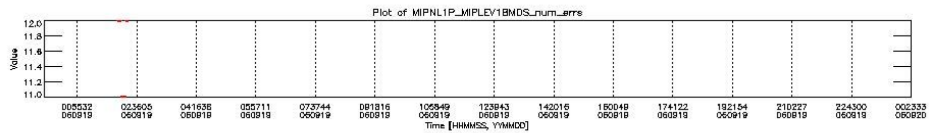
mipas_daily_report_level1_OFL_MIPAS_4_67_P_20060919_28.PNG
