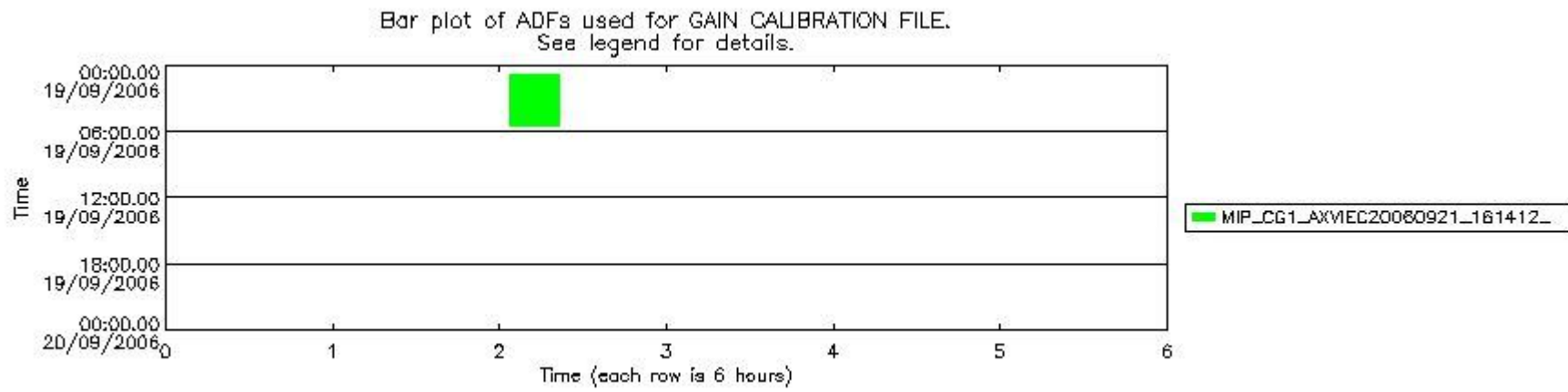
mipas_daily_report_level1_OFL_MIPAS_4_67_P_20060919_54.PNG
