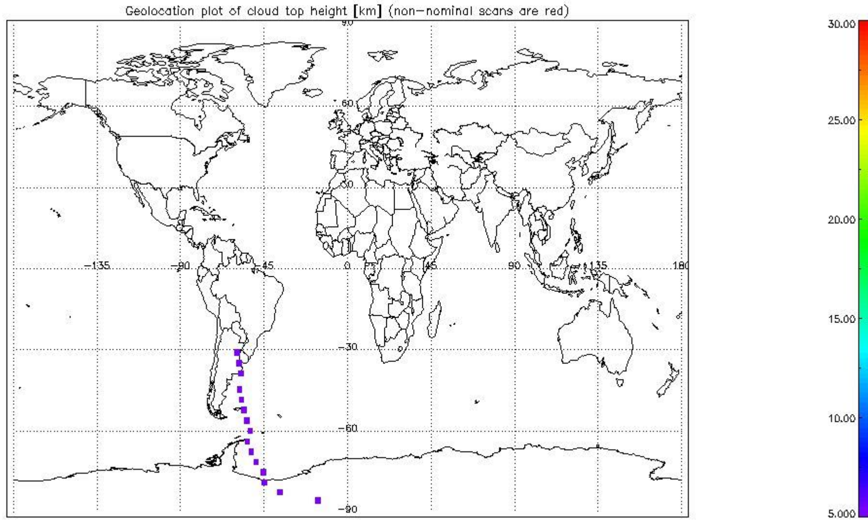
mipas_daily_report_level1_OFL_MIPAS_4_67_P_20060919_51.PNG
