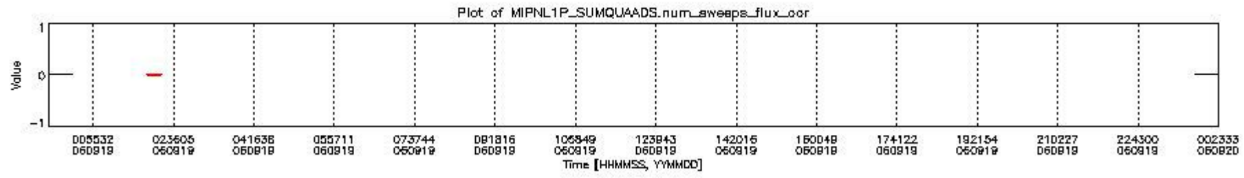
mipas_daily_report_level1_OFL_MIPAS_4_67_P_20060919_12.PNG
