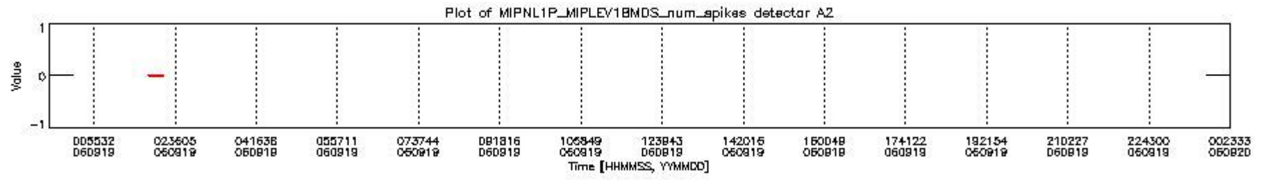
mipas_daily_report_level1_OFL_MIPAS_4_67_P_20060919_18.PNG
