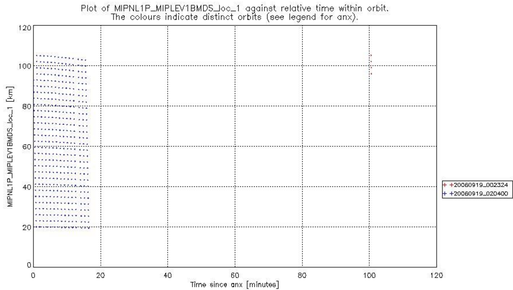
mipas_daily_report_level1_OFL_MIPAS_4_67_P_20060919_50.PNG
