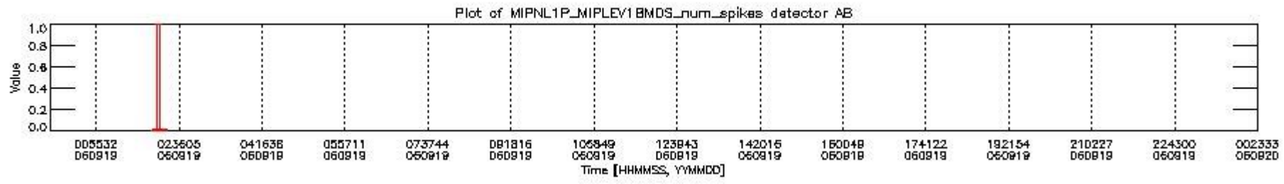
mipas_daily_report_level1_OFL_MIPAS_4_67_P_20060919_20.PNG
