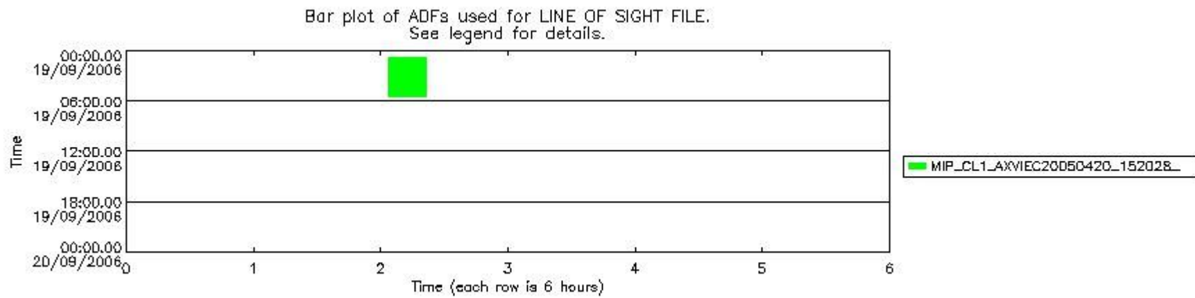
mipas_daily_report_level1_OFL_MIPAS_4_67_P_20060919_55.PNG
