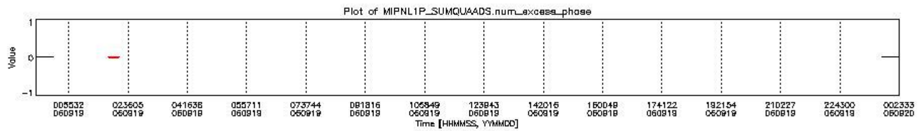
mipas_daily_report_level1_OFI_MIPAS_4_67_P_20060919_8.PNG
