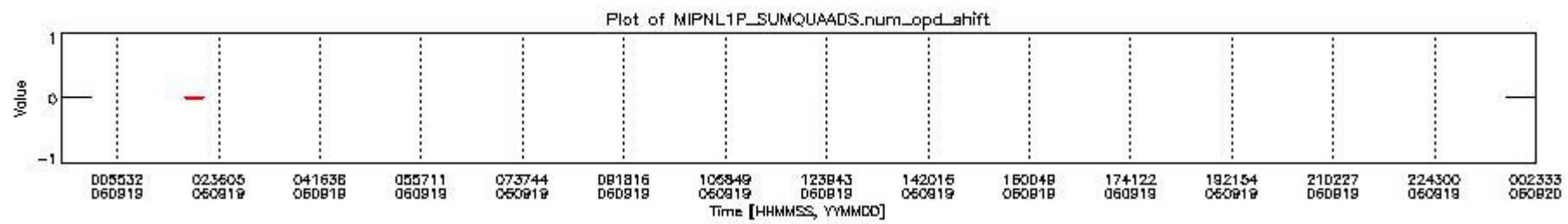
mipas_daily_report_level1_OFL_MIPAS_4_67_P_20060919_10.PNG
