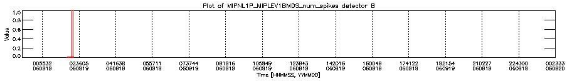
mipas_daily_report_level1_OFL_MIPAS_4_67_P_20060919_22.PNG
