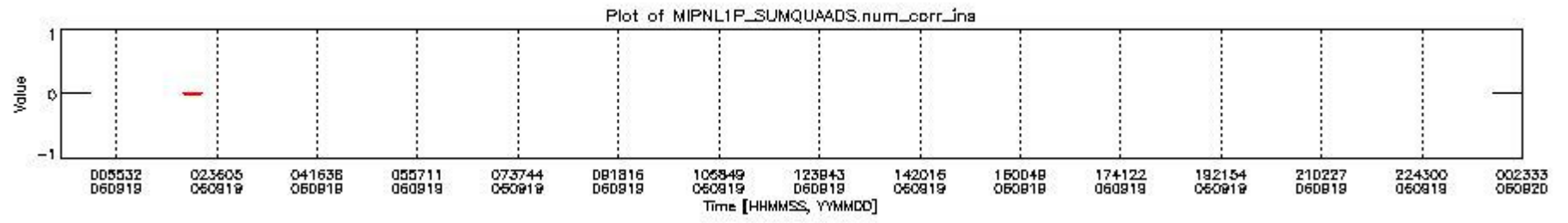
mipas_daily_report_level1_OFI_MIPAS_4_67_P_20060919_4.PNG
