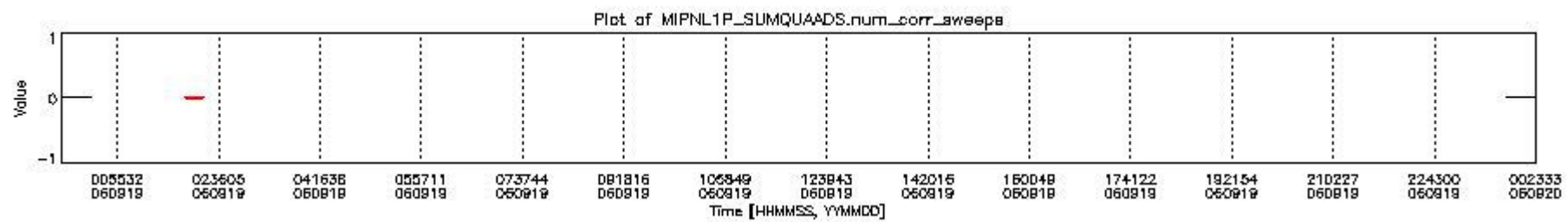
mipas_daily_report_level1_OFL_MIPAS_4_67_P_20060919_2.PNG
