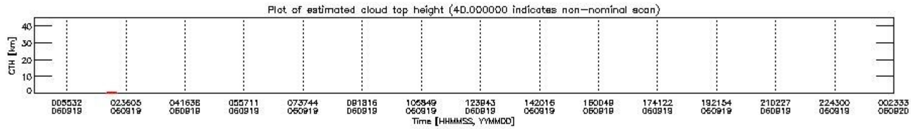
mipas_daily_report_level1_OFL_MIPAS_4_67_P_20060919_51.PNG
