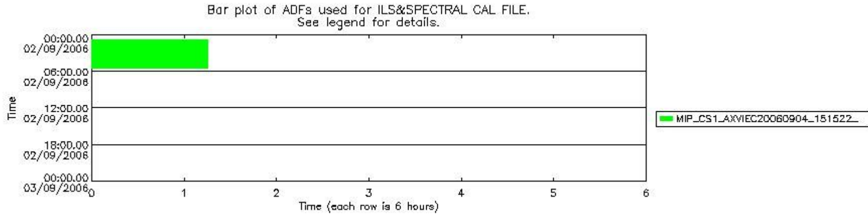
mipas_daily_report_level1_OFL_MIPAS_4_67_P_20060902_53.PNG
