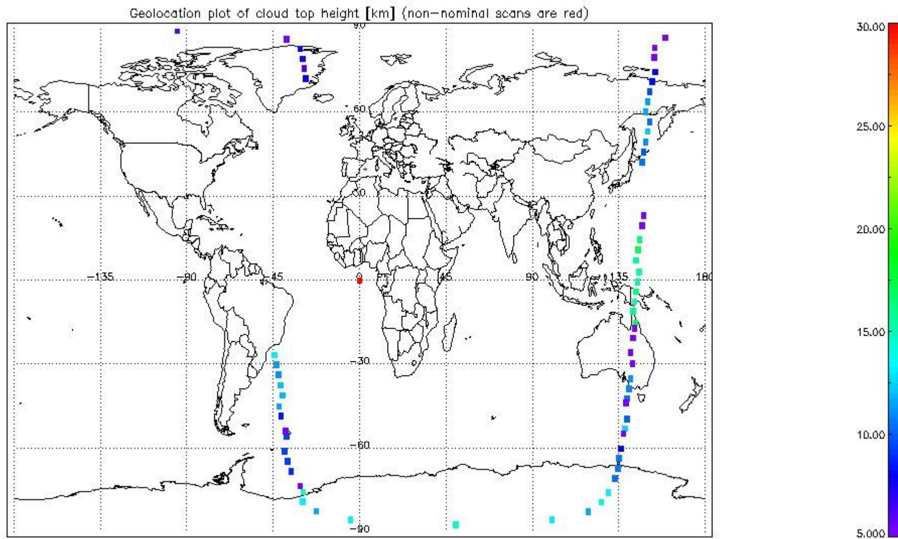
mipas_daily_report_level1_OFL_MIPAS_4_67_P_20060902_51.PNG
