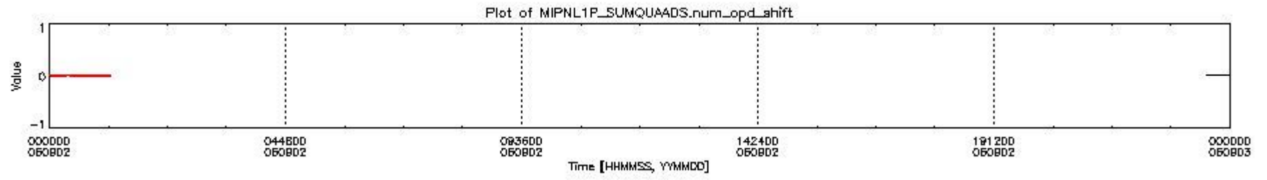
mipas_daily_report_level1_OFL_MIPAS_4_67_P_20060902_10.PNG
