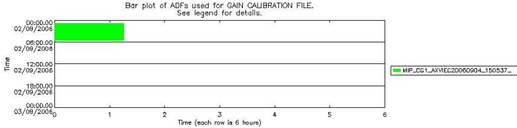
mipas_daily_report_level1_OFL_MIPAS_4_67_P_20060902_54.PNG
