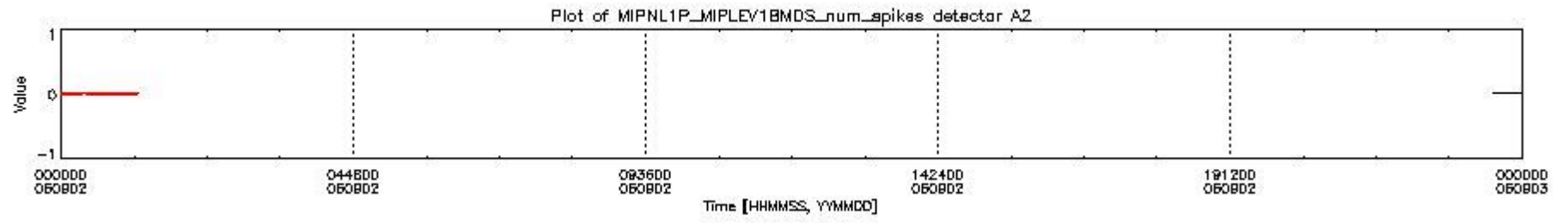
mipas_daily_report_level1_OFL_MIPAS_4_67_P_20060902_18.PNG
