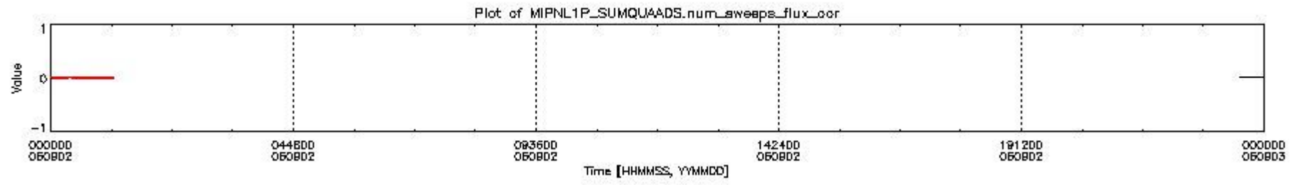
mipas_daily_report_level1_OFL_MIPAS_4_67_P_20060902_12.PNG
