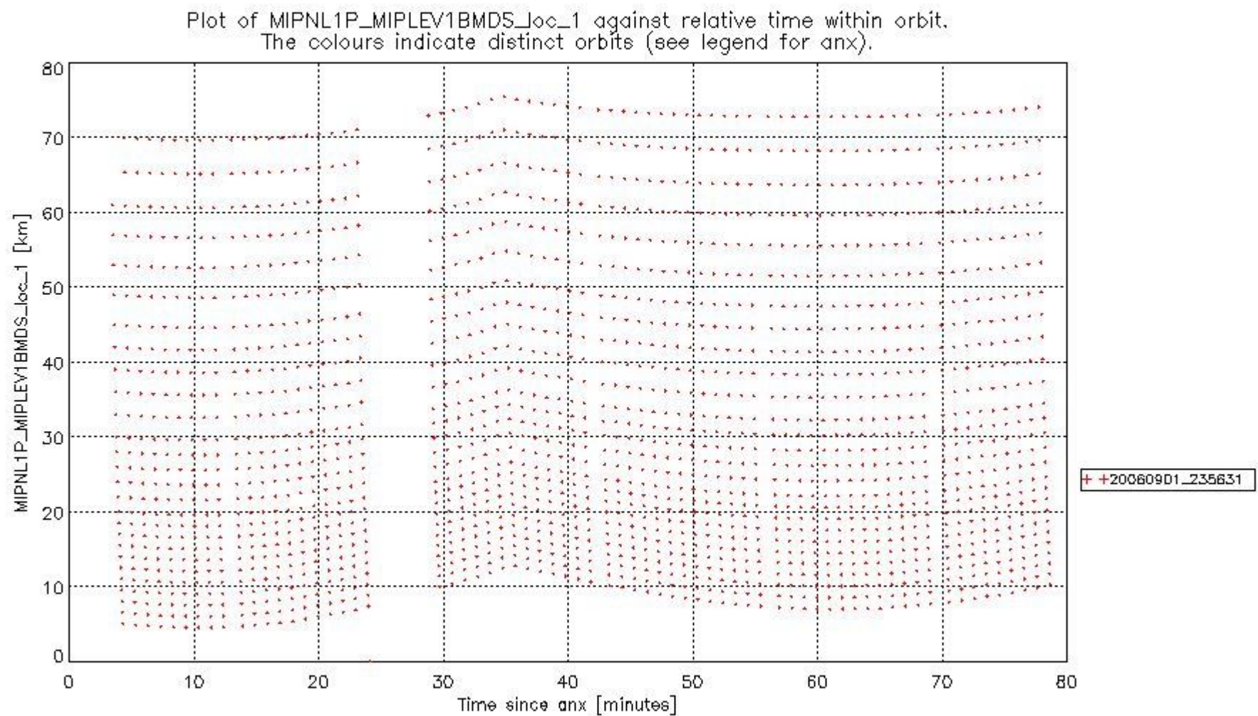
mipas_daily_report_level1_OFL_MIPAS_4_67_P_20060902_50.PNG
