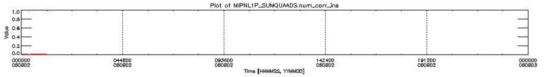
mipas_daily_report_level1_OFL_MIPAS_4_67_P_20060902_4.PNG
