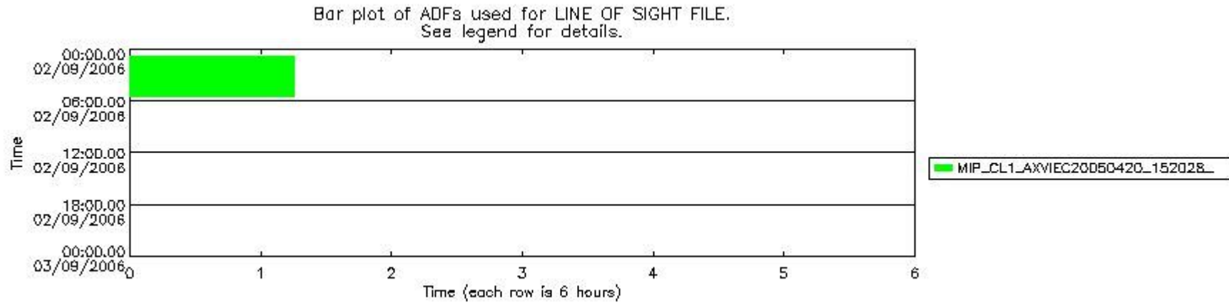
mipas_daily_report_level1_OFL_MIPAS_4_67_P_20060902_55.PNG
