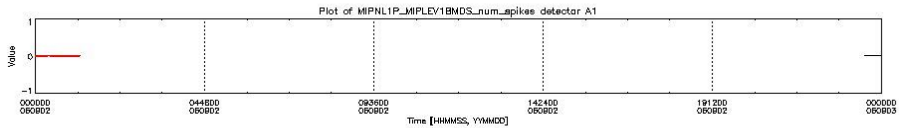
mipas_daily_report_level1_OFL_MIPAS_4_67_P_20060902_16.PNG
