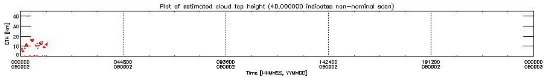
mipas_daily_report_level1_OFL_MIPAS_4_67_P_20060902_51.PNG
