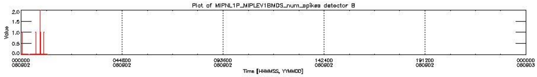
mipas_daily_report_level1_OFL_MIPAS_4_67_P_20060902_22.PNG
