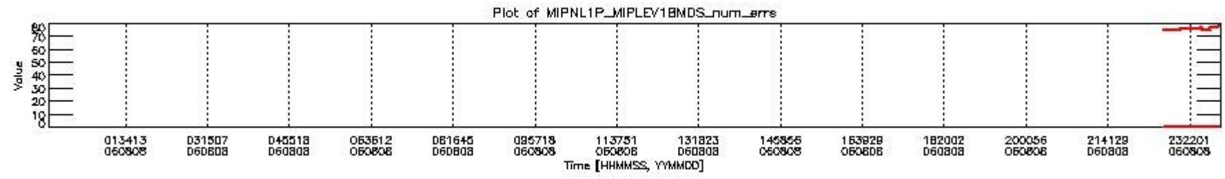
mipas_daily_report_level1_OFL_MIPAS_4_65_P_20060808_28.PNG
