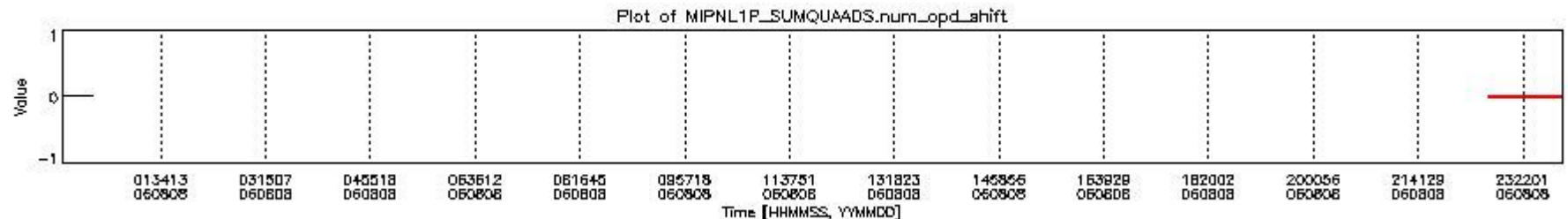
mipas_daily_report_level1_OFI_MIPAS_4_65_P_20060808_10.PNG
