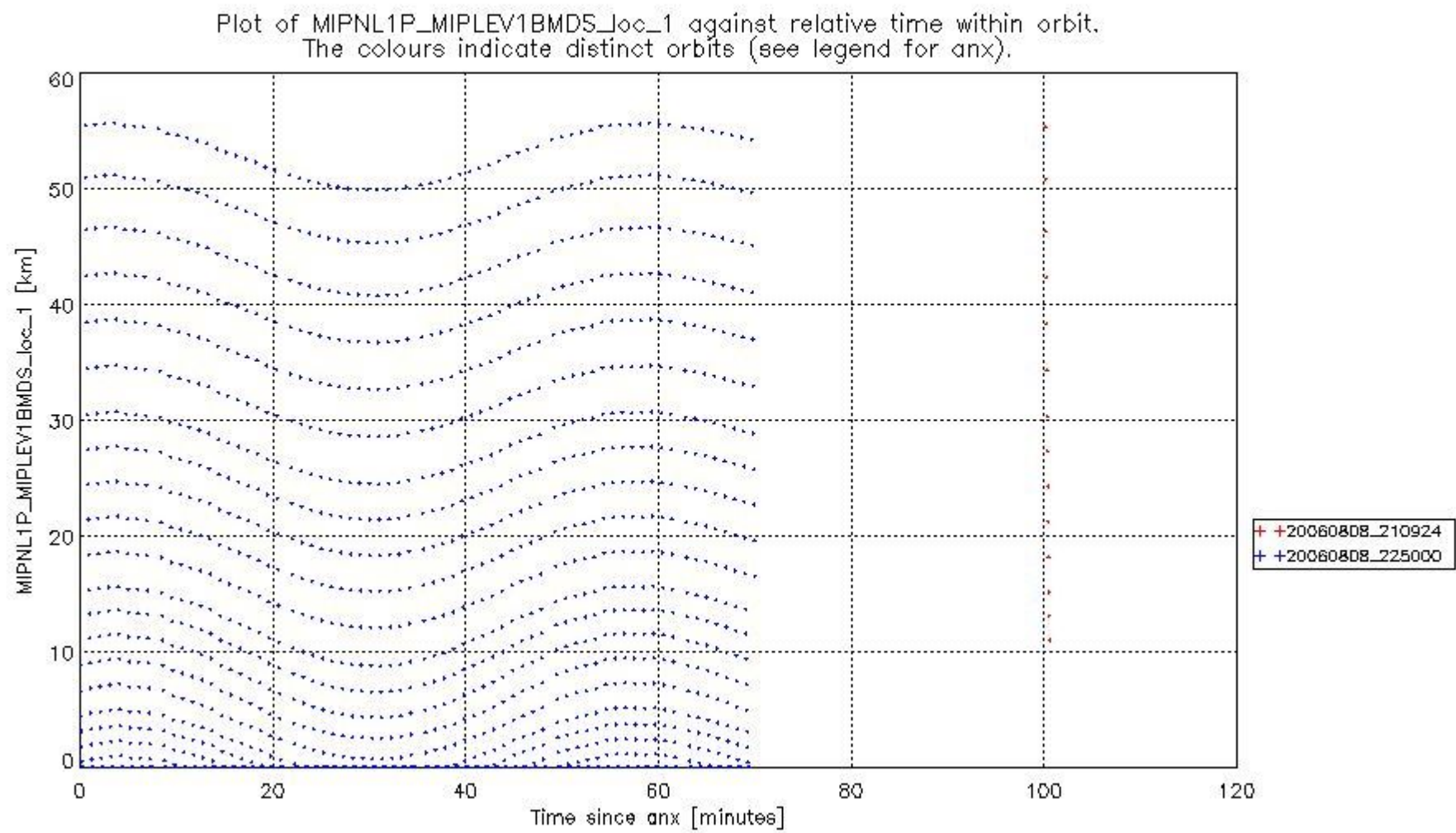
mipas_daily_report_level1_OFL_MIPAS_4_65_P_20060808_50.PNG
