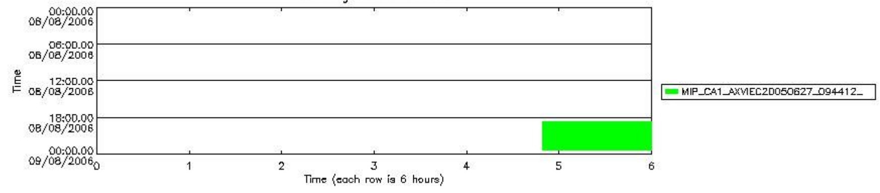
mipas_daily_report_level1_OFL_MIPAS_4_65_P_20060808_56.PNG
