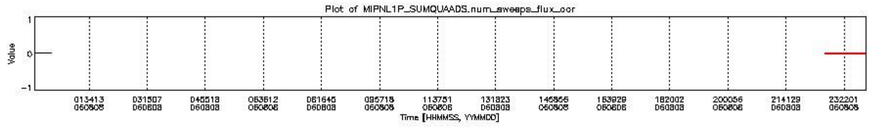
mipas_daily_report_level1_OFL_MIPAS_4_65_P_20060808_12.PNG
