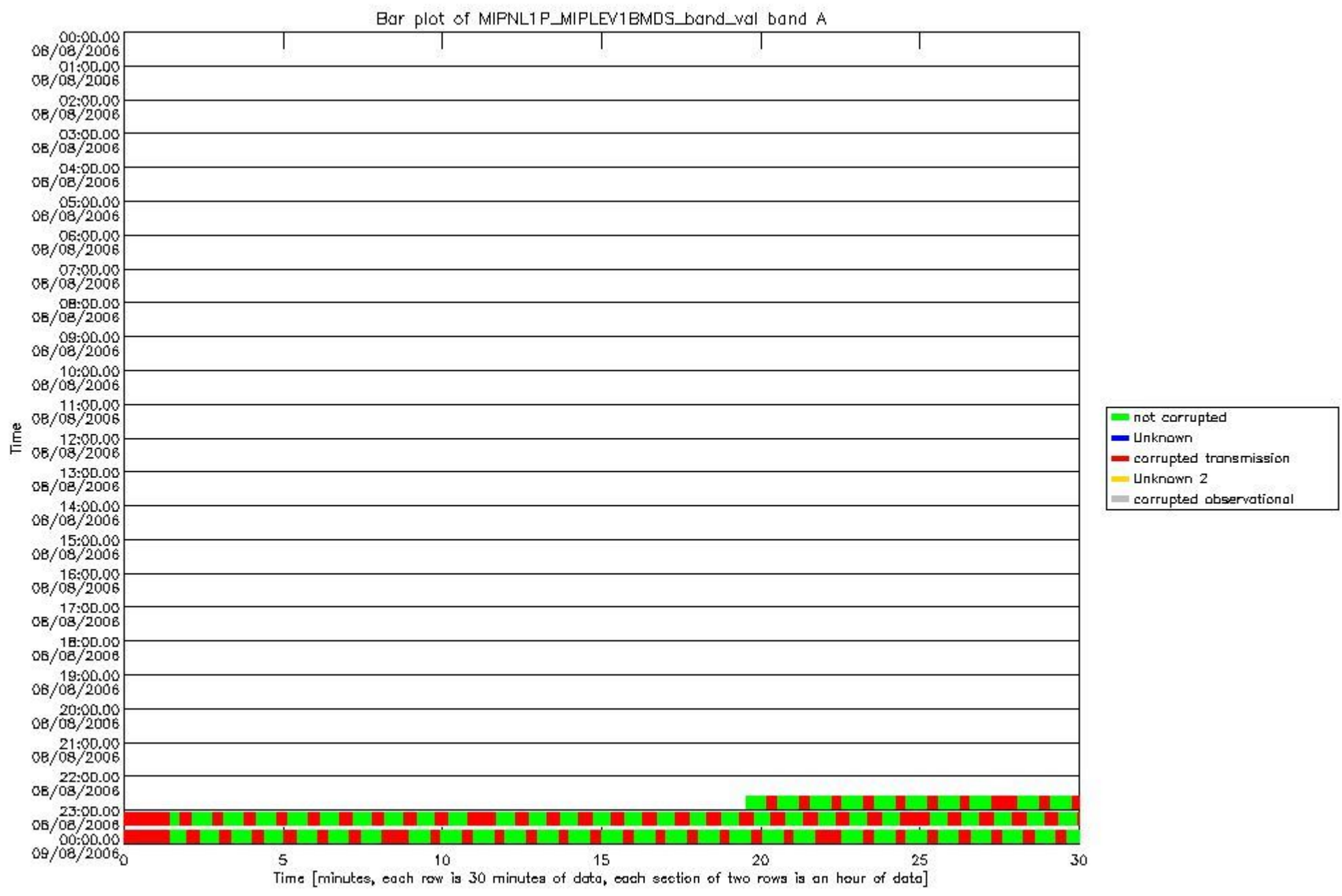
mipas_daily_report_level1_OFL_MIPAS_4_65_P_20060808_30.PNG
