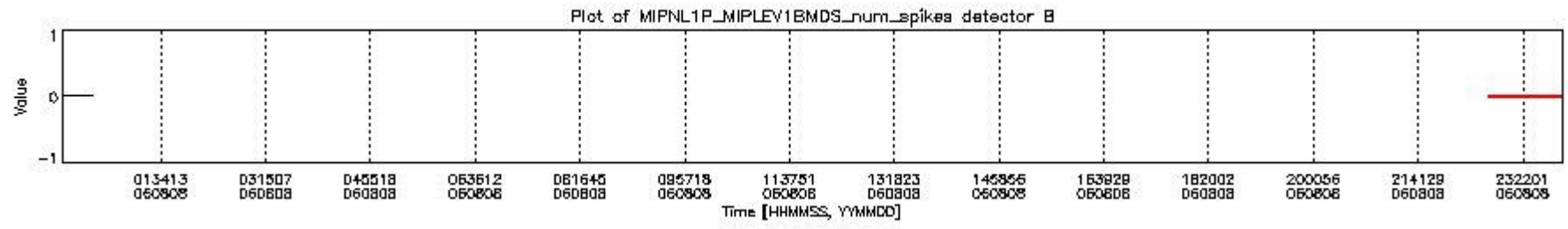
mipas_daily_report_level1_OFL_MIPAS_4_65_P_20060808_22.PNG
