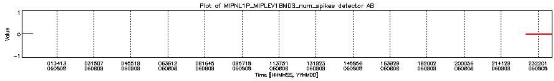
mipas_daily_report_level1_OFI_MIPAS_4_65_P_20060808_20.PNG
