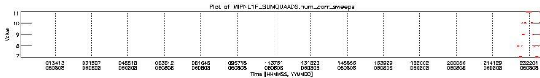
mipas_daily_report_level1_OFL_MIPAS_4_65_P_20060808_2.PNG
