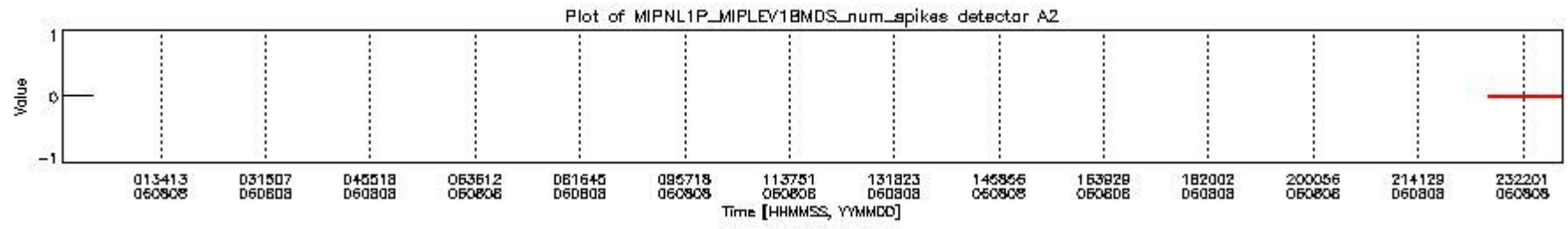
mipas_daily_report_level1_OFL_MIPAS_4_65_P_20060808_18.PNG
