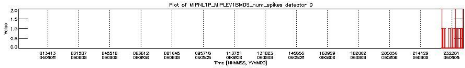
mipas_daily_report_level1_OFL_MIPAS_4_65_P_20060808_26.PNG
