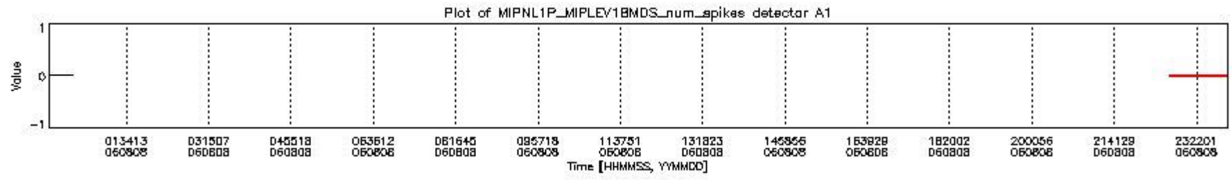
mipas_daily_report_level1_OFL_MIPAS_4_65_P_20060808_16.PNG
