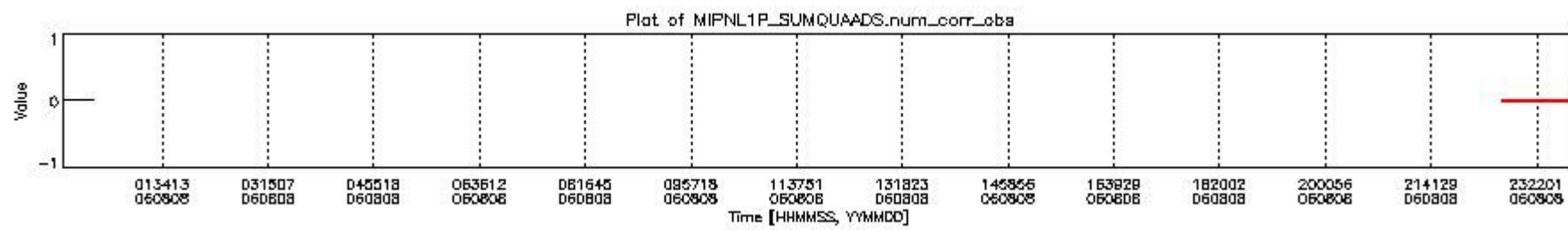
mipas_daily_report_level1_OFI_MIPAS_4_65_P_20060808_6.PNG
