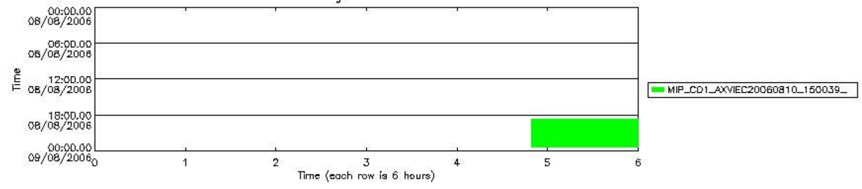
mipas_daily_report_level1_OFL_MIPAS_4_65_P_20060808_57.PNG
