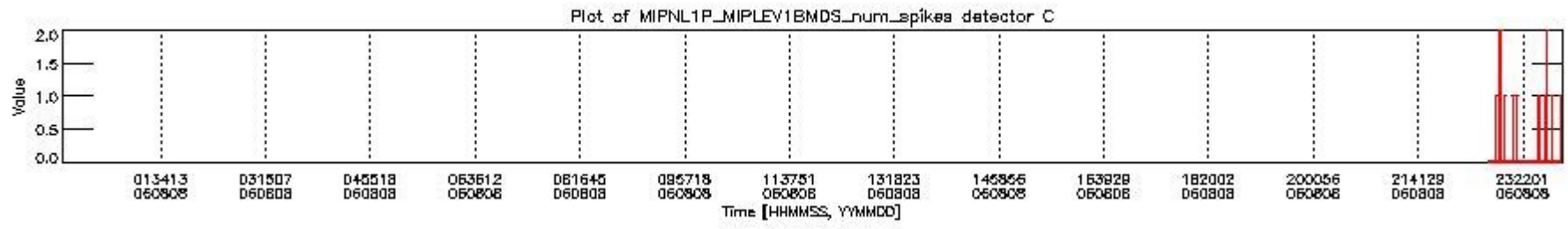
mipas_daily_report_level1_OFL_MIPAS_4_65_P_20060808_24.PNG
