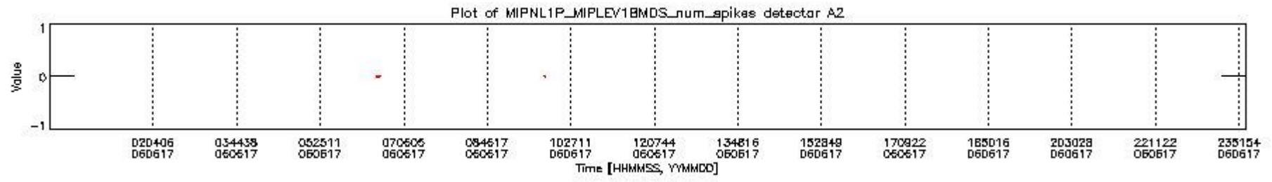
mipas_daily_report_level1_OFL_MIPAS_4_65_P_20060617_18.PNG
