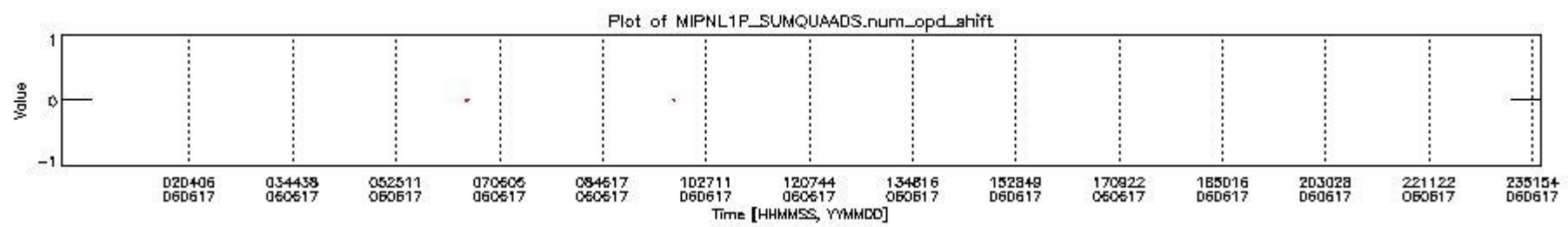
mipas_daily_report_level1_OFL_MIPAS_4_65_P_20060617_10.PNG
