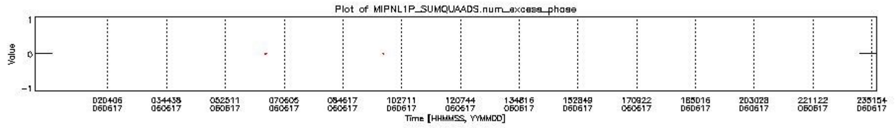
mipas_daily_report_level1_OFI_MIPAS_4_65_P_20060617_8.PNG
