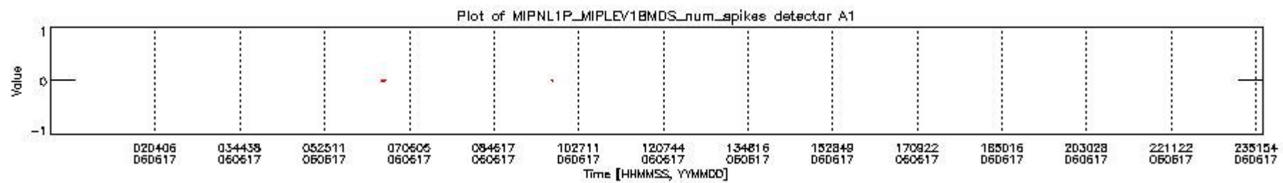
mipas_daily_report_level1_OFL_MIPAS_4_65_P_20060617_16.PNG
