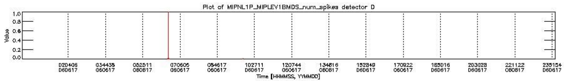
mipas_daily_report_level1_OFL_MIPAS_4_65_P_20060617_26.PNG
