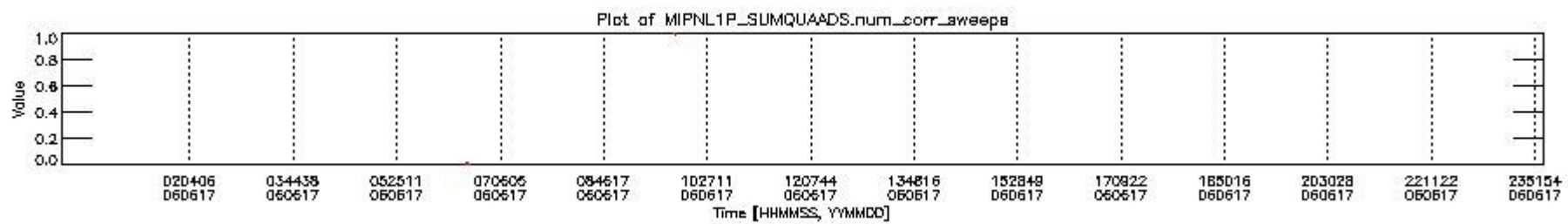
mipas_daily_report_level1_OFL_MIPAS_4_65_P_20060617_2.PNG
