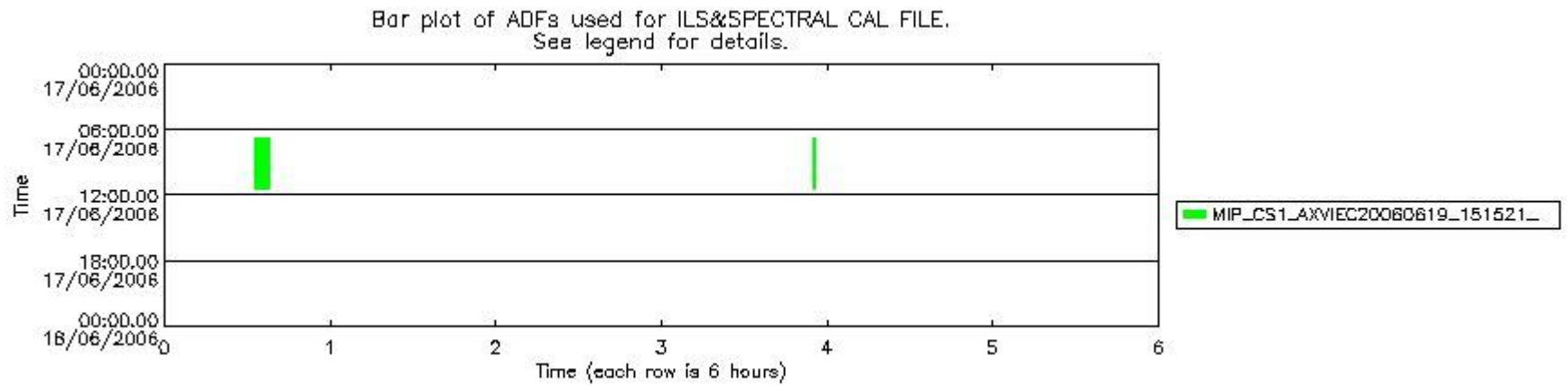
mipas_daily_report_level1_OFL_MIPAS_4_65_P_20060617_51.PNG
