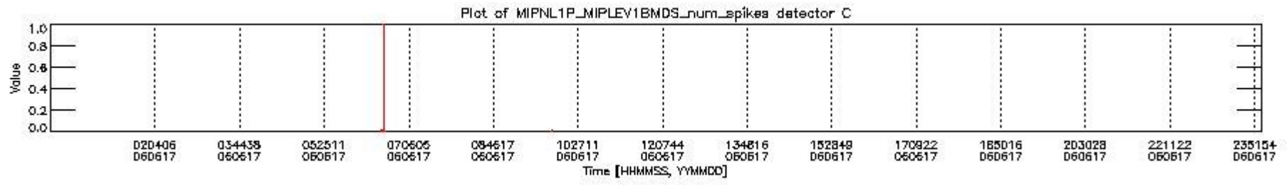
mipas_daily_report_level1_OFI_MIPAS_4_65_P_20060617_24.PNG
