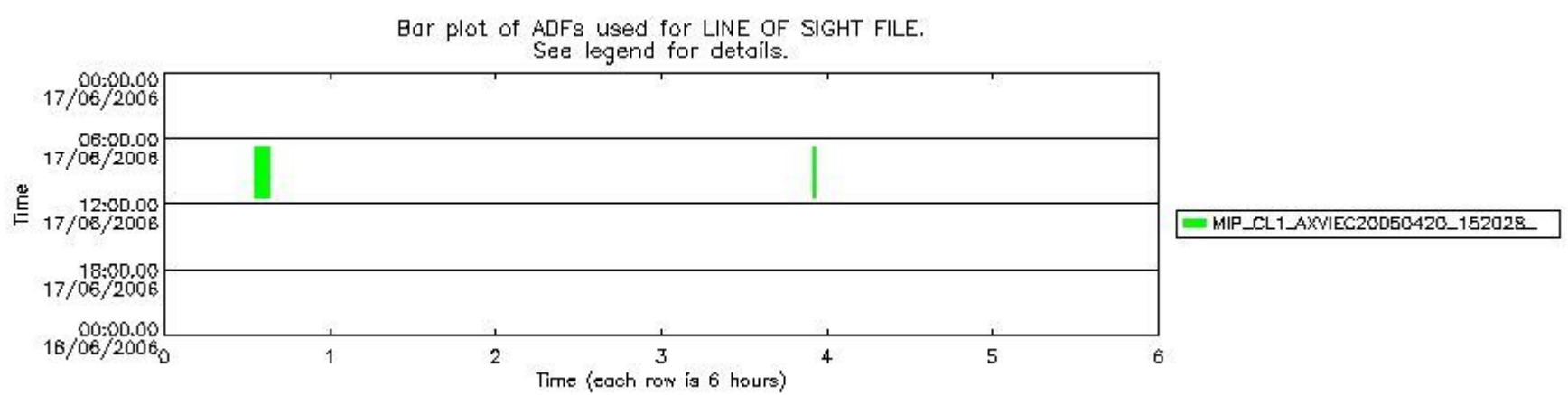
mipas_daily_report_level1_OFL_MIPAS_4_65_P_20060617_53.PNG
