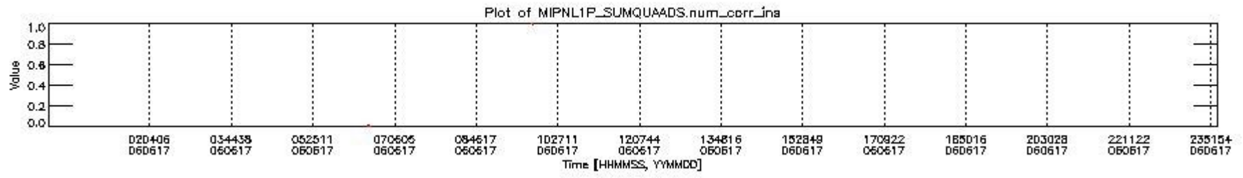
mipas_daily_report_level1_OFI_MIPAS_4_65_P_20060617_4.PNG
