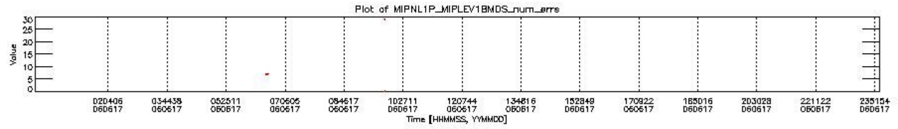
mipas_daily_report_level1_OFI_MIPAS_4_65_P_20060617_28.PNG
