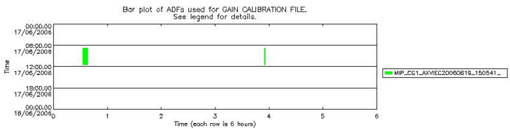
mipas_daily_report_level1_OFL_MIPAS_4_65_P_20060617_52.PNG
