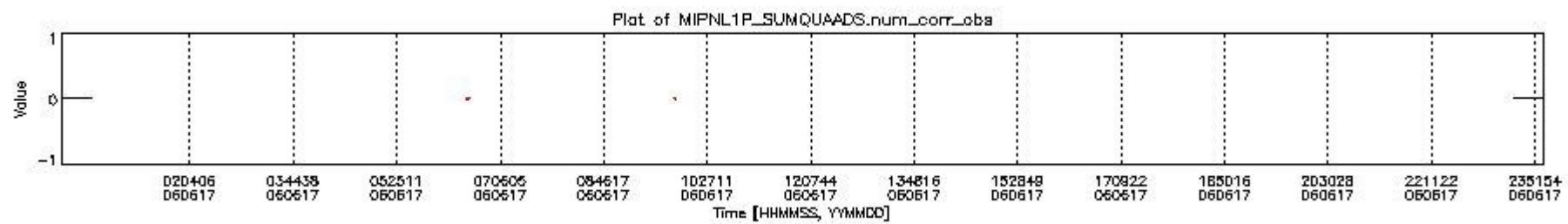
mipas_daily_report_level1_OFI_MIPAS_4_65_P_20060617_6.PNG
