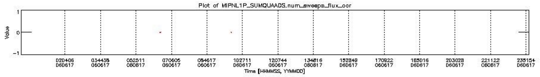
mipas_daily_report_level1_OFL_MIPAS_4_65_P_20060617_12.PNG
