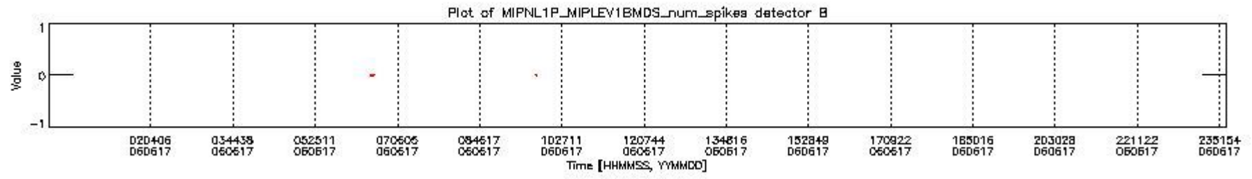
mipas_daily_report_level1_OFI_MIPAS_4_65_P_20060617_22.PNG
