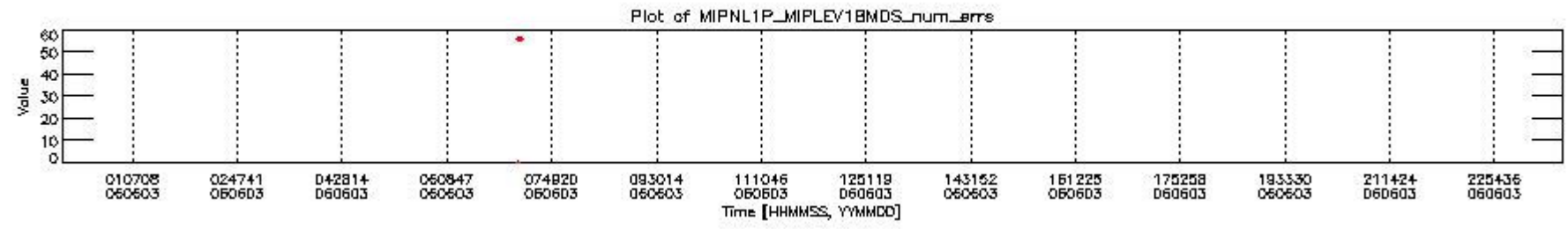
mipas_daily_report_level1_OFI_MIPAS_4_65_P_20060603_28.PNG
