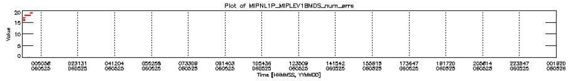
mipas_daily_report_level1_OFL_MIPAS_4_65_P_20060525_28.PNG
