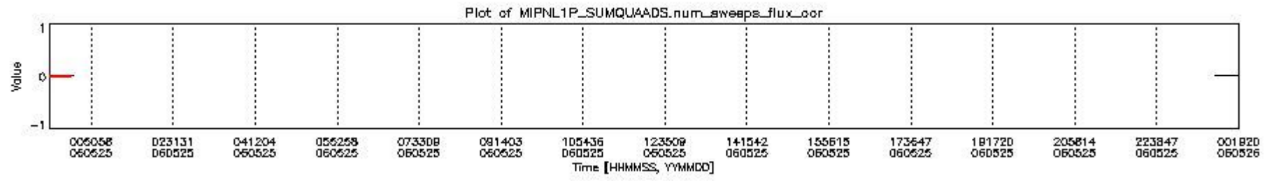
mipas_daily_report_level1_OFL_MIPAS_4_65_P_20060525_12.PNG
