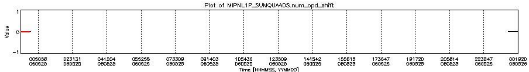
mipas_daily_report_level1_OFL_MIPAS_4_65_P_20060525_10.PNG
