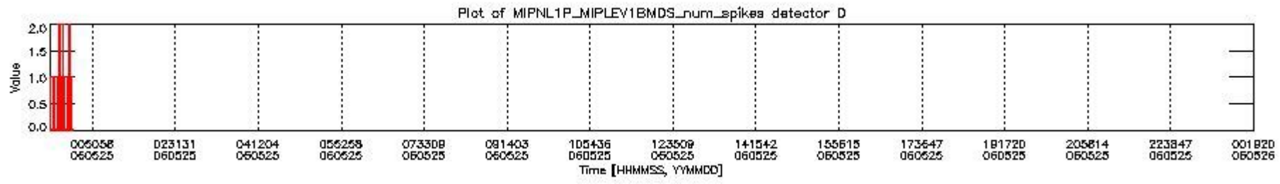
mipas_daily_report_level1_OFL_MIPAS_4_65_P_20060525_26.PNG
