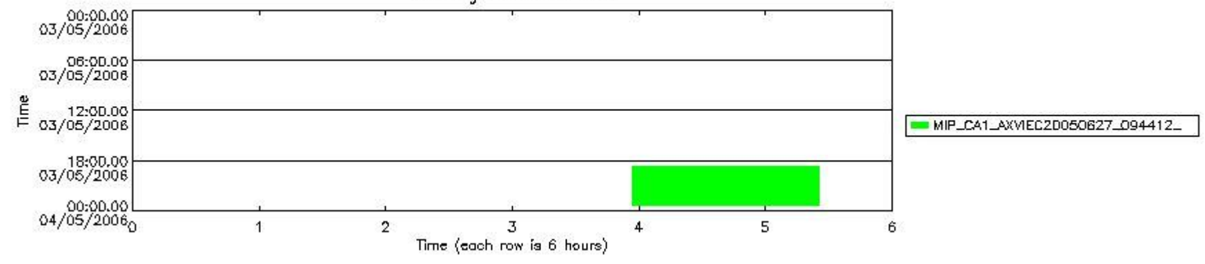
mipas_daily_report_level1_OFL_MIPAS_4_65_P_20060503_54.PNG
