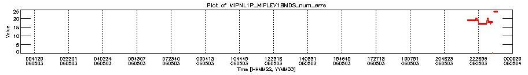
mipas_daily_report_level1_OFL_MIPAS_4_65_P_20060503_28.PNG
