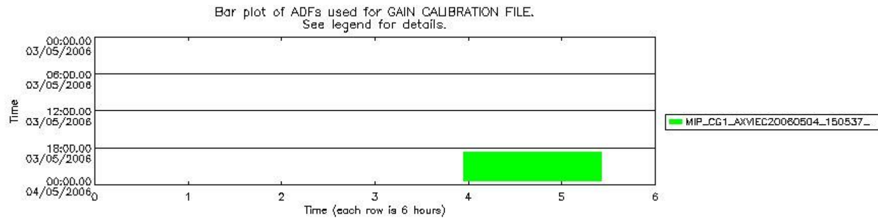
mipas_daily_report_level1_OFI_MIPAS_4_65_P_20060503_52.PNG
