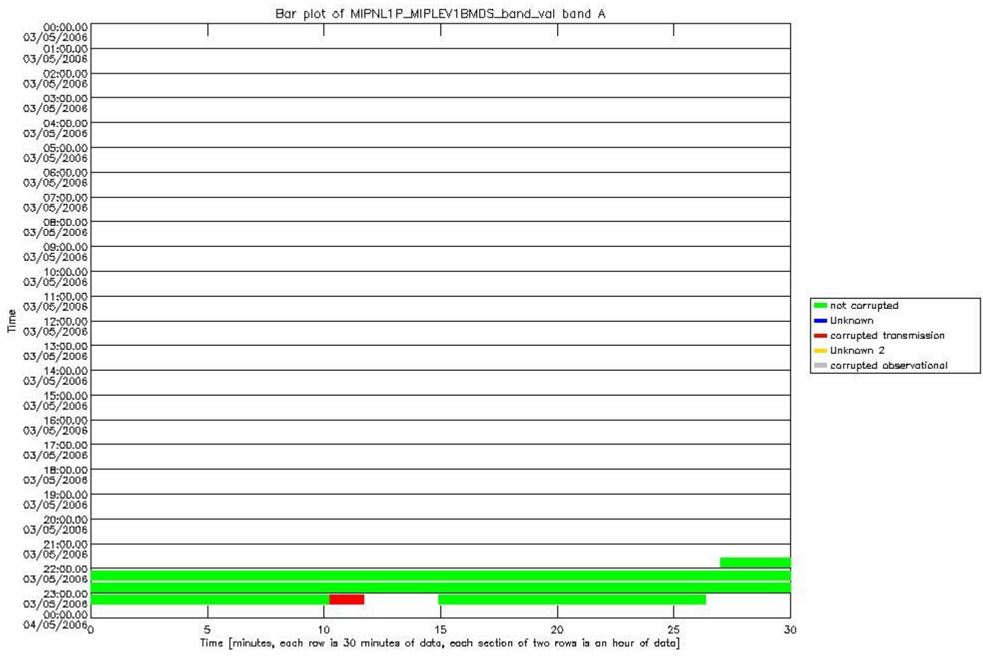
mipas_daily_report_level1_OFI_MIPAS_4_65_P_20060503_30.PNG
