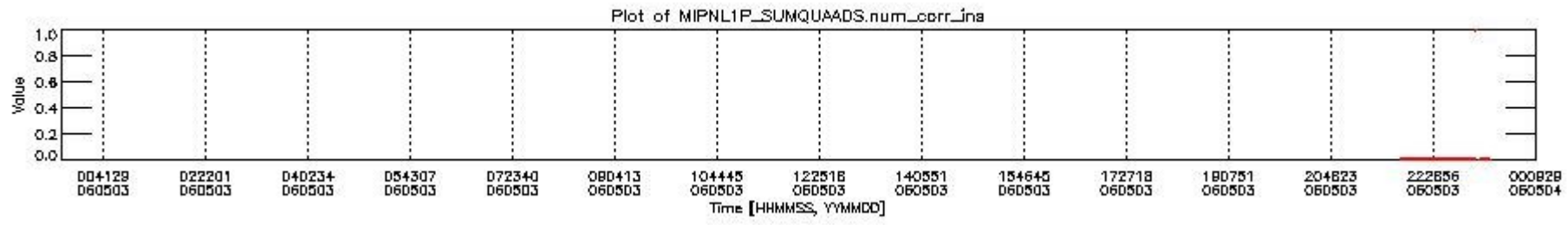
mipas_daily_report_level1_OFI_MIPAS_4_65_P_20060503_4.PNG
