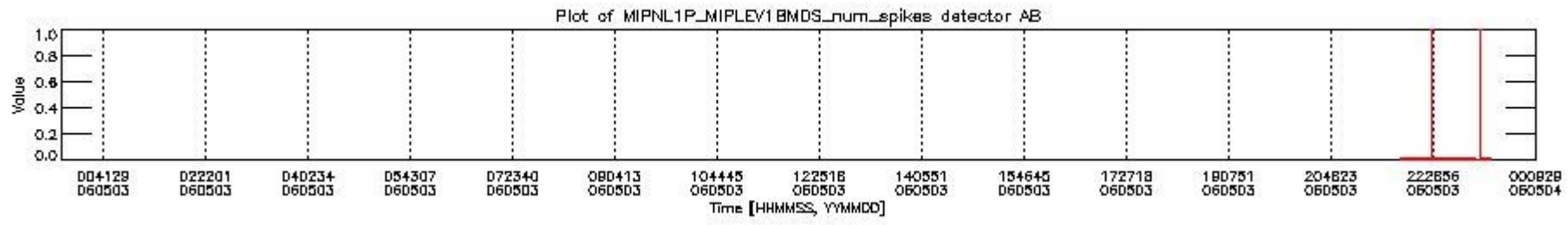
mipas_daily_report_level1_OFL_MIPAS_4_65_P_20060503_20.PNG
