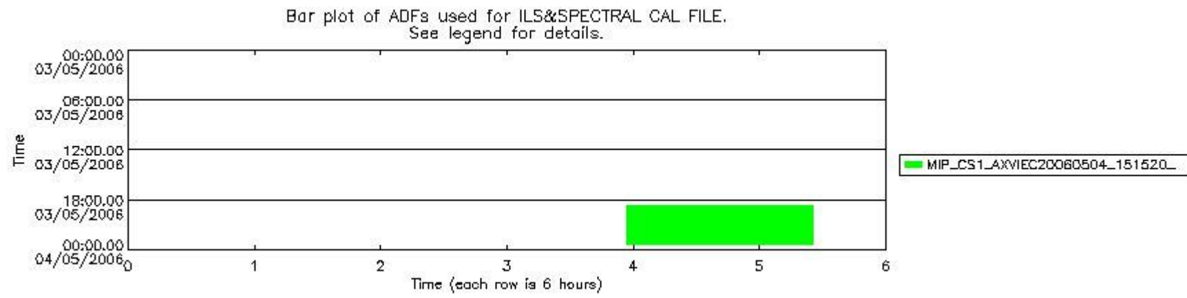
mipas_daily_report_level1_OFI_MIPAS_4_65_P_20060503_51.PNG
