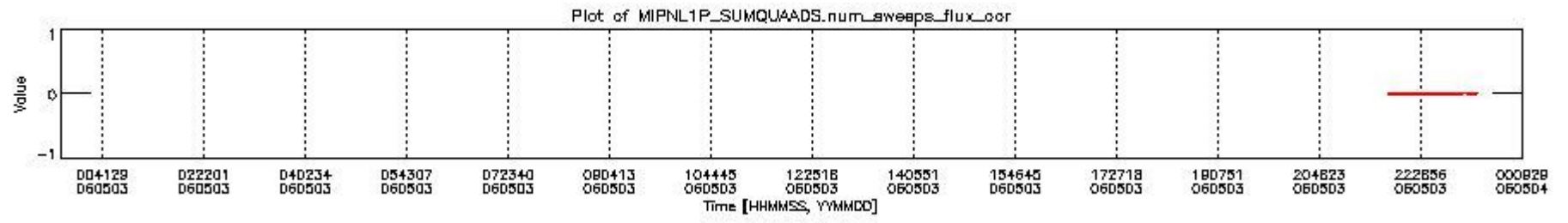
mipas_daily_report_level1_OFL_MIPAS_4_65_P_20060503_12.PNG
