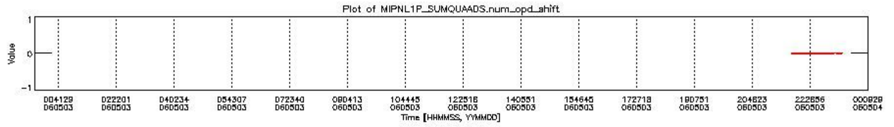
mipas_daily_report_level1_OFL_MIPAS_4_65_P_20060503_10.PNG
