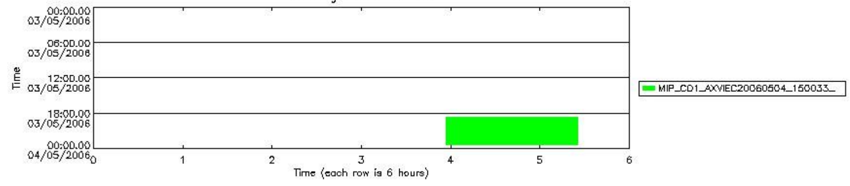
mipas_daily_report_level1_OFL_MIPAS_4_65_P_20060503_55.PNG
