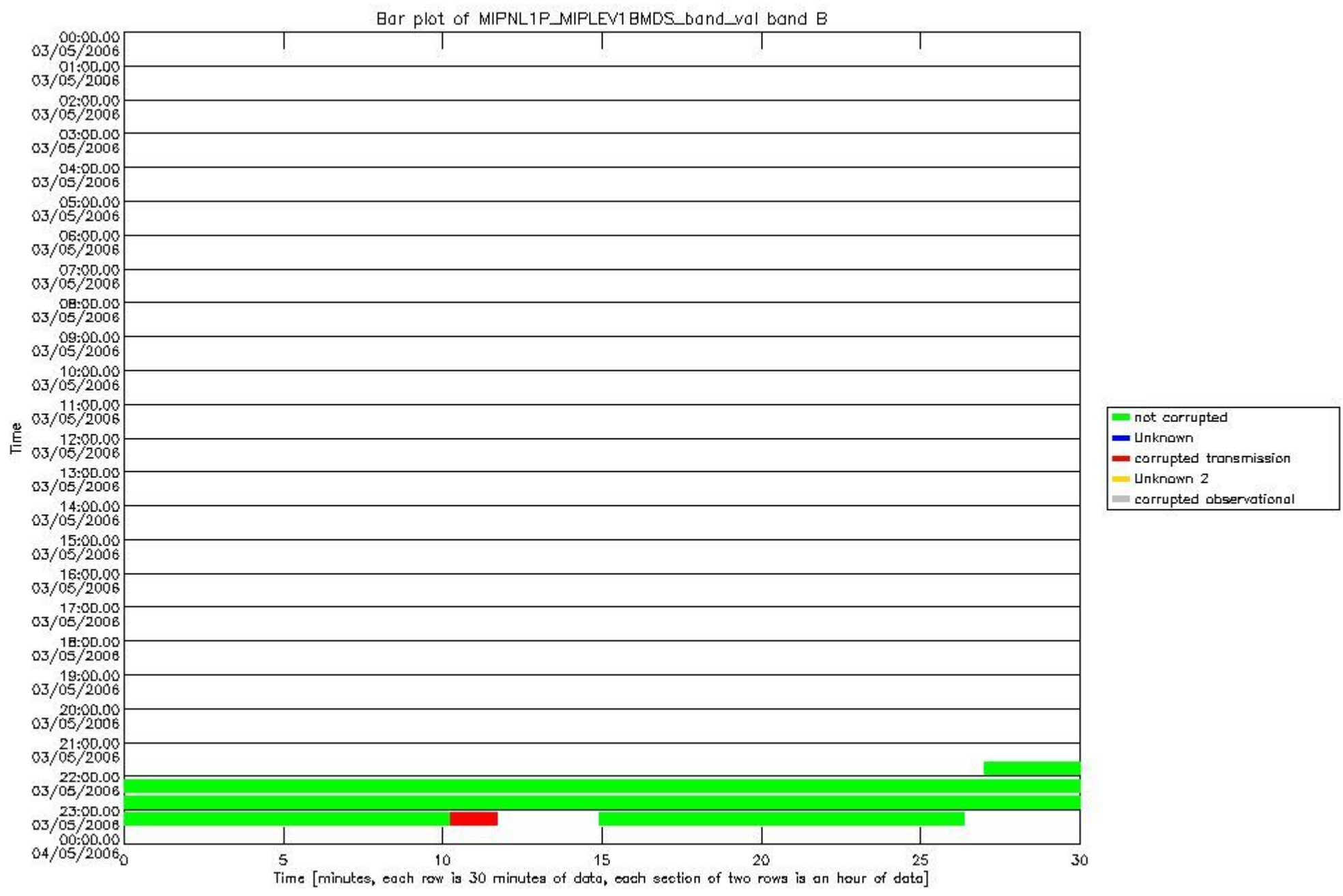
mipas_daily_report_level1_OFI_MIPAS_4_65_P_20060503_34.PNG
