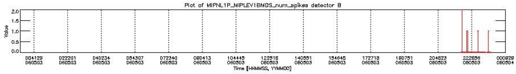
mipas_daily_report_level1_OFL_MIPAS_4_65_P_20060503_22.PNG
