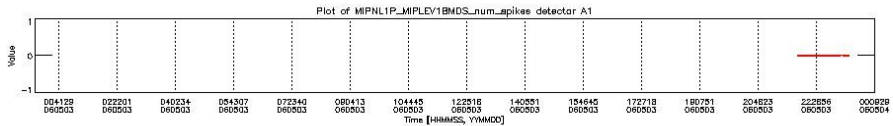
mipas_daily_report_level1_OFL_MIPAS_4_65_P_20060503_16.PNG
