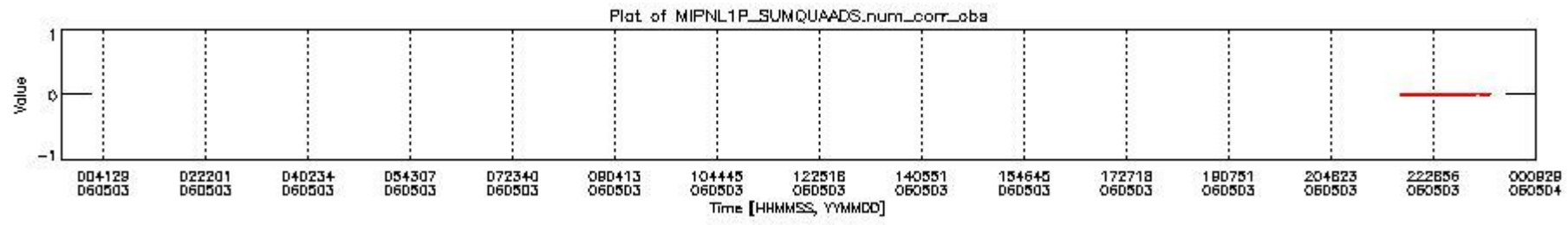
mipas_daily_report_level1_OFI_MIPAS_4_65_P_20060503_6.PNG
