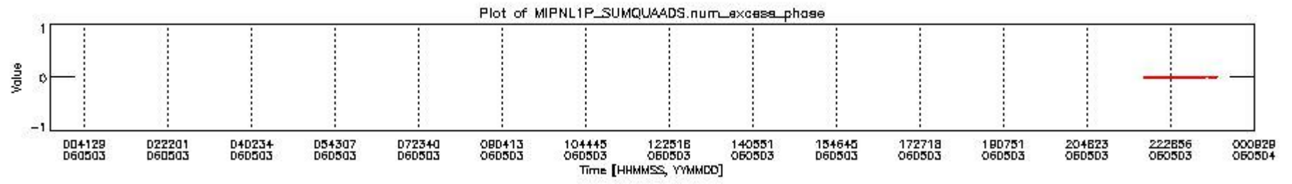
mipas_daily_report_level1_OFI_MIPAS_4_65_P_20060503_8.PNG
