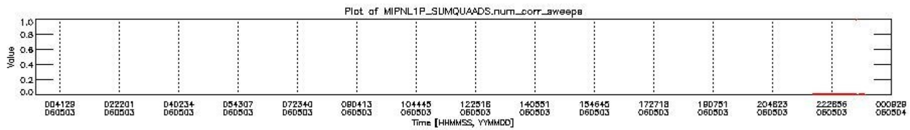
mipas_daily_report_level1_OFI_MIPAS_4_65_P_20060503_2.PNG
