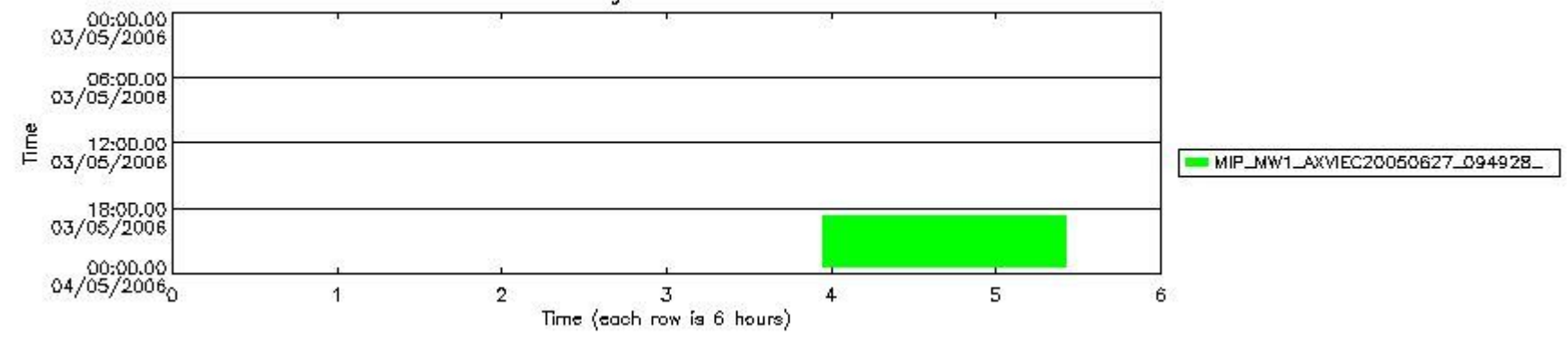
mipas_daily_report_level1_OFL_MIPAS_4_65_P_20060503_56.PNG
