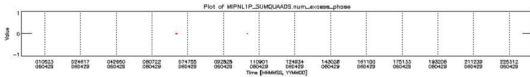
mipas_daily_report_level1_OFI_MIPAS_4_65_P_20060429_8.PNG
