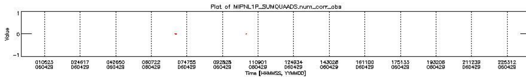
mipas_daily_report_level1_OFI_MIPAS_4_65_P_20060429_6.PNG
