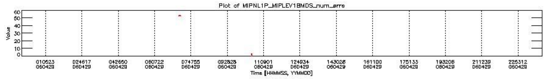
mipas_daily_report_level1_OFI_MIPAS_4_65_P_20060429_28.PNG
