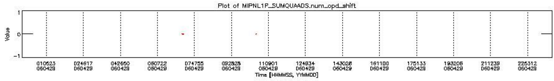
mipas_daily_report_level1_OFI_MIPAS_4_65_P_20060429_10.PNG
