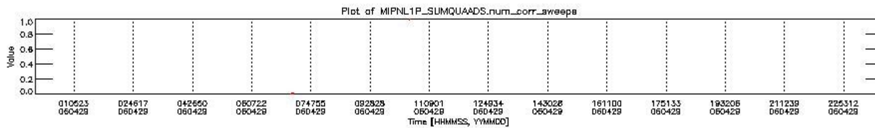
mipas_daily_report_level1_OFI_MIPAS_4_65_P_20060429_2.PNG
