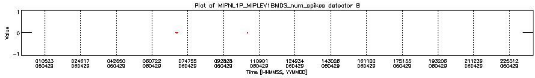
mipas_daily_report_level1_OFI_MIPAS_4_65_P_20060429_22.PNG
