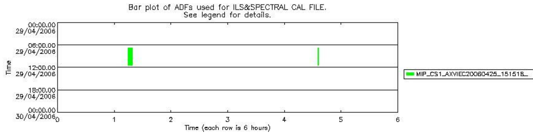
mipas_daily_report_level1_OFL_MIPAS_4_65_P_20060429_51.PNG
