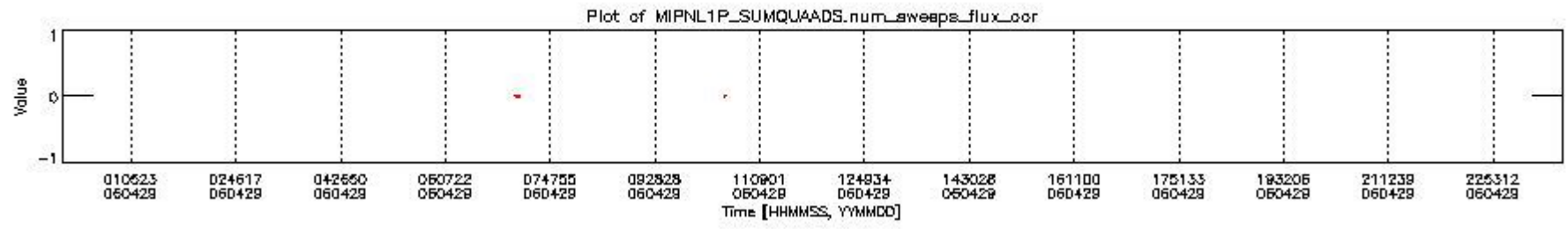
mipas_daily_report_level1_OFI_MIPAS_4_65_P_20060429_12.PNG
