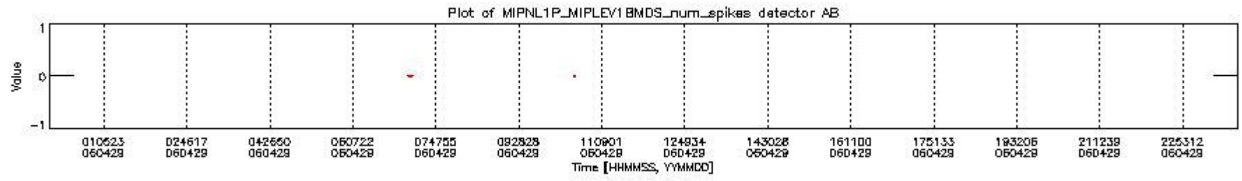
mipas_daily_report_level1_OFI_MIPAS_4_65_P_20060429_20.PNG
