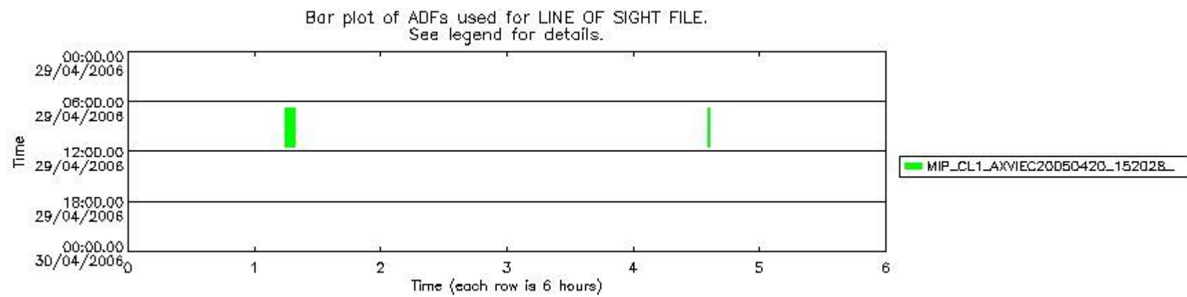
mipas_daily_report_level1_OFL_MIPAS_4_65_P_20060429_53.PNG
