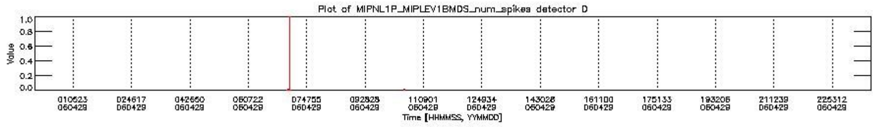
mipas_daily_report_level1_OFL_MIPAS_4_65_P_20060429_26.PNG
