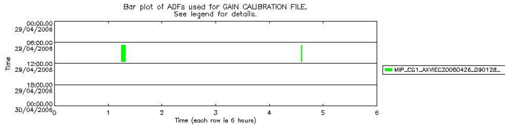
mipas_daily_report_level1_OFL_MIPAS_4_65_P_20060429_52.PNG
