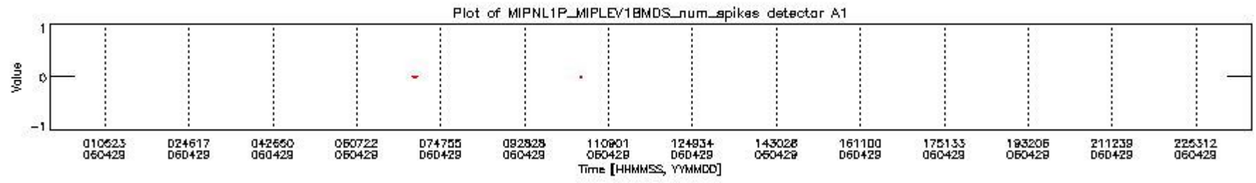
mipas_daily_report_level1_OFL_MIPAS_4_65_P_20060429_16.PNG
