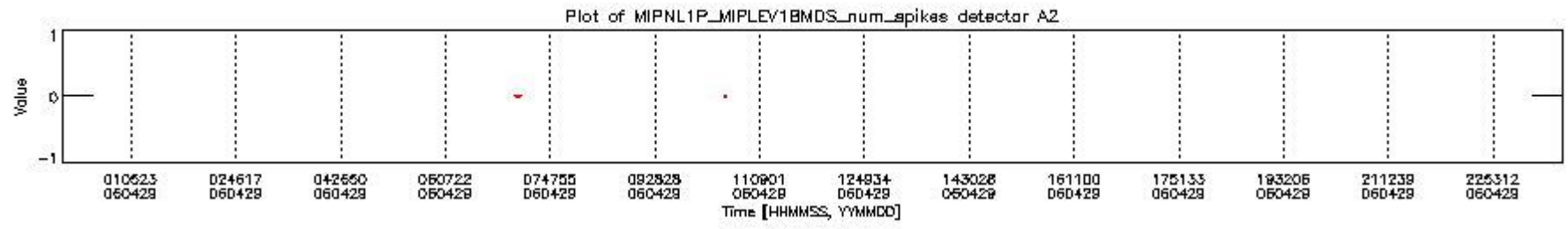
mipas_daily_report_level1_OFI_MIPAS_4_65_P_20060429_18.PNG
