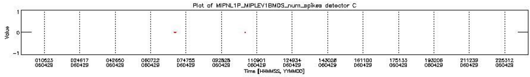
mipas_daily_report_level1_OFI_MIPAS_4_65_P_20060429_24.PNG
