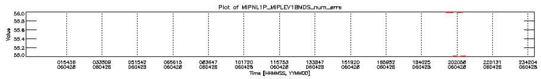
mipas_daily_report_level1_OFI_MIPAS_4_65_P_20060428_28.PNG
