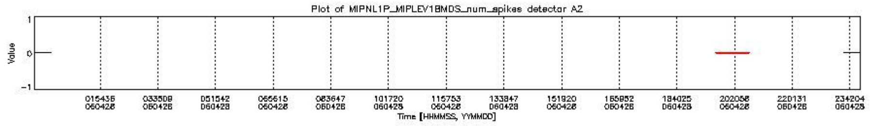
mipas_daily_report_level1_OFL_MIPAS_4_65_P_20060428_18.PNG
