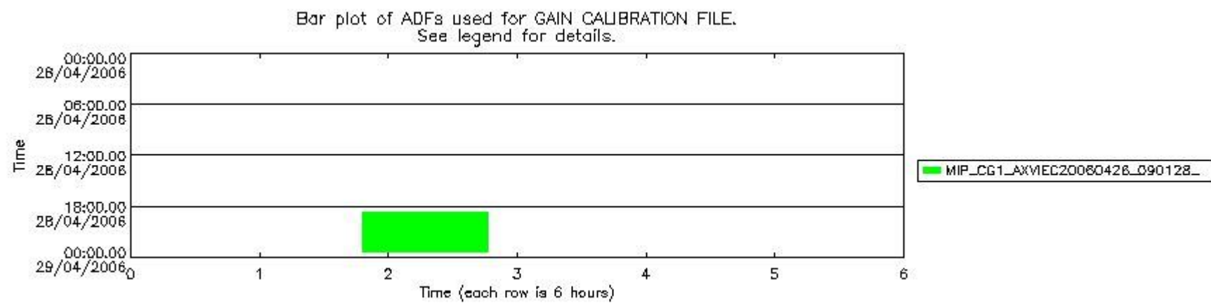
mipas_daily_report_level1_OFI_MIPAS_4_65_P_20060428_52.PNG
