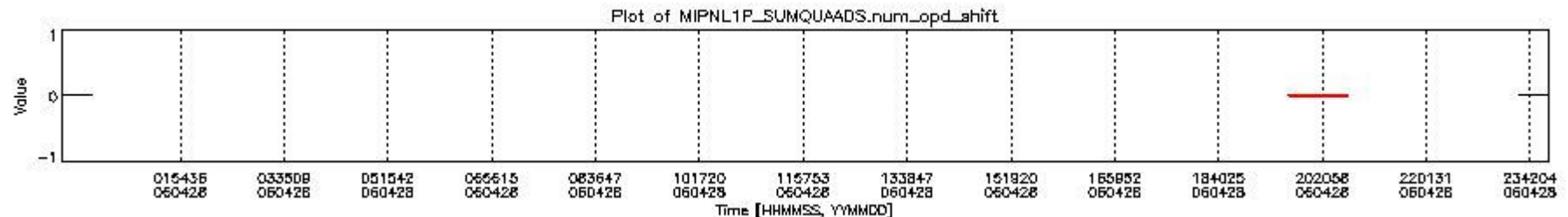
mipas_daily_report_level1_OFL_MIPAS_4_65_P_20060428_10.PNG
