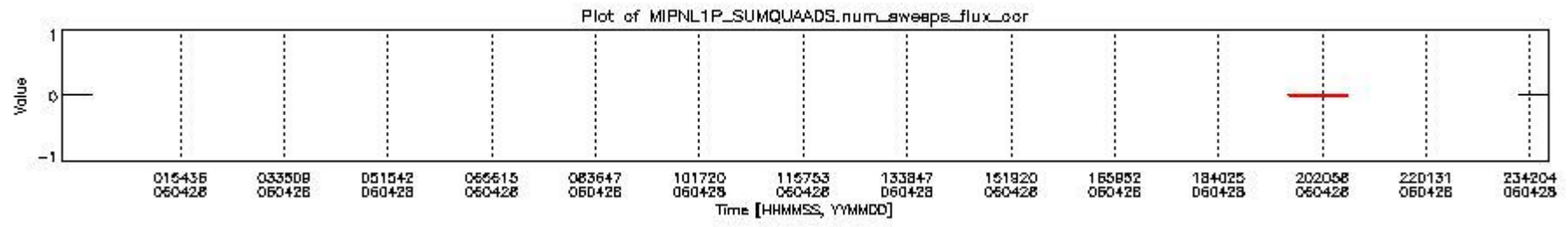
mipas_daily_report_level1_OFL_MIPAS_4_65_P_20060428_12.PNG
