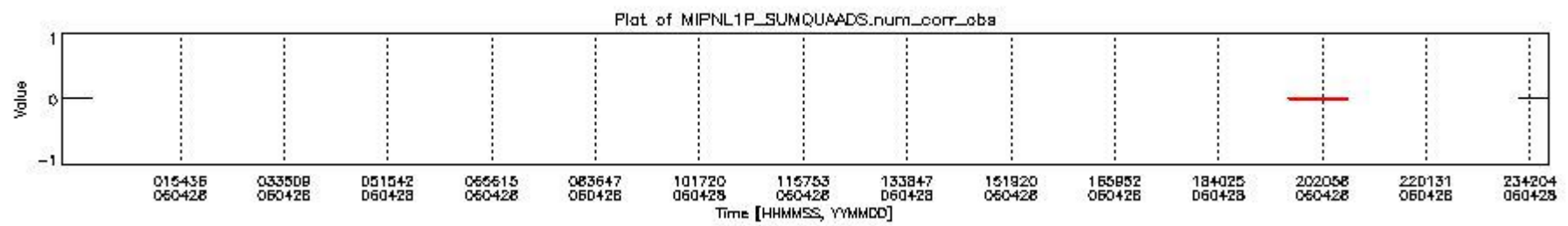
mipas_daily_report_level1_OFI_MIPAS_4_65_P_20060428_6.PNG
