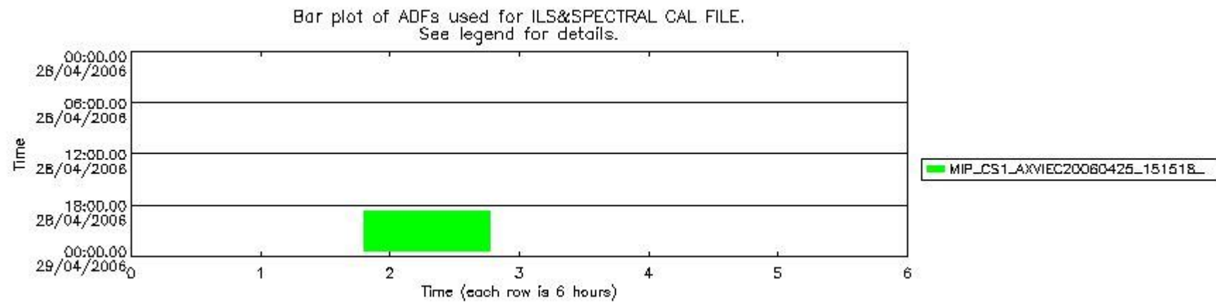
mipas_daily_report_level1_OFI_MIPAS_4_65_P_20060428_51.PNG
