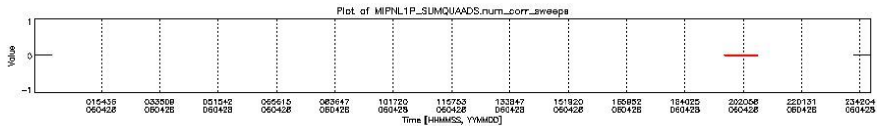
mipas_daily_report_level1_OFL_MIPAS_4_65_P_20060428_2.PNG
