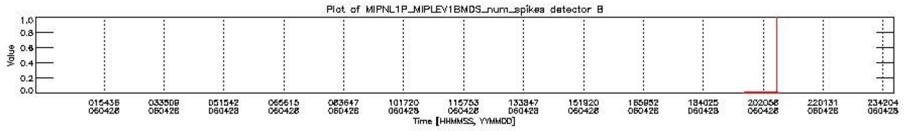
mipas_daily_report_level1_OFL_MIPAS_4_65_P_20060428_22.PNG
