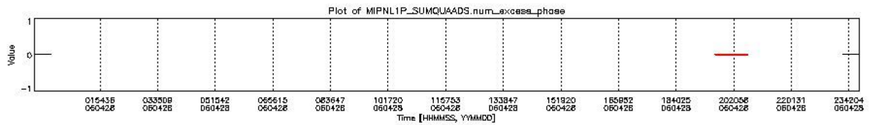
mipas_daily_report_level1_OFI_MIPAS_4_65_P_20060428_8.PNG
