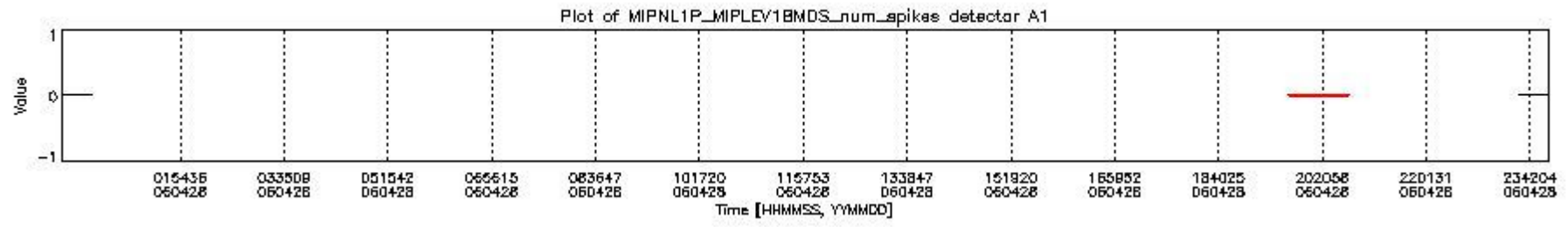
mipas_daily_report_level1_OFL_MIPAS_4_65_P_20060428_16.PNG
