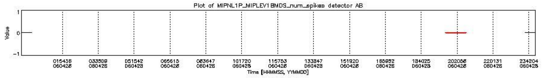
mipas_daily_report_level1_OFL_MIPAS_4_65_P_20060428_20.PNG
