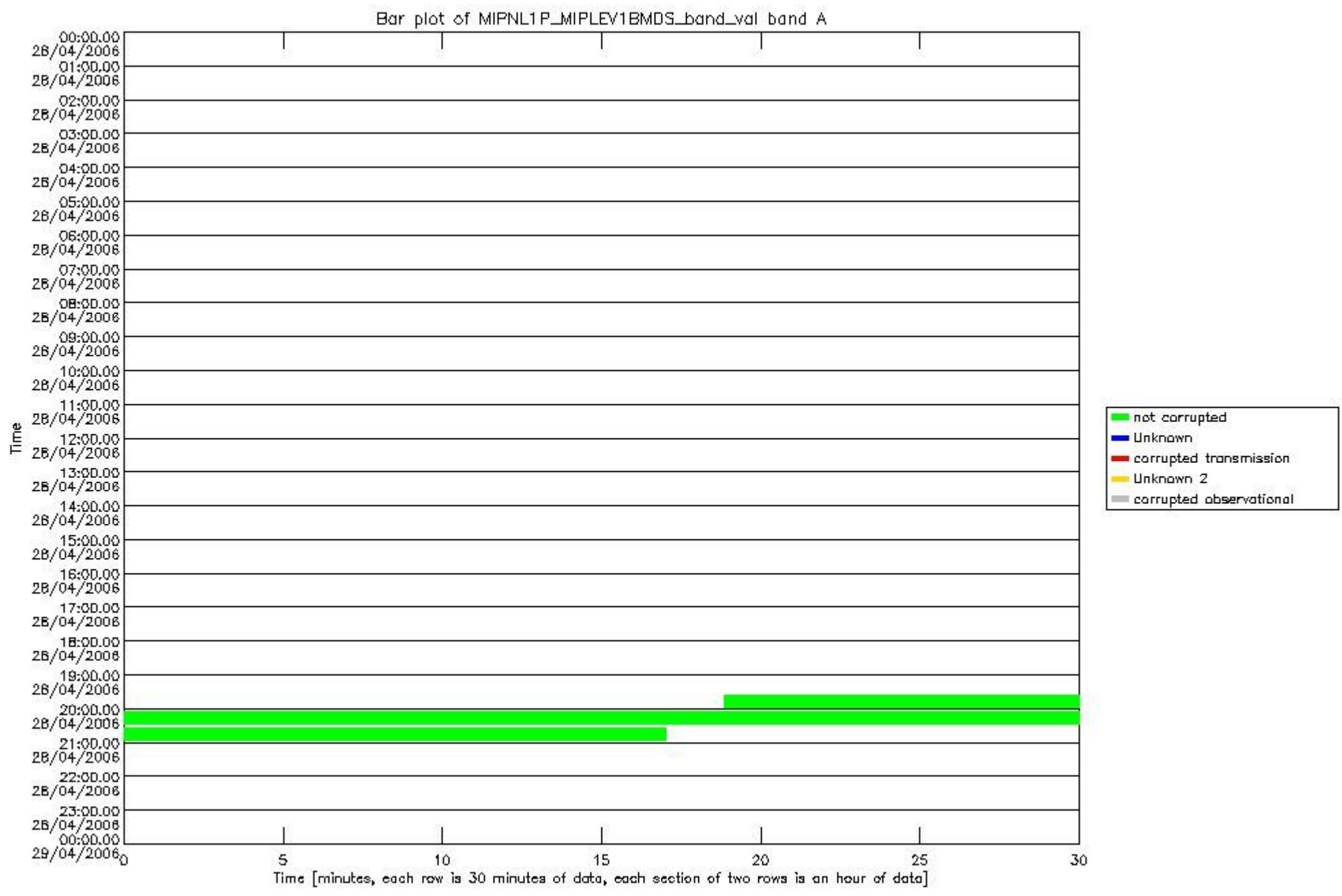
mipas_daily_report_level1_OFI_MIPAS_4_65_P_20060428_30.PNG
