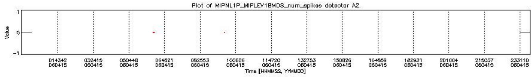
mipas_daily_report_level1_OFL_MIPAS_4_65_P_20060415_18.PNG
