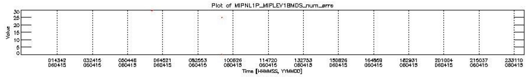
mipas_daily_report_level1_OFL_MIPAS_4_65_P_20060415_28.PNG
