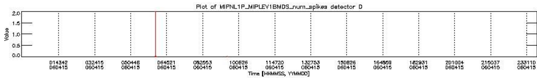
mipas_daily_report_level1_OFL_MIPAS_4_65_P_20060415_26.PNG
