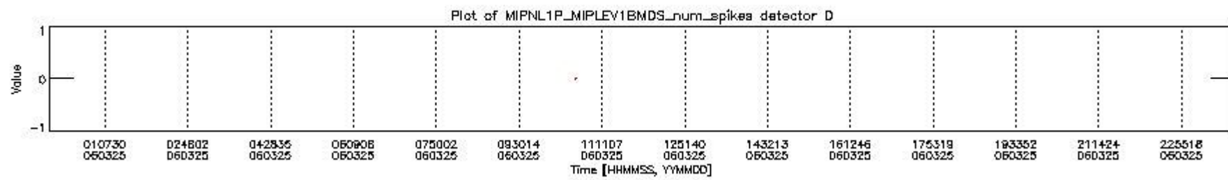
mipas_daily_report_level1_OFL_MIPAS_4_65_P_20060325_26.PNG
