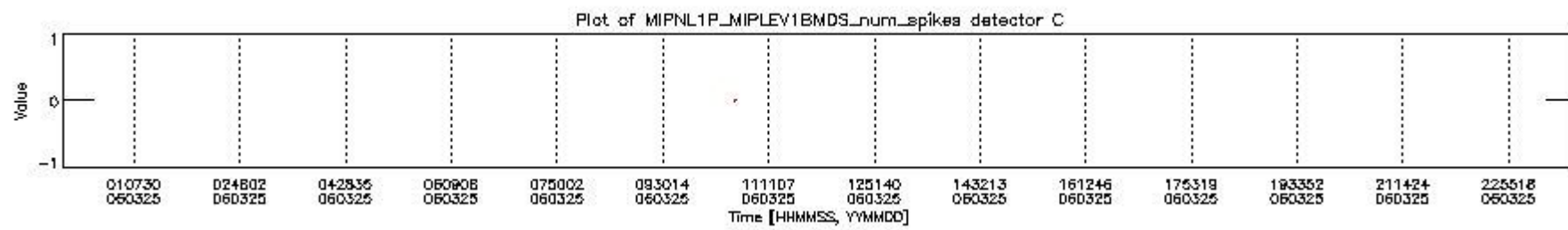
mipas_daily_report_level1_OFL_MIPAS_4_65_P_20060325_24.PNG
