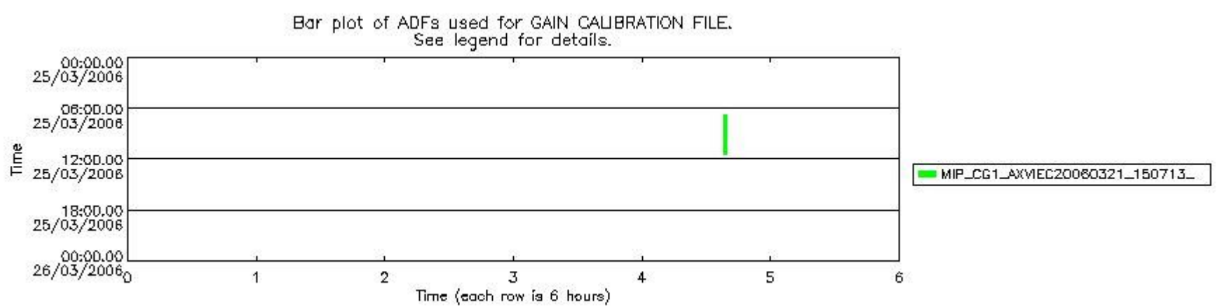
mipas_daily_report_level1_OFI_MIPAS_4_65_P_20060325_52.PNG
