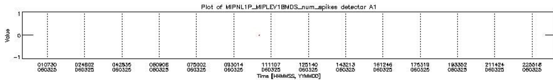
mipas_daily_report_level1_OFL_MIPAS_4_65_P_20060325_16.PNG
