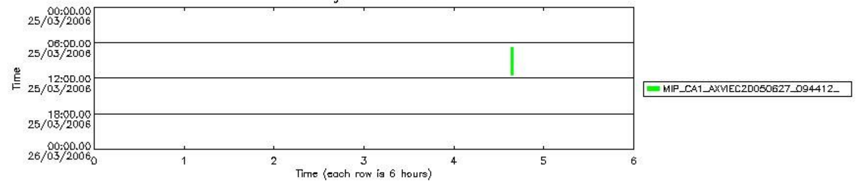
mipas_daily_report_level1_OFL_MIPAS_4_65_P_20060325_54.PNG
