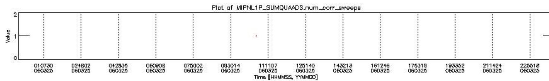
mipas_daily_report_level1_OFI_MIPAS_4_65_P_20060325_2.PNG
