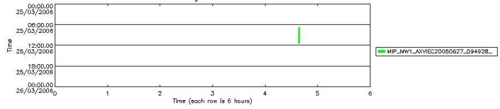
mipas_daily_report_level1_OFL_MIPAS_4_65_P_20060325_56.PNG
