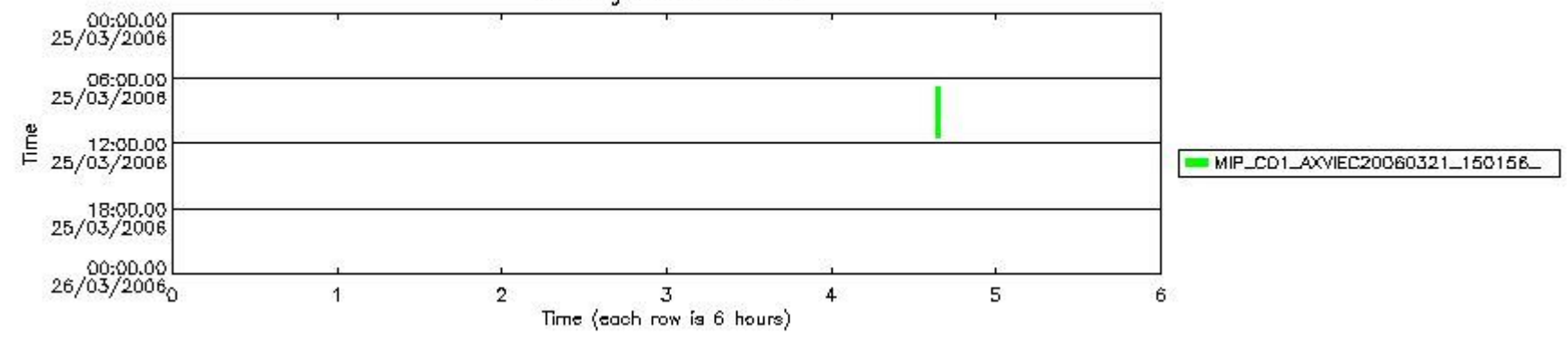
mipas_daily_report_level1_OFL_MIPAS_4_65_P_20060325_55.PNG
