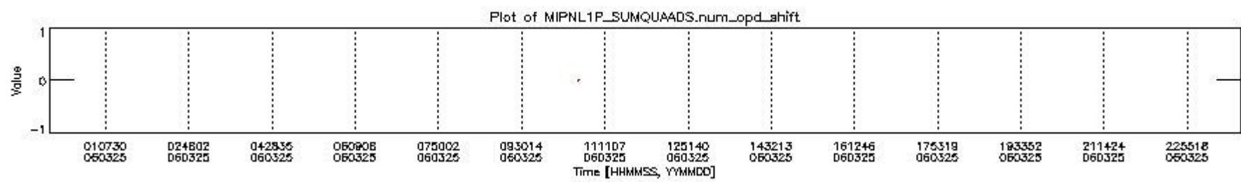
mipas_daily_report_level1_OFL_MIPAS_4_65_P_20060325_10.PNG
