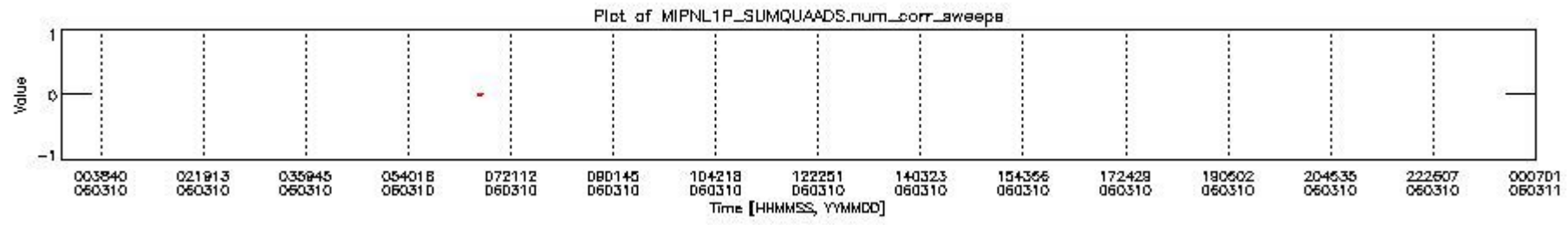
mipas_daily_report_level1_OFL_MIPAS_4_65_P_20060310_2.PNG
