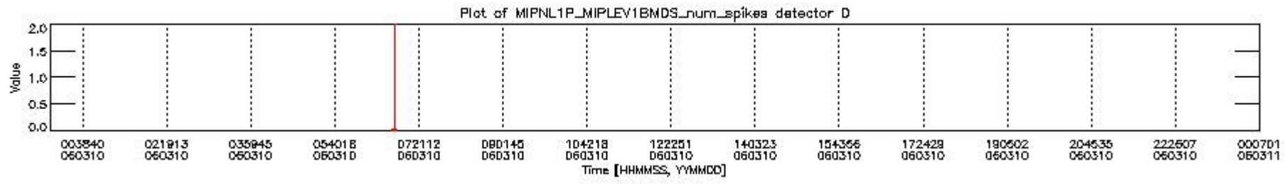
mipas_daily_report_level1_OFI_MIPAS_4_65_P_20060310_26.PNG
