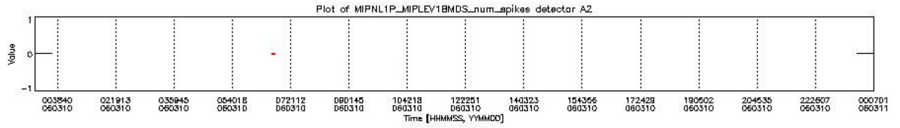
mipas_daily_report_level1_OFL_MIPAS_4_65_P_20060310_18.PNG
