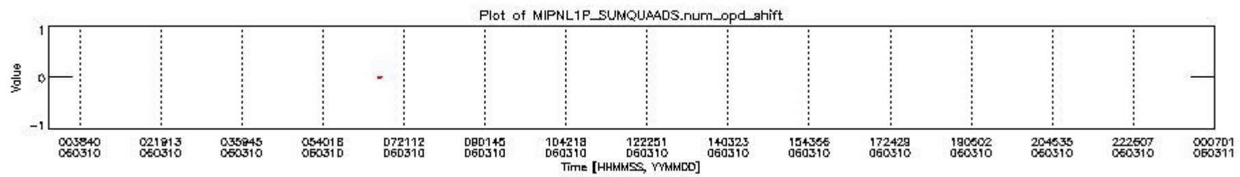
mipas_daily_report_level1_OFL_MIPAS_4_65_P_20060310_10.PNG
