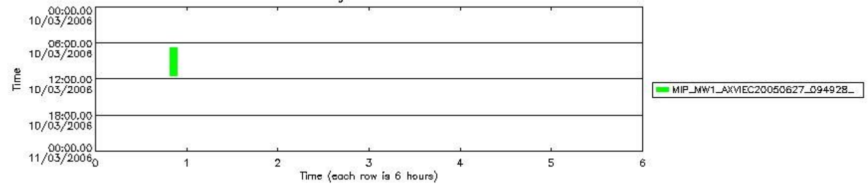
mipas_daily_report_level1_OFL_MIPAS_4_65_P_20060310_56.PNG
