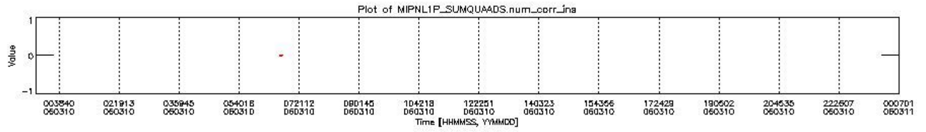
mipas_daily_report_level1_OFI_MIPAS_4_65_P_20060310_4.PNG
