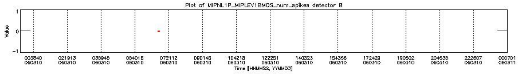
mipas_daily_report_level1_OFL_MIPAS_4_65_P_20060310_22.PNG
