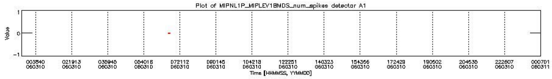
mipas_daily_report_level1_OFL_MIPAS_4_65_P_20060310_16.PNG
