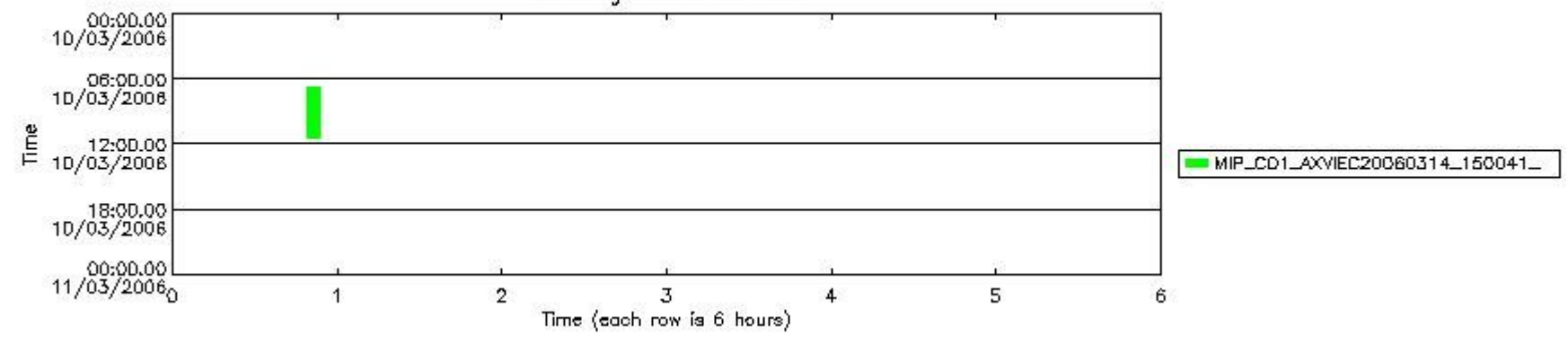
mipas_daily_report_level1_OFL_MIPAS_4_65_P_20060310_55.PNG
