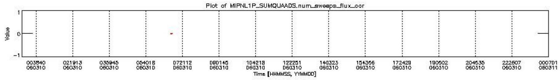
mipas_daily_report_level1_OFI_MIPAS_4_65_P_20060310_12.PNG
