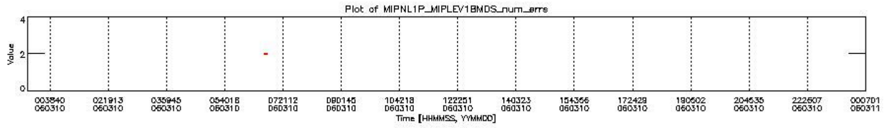
mipas_daily_report_level1_OFI_MIPAS_4_65_P_20060310_28.PNG
