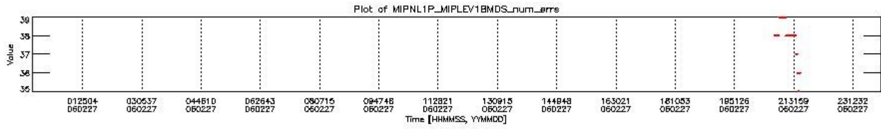
mipas_daily_report_level1_OFL_MIPAS_4_65_P_20060227_28.PNG
