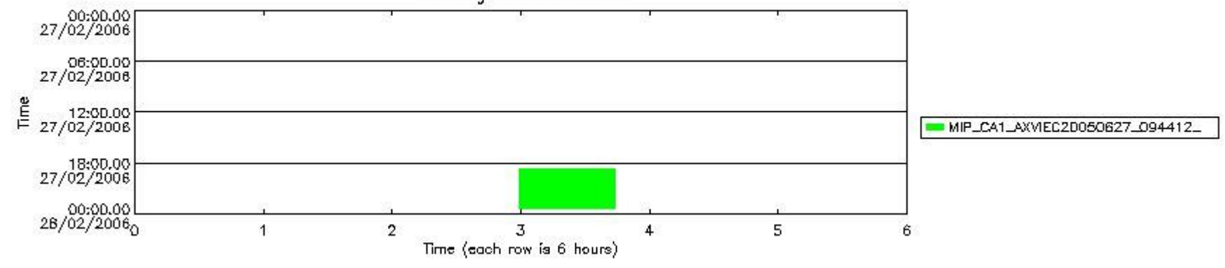
mipas_daily_report_level1_OFL_MIPAS_4_65_P_20060227_54.PNG
