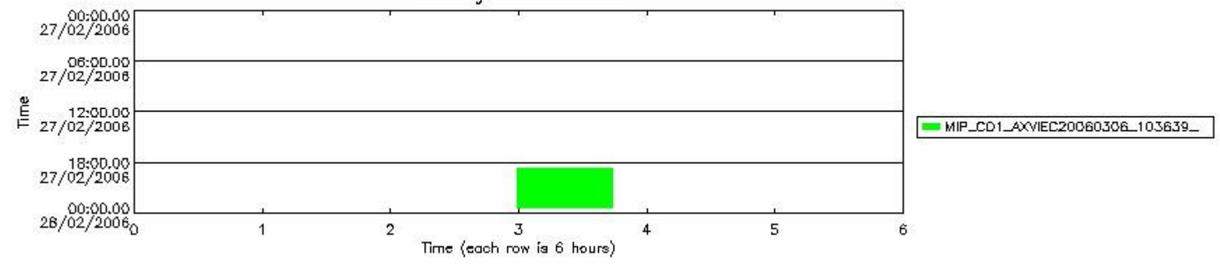
mipas_daily_report_level1_OFL_MIPAS_4_65_P_20060227_55.PNG
