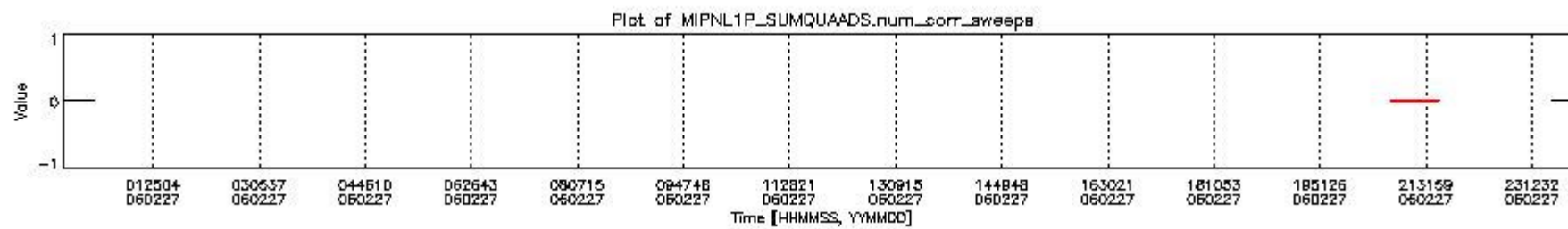
mipas_daily_report_level1_OFL_MIPAS_4_65_P_20060227_2.PNG
