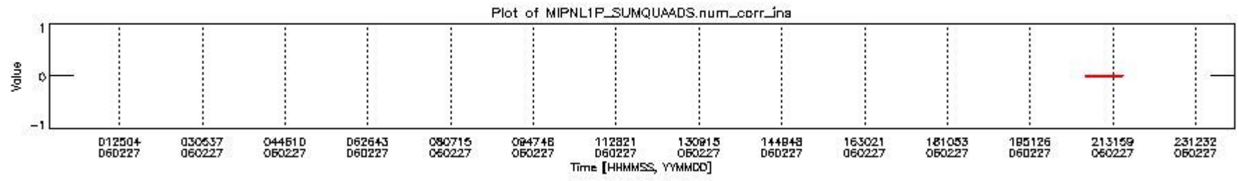
mipas_daily_report_level1_OFL_MIPAS_4_65_P_20060227_4.PNG
