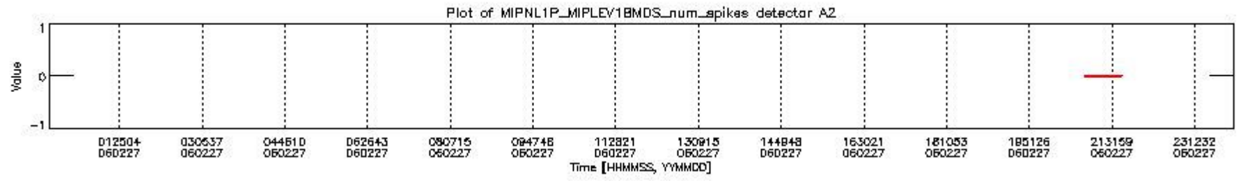
mipas_daily_report_level1_OFL_MIPAS_4_65_P_20060227_18.PNG
