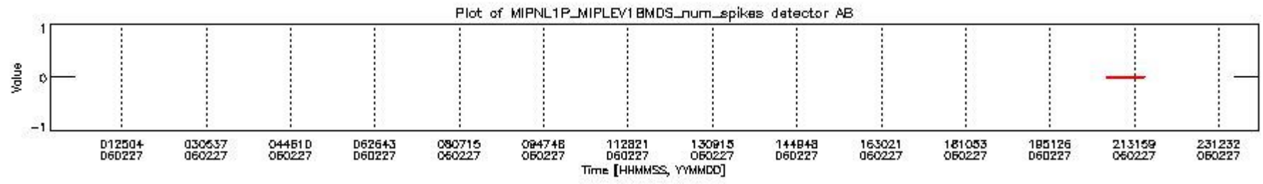
mipas_daily_report_level1_OFL_MIPAS_4_65_P_20060227_20.PNG
