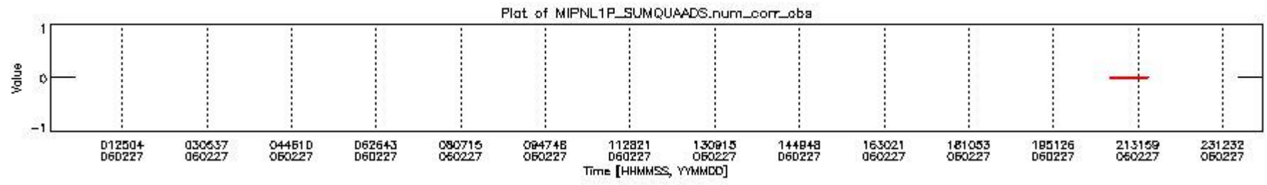
mipas_daily_report_level1_OFI_MIPAS_4_65_P_20060227_6.PNG
