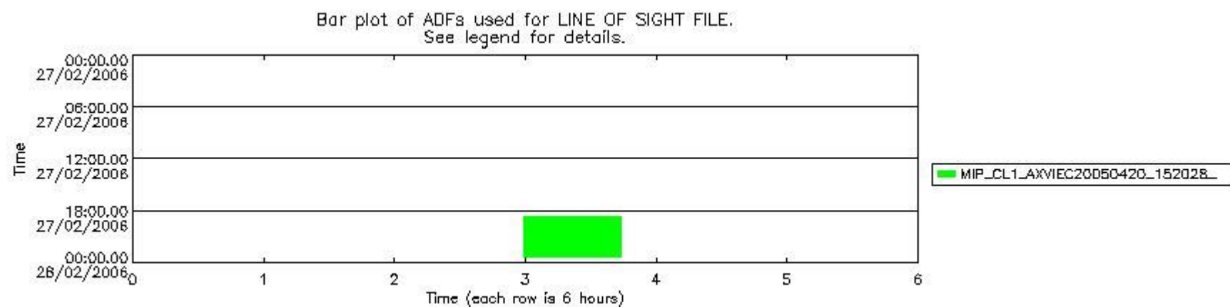
mipas_daily_report_level1_OFL_MIPAS_4_65_P_20060227_53.PNG
