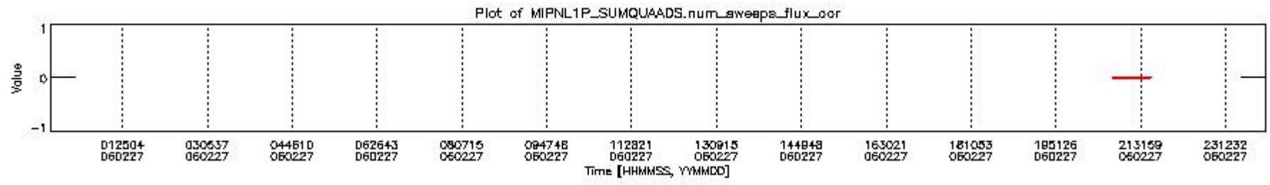
mipas_daily_report_level1_OFL_MIPAS_4_65_P_20060227_12.PNG
