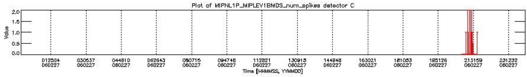
mipas_daily_report_level1_OFL_MIPAS_4_65_P_20060227_24.PNG
