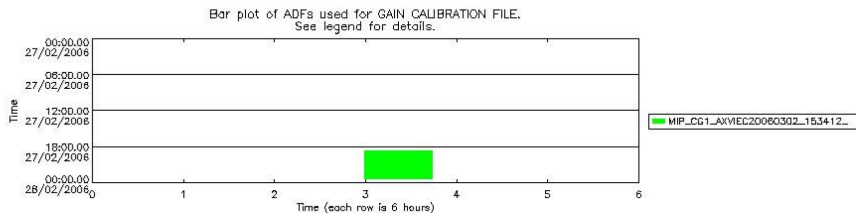
mipas_daily_report_level1_OFL_MIPAS_4_65_P_20060227_52.PNG
