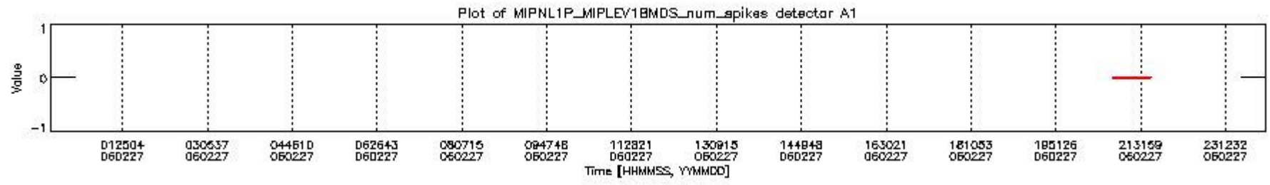
mipas_daily_report_level1_OFL_MIPAS_4_65_P_20060227_16.PNG
