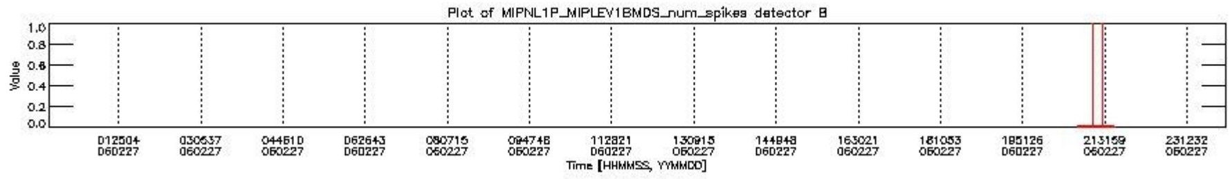
mipas_daily_report_level1_OFL_MIPAS_4_65_P_20060227_22.PNG
