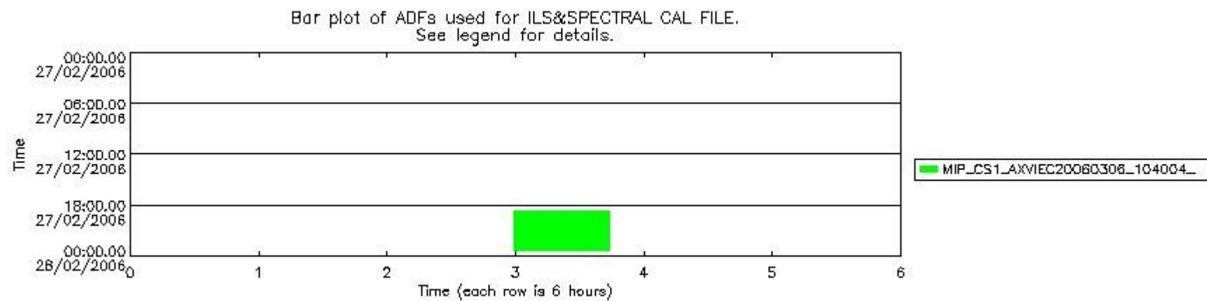
mipas_daily_report_level1_OFL_MIPAS_4_65_P_20060227_51.PNG
