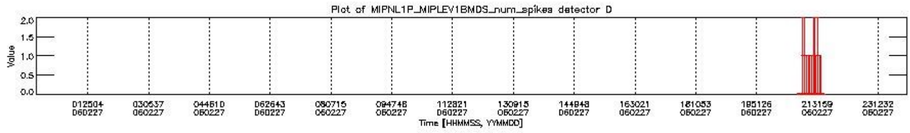
mipas_daily_report_level1_OFL_MIPAS_4_65_P_20060227_26.PNG
