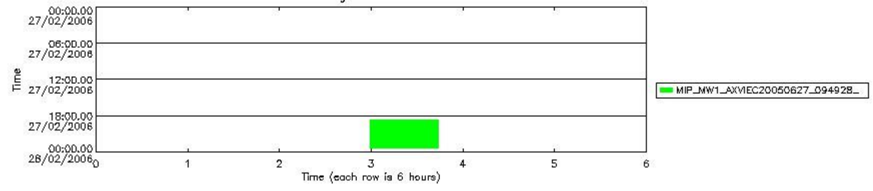
mipas_daily_report_level1_OFL_MIPAS_4_65_P_20060227_56.PNG
