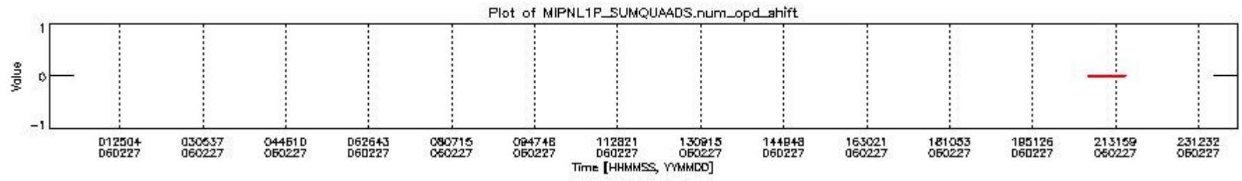
mipas_daily_report_level1_OFL_MIPAS_4_65_P_20060227_10.PNG
