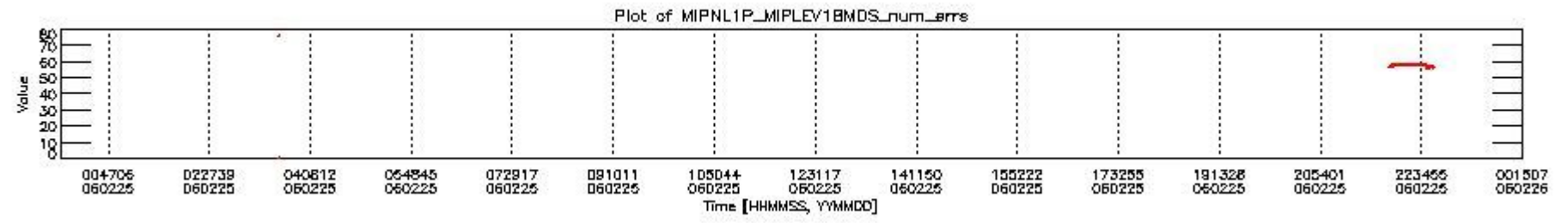
mipas_daily_report_level1_OFL_MIPAS_4_65_P_20060225_28.PNG
