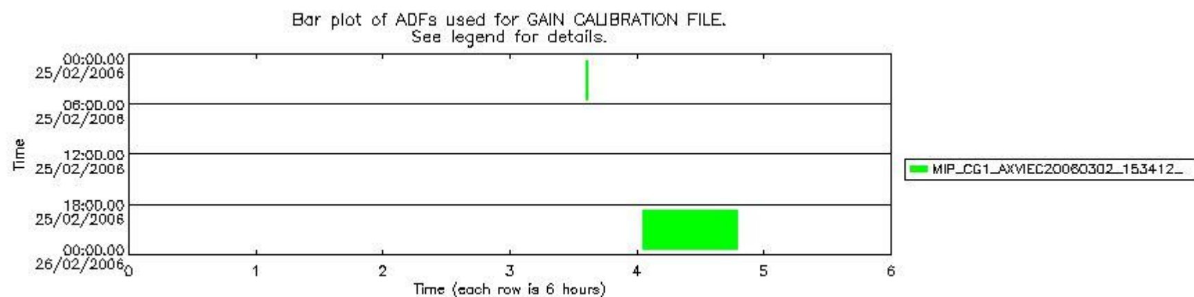
mipas_daily_report_level1_OFL_MIPAS_4_65_P_20060225_52.PNG
