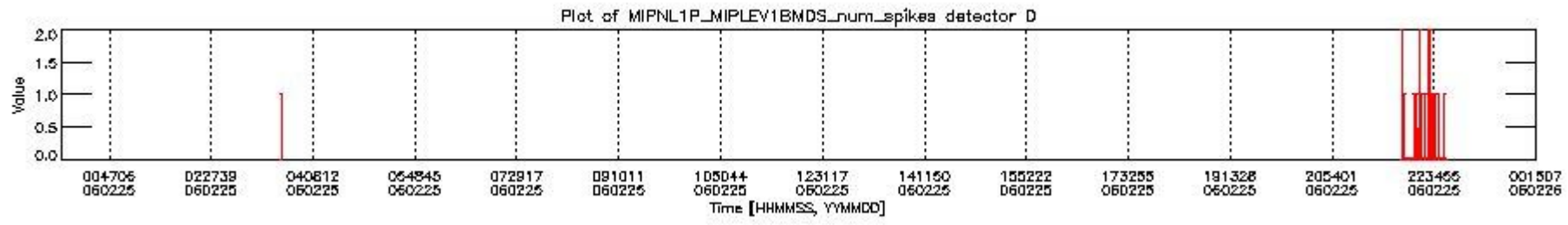
mipas_daily_report_level1_OFL_MIPAS_4_65_P_20060225_26.PNG
