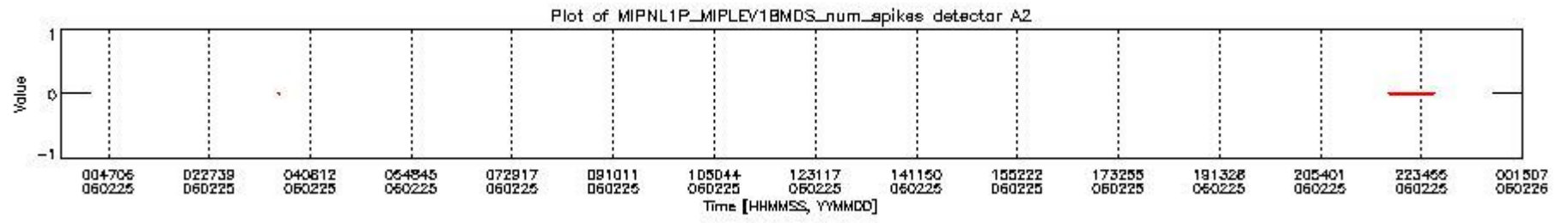
mipas_daily_report_level1_OFL_MIPAS_4_65_P_20060225_18.PNG
