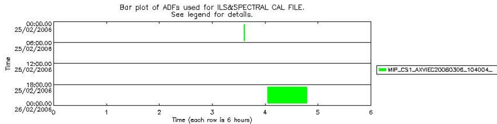
mipas_daily_report_level1_OFL_MIPAS_4_65_P_20060225_51.PNG
