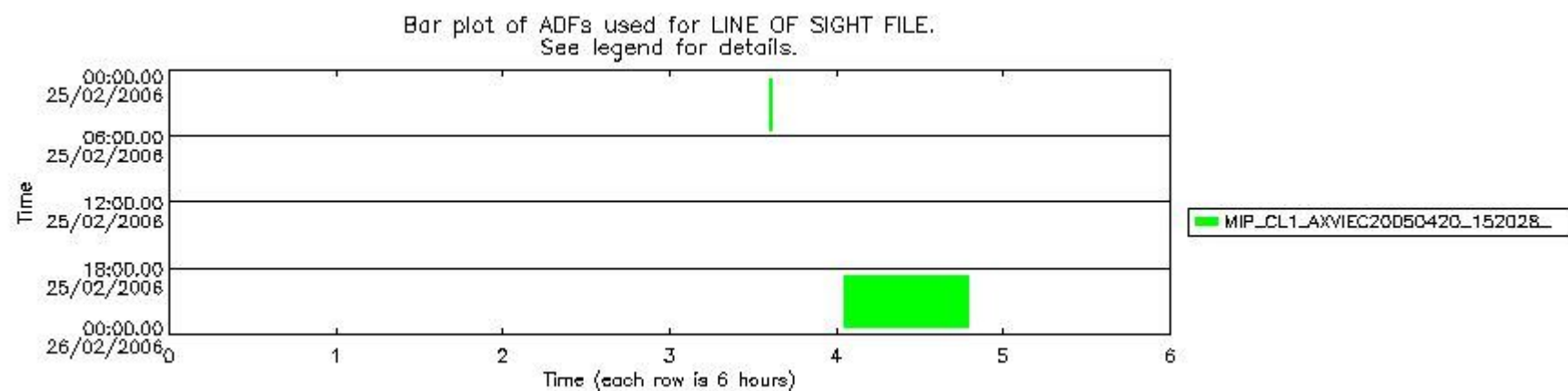
mipas_daily_report_level1_OFL_MIPAS_4_65_P_20060225_53.PNG
