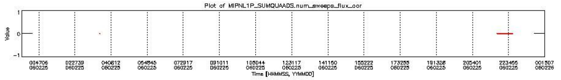
mipas_daily_report_level1_OFL_MIPAS_4_65_P_20060225_12.PNG
