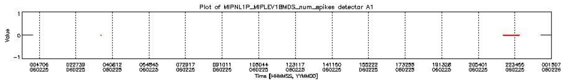
mipas_daily_report_level1_OFL_MIPAS_4_65_P_20060225_16.PNG
