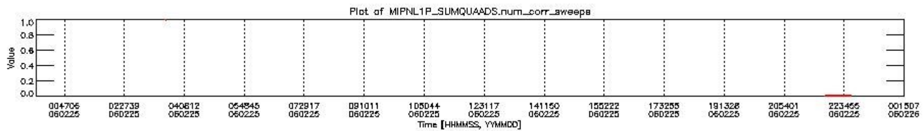
mipas_daily_report_level1_OFI_MIPAS_4_65_P_20060225_2.PNG
