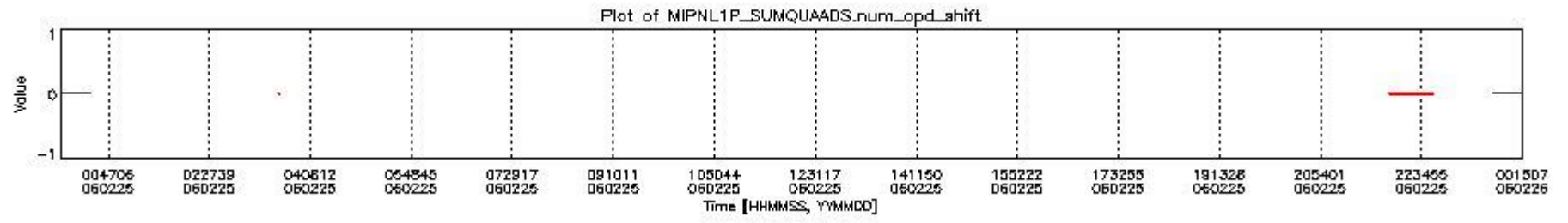
mipas_daily_report_level1_OFL_MIPAS_4_65_P_20060225_10.PNG
