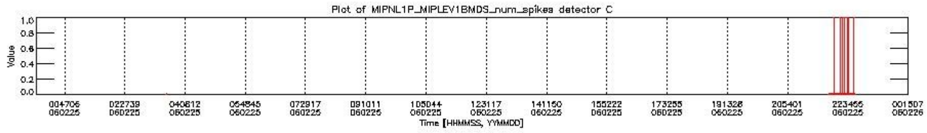
mipas_daily_report_level1_OFL_MIPAS_4_65_P_20060225_24.PNG
