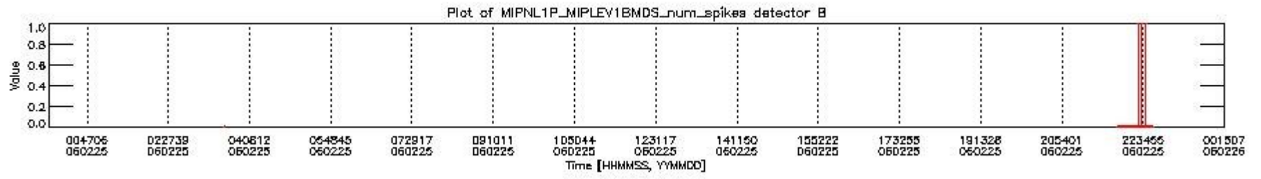
mipas_daily_report_level1_OFL_MIPAS_4_65_P_20060225_22.PNG
