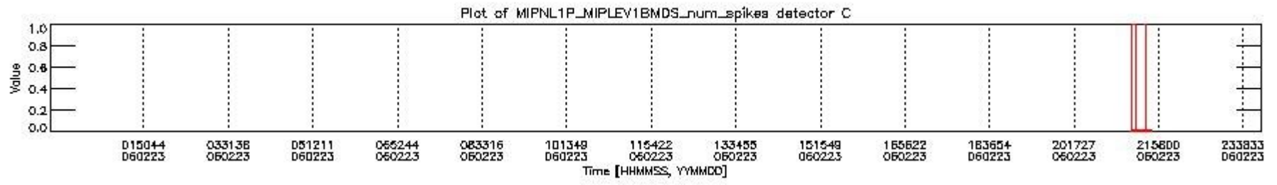
mipas_daily_report_level1_OFL_MIPAS_4_65_P_20060223_24.PNG
