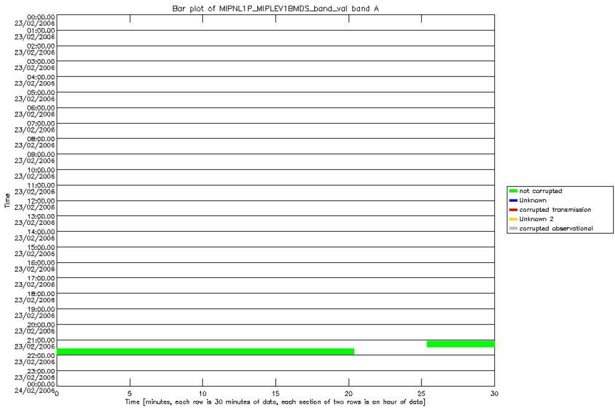
mipas_daily_report_level1_OFI_MIPAS_4_65_P_20060223_30.PNG
