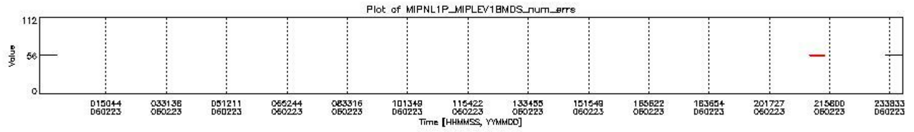
mipas_daily_report_level1_OFL_MIPAS_4_65_P_20060223_28.PNG
