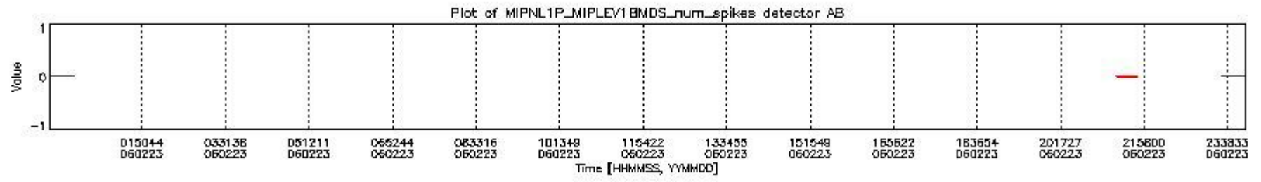
mipas_daily_report_level1_OFL_MIPAS_4_65_P_20060223_20.PNG
