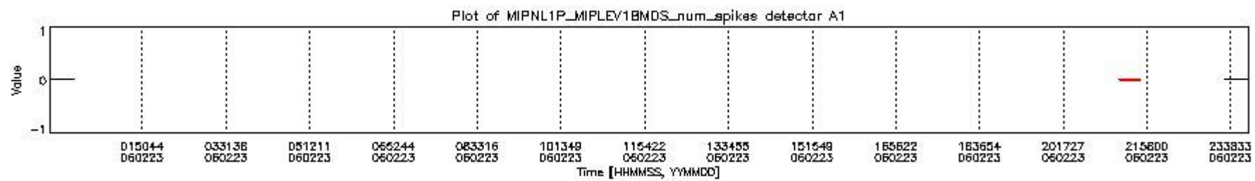
mipas_daily_report_level1_OFL_MIPAS_4_65_P_20060223_16.PNG
