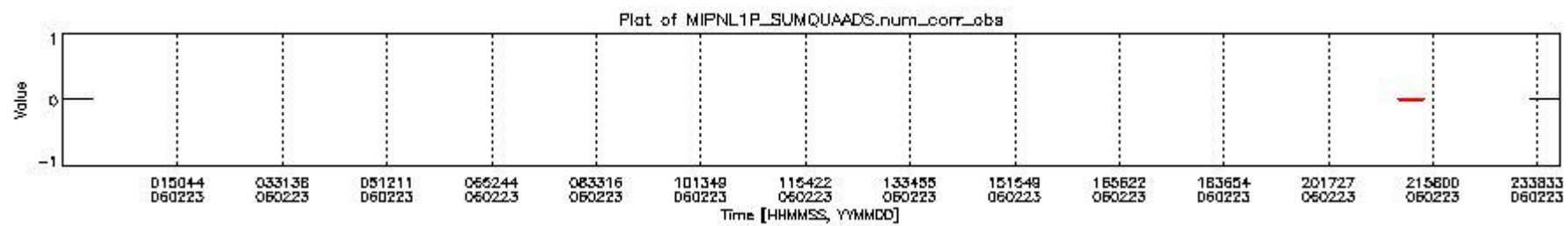
mipas_daily_report_level1_OFI_MIPAS_4_65_P_20060223_6.PNG
