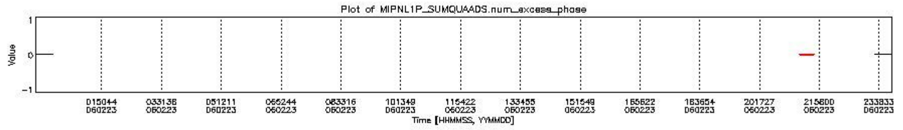
mipas_daily_report_level1_OFI_MIPAS_4_65_P_20060223_8.PNG
