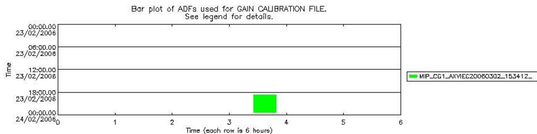
mipas_daily_report_level1_OFI_MIPAS_4_65_P_20060223_52.PNG
