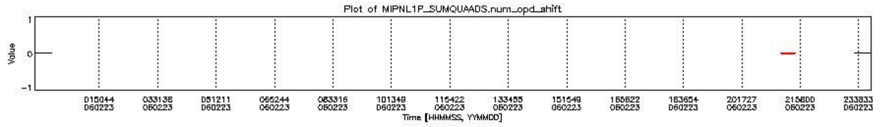
mipas_daily_report_level1_OFL_MIPAS_4_65_P_20060223_10.PNG
