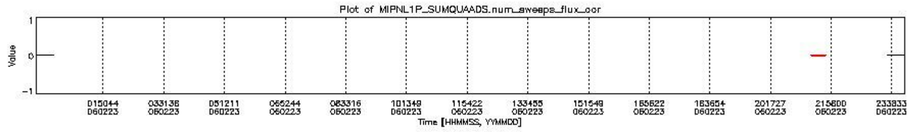
mipas_daily_report_level1_OFL_MIPAS_4_65_P_20060223_12.PNG
