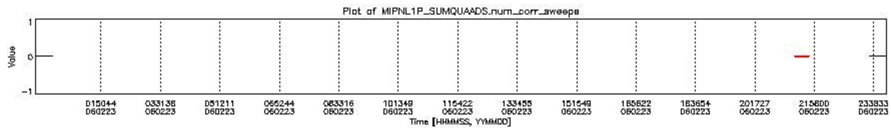
mipas_daily_report_level1_OFI_MIPAS_4_65_P_20060223_2.PNG
