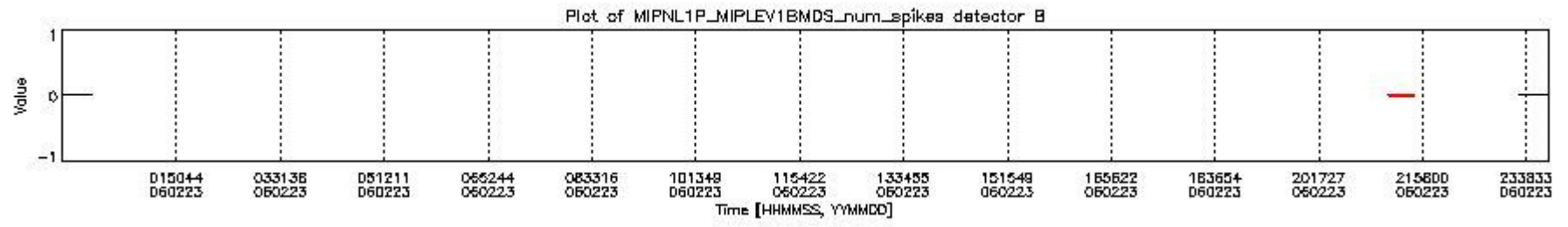
mipas_daily_report_level1_OFL_MIPAS_4_65_P_20060223_22.PNG
