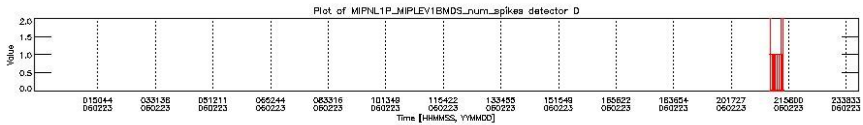
mipas_daily_report_level1_OFL_MIPAS_4_65_P_20060223_26.PNG
