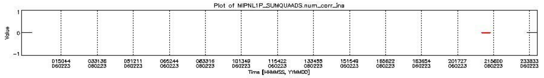
mipas_daily_report_level1_OFI_MIPAS_4_65_P_20060223_4.PNG
