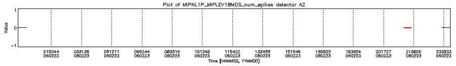
mipas_daily_report_level1_OFL_MIPAS_4_65_P_20060223_18.PNG
