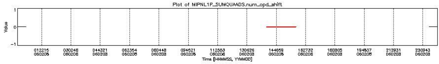
mipas_daily_report_level1_OFL_MIPAS_4_65_P_20060208_10.PNG
