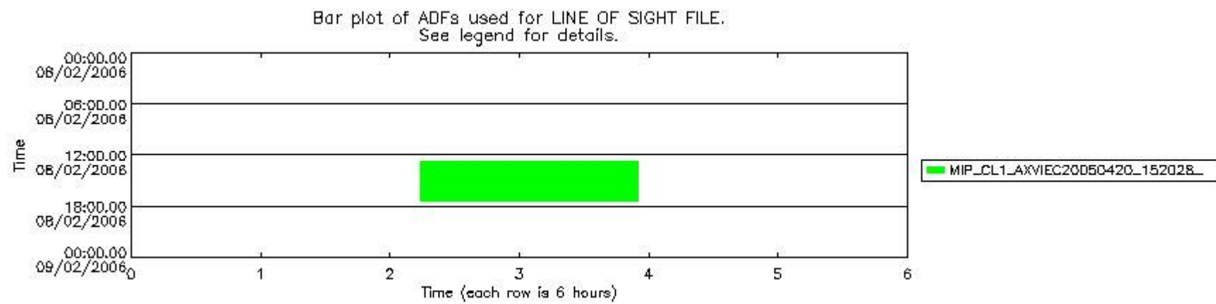
mipas_daily_report_level1_OFI_MIPAS_4_65_P_20060208_54.PNG
