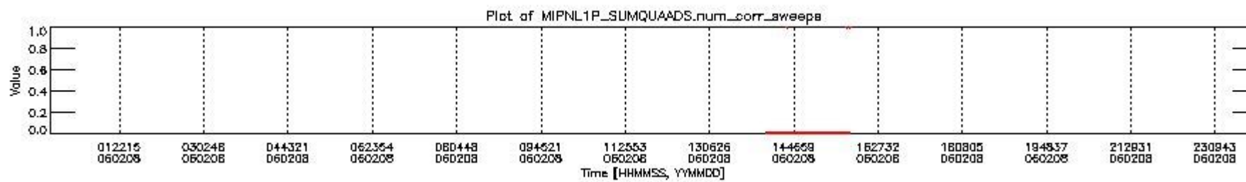
mipas_daily_report_level1_OFL_MIPAS_4_65_P_20060208_2.PNG
