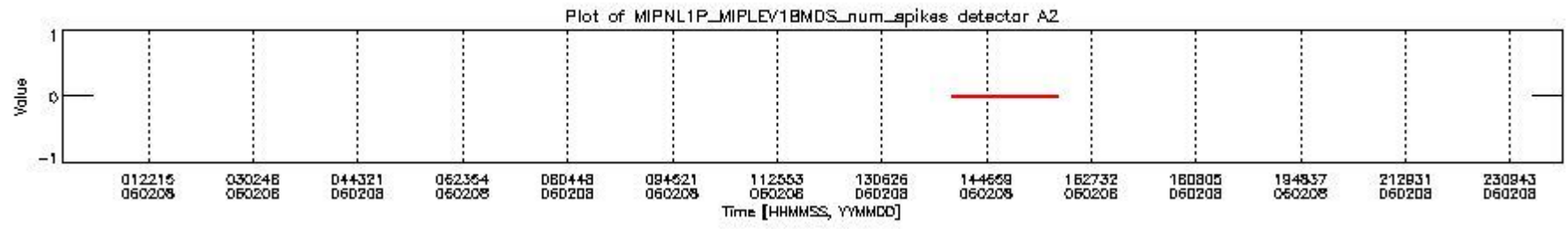
mipas_daily_report_level1_OFL_MIPAS_4_65_P_20060208_18.PNG
