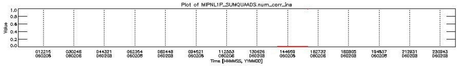
mipas_daily_report_level1_OFI_MIPAS_4_65_P_20060208_4.PNG
