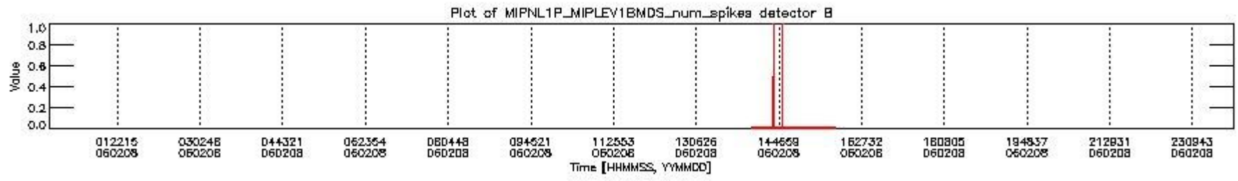
mipas_daily_report_level1_OFL_MIPAS_4_65_P_20060208_22.PNG
