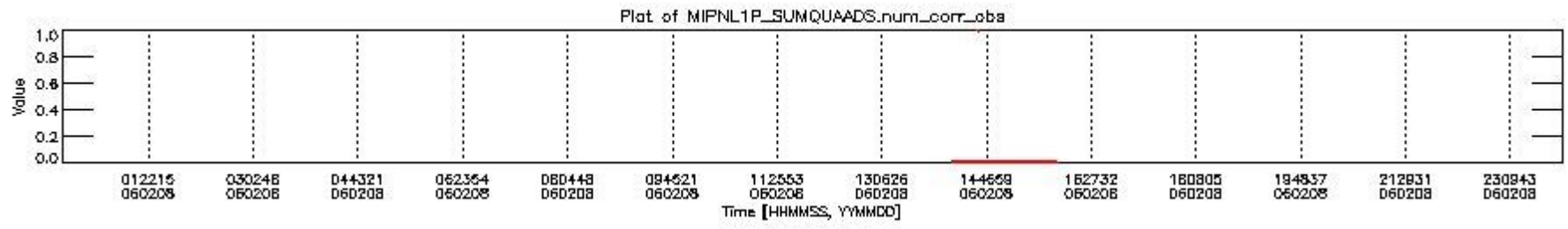
mipas_daily_report_level1_OFI_MIPAS_4_65_P_20060208_6.PNG
