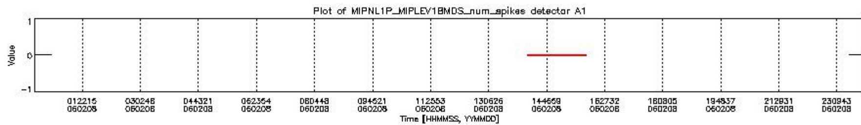
mipas_daily_report_level1_OFL_MIPAS_4_65_P_20060208_16.PNG
