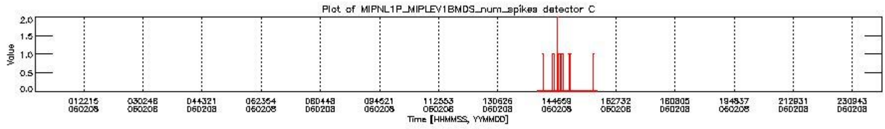
mipas_daily_report_level1_OFL_MIPAS_4_65_P_20060208_24.PNG
