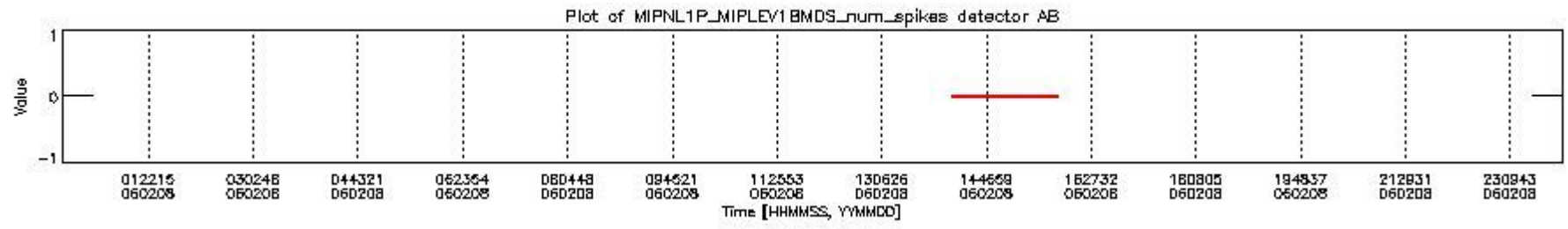
mipas_daily_report_level1_OFL_MIPAS_4_65_P_20060208_20.PNG
