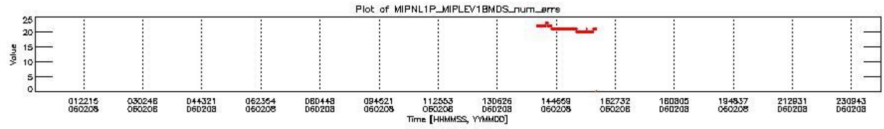
mipas_daily_report_level1_OFL_MIPAS_4_65_P_20060208_28.PNG
