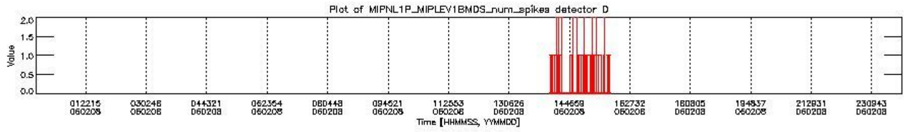
mipas_daily_report_level1_OFL_MIPAS_4_65_P_20060208_26.PNG
