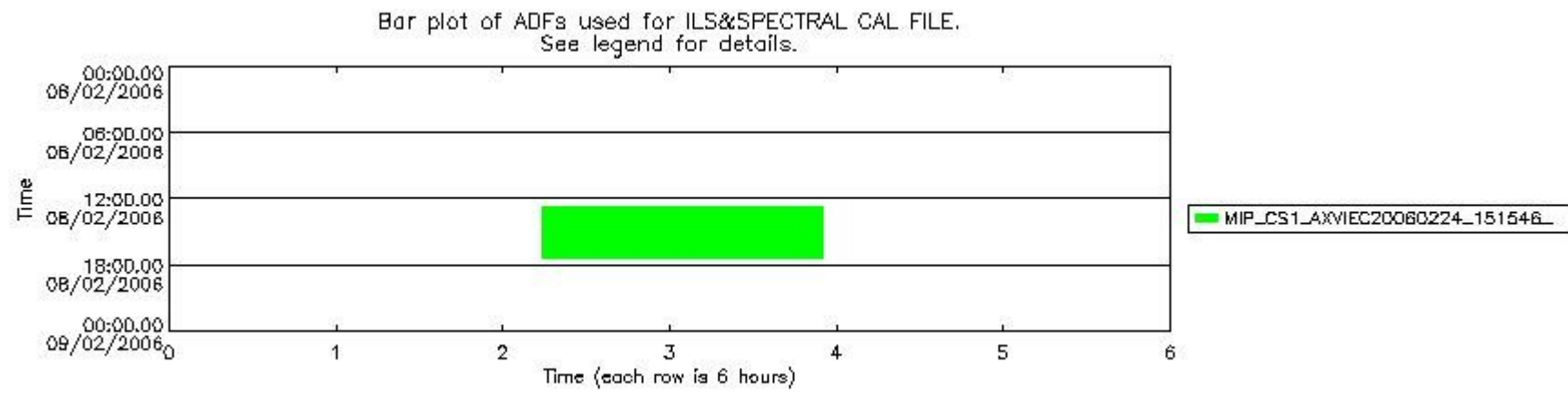
mipas_daily_report_level1_OFI_MIPAS_4_65_P_20060208_52.PNG
