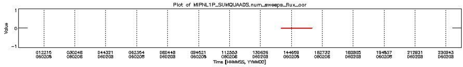
mipas_daily_report_level1_OFL_MIPAS_4_65_P_20060208_12.PNG
