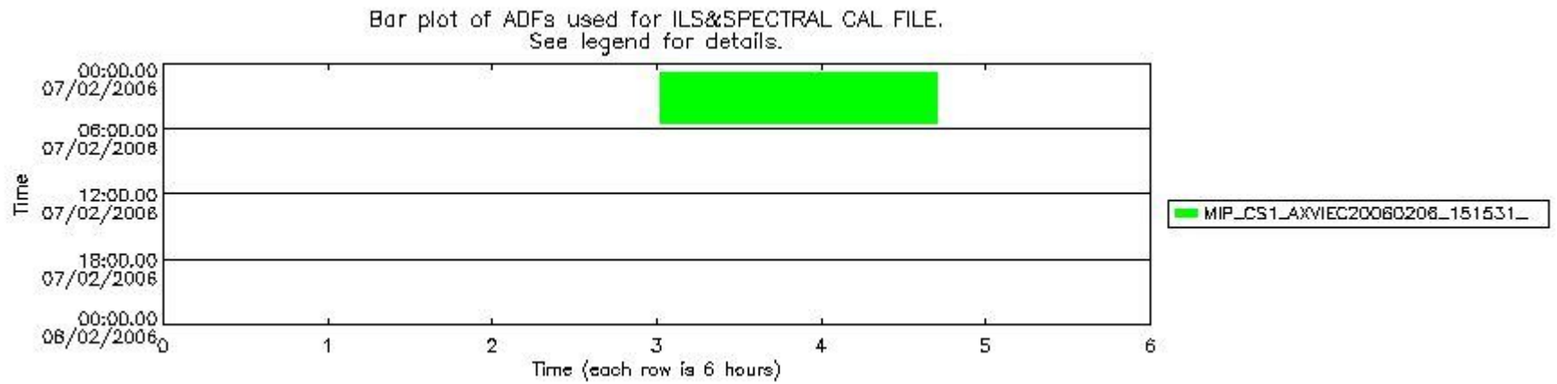
mipas_daily_report_level1_OFL_MIPAS_4_65_P_20060207_52.PNG
