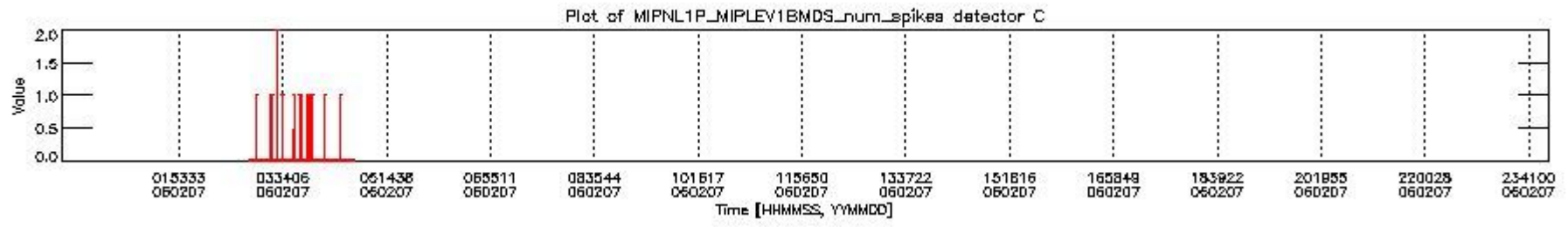
mipas_daily_report_level1_OFL_MIPAS_4_65_P_20060207_24.PNG
