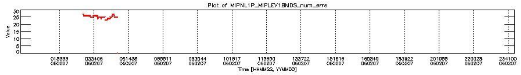
mipas_daily_report_level1_OFL_MIPAS_4_65_P_20060207_28.PNG
