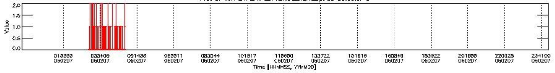
mipas_daily_report_level1_OFL_MIPAS_4_65_P_20060207_26.PNG
