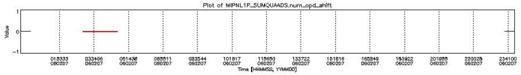
mipas_daily_report_level1_OFL_MIPAS_4_65_P_20060207_10.PNG
