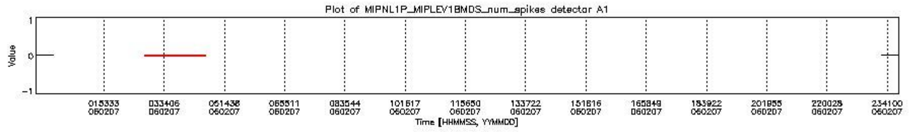
mipas_daily_report_level1_OFL_MIPAS_4_65_P_20060207_16.PNG
