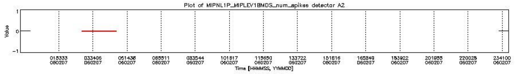
mipas_daily_report_level1_OFL_MIPAS_4_65_P_20060207_18.PNG
