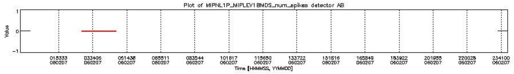
mipas_daily_report_level1_OFL_MIPAS_4_65_P_20060207_20.PNG
