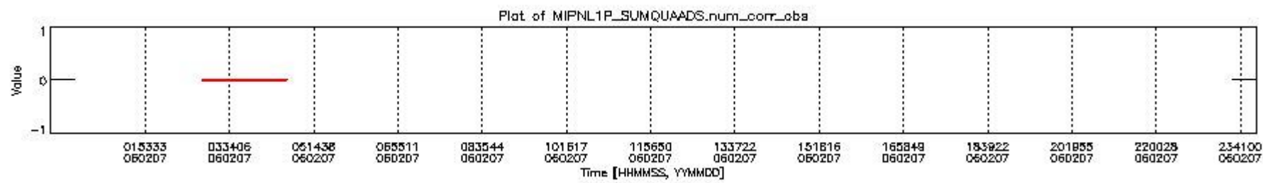
mipas_daily_report_level1_OFI_MIPAS_4_65_P_20060207_6.PNG
