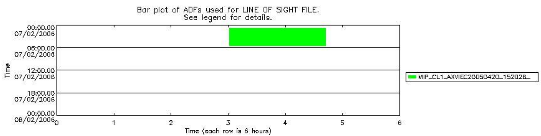
mipas_daily_report_level1_OFL_MIPAS_4_65_P_20060207_54.PNG
