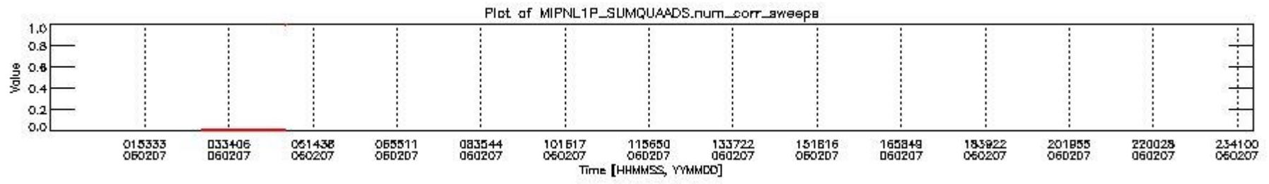
mipas_daily_report_level1_OFI_MIPAS_4_65_P_20060207_2.PNG
