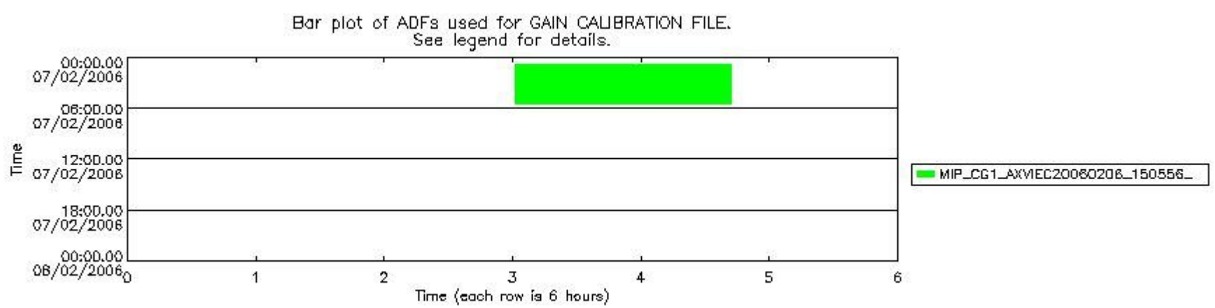
mipas_daily_report_level1_OFL_MIPAS_4_65_P_20060207_53.PNG
