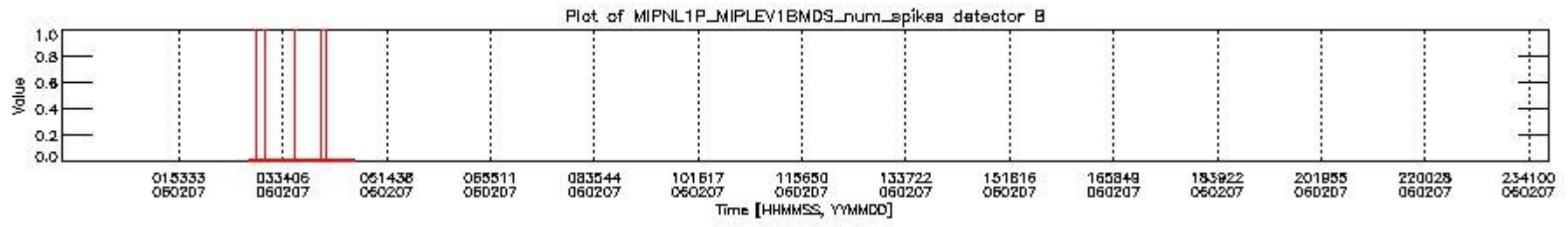
mipas_daily_report_level1_OFL_MIPAS_4_65_P_20060207_22.PNG
