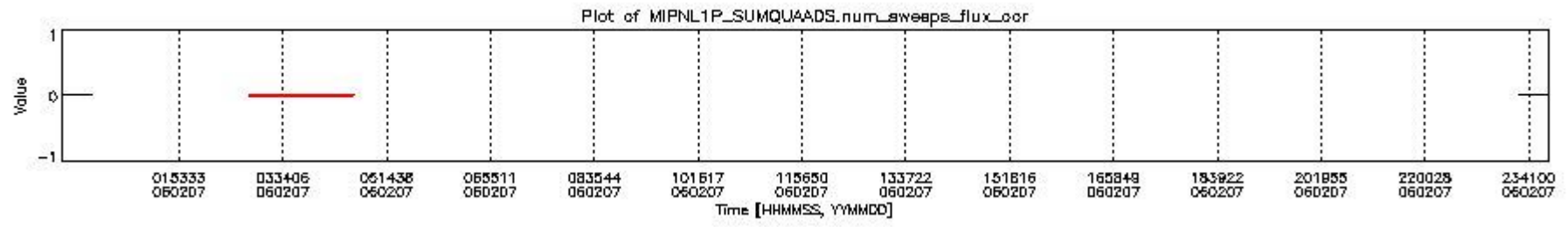
mipas_daily_report_level1_OFL_MIPAS_4_65_P_20060207_12.PNG
