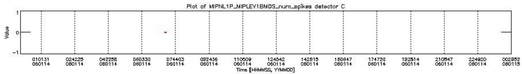
mipas_daily_report_level1_OFL_MIPAS_4_65_P_20060114_24.PNG
