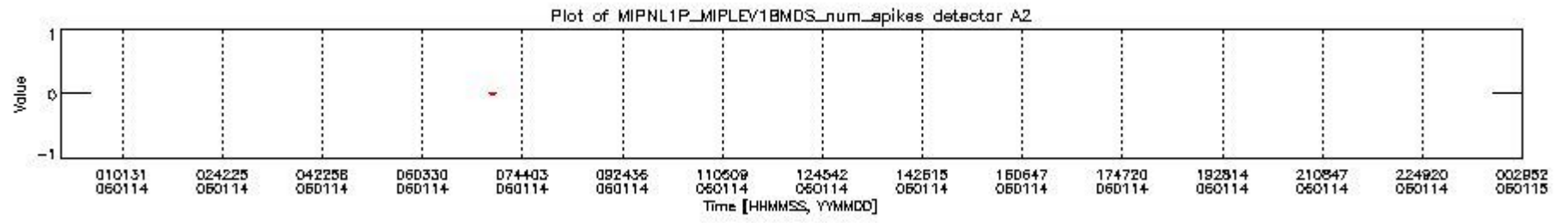
mipas_daily_report_level1_OFI_MIPAS_4_65_P_20060114_18.PNG
