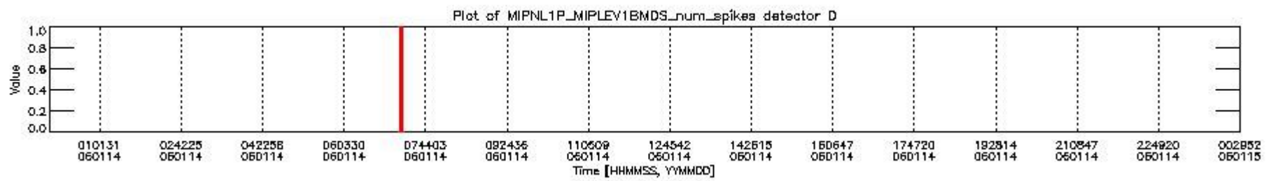
mipas_daily_report_level1_OFL_MIPAS_4_65_P_20060114_26.PNG
