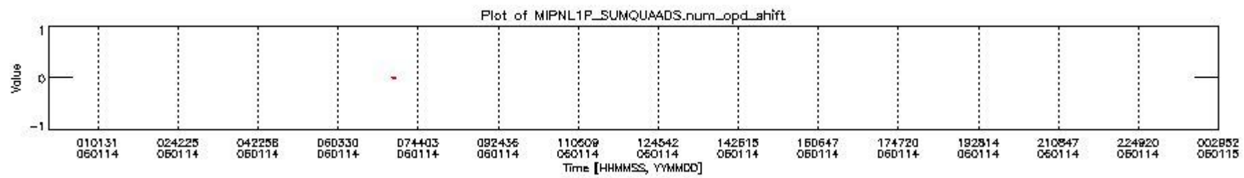
mipas_daily_report_level1_OFL_MIPAS_4_65_P_20060114_10.PNG
