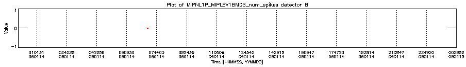
mipas_daily_report_level1_OFL_MIPAS_4_65_P_20060114_22.PNG
