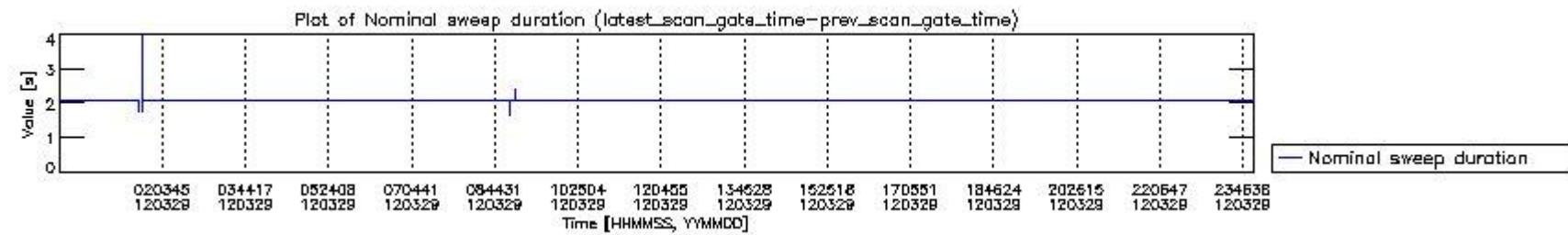
mipas_daily_report_level0_KSPT_L0_4504_N_20120329_4.PNG
