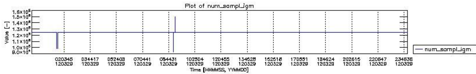
mipas_daily_report_level0_KSPT_L0_4504_N_20120329_0.PNG
