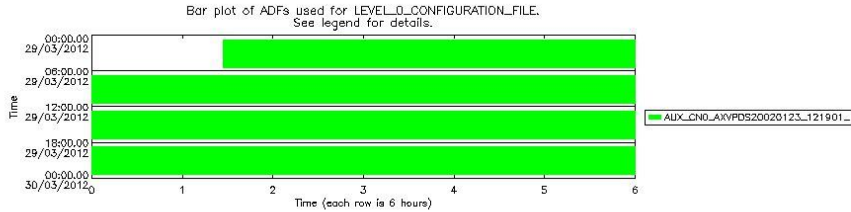
mipas_daily_report_level0_KSPT_L0_4504_N_20120329_12.PNG
