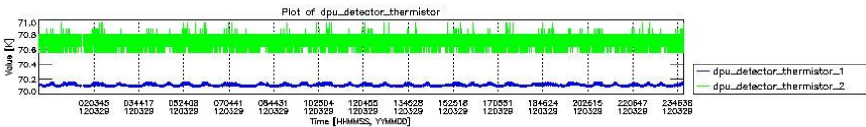
mipas_daily_report_level0_KSPT_L0_4504_N_20120329_3.PNG
