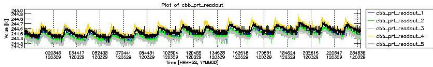
mipas_daily_report_level0_KSPT_L0_4504_N_20120329_9.PNG
