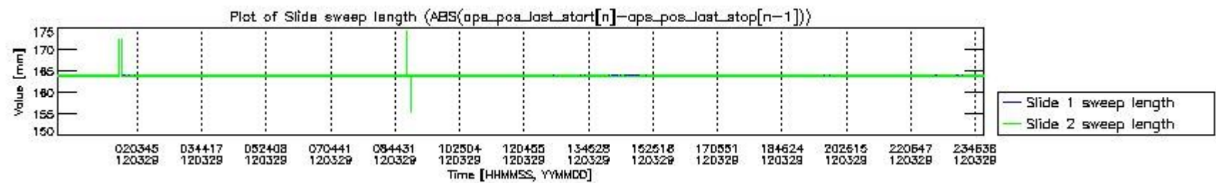
mipas_daily_report_level0_KSPT_L0_4504_N_20120329_7.PNG
