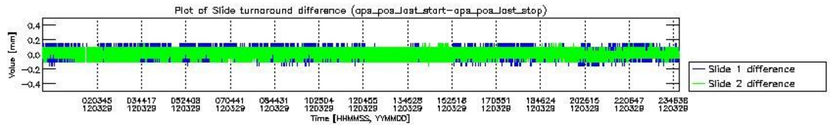
mipas_daily_report_level0_KSPT_L0_4504_N_20120329_5.PNG
