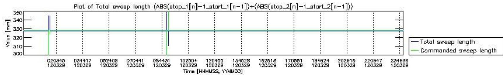
mipas_daily_report_level0_KSPT_L0_4504_N_20120329_6.PNG
