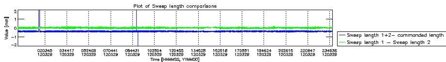
mipas_daily_report_level0_KSPT_L0_4504_N_20120329_8.PNG
