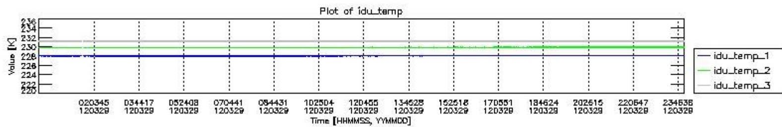
mipas_daily_report_level0_KSPT_L0_4504_N_20120329_2.PNG
