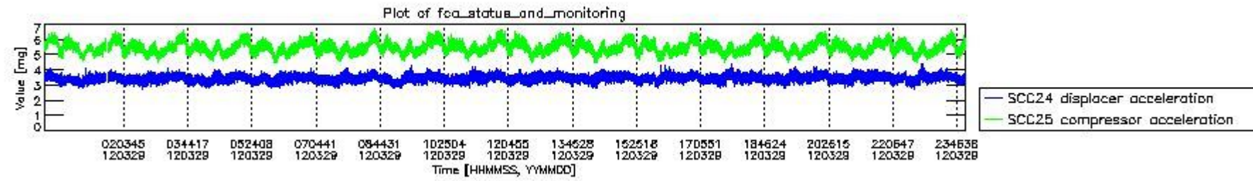
mipas_daily_report_level0_KSPT_L0_4504_N_20120329_10.PNG
