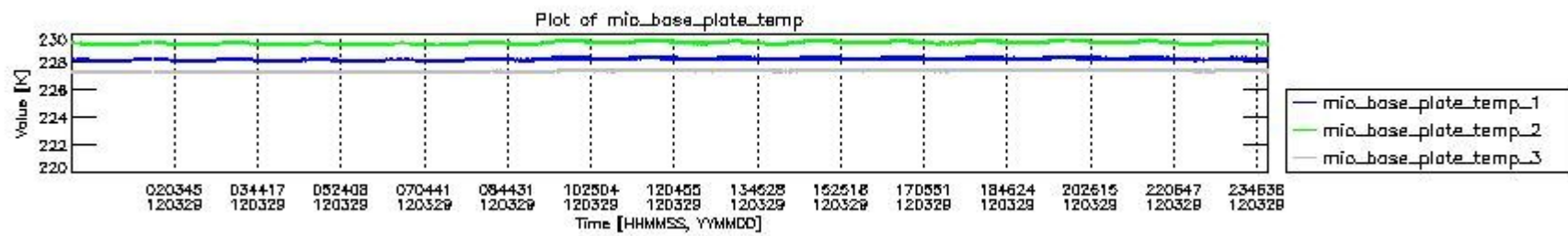
mipas_daily_report_level0_KSPT_L0_4504_N_20120329_1.PNG
