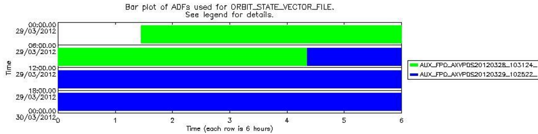
mipas_daily_report_level0_KSPT_L0_4504_N_20120329_13.PNG
