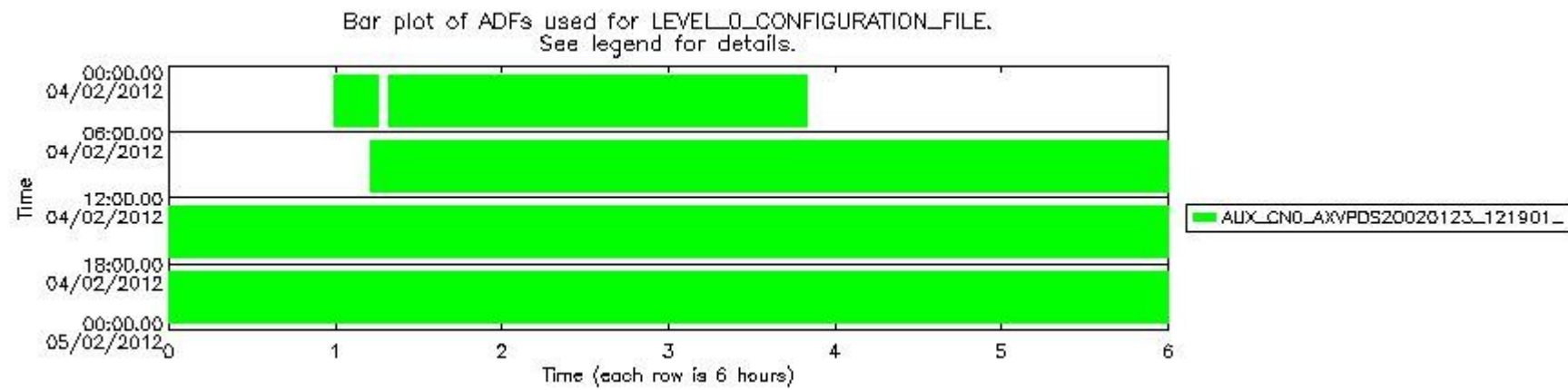
mipas_daily_report_level0_KSPT_L0_4504_N_20120204_12.PNG
