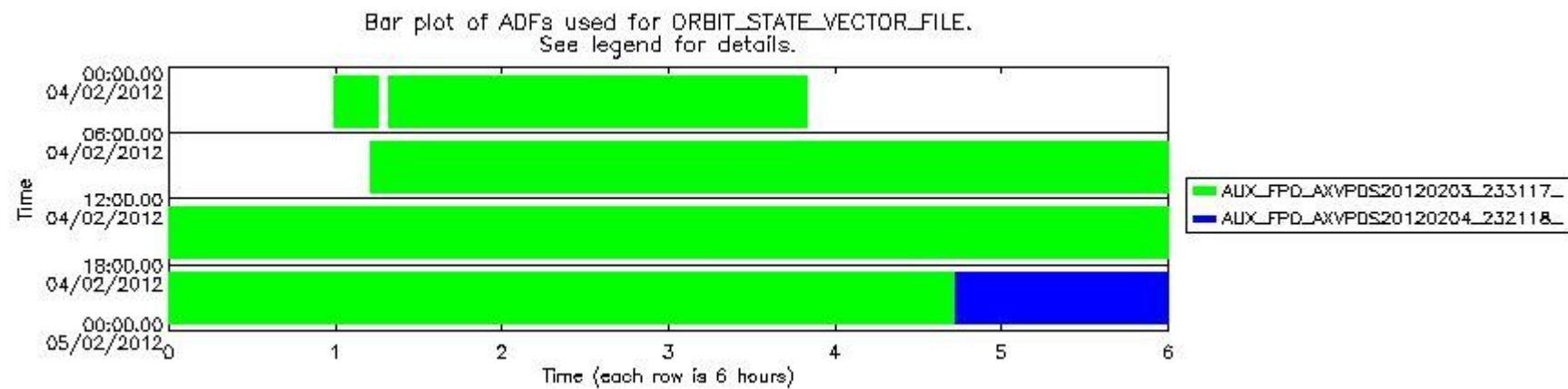
mipas_daily_report_level0_KSPT_L0_4504_N_20120204_13.PNG
