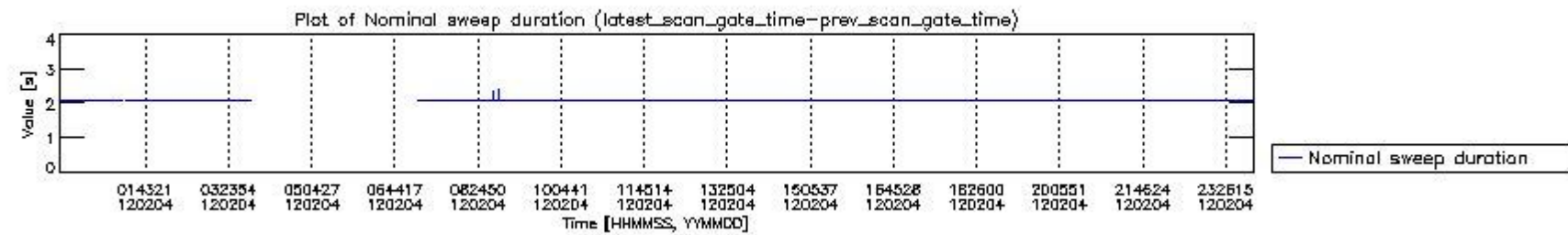
mipas_daily_report_level0_KSPT_L0_4504_N_20120204_4.PNG
