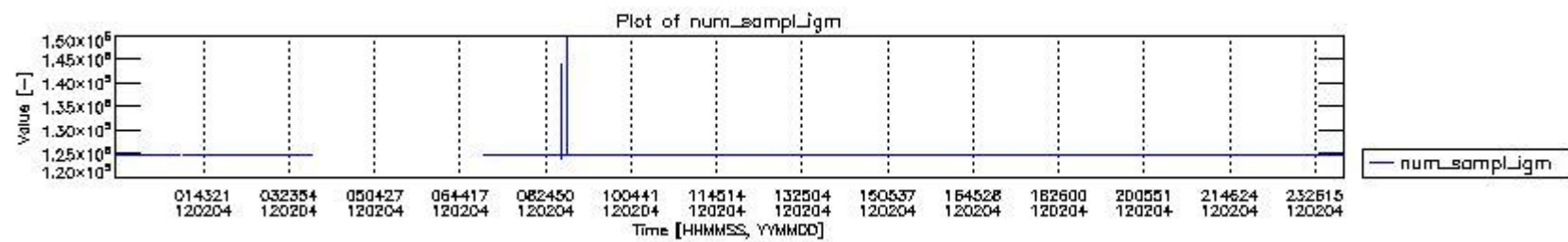
mipas_daily_report_level0_KSPT_L0_4504_N_20120204_0.PNG
