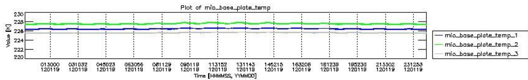
mipas_daily_report_level0_KSPT_L0_4504_N_20120119_1.PNG
