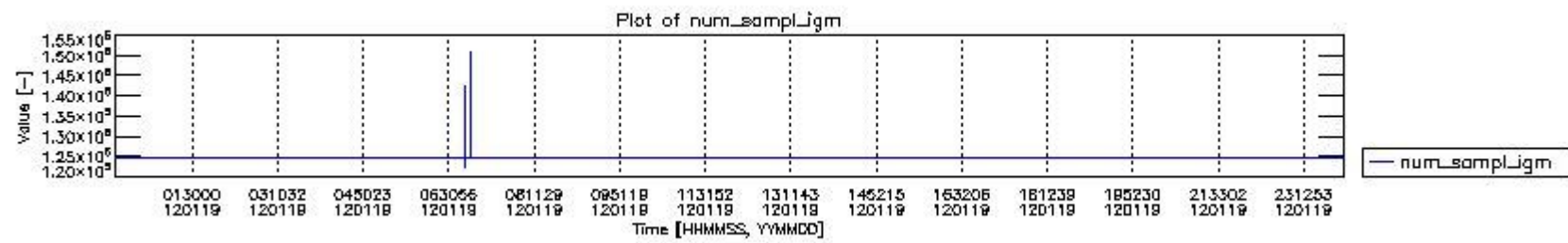
mipas_daily_report_level0_KSPT_L0_4504_N_20120119_0.PNG
