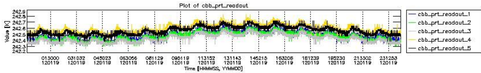
mipas_daily_report_level0_KSPT_L0_4504_N_20120119_9.PNG
