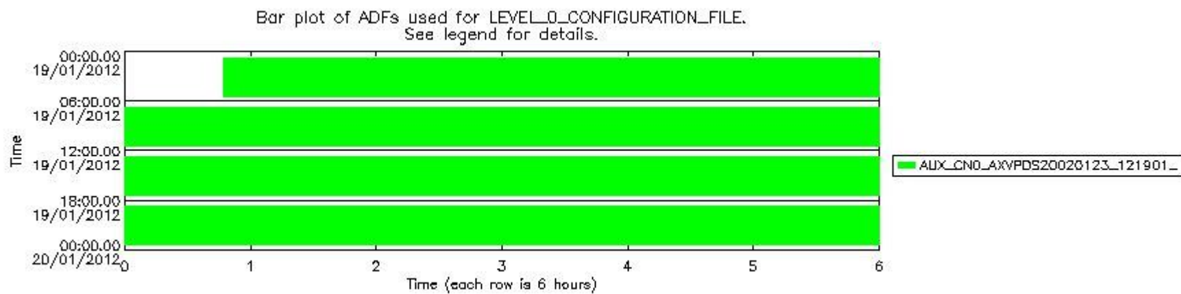
mipas_daily_report_level0_KSPT_L0_4504_N_20120119_12.PNG
