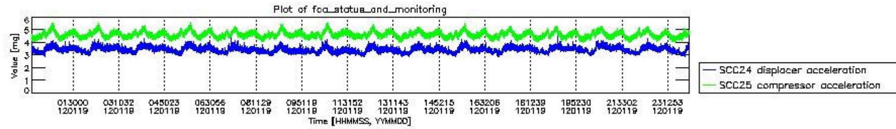
mipas_daily_report_level0_KSPT_L0_4504_N_20120119_10.PNG
