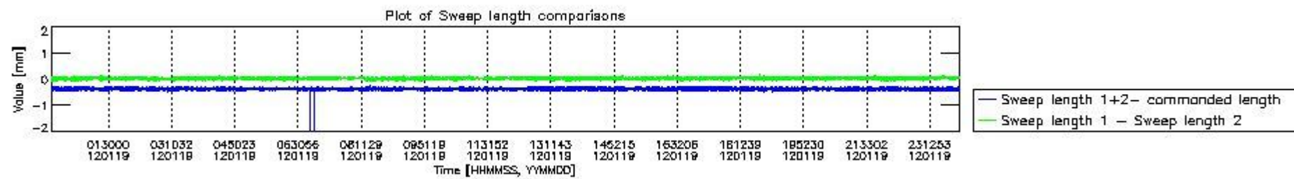
mipas_daily_report_level0_KSPT_L0_4504_N_20120119_8.PNG
