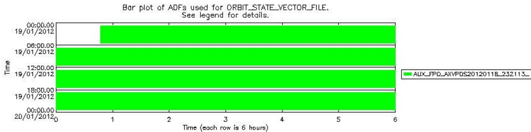
mipas_daily_report_level0_KSPT_L0_4504_N_20120119_13.PNG
