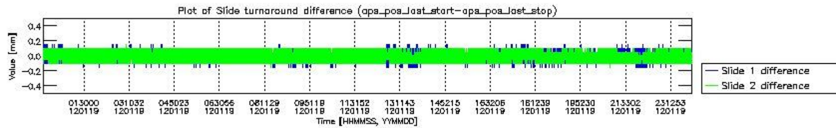
mipas_daily_report_level0_KSPT_L0_4504_N_20120119_5.PNG
