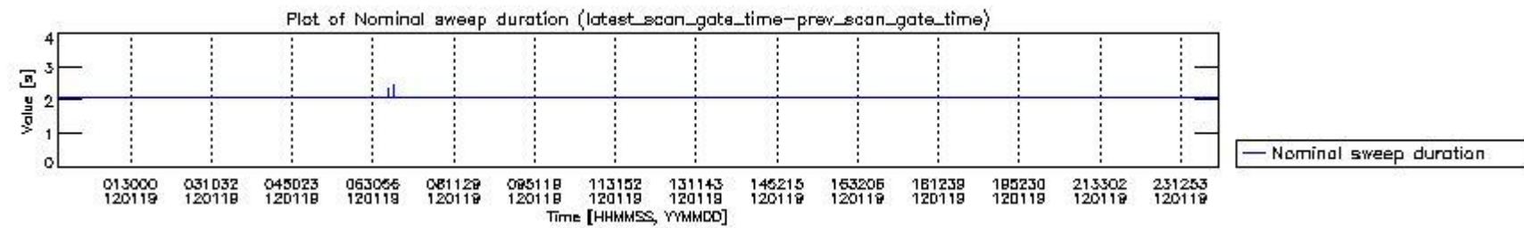
mipas_daily_report_level0_KSPT_L0_4504_N_20120119_4.PNG
