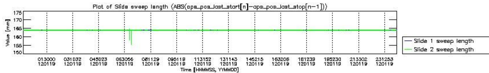
mipas_daily_report_level0_KSPT_L0_4504_N_20120119_7.PNG
