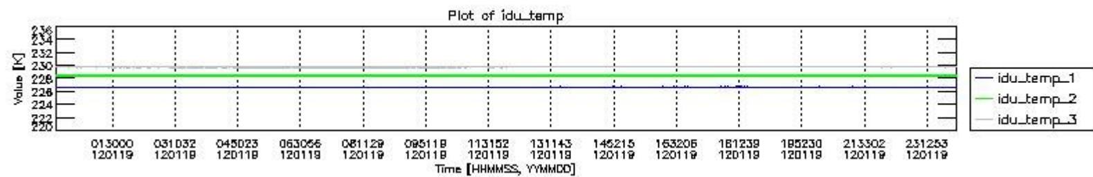
mipas_daily_report_level0_KSPT_L0_4504_N_20120119_2.PNG
