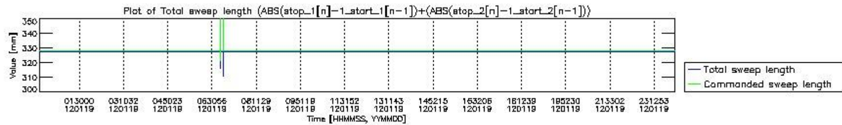
mipas_daily_report_level0_KSPT_L0_4504_N_20120119_6.PNG
