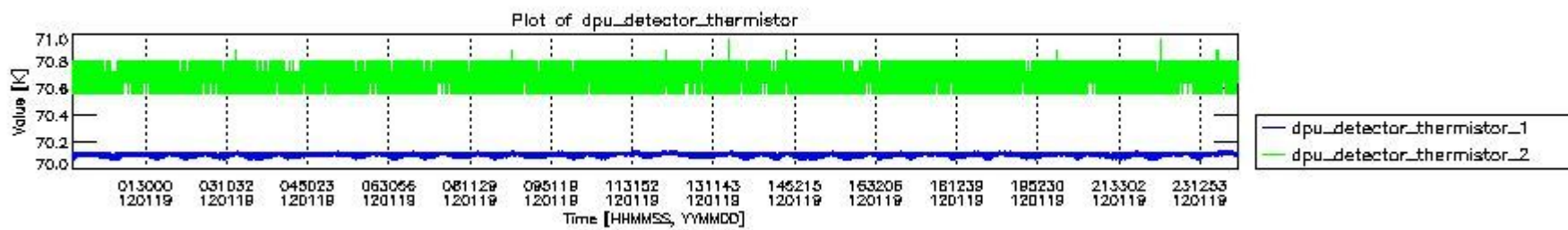
mipas_daily_report_level0_KSPT_L0_4504_N_20120119_3.PNG
