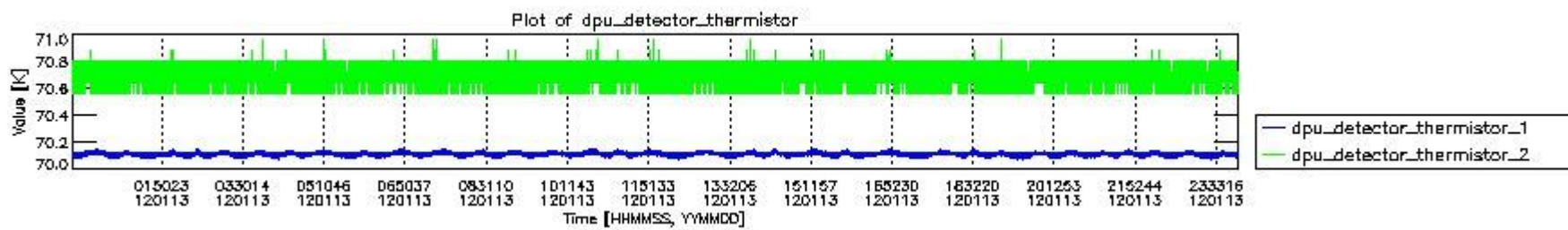
mipas_daily_report_level0_KSPT_L0_4504_N_20120113_3.PNG
