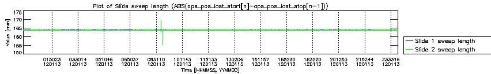
mipas_daily_report_level0_KSPT_L0_4504_N_20120113_7.PNG
