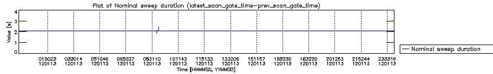
mipas_daily_report_level0_KSPT_L0_4504_N_20120113_4.PNG
