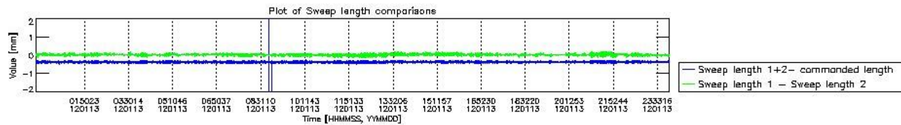
mipas_daily_report_level0_KSPT_L0_4504_N_20120113_8.PNG
