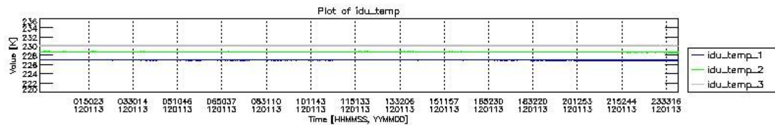
mipas_daily_report_level0_KSPT_L0_4504_N_20120113_2.PNG
