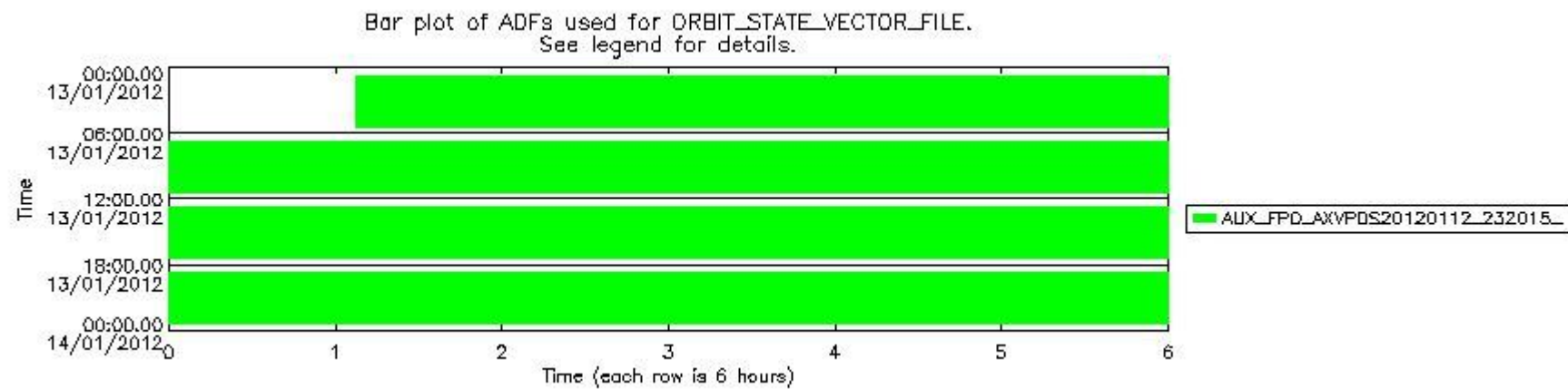
mipas_daily_report_level0_KSPT_L0_4504_N_20120113_13.PNG
