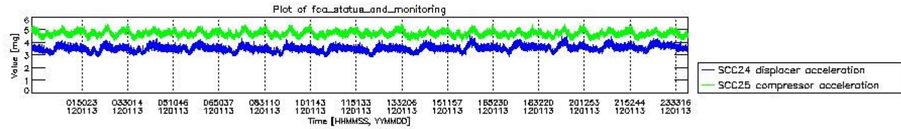
mipas_daily_report_level0_KSPT_L0_4504_N_20120113_10.PNG
