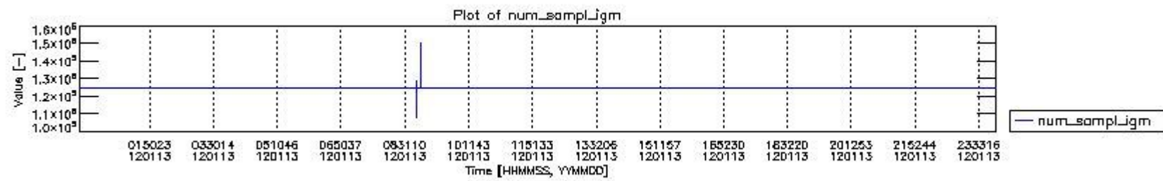
mipas_daily_report_level0_KSPT_L0_4504_N_20120113_0.PNG
