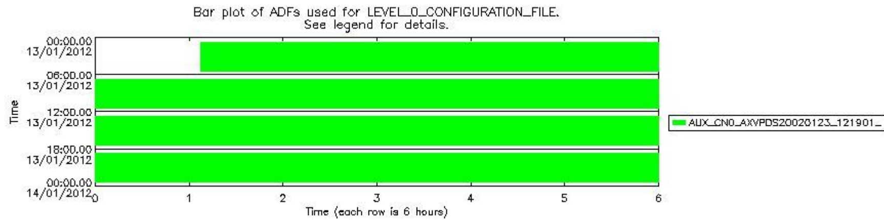
mipas_daily_report_level0_KSPT_L0_4504_N_20120113_12.PNG
