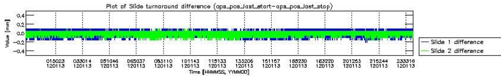
mipas_daily_report_level0_KSPT_L0_4504_N_20120113_5.PNG
