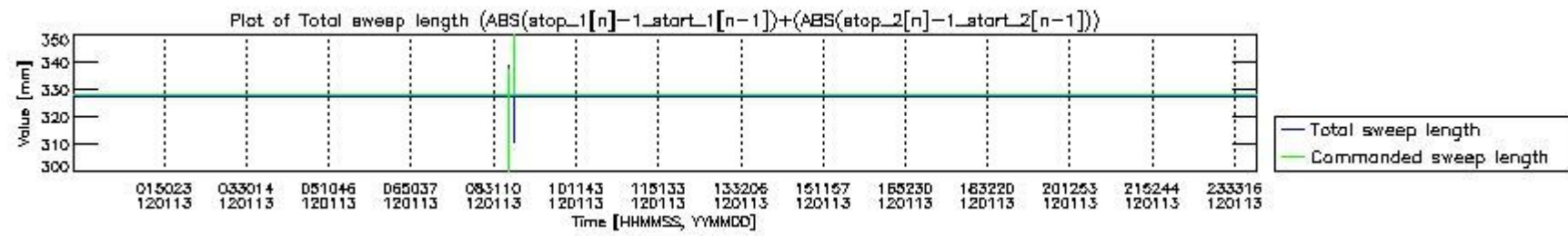
mipas_daily_report_level0_KSPT_L0_4504_N_20120113_6.PNG
