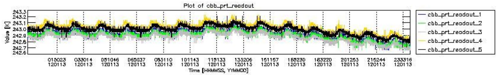
mipas_daily_report_level0_KSPT_L0_4504_N_20120113_9.PNG
