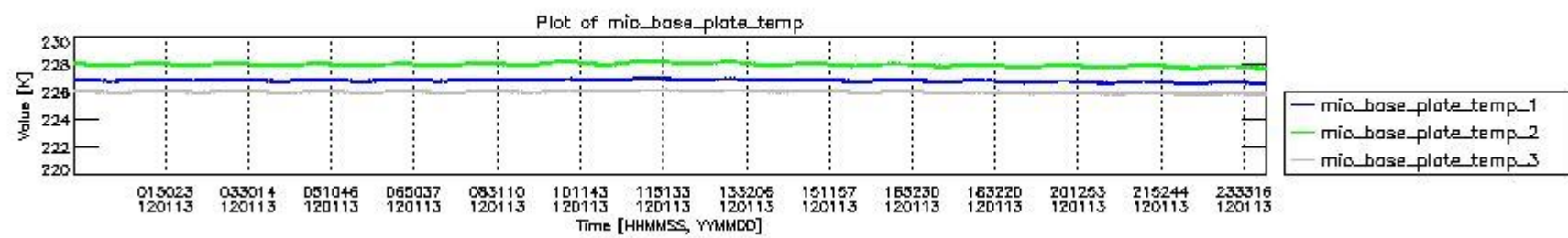
mipas_daily_report_level0_KSPT_L0_4504_N_20120113_1.PNG
