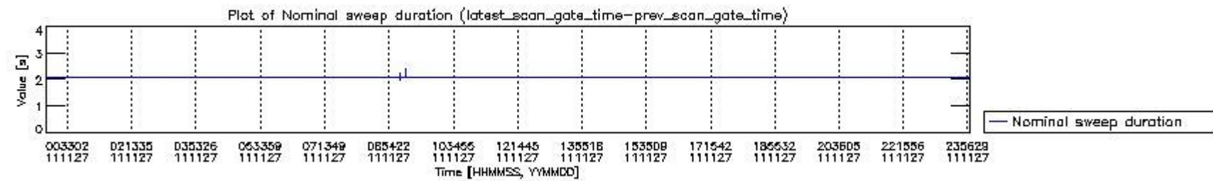
mipas_daily_report_level0_KSPT_L0_4504_N_20111127_4.PNG
