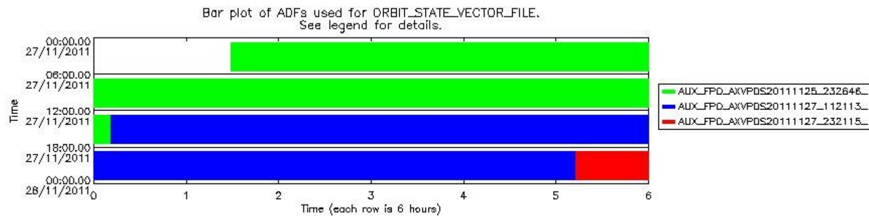
mipas_daily_report_level0_KSPT_L0_4504_N_20111127_13.PNG
