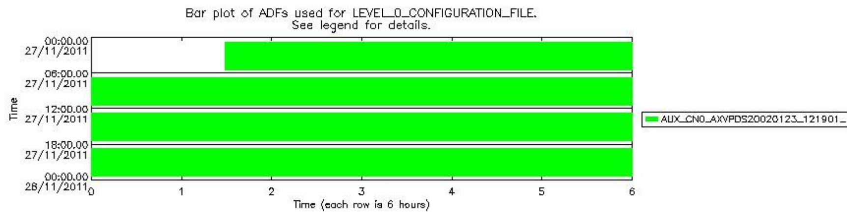
mipas_daily_report_level0_KSPT_L0_4504_N_20111127_12.PNG
