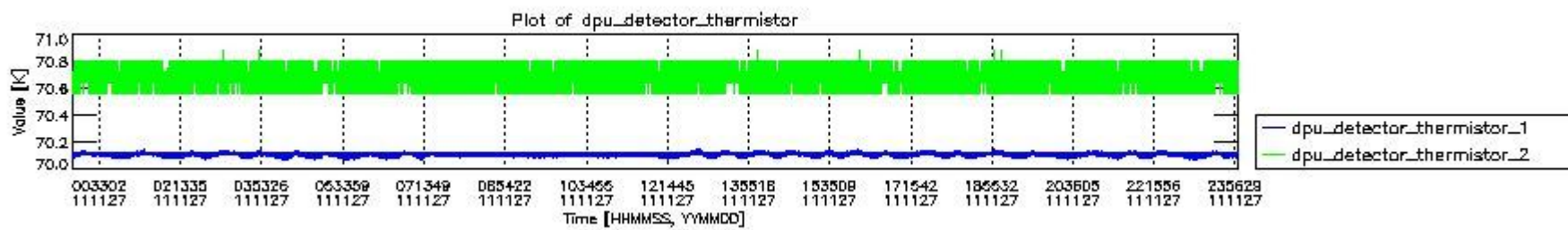
mipas_daily_report_level0_KSPT_L0_4504_N_20111127_3.PNG
