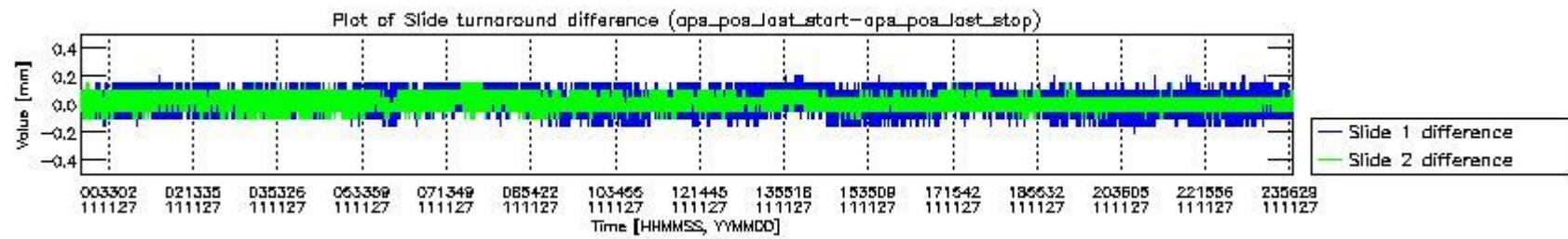
mipas_daily_report_level0_KSPT_L0_4504_N_20111127_5.PNG
