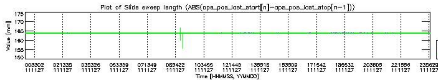
mipas_daily_report_level0_KSPT_L0_4504_N_20111127_7.PNG
