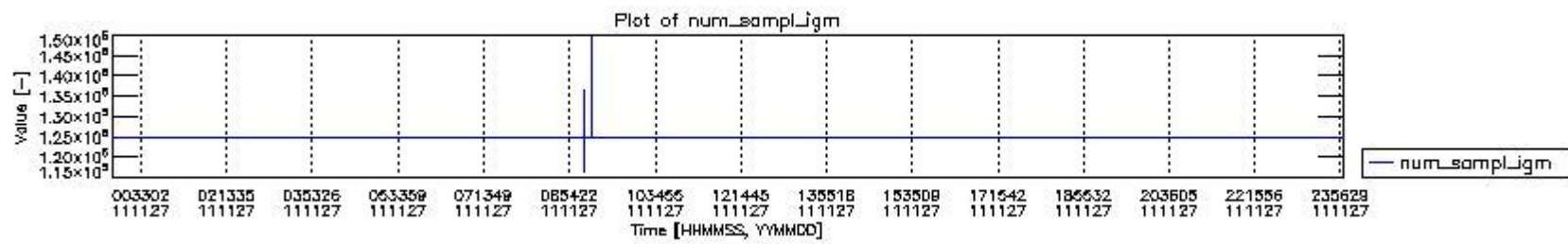
mipas_daily_report_level0_KSPT_L0_4504_N_20111127_0.PNG
