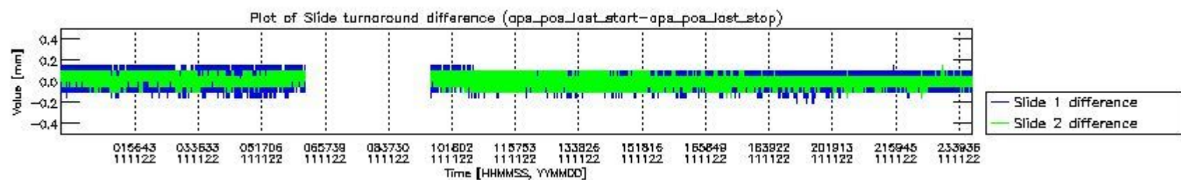
mipas_daily_report_level0_KSPT_L0_4504_N_20111122_5.PNG
