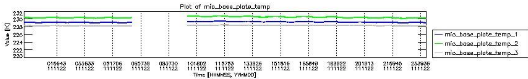
mipas_daily_report_level0_KSPT_L0_4504_N_20111122_1.PNG
