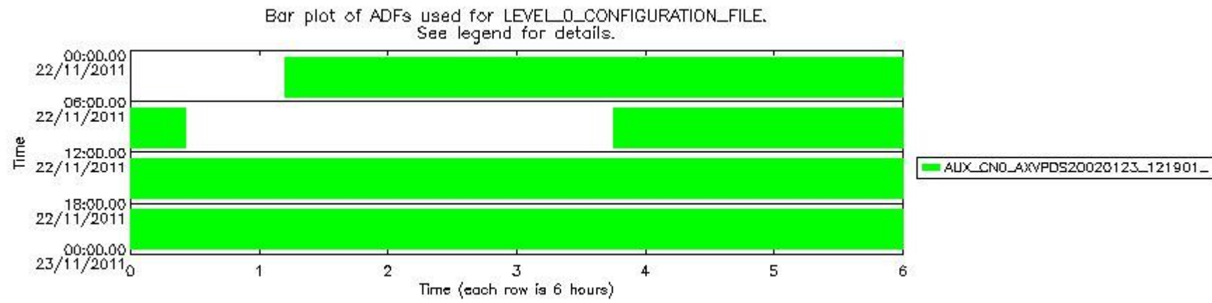
mipas_daily_report_level0_KSPT_L0_4504_N_20111122_12.PNG
