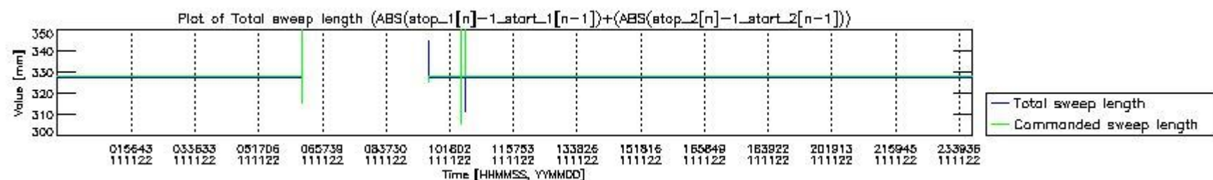
mipas_daily_report_level0_KSPT_L0_4504_N_20111122_6.PNG
