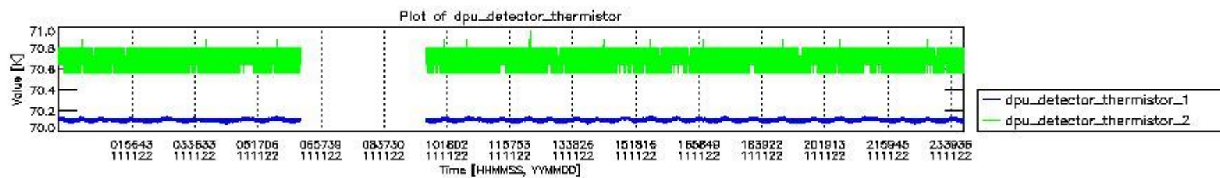
mipas_daily_report_level0_KSPT_L0_4504_N_20111122_3.PNG
