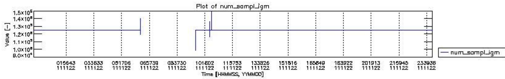
mipas_daily_report_level0_KSPT_L0_4504_N_20111122_0.PNG
