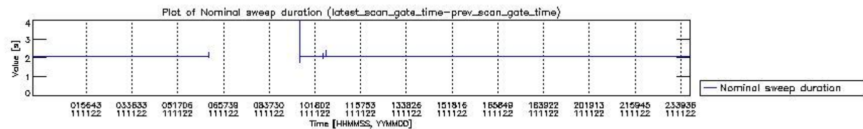
mipas_daily_report_level0_KSPT_L0_4504_N_20111122_4.PNG
