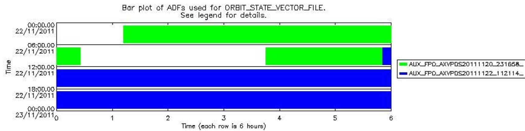
mipas_daily_report_level0_KSPT_L0_4504_N_20111122_13.PNG
