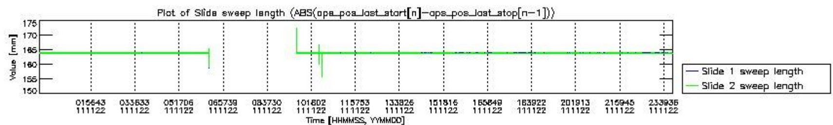
mipas_daily_report_level0_KSPT_L0_4504_N_20111122_7.PNG
