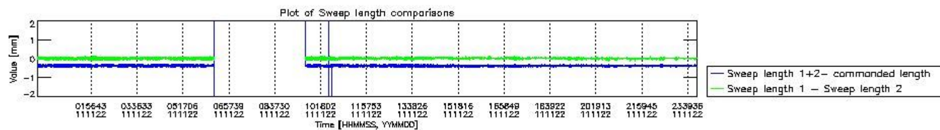
mipas_daily_report_level0_KSPT_L0_4504_N_20111122_8.PNG
