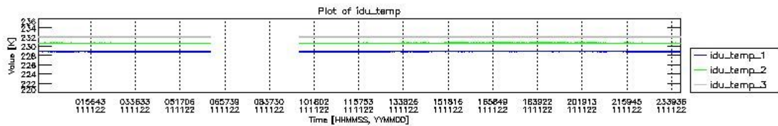
mipas_daily_report_level0_KSPT_L0_4504_N_20111122_2.PNG
