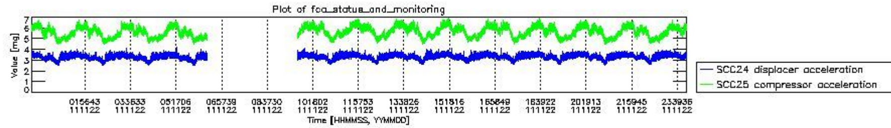
mipas_daily_report_level0_KSPT_L0_4504_N_20111122_10.PNG
