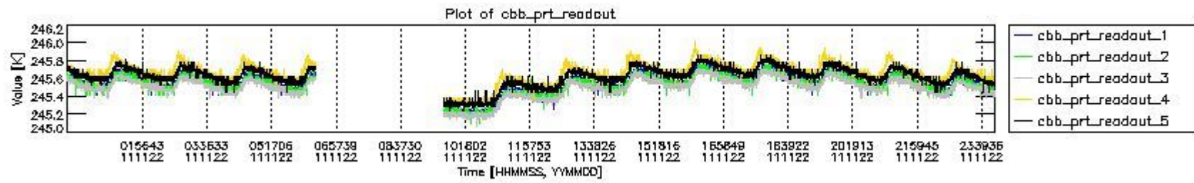
mipas_daily_report_level0_KSPT_L0_4504_N_20111122_9.PNG
