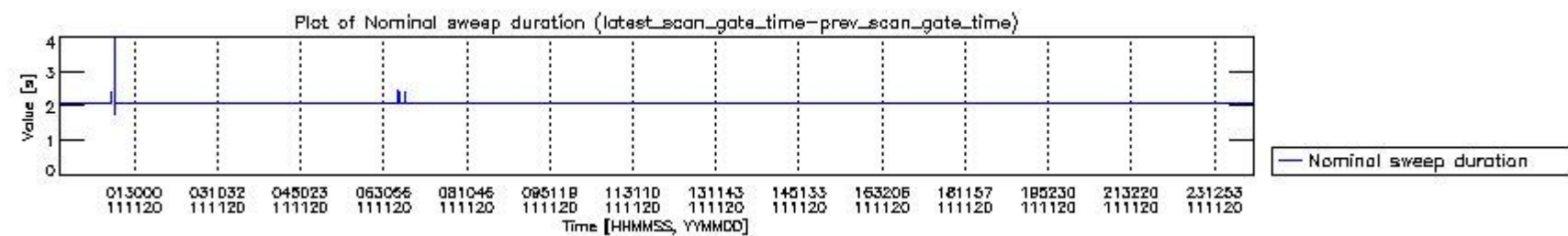
mipas_daily_report_level0_KSPT_L0_4504_N_20111120_4.PNG
