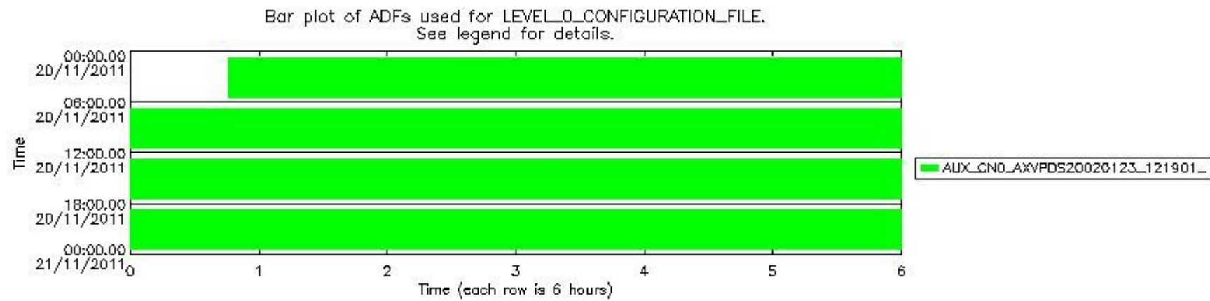
mipas_daily_report_level0_KSPT_L0_4504_N_20111120_12.PNG
