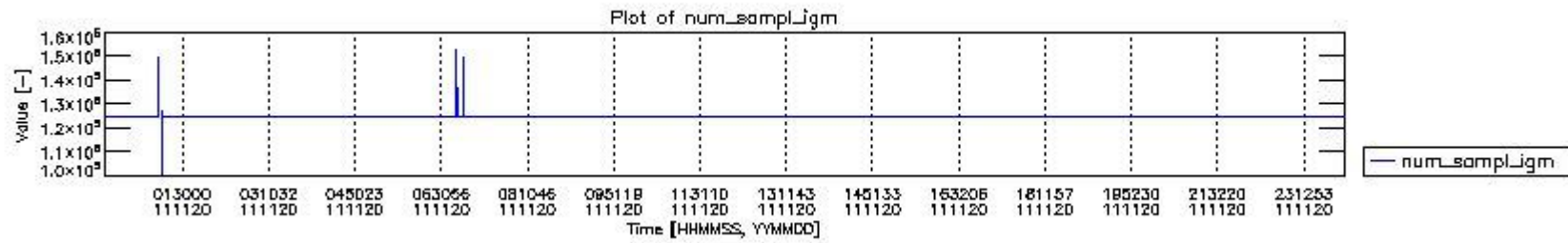
mipas_daily_report_level0_KSPT_L0_4504_N_20111120_0.PNG
