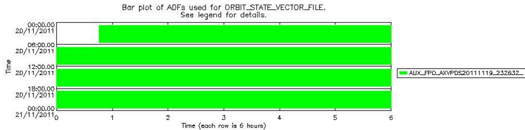
mipas_daily_report_level0_KSPT_L0_4504_N_20111120_13.PNG
