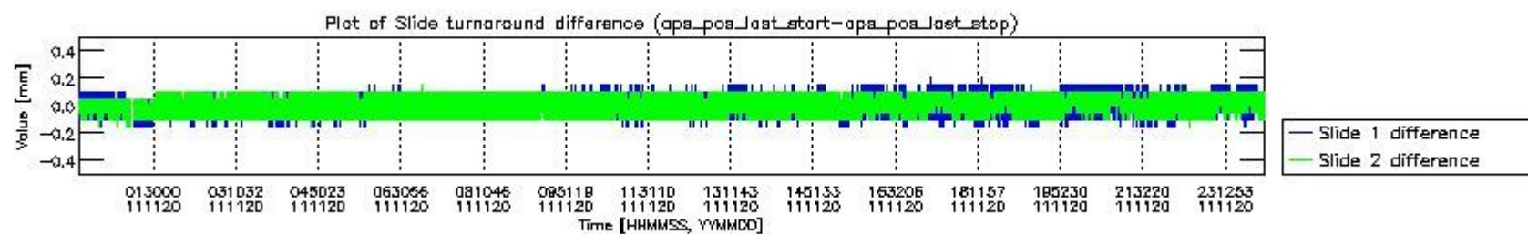
mipas_daily_report_level0_KSPT_L0_4504_N_20111120_5.PNG
