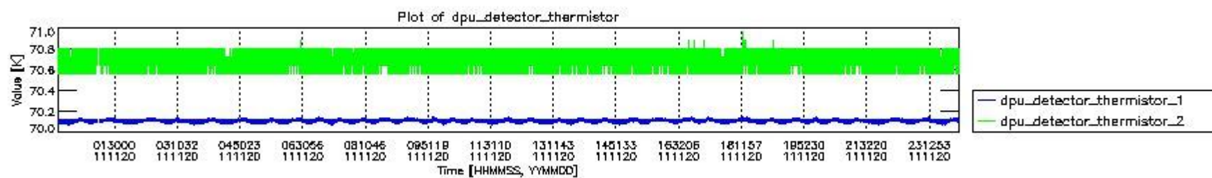
mipas_daily_report_level0_KSPT_L0_4504_N_20111120_3.PNG
