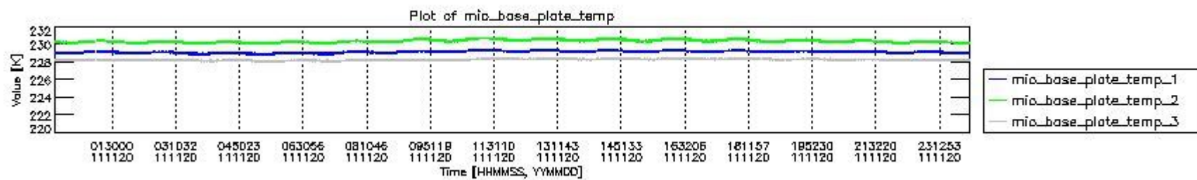
mipas_daily_report_level0_KSPT_L0_4504_N_20111120_1.PNG
