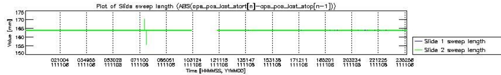
mipas_daily_report_level0_KSPT_L0_4504_N_20111108_7.PNG
