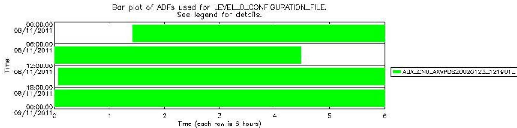
mipas_daily_report_level0_KSPT_L0_4504_N_20111108_12.PNG
