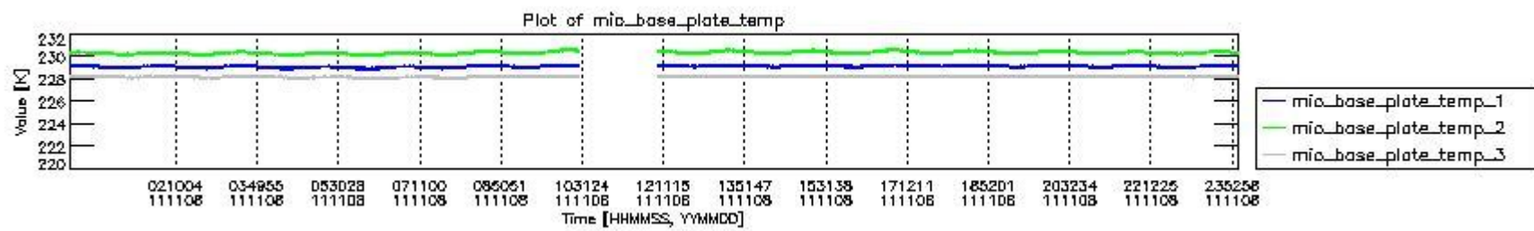
mipas_daily_report_level0_KSPT_L0_4504_N_20111108_1.PNG
