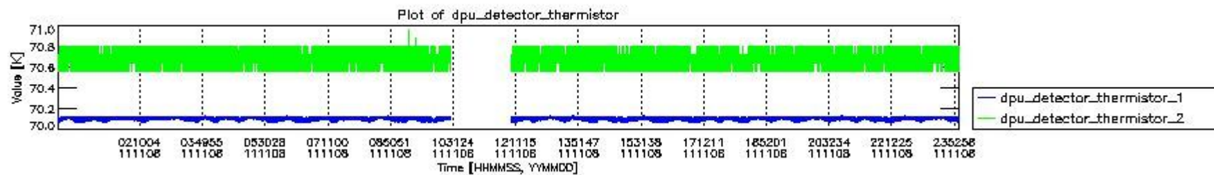
mipas_daily_report_level0_KSPT_L0_4504_N_20111108_3.PNG
