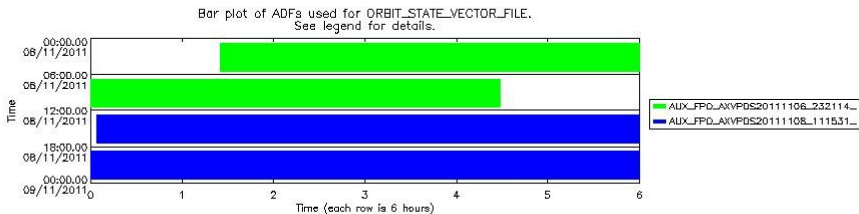
mipas_daily_report_level0_KSPT_L0_4504_N_20111108_13.PNG
