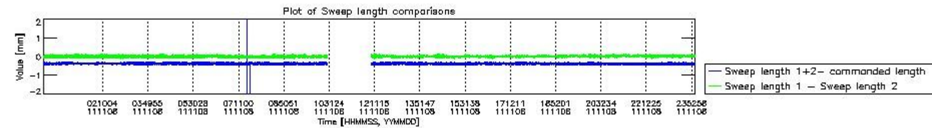
mipas_daily_report_level0_KSPT_L0_4504_N_20111108_8.PNG
