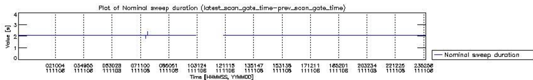
mipas_daily_report_level0_KSPT_L0_4504_N_20111108_3.PNG
