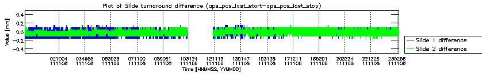
mipas_daily_report_level0_KSPT_L0_4504_N_20111108_5.PNG
