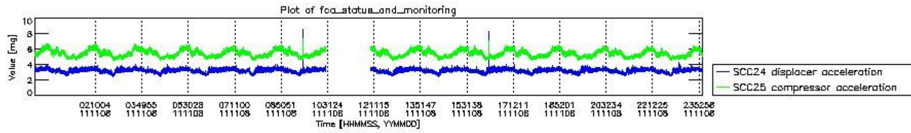
mipas_daily_report_level0_KSPT_L0_4504_N_20111108_10.PNG
