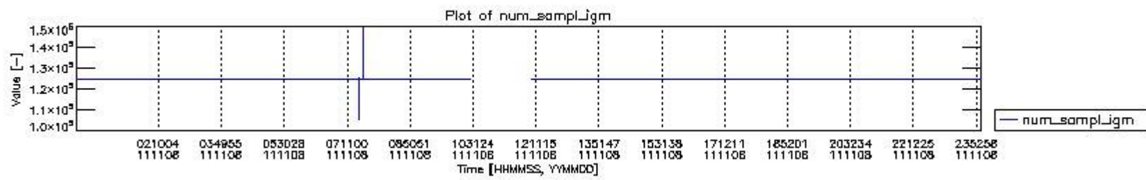
mipas_daily_report_level0_KSPT_L0_4504_N_20111108_0.PNG
