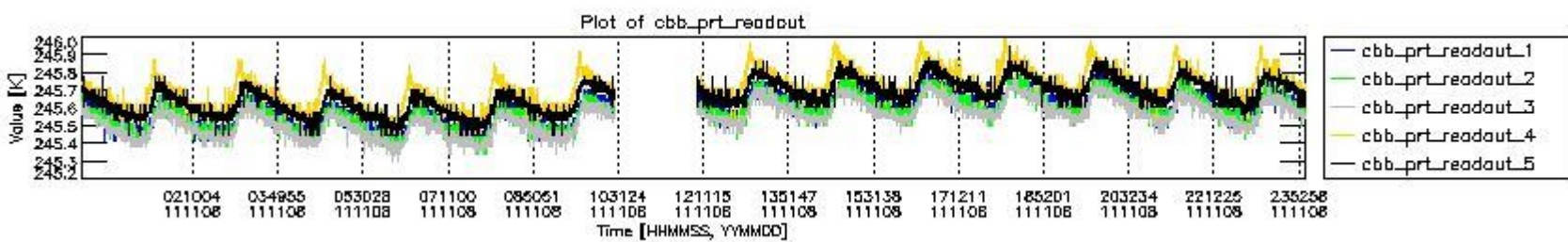
mipas_daily_report_level0_KSPT_L0_4504_N_20111108_9.PNG
