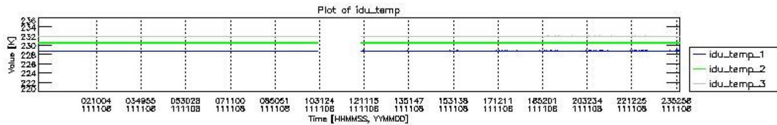
mipas_daily_report_level0_KSPT_L0_4504_N_20111108_2.PNG
