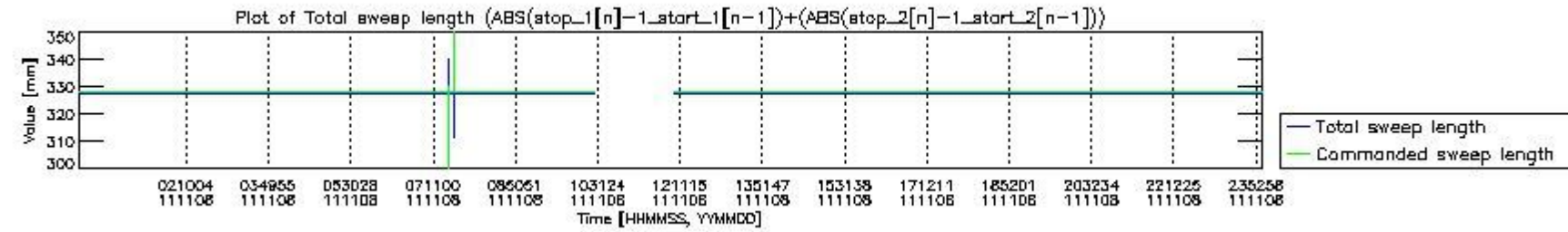
mipas_daily_report_level0_KSPT_L0_4504_N_20111108_6.PNG
