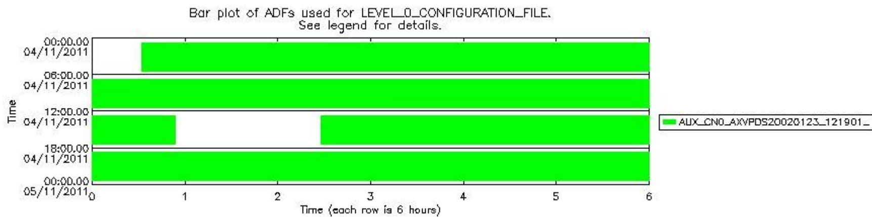
mipas_daily_report_level0_KSPT_L0_4504_N_20111104_12.PNG
