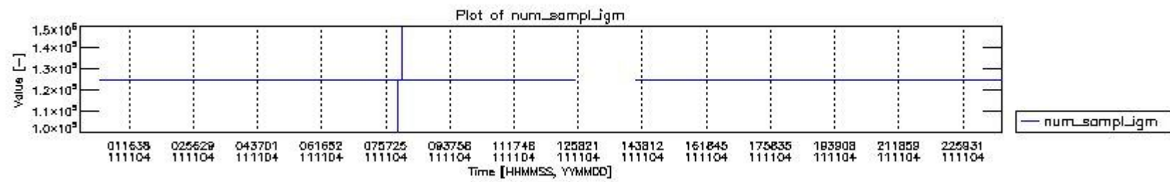
mipas_daily_report_level0_KSPT_L0_4504_N_20111104_0.PNG
