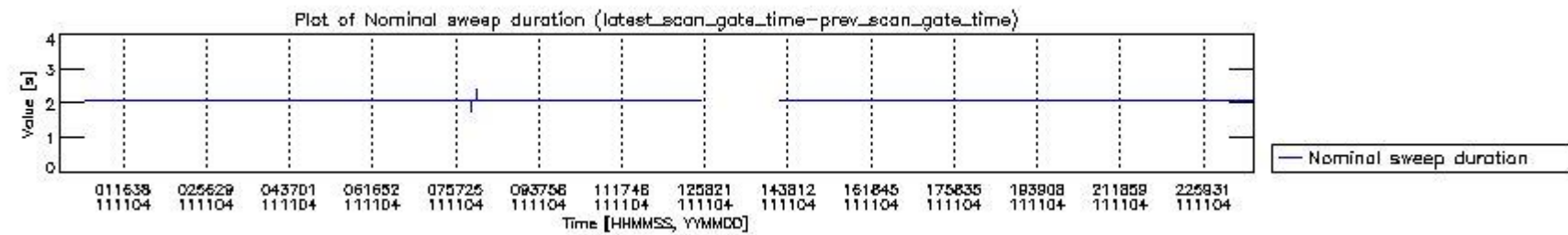
mipas_daily_report_level0_KSPT_L0_4504_N_20111104_4.PNG
