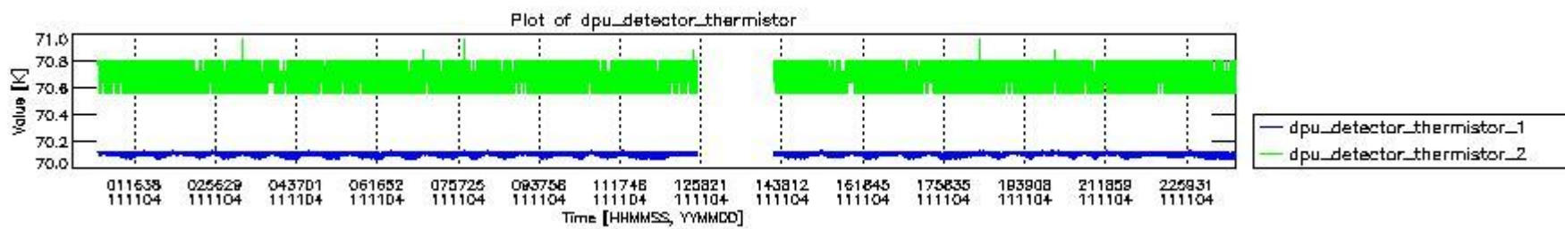
mipas_daily_report_level0_KSPT_L0_4504_N_20111104_3.PNG
