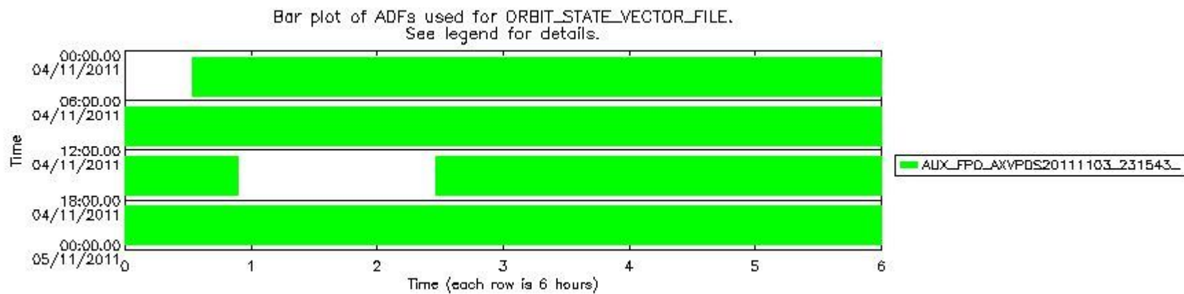
mipas_daily_report_level0_KSPT_L0_4504_N_20111104_13.PNG
