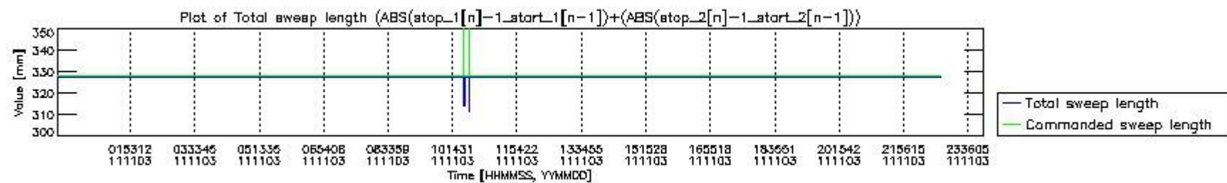
mipas_daily_report_level0_KSPT_L0_4504_N_20111103_6.PNG
