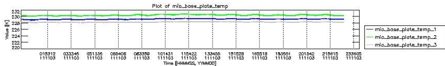
mipas_daily_report_level0_KSPT_L0_4504_N_20111103_1.PNG
