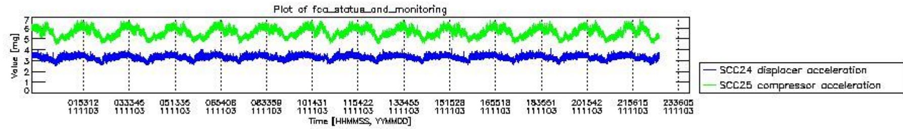
mipas_daily_report_level0_KSPT_L0_4504_N_20111103_10.PNG
