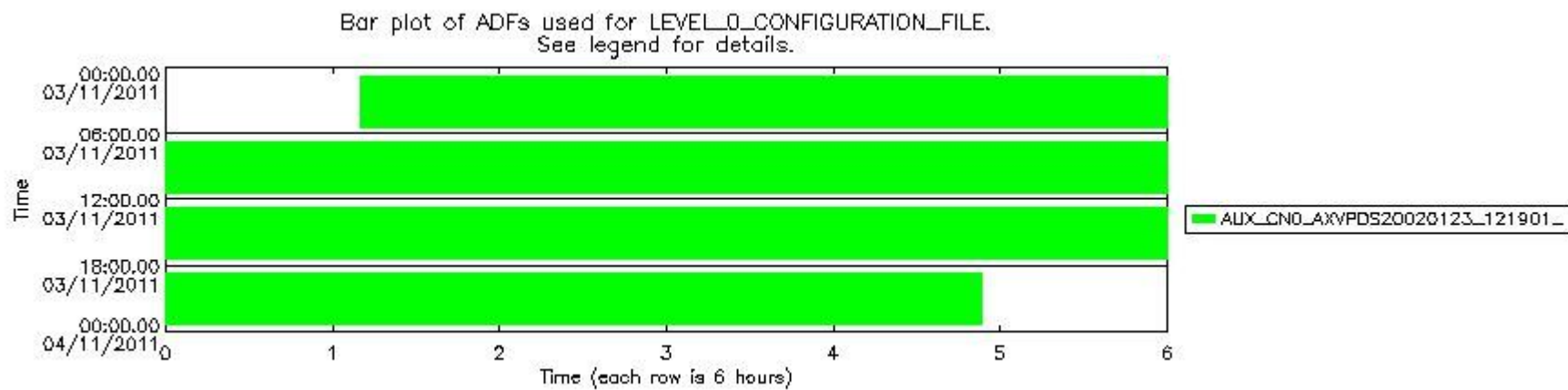
mipas_daily_report_level0_KSPT_L0_4504_N_20111103_12.PNG
