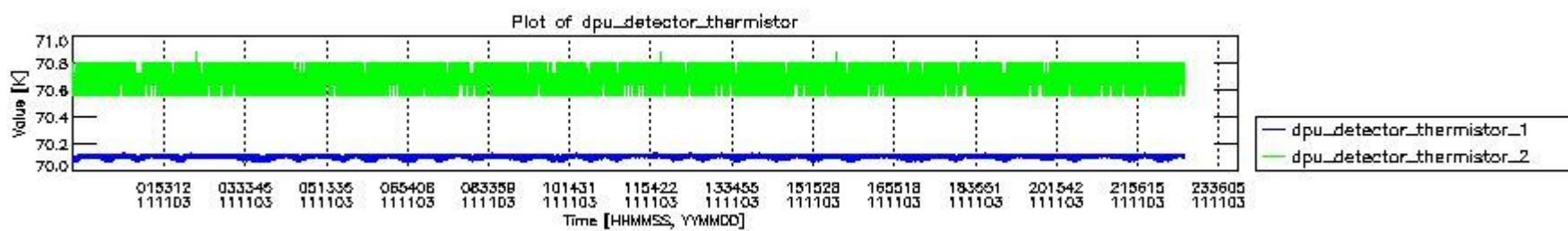
mipas_daily_report_level0_KSPT_L0_4504_N_20111103_3.PNG
