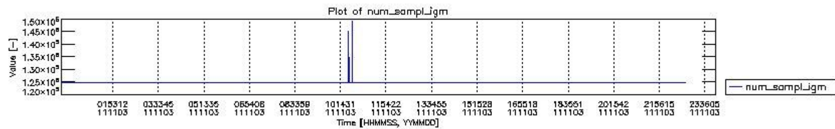
mipas_daily_report_level0_KSPT_L0_4504_N_20111103_0.PNG
