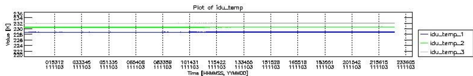
mipas_daily_report_level0_KSPT_L0_4504_N_20111103_2.PNG
