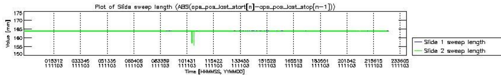
mipas_daily_report_level0_KSPT_L0_4504_N_20111103_7.PNG
