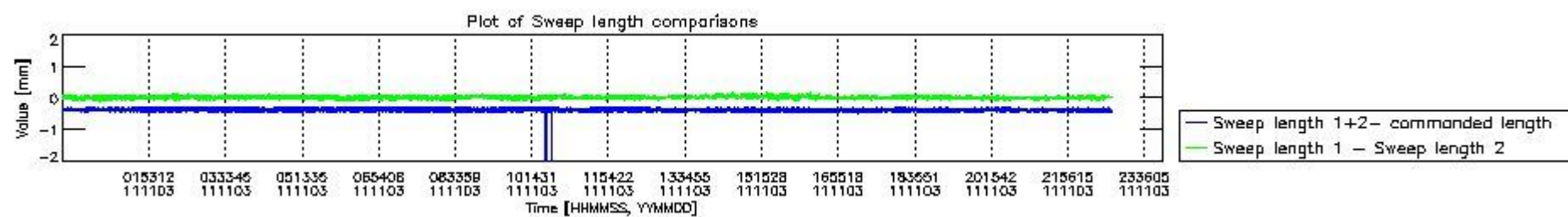
mipas_daily_report_level0_KSPT_L0_4504_N_20111103_8.PNG
