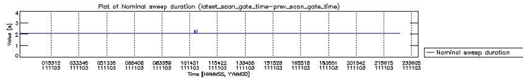
mipas_daily_report_level0_KSPT_L0_4504_N_20111103_4.PNG
