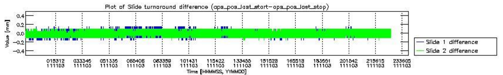
mipas_daily_report_level0_KSPT_L0_4504_N_20111103_5.PNG
