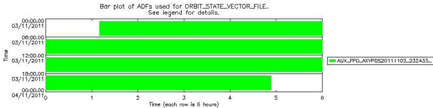
mipas_daily_report_level0_KSPT_L0_4504_N_20111103_13.PNG
