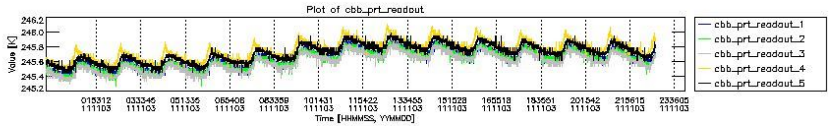
mipas_daily_report_level0_KSPT_L0_4504_N_20111103_9.PNG
