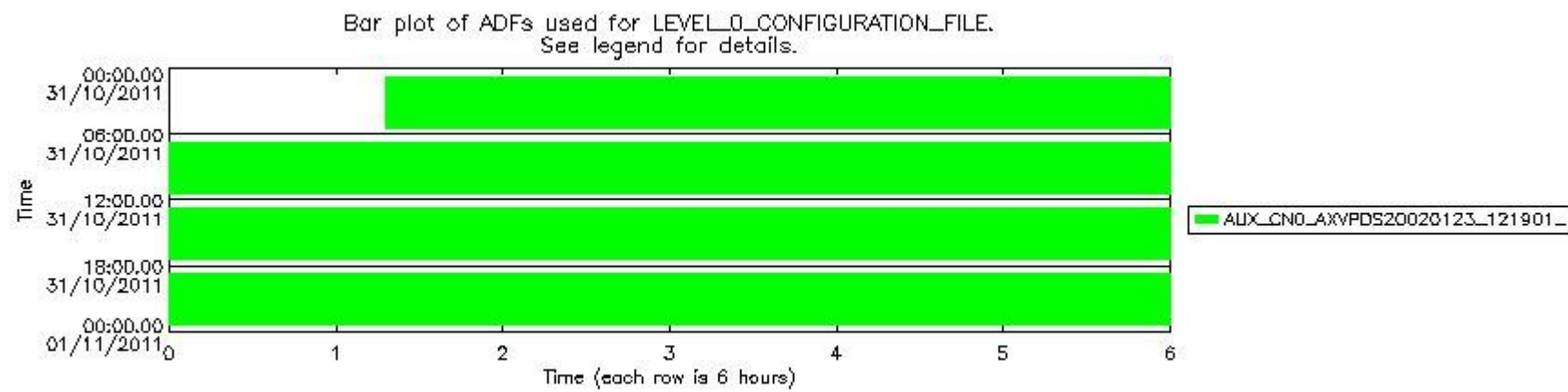
mipas_daily_report_level0_KSPT_L0_4504_N_20111031_12.PNG
