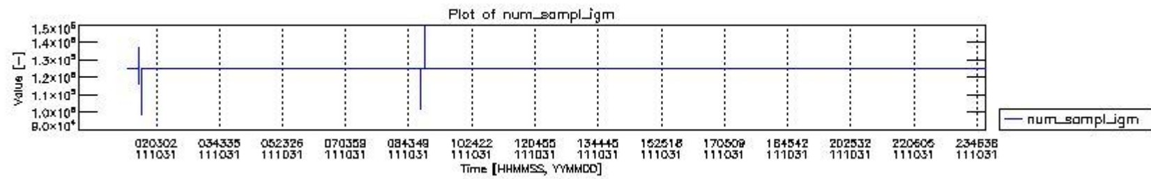
mipas_daily_report_level0_KSPT_L0_4504_N_20111031_0.PNG
