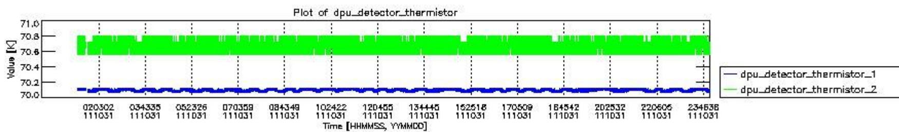
mipas_daily_report_level0_KSPT_L0_4504_N_20111031_3.PNG
