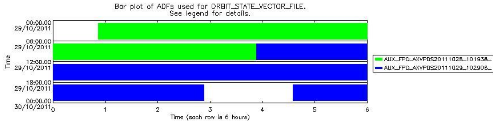
mipas_daily_report_level0_KSPT_L0_4504_N_20111029_13.PNG
