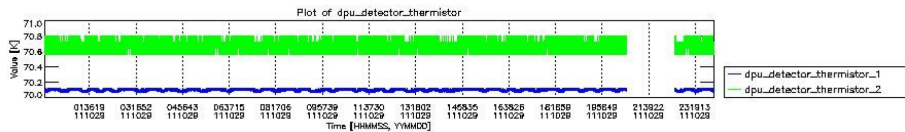
mipas_daily_report_level0_KSPT_L0_4504_N_20111029_3.PNG
