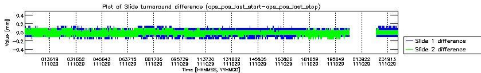
mipas_daily_report_level0_KSPT_L0_4504_N_20111029_5.PNG
