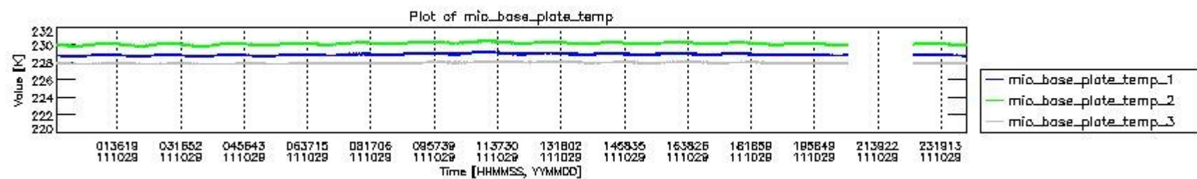
mipas_daily_report_level0_KSPT_L0_4504_N_20111029_1.PNG
