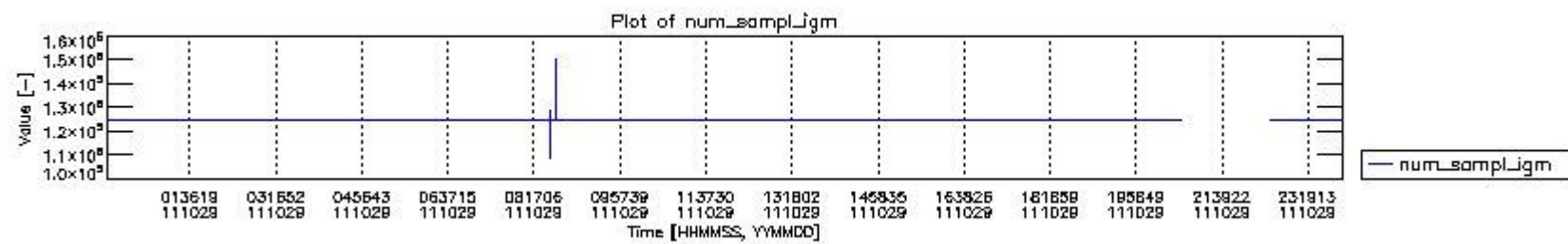
mipas_daily_report_level0_KSPT_L0_4504_N_20111029_0.PNG
