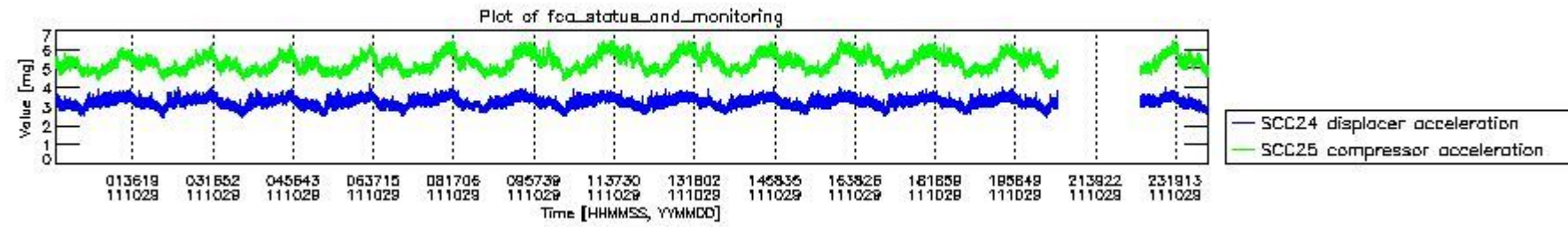
mipas_daily_report_level0_KSPT_L0_4504_N_20111029_10.PNG
