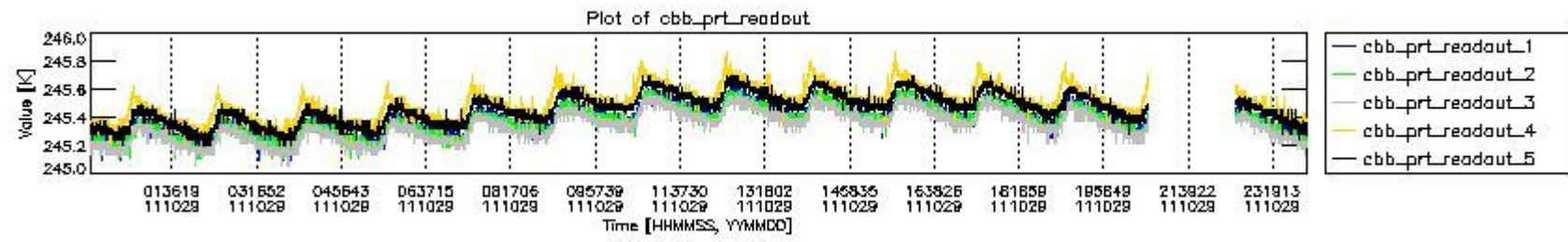
mipas_daily_report_level0_KSPT_L0_4504_N_20111029_9.PNG
