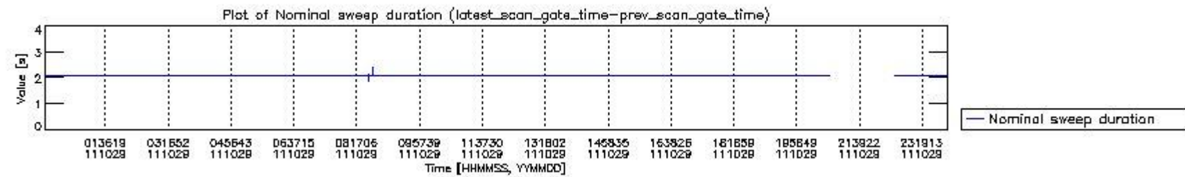
mipas_daily_report_level0_KSPT_L0_4504_N_20111029_4.PNG
