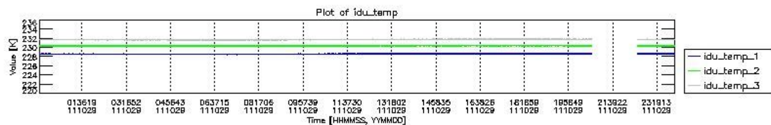
mipas_daily_report_level0_KSPT_L0_4504_N_20111029_2.PNG
