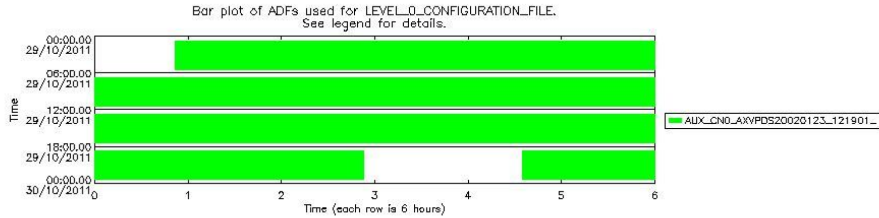
mipas_daily_report_level0_KSPT_L0_4504_N_20111029_12.PNG
