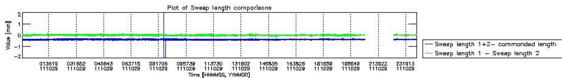
mipas_daily_report_level0_KSPT_L0_4504_N_20111029_8.PNG
