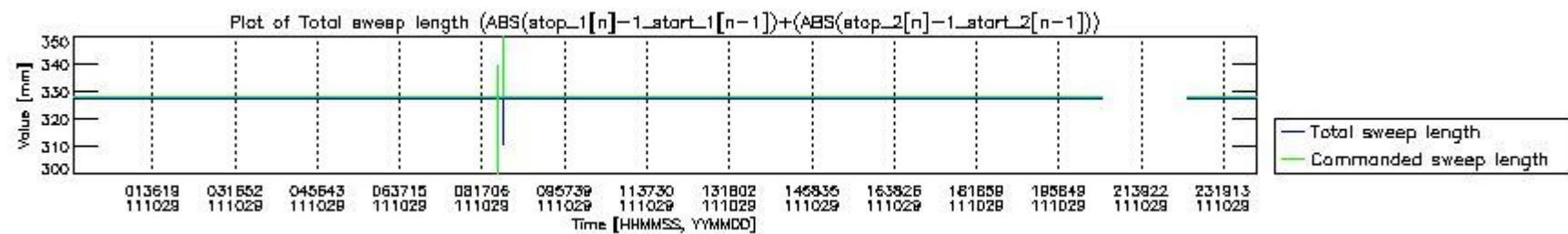
mipas_daily_report_level0_KSPT_L0_4504_N_20111029_6.PNG
