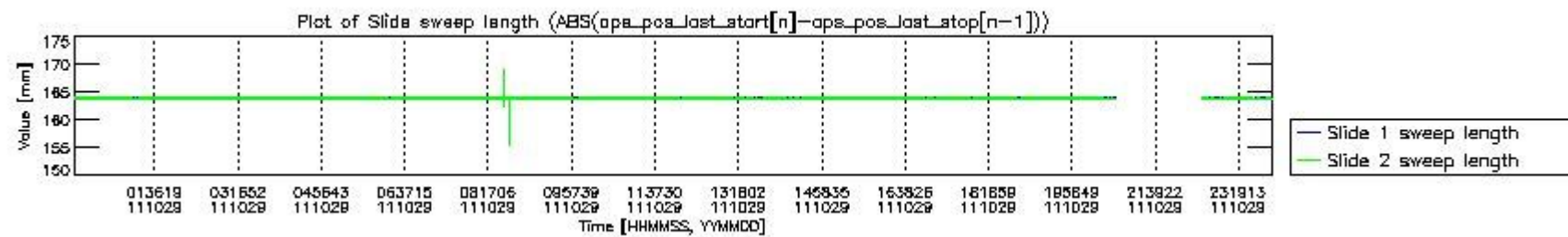
mipas_daily_report_level0_KSPT_L0_4504_N_20111029_7.PNG
