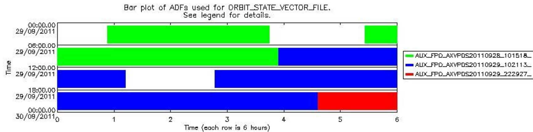
mipas_daily_report_level0_KSPT_L0_4504_N_20110929_13.PNG
