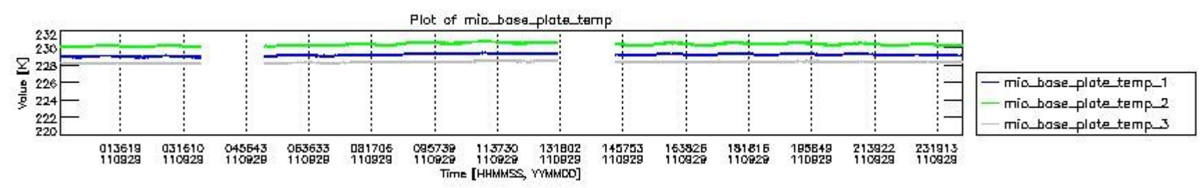
mipas_daily_report_level0_KSPT_L0_4504_N_20110929_1.PNG
