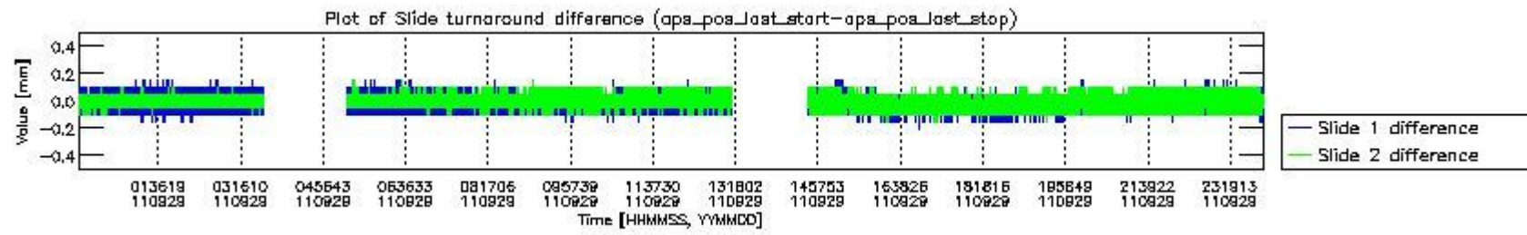
mipas_daily_report_level0_KSPT_L0_4504_N_20110929_5.PNG
