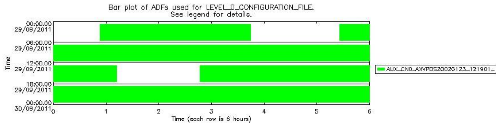
mipas_daily_report_level0_KSPT_L0_4504_N_20110929_12.PNG
