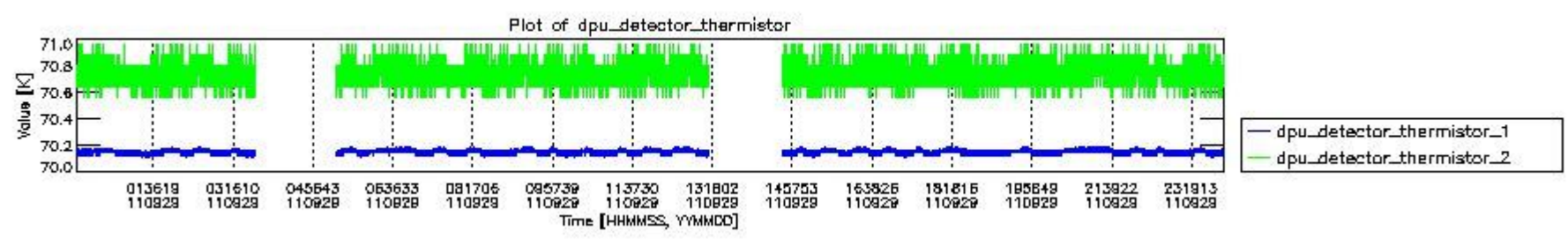
mipas_daily_report_level0_KSPT_L0_4504_N_20110929_3.PNG
