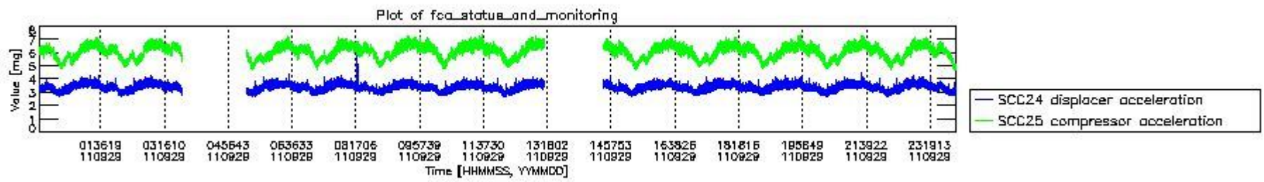
mipas_daily_report_level0_KSPT_L0_4504_N_20110929_10.PNG
