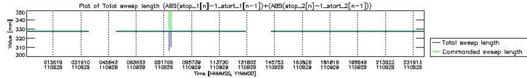
mipas_daily_report_level0_KSPT_L0_4504_N_20110929_6.PNG
