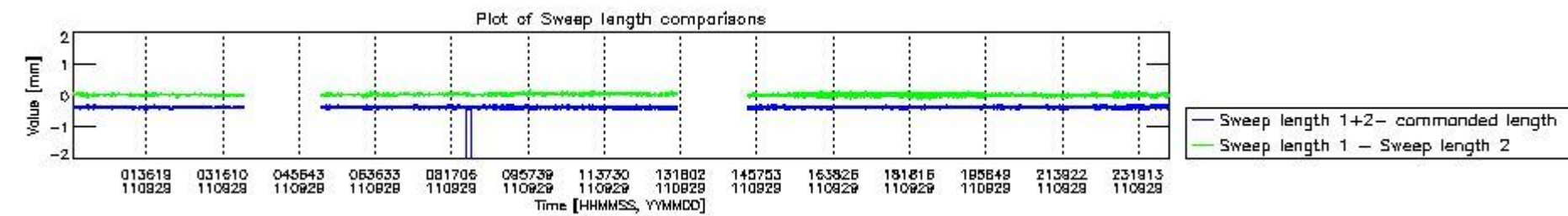
mipas_daily_report_level0_KSPT_L0_4504_N_20110929_8.PNG
