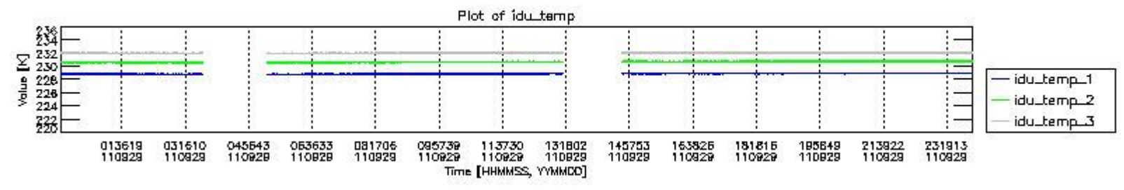
mipas_daily_report_level0_KSPT_L0_4504_N_20110929_2.PNG
