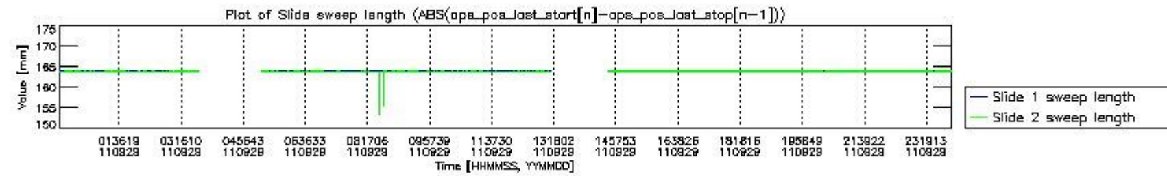
mipas_daily_report_level0_KSPT_L0_4504_N_20110929_7.PNG
