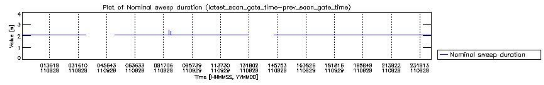
mipas_daily_report_level0_KSPT_L0_4504_N_20110929_3.PNG
