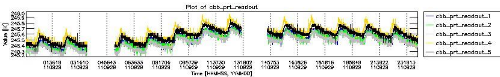
mipas_daily_report_level0_KSPT_L0_4504_N_20110929_9.PNG
