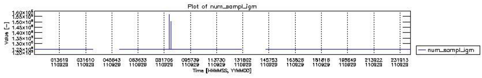
mipas_daily_report_level0_KSPT_L0_4504_N_20110929_0.PNG
