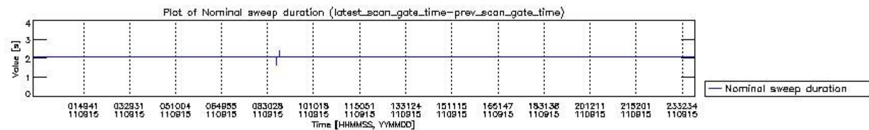
mipas_daily_report_level0_KSPT_L0_4504_N_20110915_4.PNG
