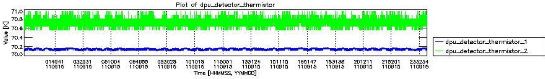
mipas_daily_report_level0_KSPT_L0_4504_N_20110915_3.PNG
