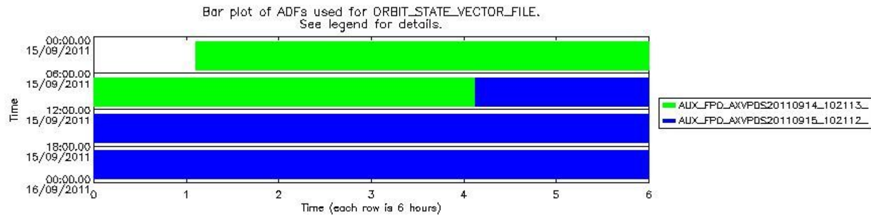
mipas_daily_report_level0_KSPT_L0_4504_N_20110915_13.PNG
