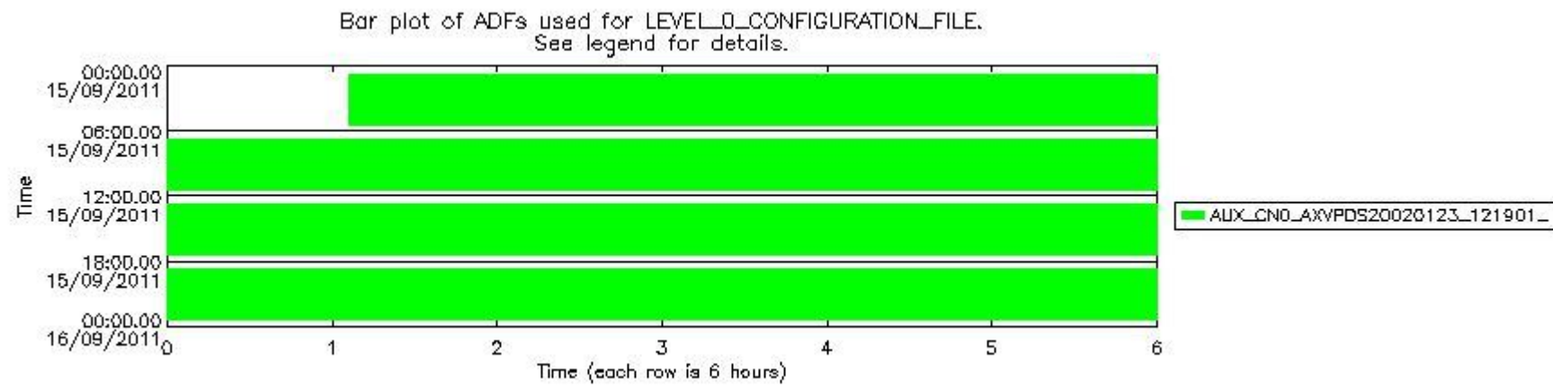
mipas_daily_report_level0_KSPT_L0_4504_N_20110915_12.PNG
