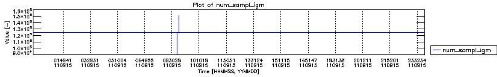
mipas_daily_report_level0_KSPT_L0_4504_N_20110915_0.PNG
