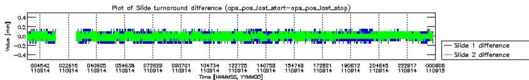
mipas_daily_report_level0_KSPT_L0_4504_N_20110914_5.PNG
