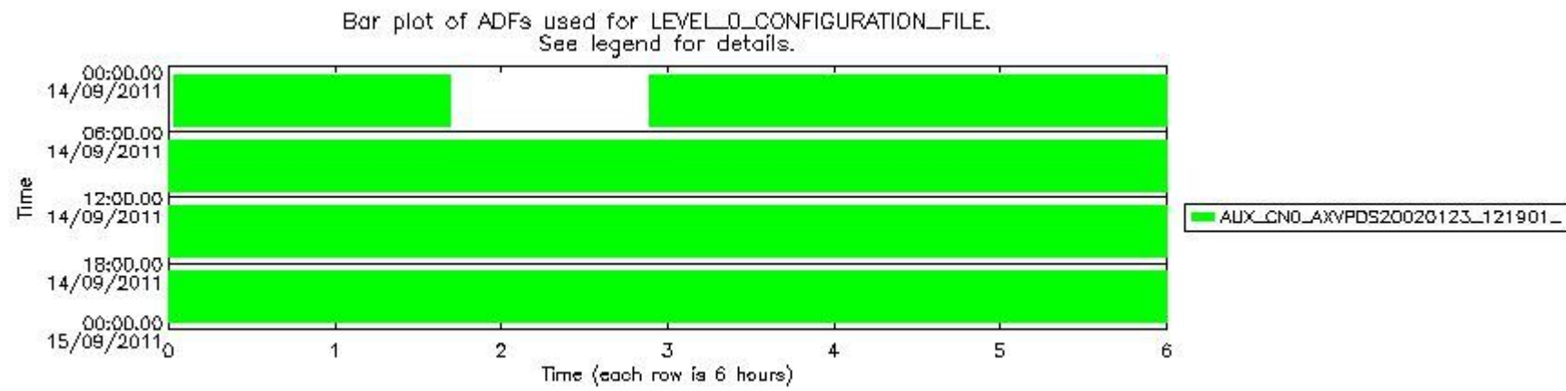
mipas_daily_report_level0_KSPT_L0_4504_N_20110914_12.PNG
