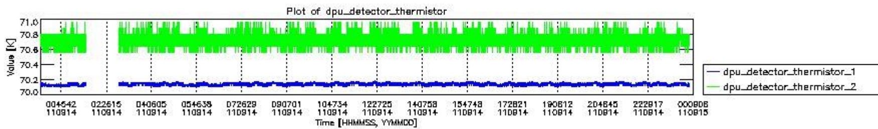
mipas_daily_report_level0_KSPT_L0_4504_N_20110914_3.PNG
