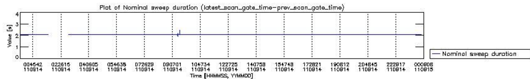
mipas_daily_report_level0_KSPT_L0_4504_N_20110914_4.PNG
