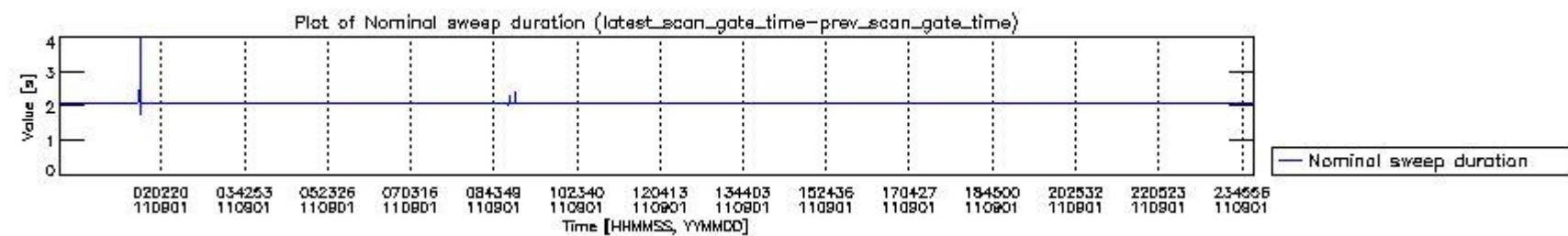
mipas_daily_report_level0_KSPT_L0_4504_N_20110901_4.PNG
