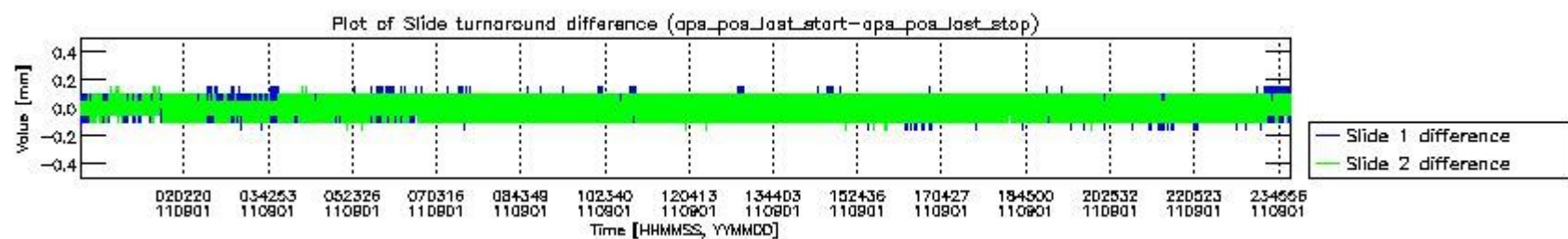
mipas_daily_report_level0_KSPT_L0_4504_N_20110901_5.PNG
