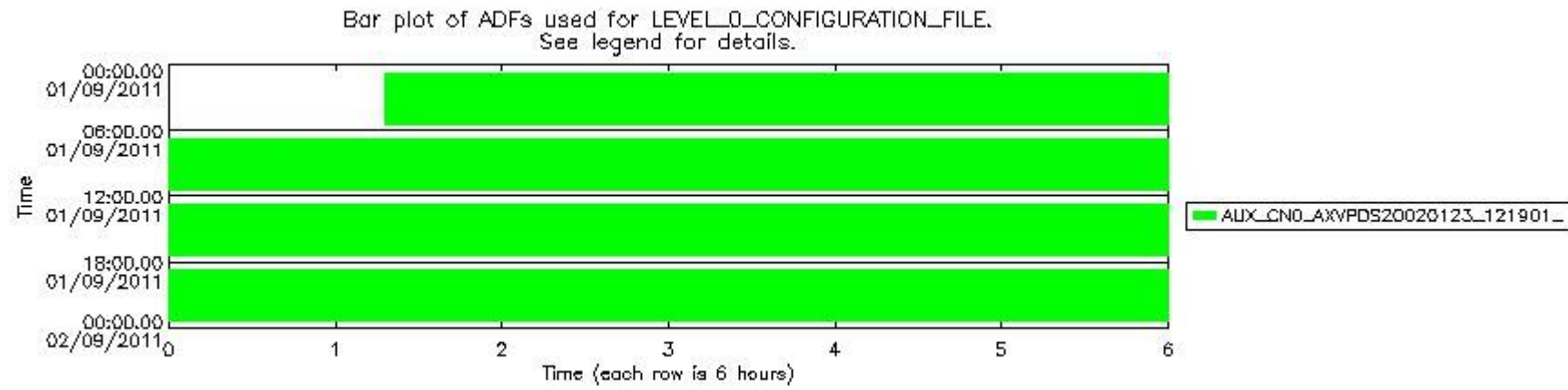
mipas_daily_report_level0_KSPT_L0_4504_N_20110901_12.PNG
