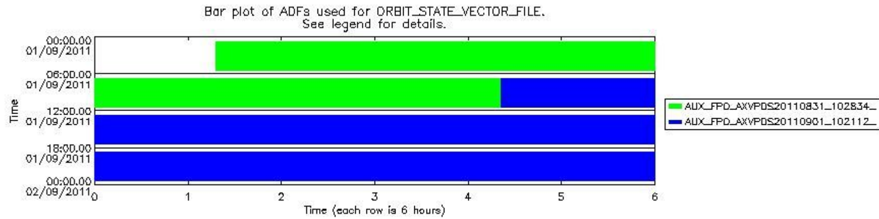
mipas_daily_report_level0_KSPT_L0_4504_N_20110901_13.PNG
