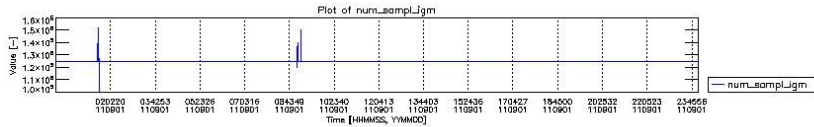
mipas_daily_report_level0_KSPT_L0_4504_N_20110901_0.PNG
