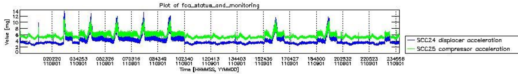
mipas_daily_report_level0_KSPT_L0_4504_N_20110901_10.PNG
