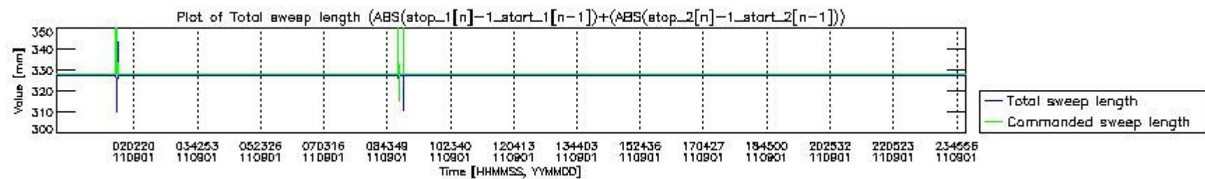
mipas_daily_report_level0_KSPT_L0_4504_N_20110901_6.PNG
