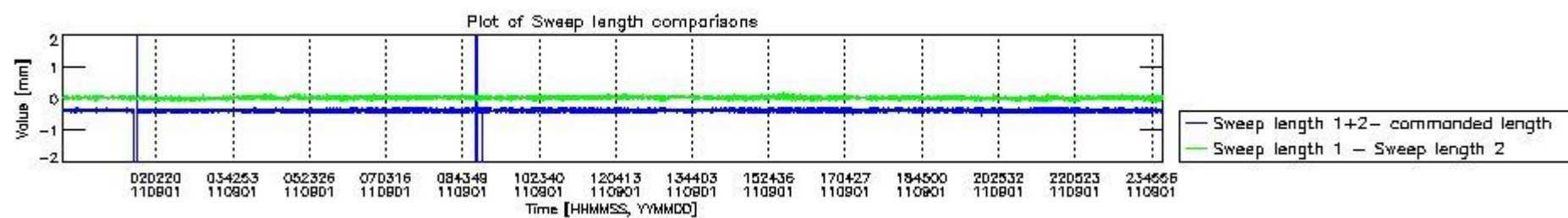
mipas_daily_report_level0_KSPT_L0_4504_N_20110901_8.PNG
