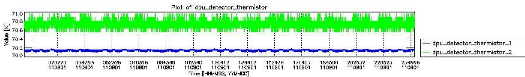
mipas_daily_report_level0_KSPT_L0_4504_N_20110901_3.PNG
