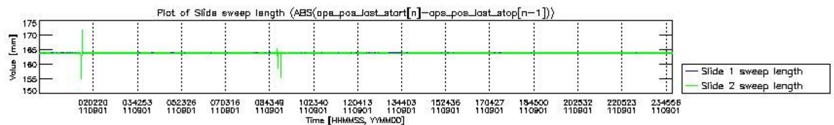
mipas_daily_report_level0_KSPT_L0_4504_N_20110901_7.PNG
