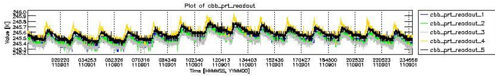
mipas_daily_report_level0_KSPT_L0_4504_N_20110901_9.PNG
