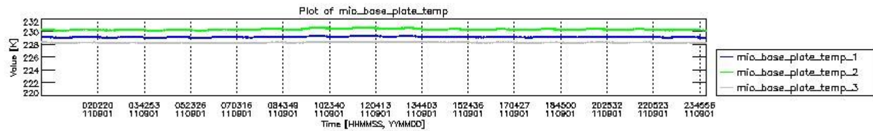
mipas_daily_report_level0_KSPT_L0_4504_N_20110901_1.PNG
