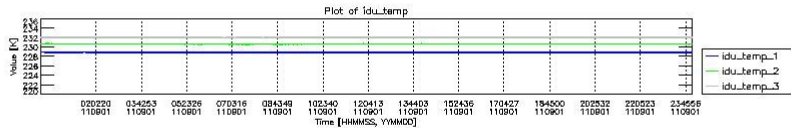
mipas_daily_report_level0_KSPT_L0_4504_N_20110901_2.PNG
