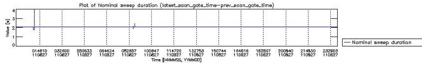
mipas_daily_report_level0_KSPT_L0_4504_N_20110827_4.PNG
