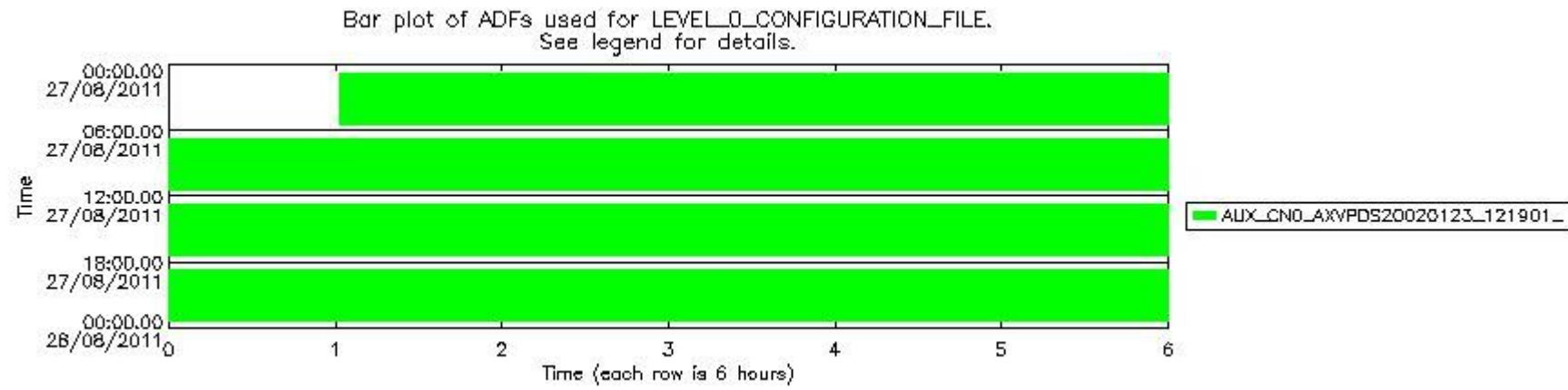
mipas_daily_report_level0_KSPT_L0_4504_N_20110827_12.PNG
