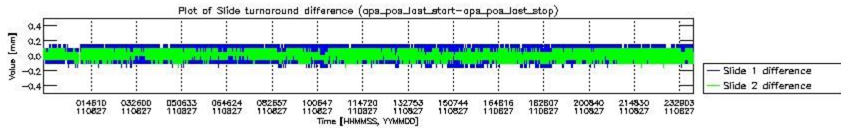
mipas_daily_report_level0_KSPT_L0_4504_N_20110827_5.PNG
