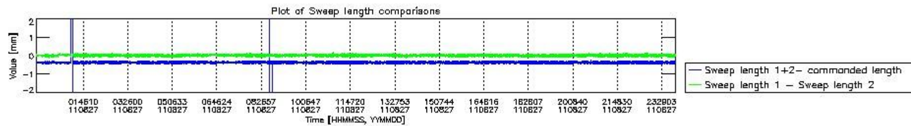
mipas_daily_report_level0_KSPT_L0_4504_N_20110827_8.PNG
