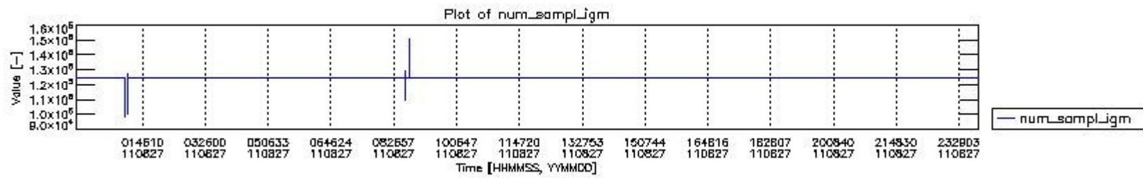
mipas_daily_report_level0_KSPT_L0_4504_N_20110827_0.PNG
