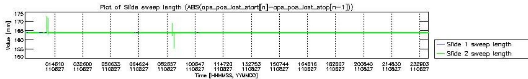
mipas_daily_report_level0_KSPT_L0_4504_N_20110827_7.PNG
