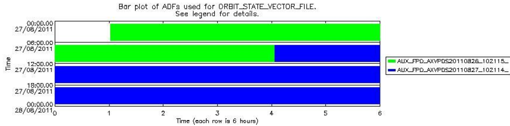
mipas_daily_report_level0_KSPT_L0_4504_N_20110827_13.PNG
