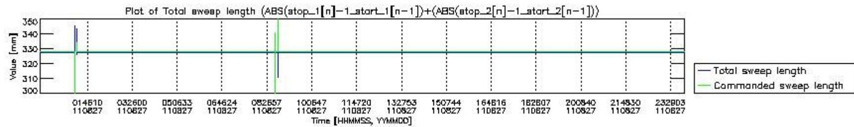
mipas_daily_report_level0_KSPT_L0_4504_N_20110827_6.PNG
