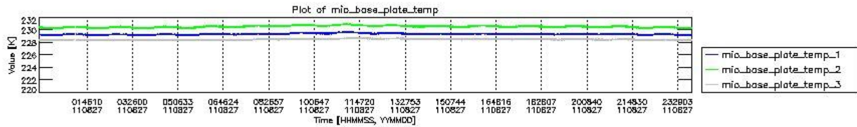
mipas_daily_report_level0_KSPT_L0_4504_N_20110827_1.PNG
