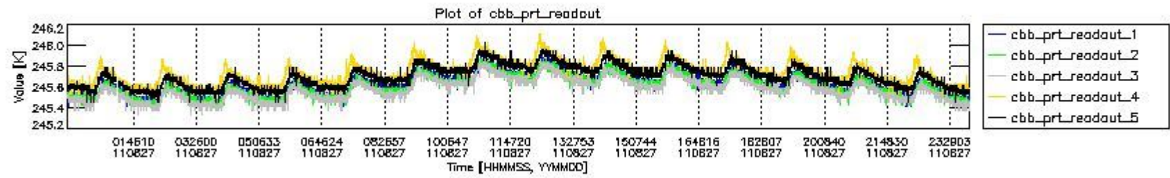
mipas_daily_report_level0_KSPT_L0_4504_N_20110827_9.PNG
