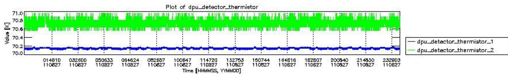
mipas_daily_report_level0_KSPT_L0_4504_N_20110827_3.PNG
