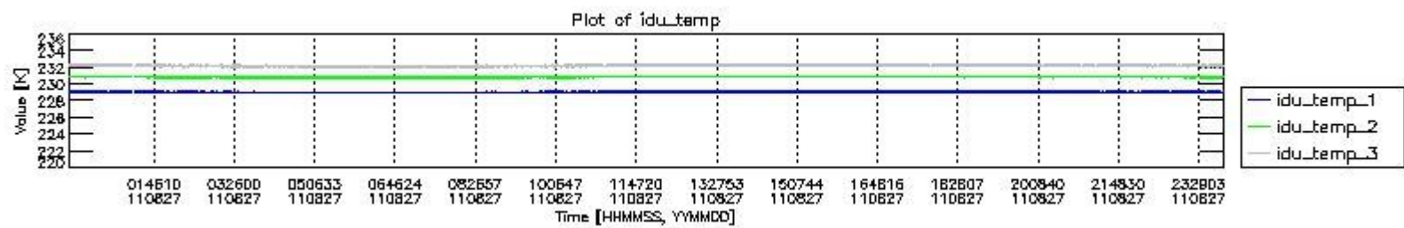
mipas_daily_report_level0_KSPT_L0_4504_N_20110827_2.PNG
