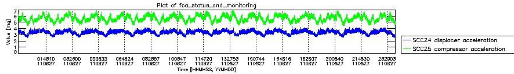
mipas_daily_report_level0_KSPT_L0_4504_N_20110827_10.PNG
