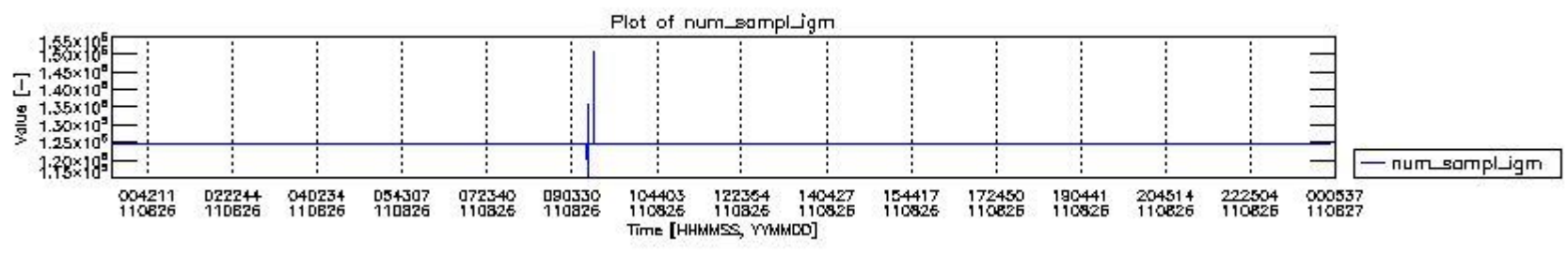
mipas_daily_report_level0_KSPT_L0_4504_N_20110826_0.PNG
