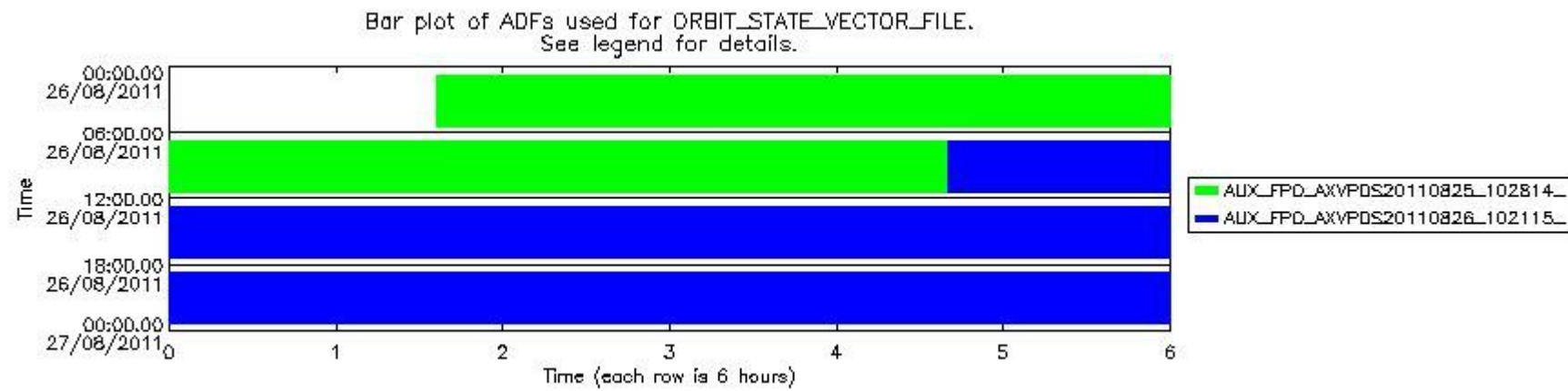
mipas_daily_report_level0_KSPT_L0_4504_N_20110826_13.PNG
