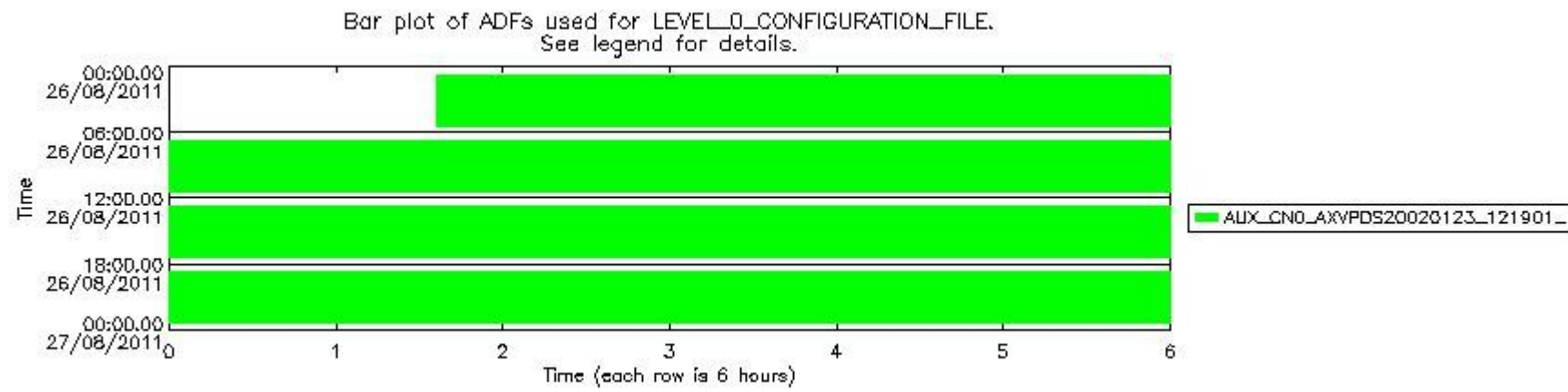
mipas_daily_report_level0_KSPT_L0_4504_N_20110826_12.PNG
