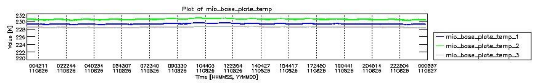
mipas_daily_report_level0_KSPT_L0_4504_N_20110826_1.PNG
