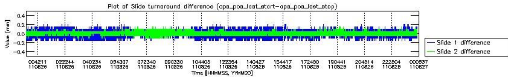
mipas_daily_report_level0_KSPT_L0_4504_N_20110826_5.PNG
