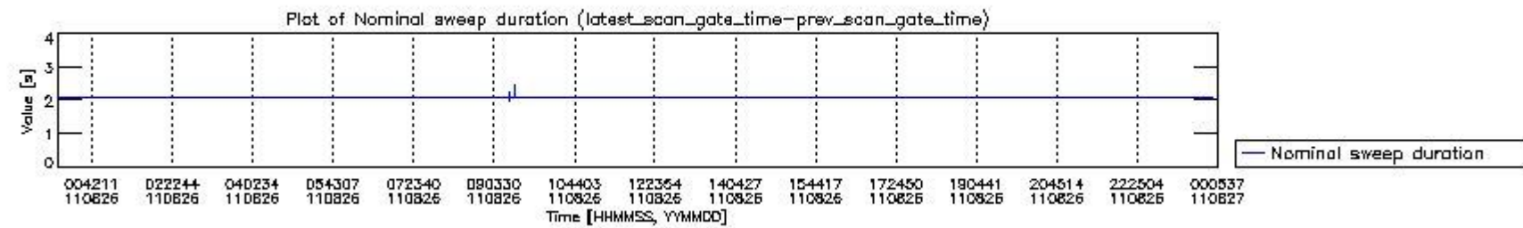
mipas_daily_report_level0_KSPT_L0_4504_N_20110826_4.PNG
