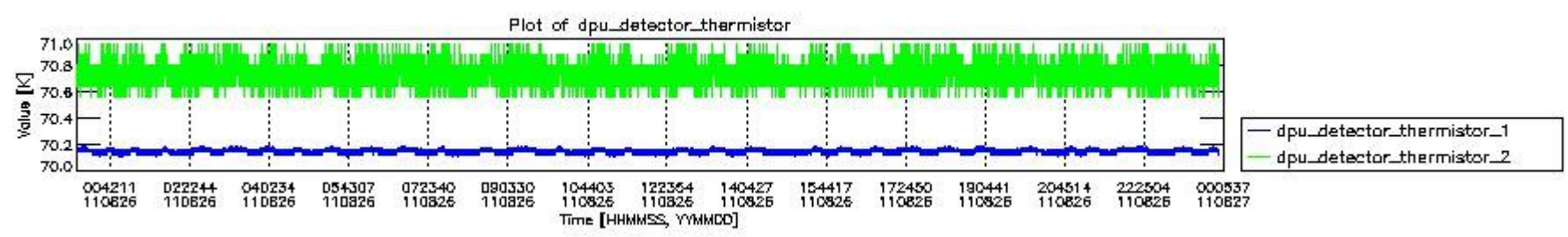
mipas_daily_report_level0_KSPT_L0_4504_N_20110826_3.PNG
