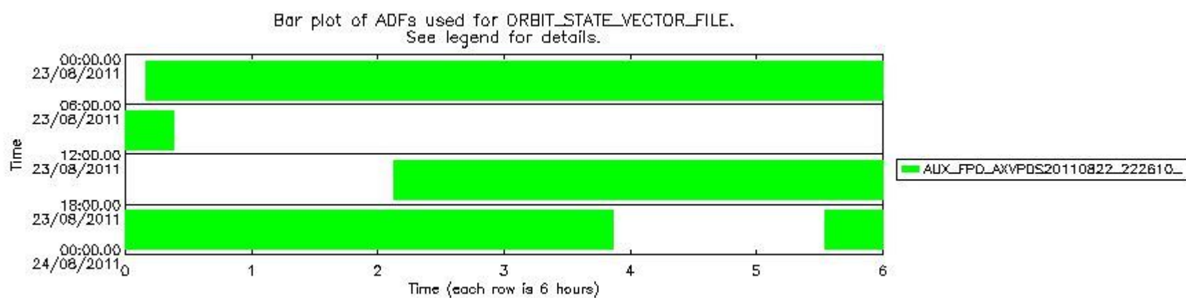
mipas_daily_report_level0_KSPT_L0_4504_N_20110823_13.PNG
