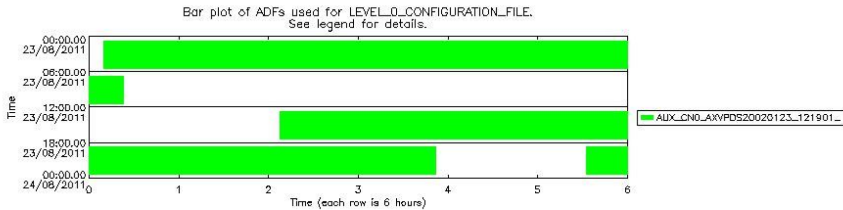
mipas_daily_report_level0_KSPT_L0_4504_N_20110823_12.PNG
