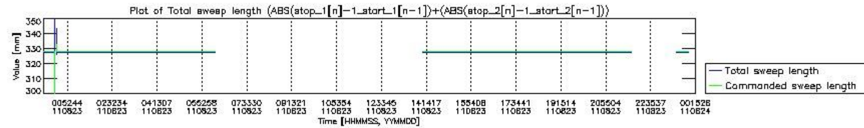
mipas_daily_report_level0_KSPT_L0_4504_N_20110823_6.PNG
