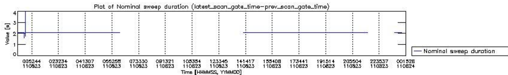
mipas_daily_report_level0_KSPT_L0_4504_N_20110823_4.PNG
