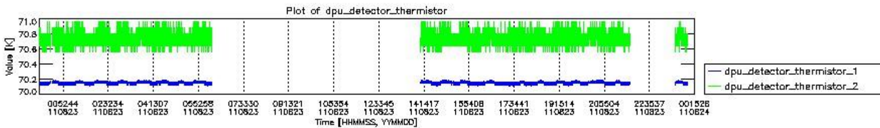
mipas_daily_report_level0_KSPT_L0_4504_N_20110823_3.PNG
