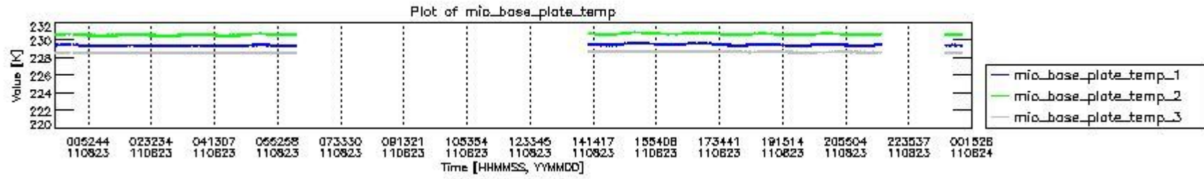
mipas_daily_report_level0_KSPT_L0_4504_N_20110823_1.PNG
