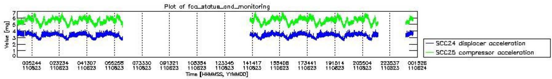
mipas_daily_report_level0_KSPT_L0_4504_N_20110823_10.PNG
