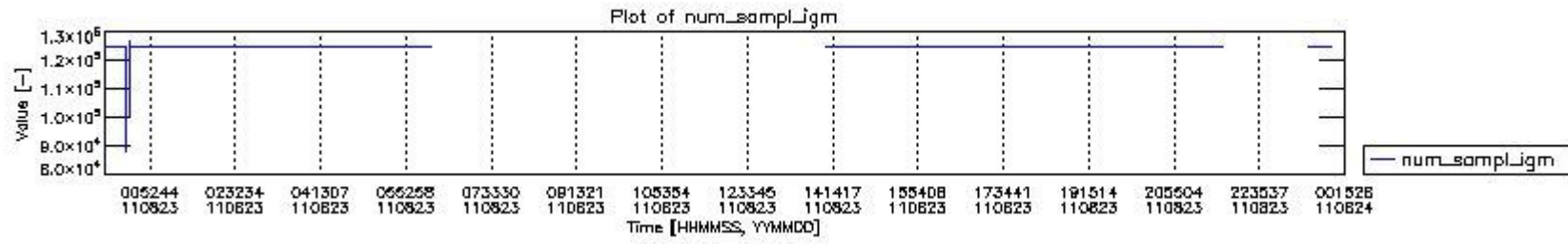
mipas_daily_report_level0_KSPT_L0_4504_N_20110823_0.PNG
