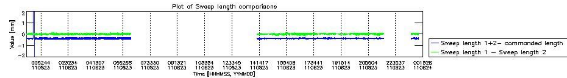
mipas_daily_report_level0_KSPT_L0_4504_N_20110823_8.PNG
