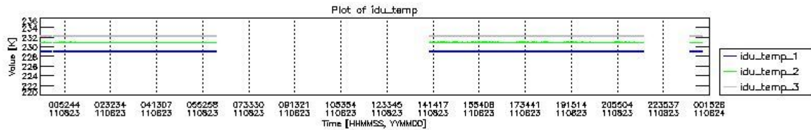
mipas_daily_report_level0_KSPT_L0_4504_N_20110823_2.PNG
