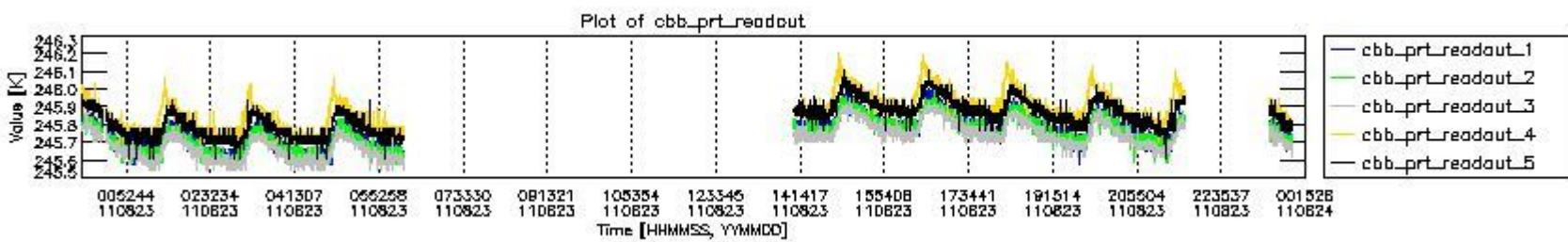
mipas_daily_report_level0_KSPT_L0_4504_N_20110823_9.PNG
