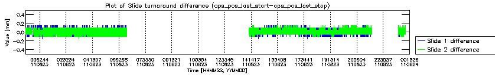
mipas_daily_report_level0_KSPT_L0_4504_N_20110823_5.PNG
