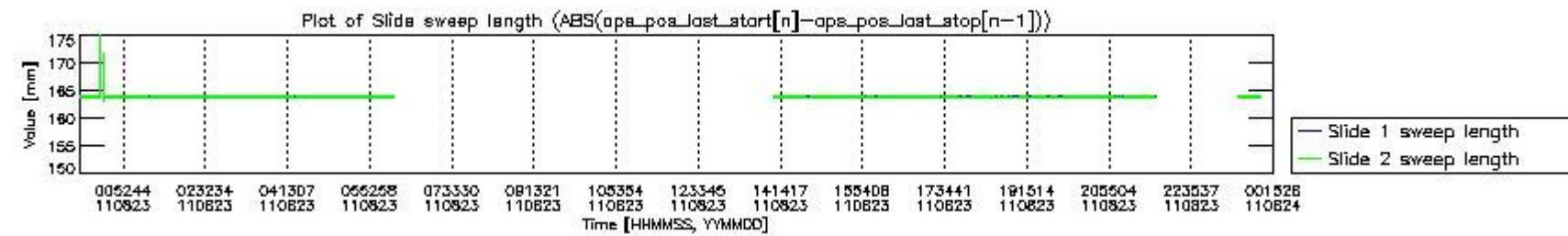
mipas_daily_report_level0_KSPT_L0_4504_N_20110823_7.PNG
