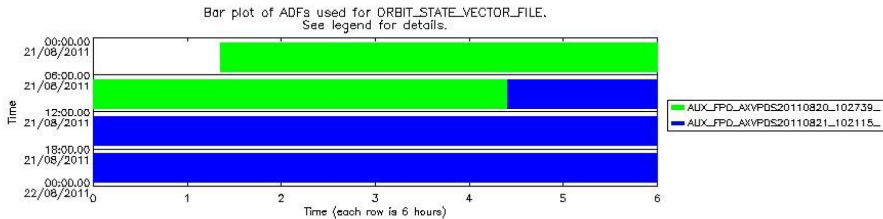
mipas_daily_report_level0_KSPT_L0_4504_N_20110821_13.PNG
