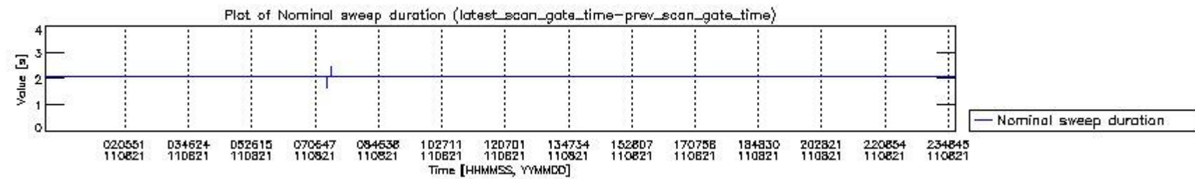
mipas_daily_report_level0_KSPT_L0_4504_N_20110821_4.PNG
