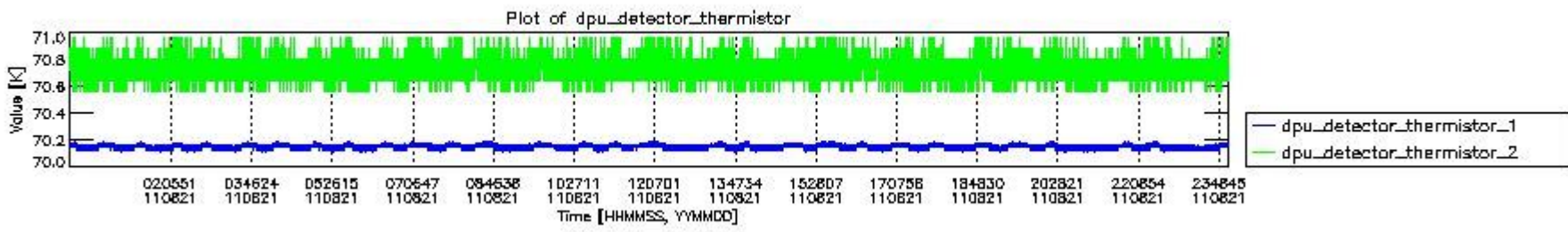
mipas_daily_report_level0_KSPT_L0_4504_N_20110821_3.PNG
