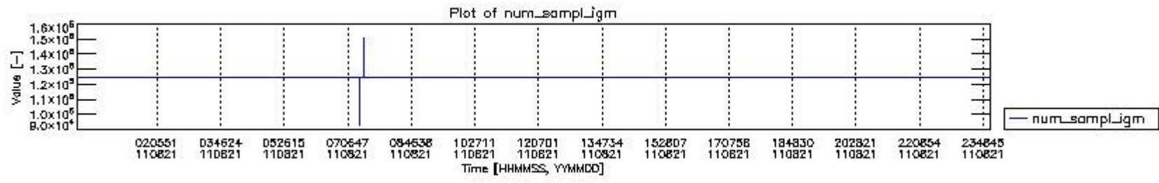
mipas_daily_report_level0_KSPT_L0_4504_N_20110821_0.PNG
