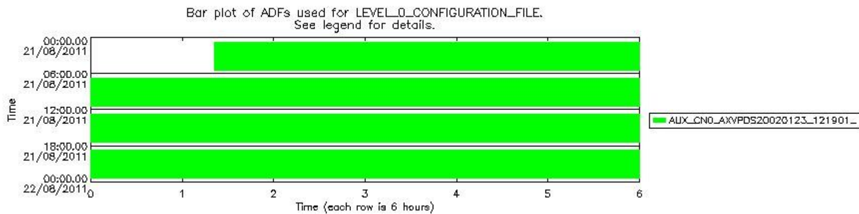
mipas_daily_report_level0_KSPT_L0_4504_N_20110821_12.PNG
